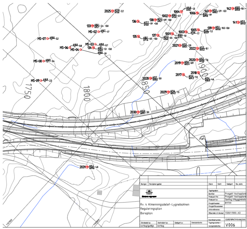
Figur 56: Borepunkt for geotekniske undersøkelser
