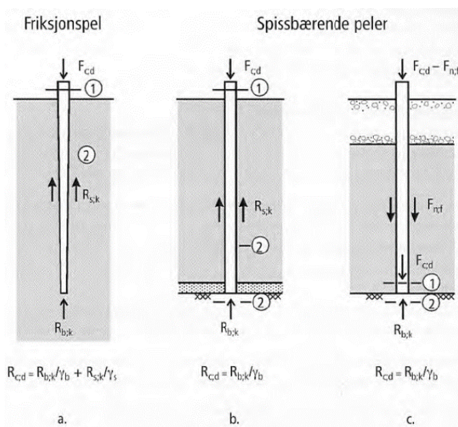
Figur 17: illustrasjoner av friksjonspeler, spissbærende peler med og uten konsolidert masse (Statens Vegvesen, 2022)
