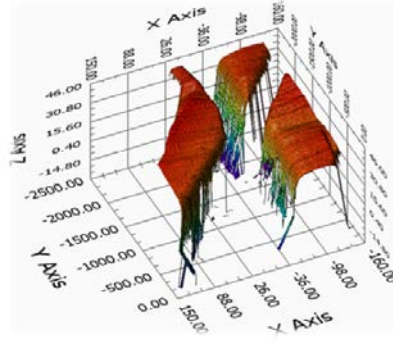
Figur 11: Inspeksjonsrobot og eksempel på måleresultat ©2014 Loccioni Group
