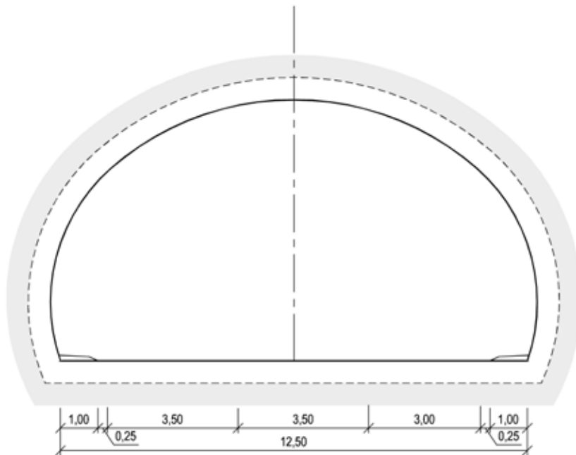
Figur V1.8 Tunnelprofil T12,5 (mål i m)
