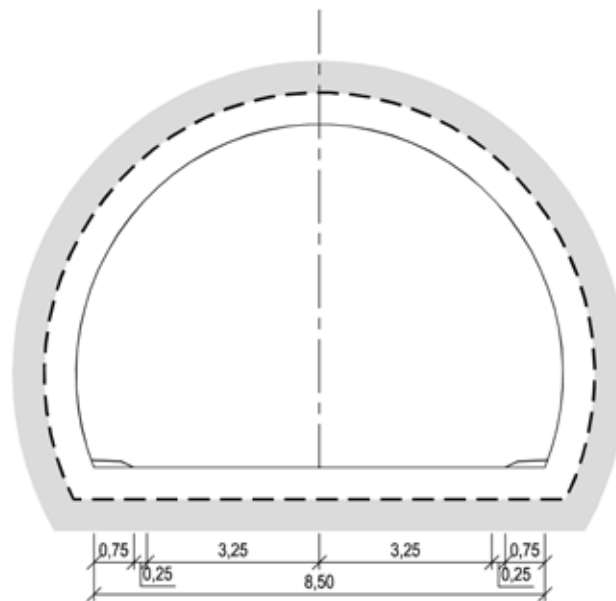
Figur V1.5 Tunnelprofil T8,5 (mål i m)
