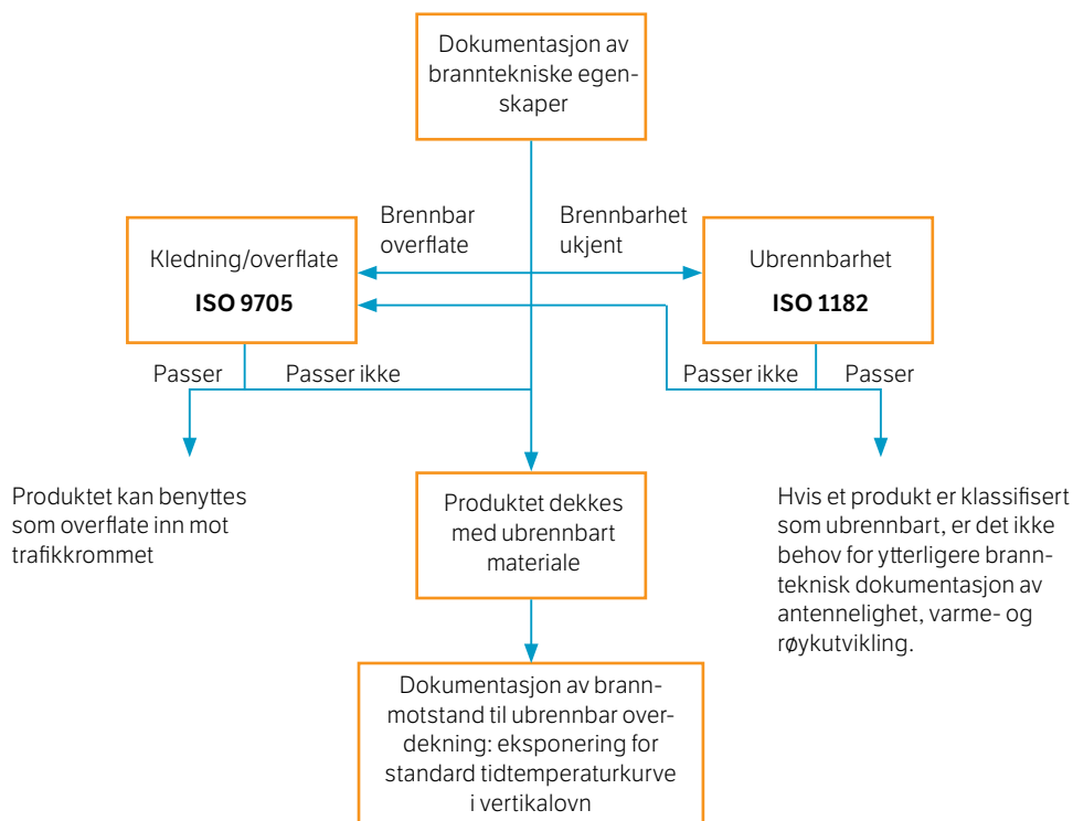
Figur 4.8 Diagram for dokumentasjon av branntekniske egenskaper for konstruksjoner benyttet i tunneler (NS-EN ISO 1182 [23], ISO 9705 [24])
