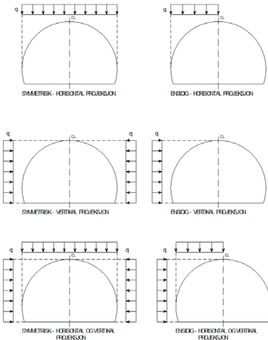
Figur 7.2 Generell variabel last – lasttilfeller
