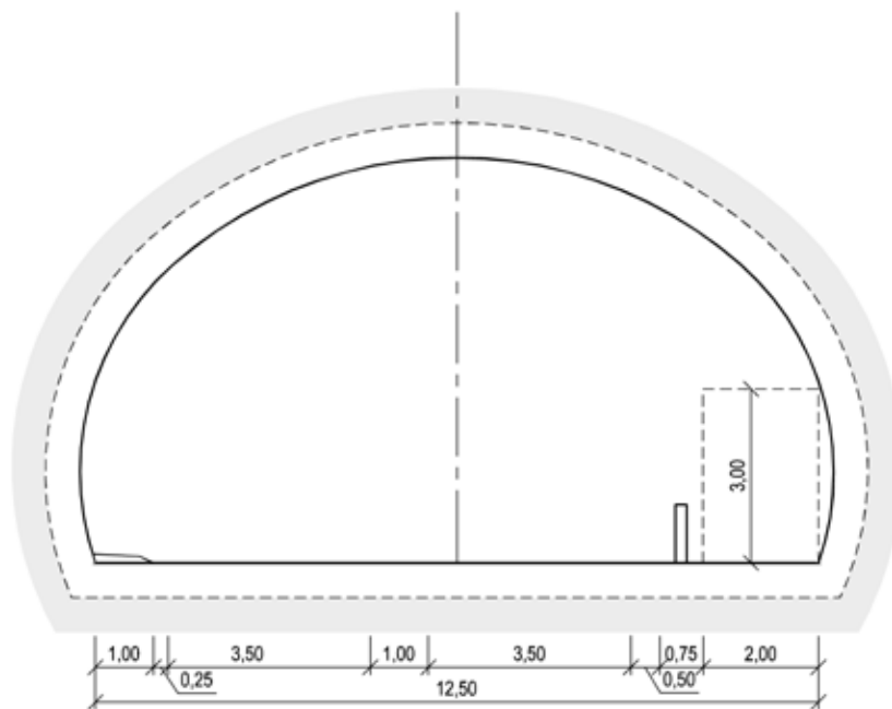
Figur V1.15 Tunnelprofil T12,5GS (mål i m)
