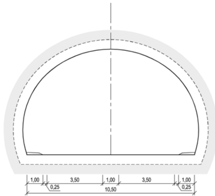
Figur V1.9 Tunnelprofil T10,5 (mål i m)
