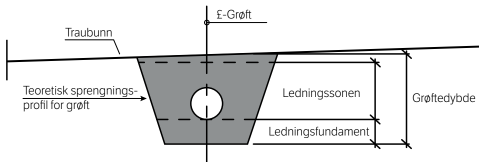
Figur 8.1 Prinsippskisse, grøftedybde
