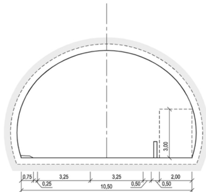
Figur V1.14 Tunnelprofil T10,5GS (mål i m)
