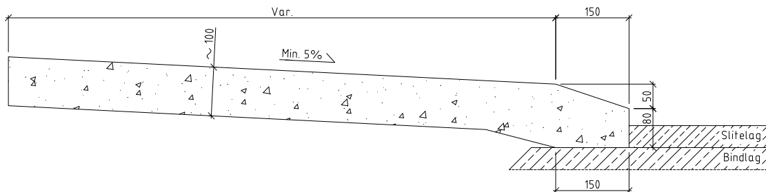
Figur 3.4 Eksempel på kantstein og betongsåle, her vist som plasstøpt løsning. Mål i mm.
