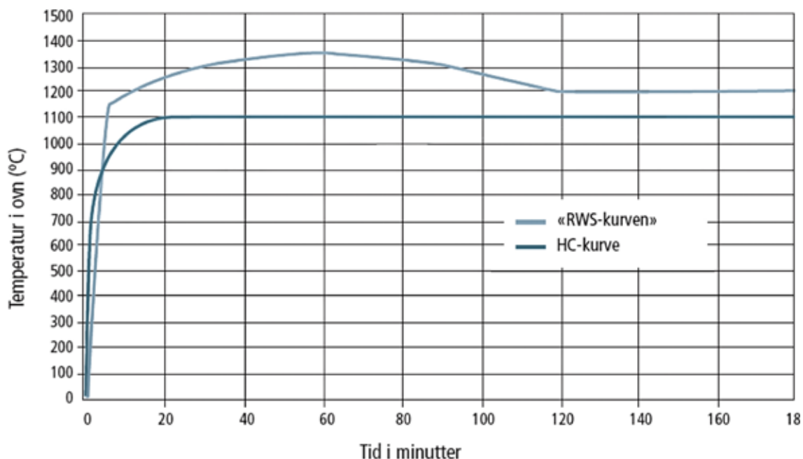
Figur 4.7 Standard tid-temperaturkurver som benyttes ved branndimensjonering. – RWS-kurven [20] – Hydrocarbon- (HC-) kurven definert i ISO 834-3 [21] og NS-EN 1363-2 [22].
