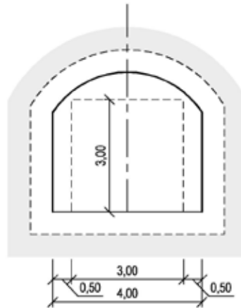
Figur V1.1 Tunnelprofil T4 (mål i m)
