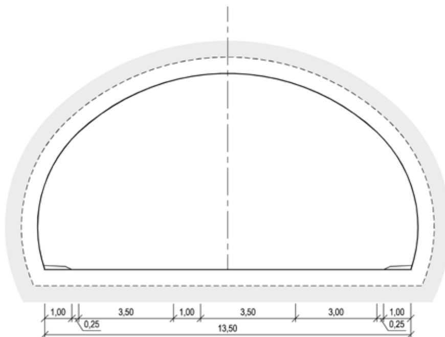
Figur V1.10 Tunnelprofil T13,5 (mål i m)
