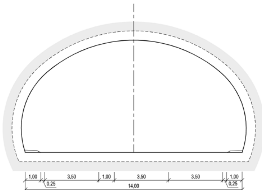
Figur V1.12 Tunnelprofil T14 (mål i m)
