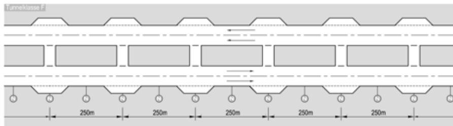
Havarinisjer for hver 250 meter for hvert løp – Tverrforbindelser for hver 250 meter N Nødstasjoner per løp hver 125 meter
