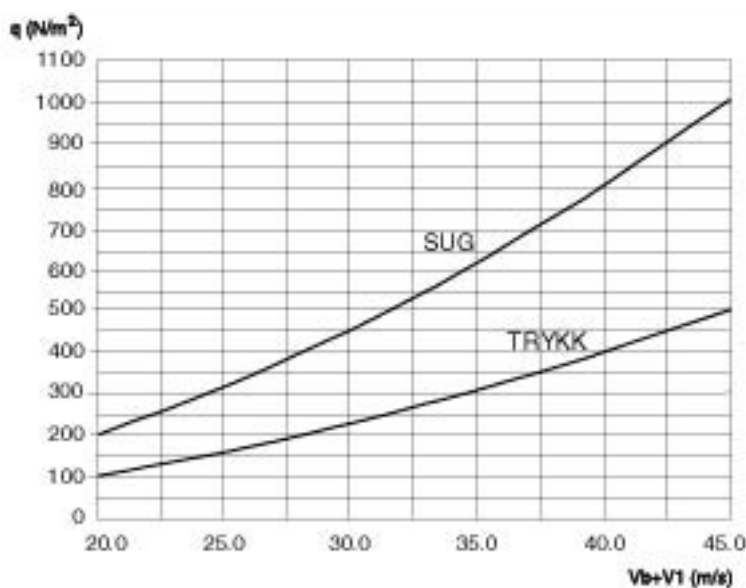
Figur 7.1 Variasjon av trykk/sug med total lufthastighet
