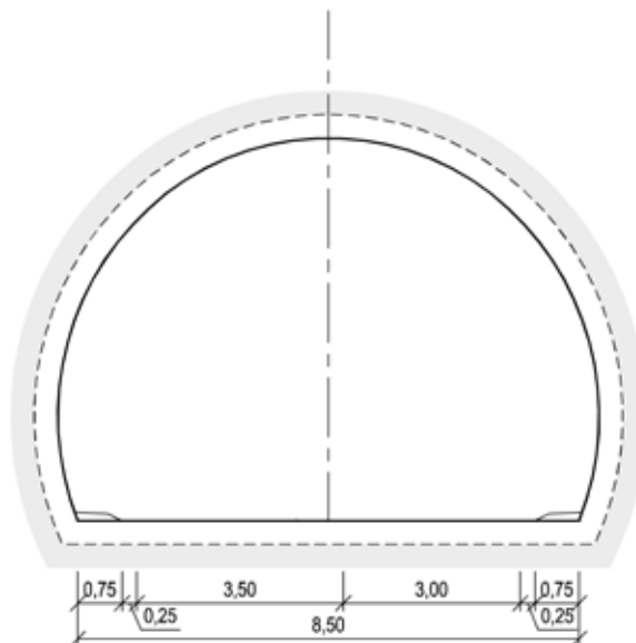
Figur V1.4 Tunnelprofil T8,5 (mål i m)
