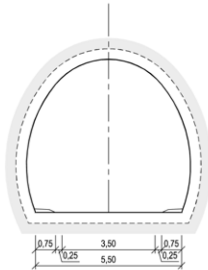
Figur V1.3 Tunnelprofil T5,5 (mål i m)
