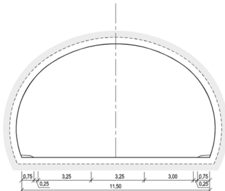
Figur V1.6 Tunnelprofil T11,5 (mål i m)
