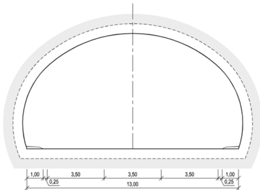
Figur V1.11 Tunnelprofil T13 (mål i m)
