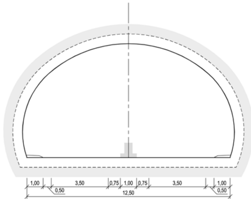
Figur V1.13 Tunnelprofil T12,5 (mål i m).
