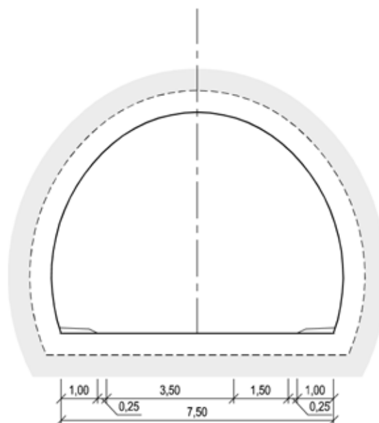
Figur V1.2 Tunnelprofil T7,5 (mål i m)
