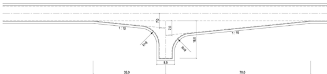
Figur 3.6 Eksempel på utforming av snunisje.
