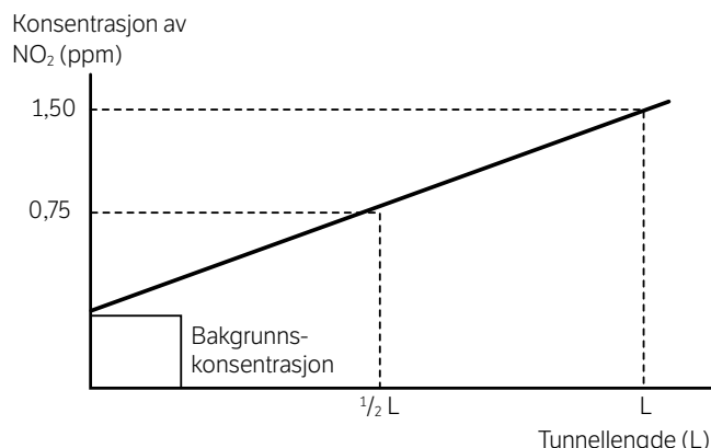
Figur 9.1 Dimensjonerende NO 2 -konsentrasjon i tunneler
