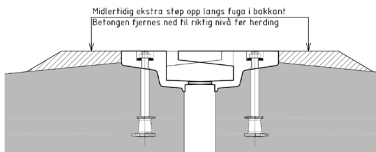
Figur 6 Viktig del av støpeprosedyren
