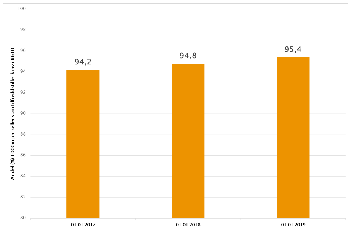
Figur 8. Andelen 1000m parseller på rv i Rø som tilfredsstillende krav til tilstand i R610 («ny tilstandsindikator»)
