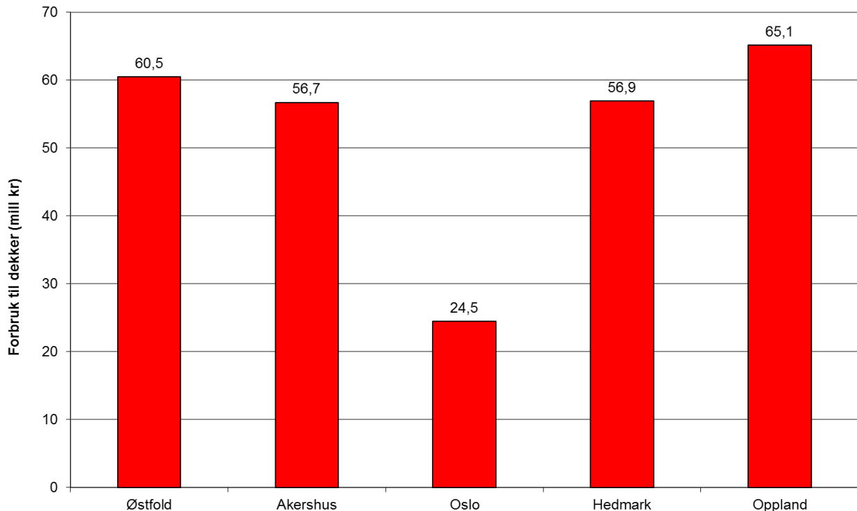
Figur 2. Forbruk på riksveger i 2018
