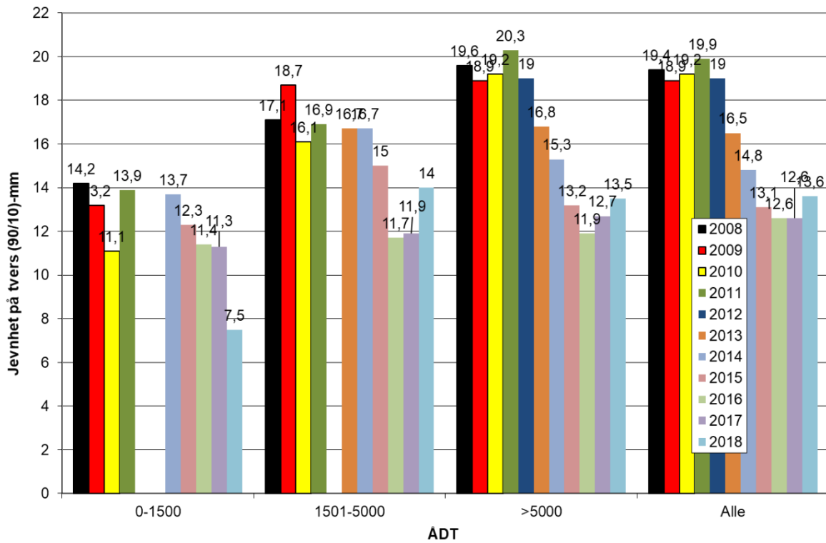
Figur V2-9. Jevnhet på tvers (90/10) på riksvegnettet i Oslo
