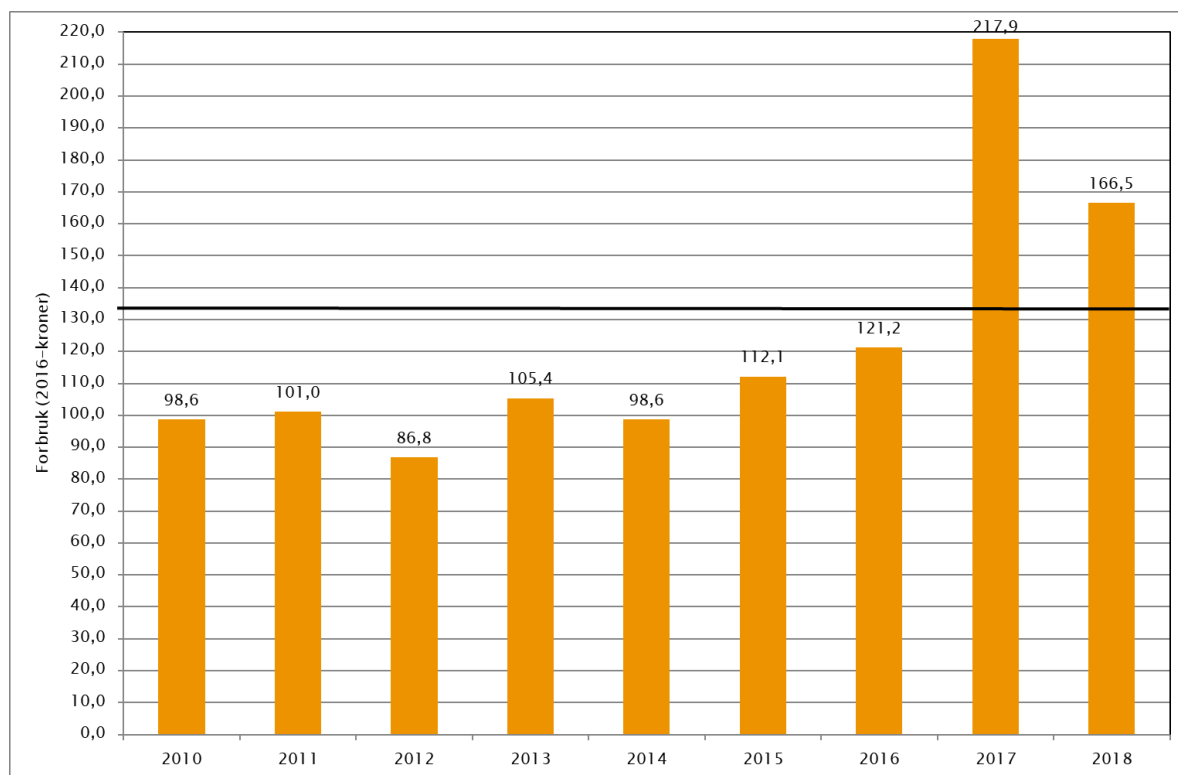
Figur 41. Forbruk på fylkesveger i Oppland i perioden 2010-2018 (omregnet til 2018-kroner) (horisontal strek er beregnet budsjettbehov iht. /1/ for å unngå økt etterslep)
