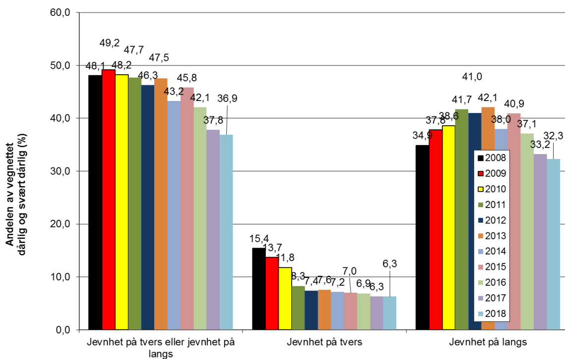
Figur 17. Utviklingen av andelen dårlig og svært dårlig (jevnhhet på tvers > 18mm og jevnhet på langs IRI > 3,1) på fylkesveger i Rø
