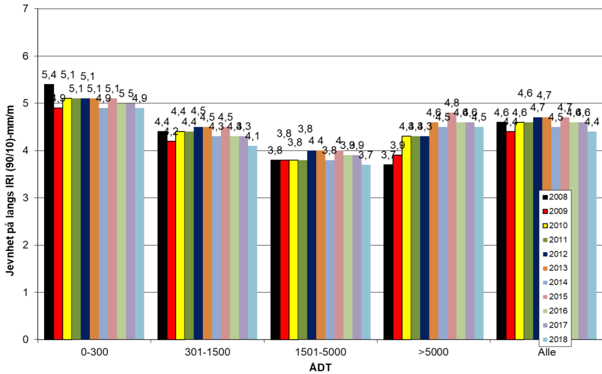
Figur 32. Jevnhet på langs IRI (90/10) på fylkesveger i Hedmark
