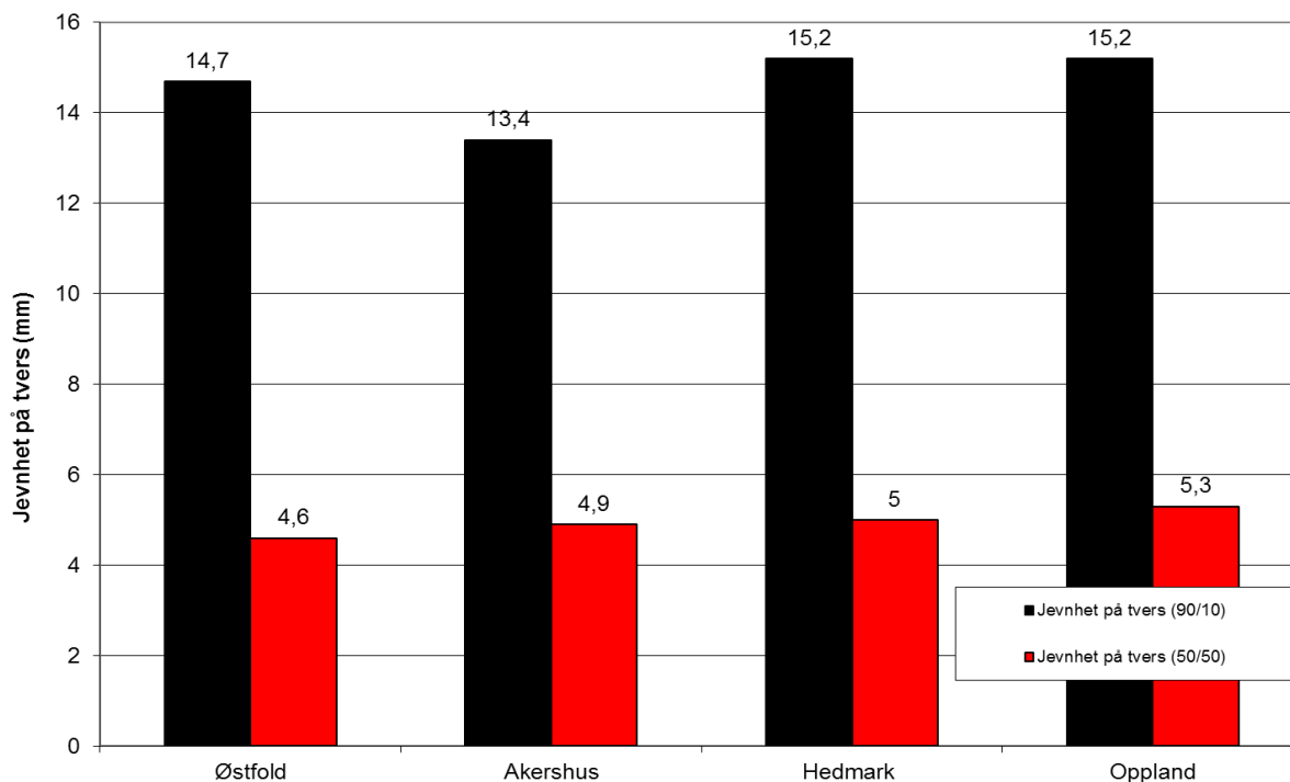
Figur 15. Jevnhet på tvers for fylkesveger per 1/1-2019
