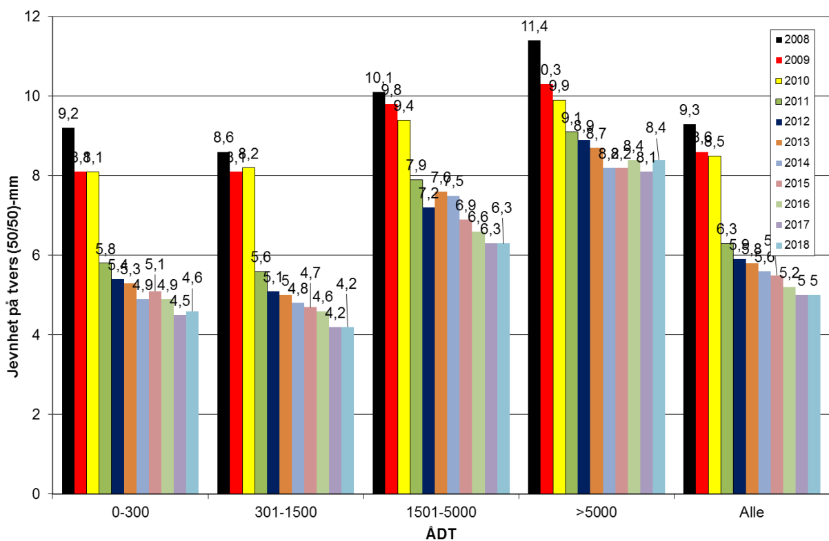
Figur 12. Jevnhet på tvers (50/50) for fylkesveger i Rø
