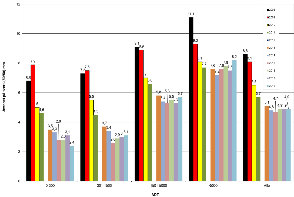
Figur 25. Jevnhet på tvers (50/50) på fylkesveger i Akershus
