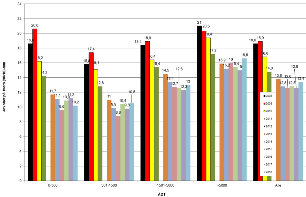
Figur 24. Jevnhet på tvers (90/10) på fylkesveger i Akershus
