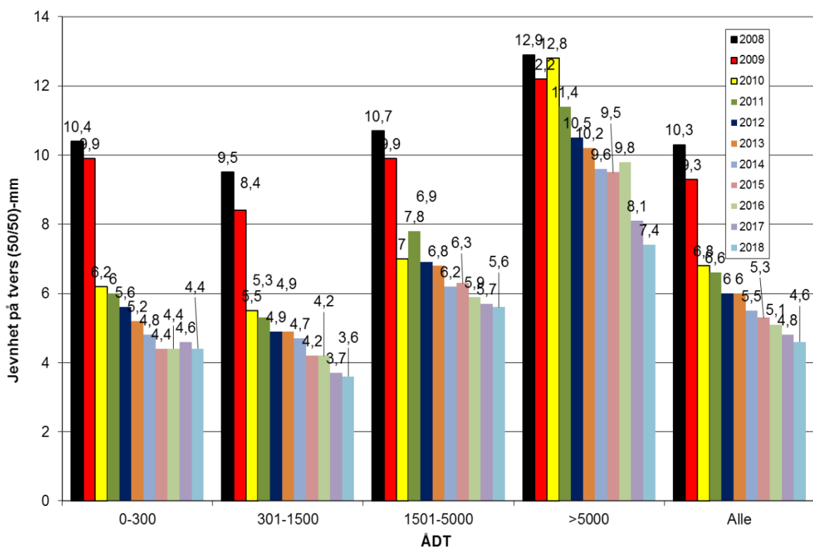
Figur 19. Jevnhet på tvers (50/50) på fylkesveger i Østfold
