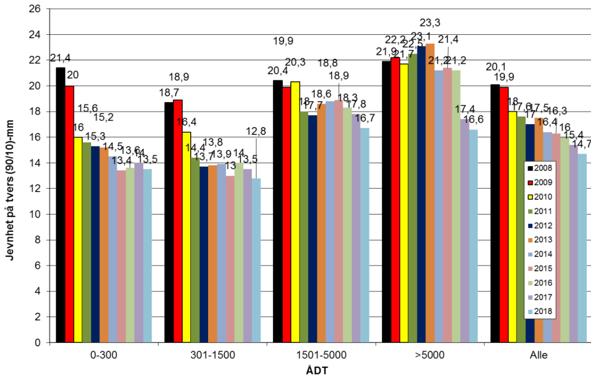
Figur 18. Jevnhet på tvers (90/10) på fylkesveger i Østfold
