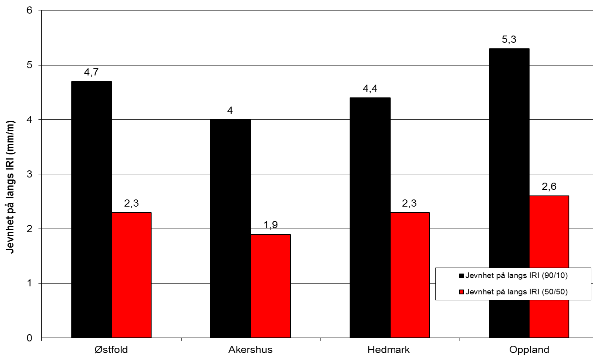
Figur 16. Jevnhet på langs IRI for fylkesveger per 1/1-2019
