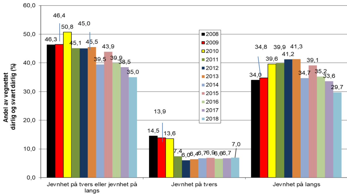
Figur 34. Utviklingen av andelen dårlig og svært dårlig (jevnhet på tvers > 18mm og jevnhet på langs IRI > 3,1) på fylkesveger i Hedmark.
