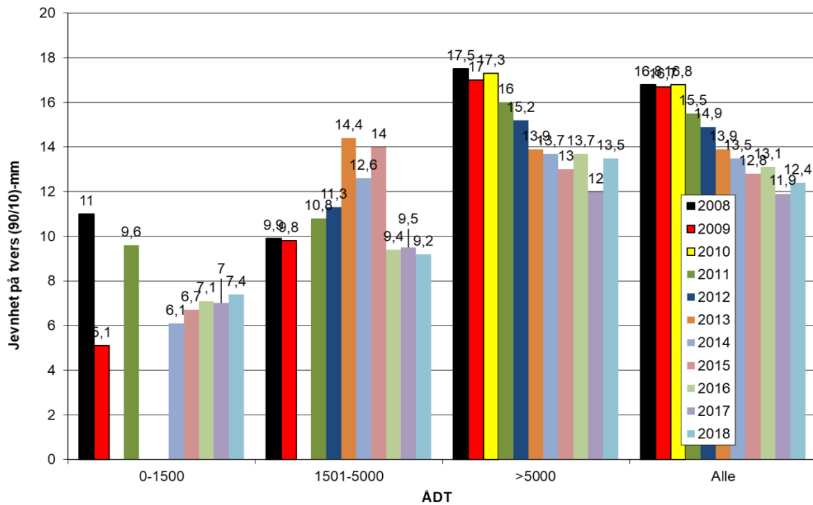
Figur V2-5. Jevnhet på tvers (90/10) på riksvegnettet i Akershus
