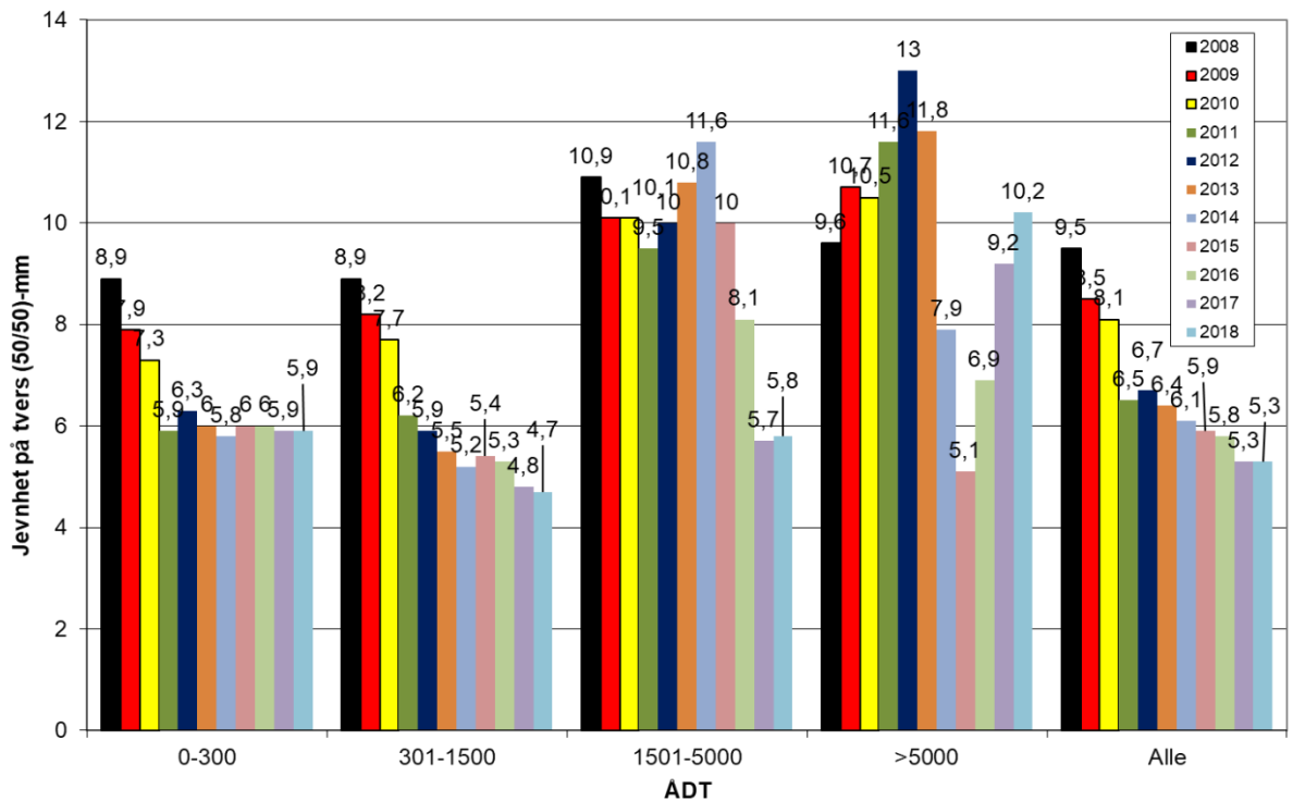
Figur 37. Jevnhet på tvers (50/50) på fylkesveger i Oppland
