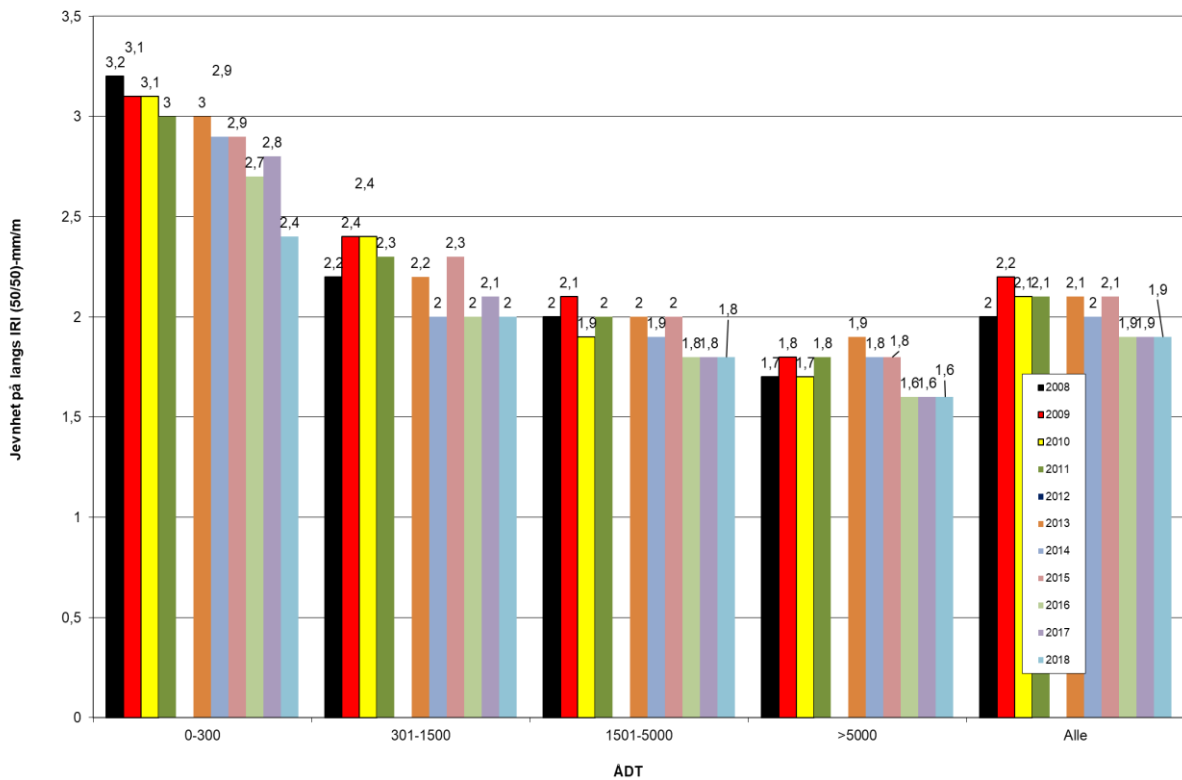
Figur 27. Jevnhet på langs IRI (50/50) på fylkesveger i Akershus
