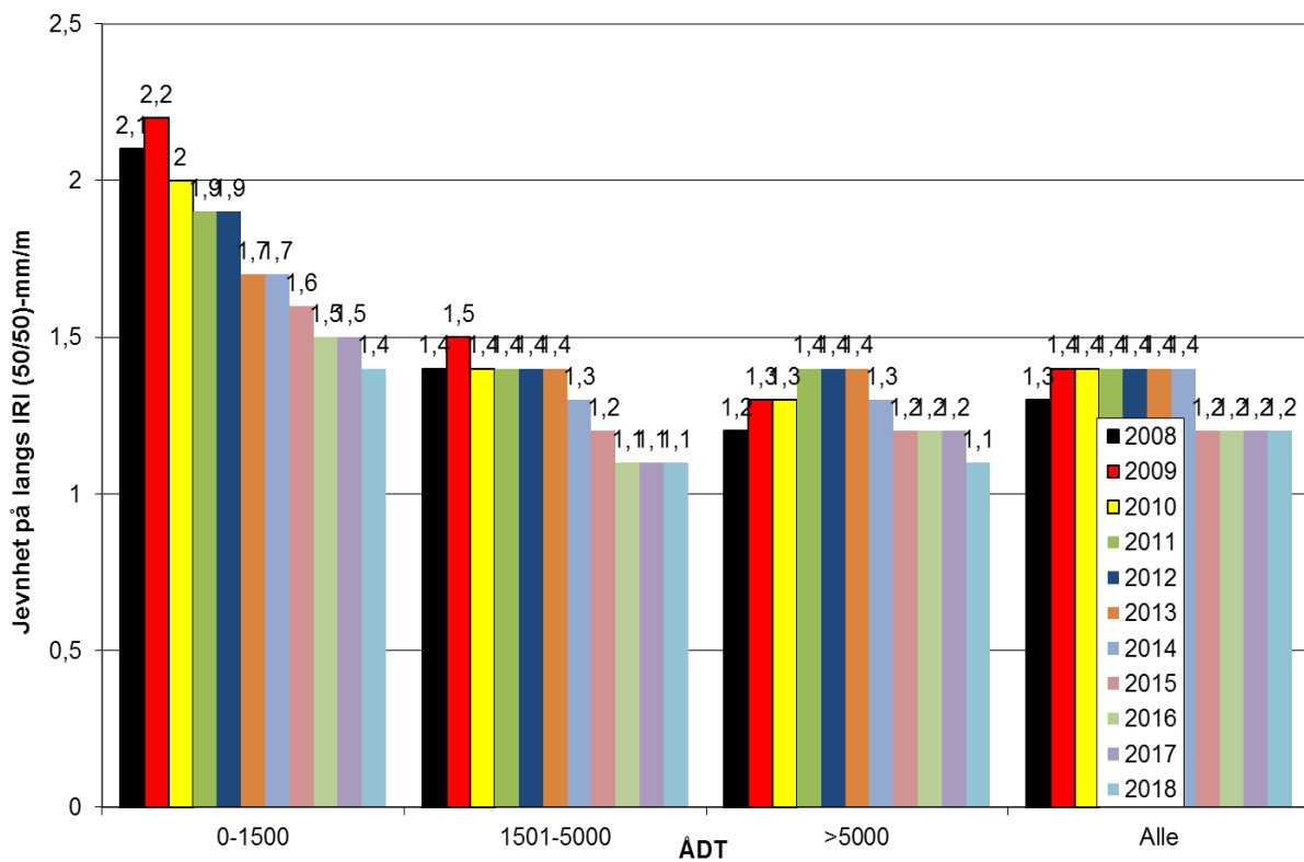
Figur 6. Utviklingen av jevnhet på langs IRI (50/50) på riksvegnettet i Rø
