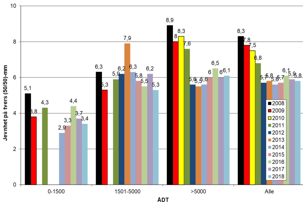
Figur V2-6. Jevnhet på tvers (50/50) på riksvegnettet i Akershus
