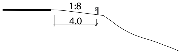
Figur 5-7. Høy fylling med rekkverk. Her er det anlagt en utvidet skulder med fresfelt.
