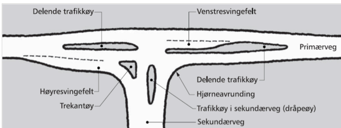
Figur E.1: Elementer i kanalisert kryss
