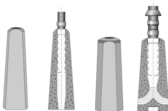
Betongfundament med låsering uten kabelinntak
