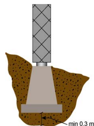
Betongfundament for mast og portal
