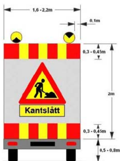
Figur 4. 3: Eksempel på varselpanel, normal størelse
