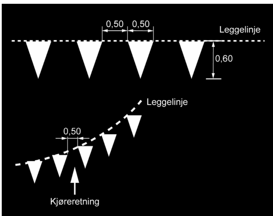
Figur 6.11: Skisse for vikelinjer
