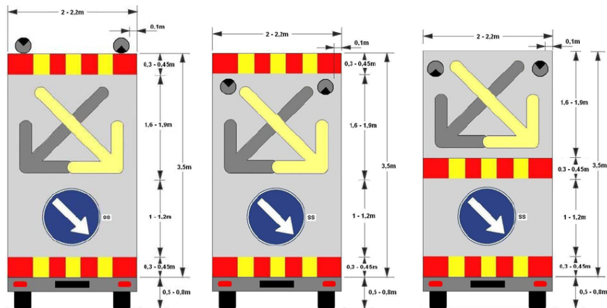
Figur 4. 4: Eksempel på varselpanel, stor størrelse
