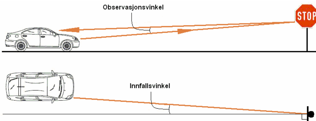
Figur 1. 3: Definisjon av observasjonsvinkel og innfallsvinkel (standard geometri).
