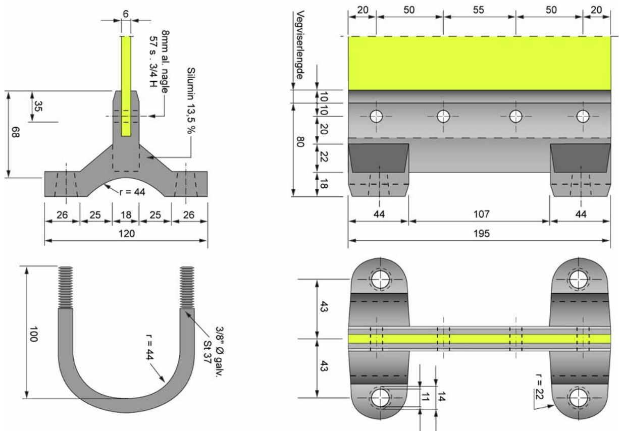
Figur 1. 17: Eksempel på vegviserfløy
