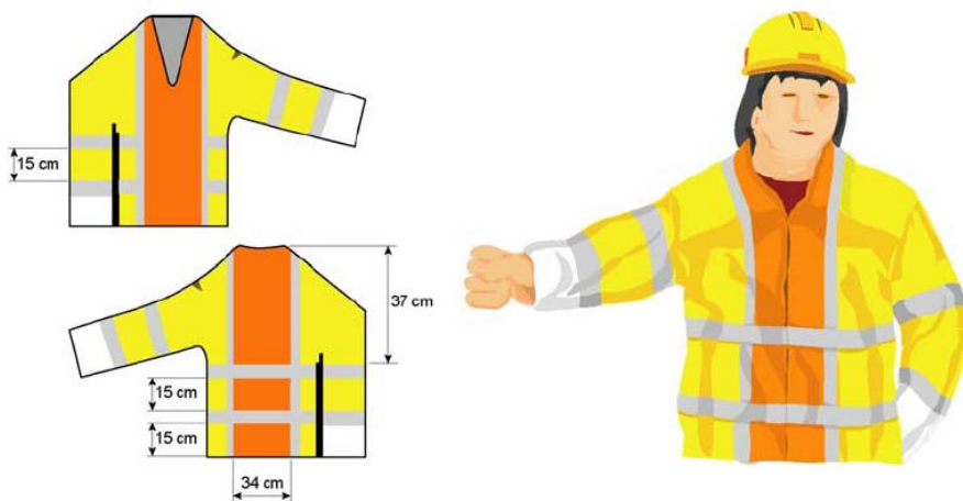
Figur 4. 16: Jakke for manuell dirigering (Mål for størrelse ”L”)
