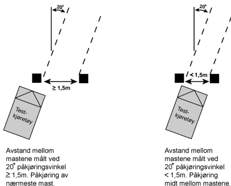
Figur 5.10 Krav til stolpeavstand.
