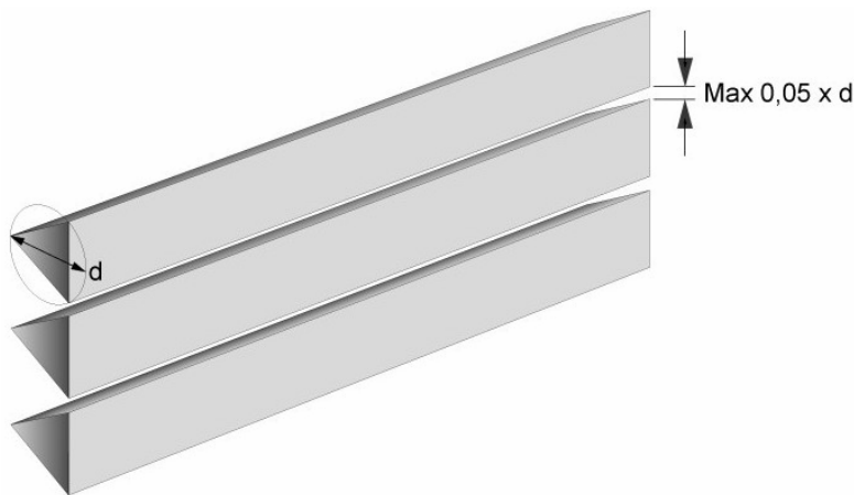
Figur 2. 9: Avstand mellom tilstøtende flatelementer
