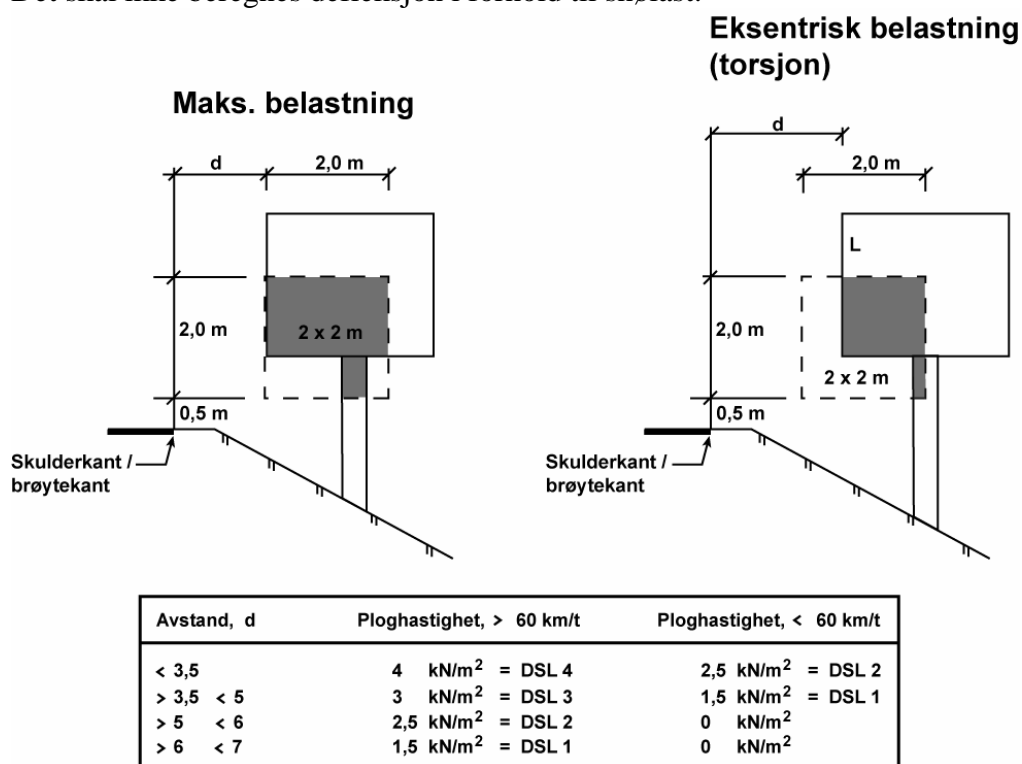
Figur 5.3 Beregning av dynamisk brøytelast.
