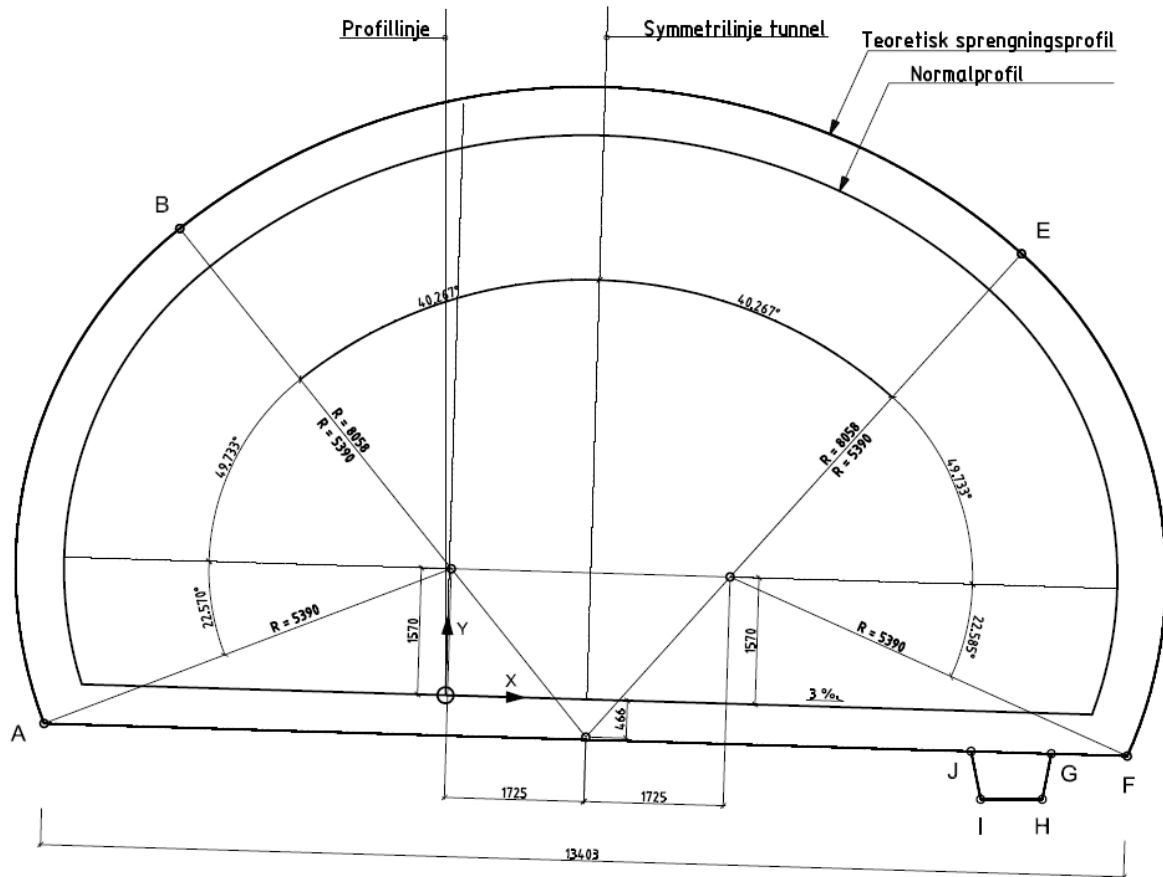
Ⓐ TUNNELPROFIL - T12.5 1:25 Areal teoretisk sprengningsprofil = 96.735 m 2
