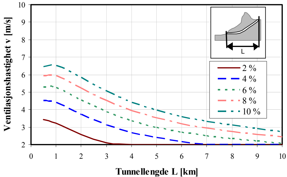
Figur D.13 Ventilasjonshastighet 50 MW brann, jevn stigning og \Delta p = 0 Pa.
