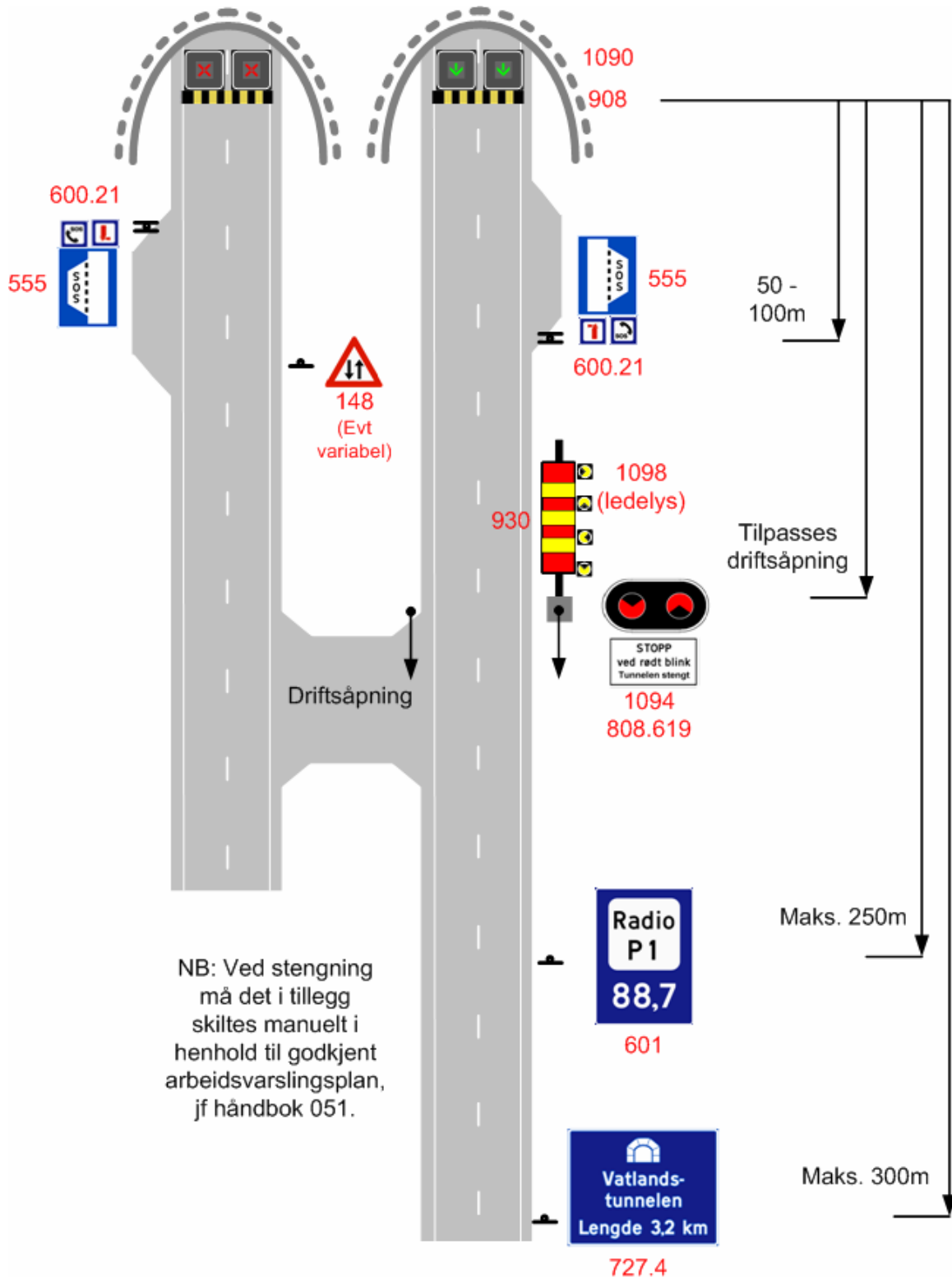
Figur 6.3 Prinsippskisse som viser plassering av skilt i portalene for toløpstunnel
