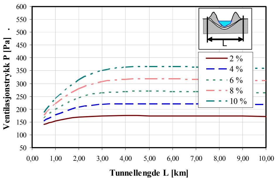
Figur D.12 Ventilasjonstrykk 20 MW brann, jevn stigning over halv lengde og \Delta p = 64 Pa.
