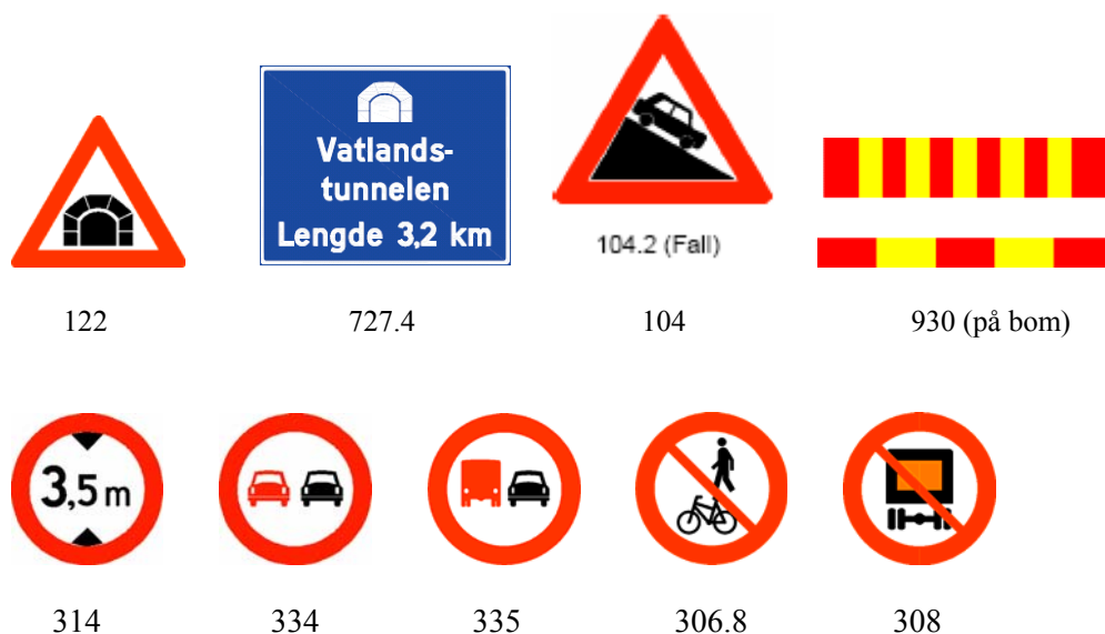
Figur 6.1 Aktuelle skilt utenfor tunnel
