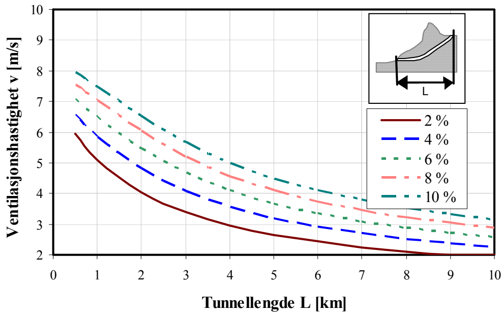
Figur D.29 Ventilasjonshastighet 50 MW brann, jevn stigning og \Delta p = 64 Pa.
