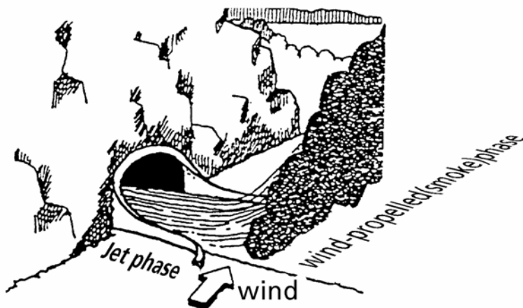
Figur A.1 Jettefase og vinddrevet (plume-) fase
