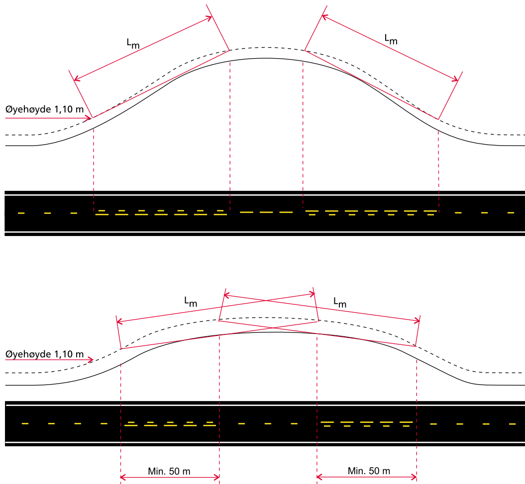
Figur 4.3 Midtlinje i uoversiktlige vertikalkurver
