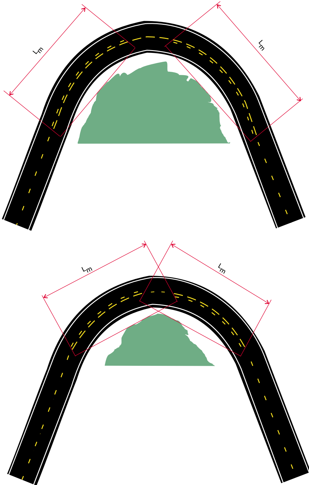
Figur 4.4 Midtlinje i uoversiktlige horisontalkurver
