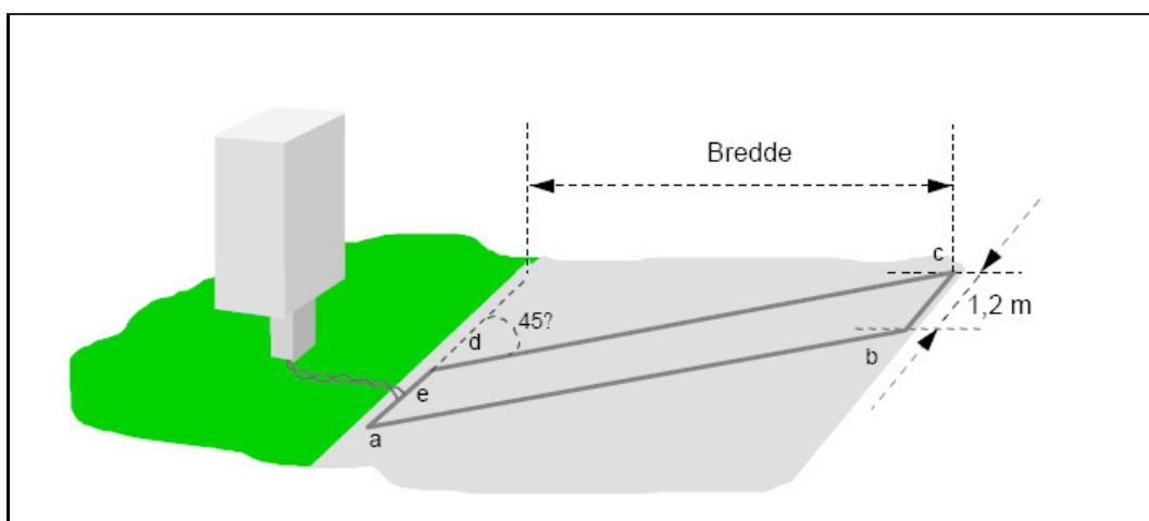
Figur 4.5 Prinsippkisse for detektering av sykkel ved bruk av induktiv sløyfe og Dr410.
