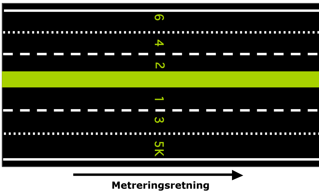
Figur 2.5 Feltnummerering av veg med et kollektivfelt i hver kjøreretning
