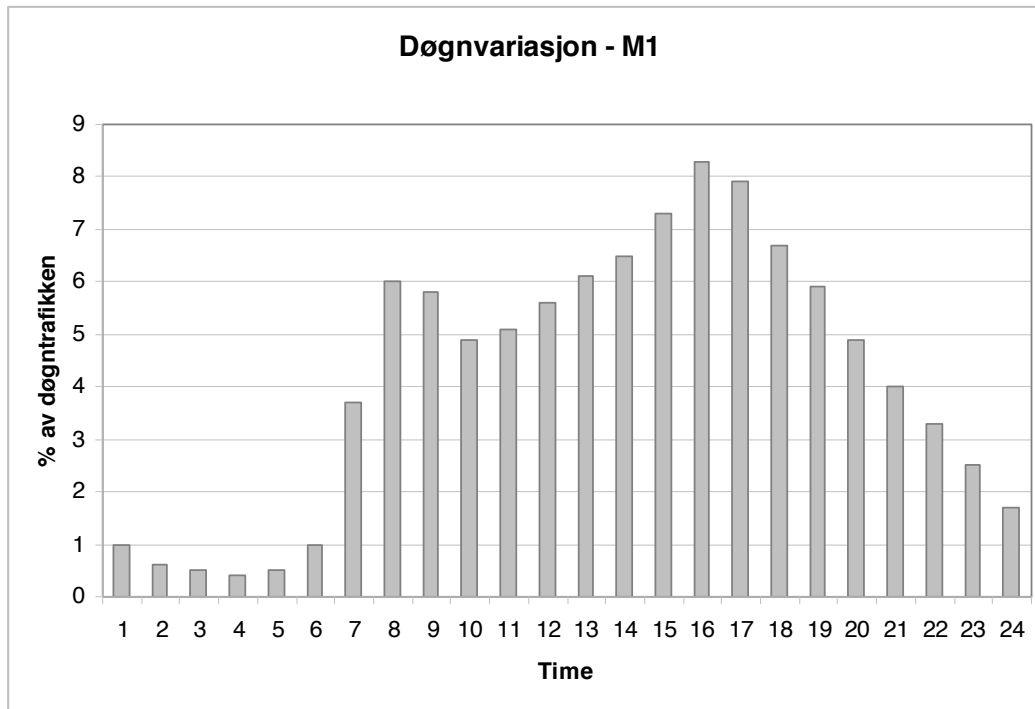
Figur 3.1 Eksempel på døgnvariasjonskurve som viser hvordan trafikken varierer over døgnet som prosent av DT.
