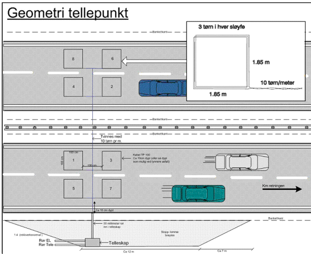
Figur 4.23 Geometrisk utforming av registreringspunkt
