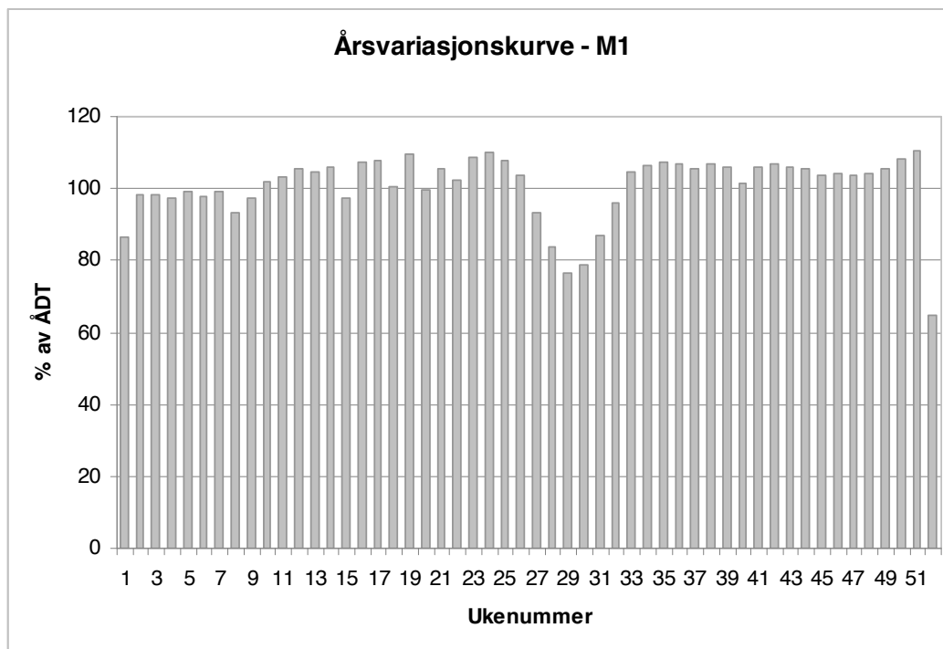
Figur 3.3 Eksempel på årsvariasjonskurve som viser hvordan trafikken varierer for hver enkelt uke i forhold til ÅDT.
