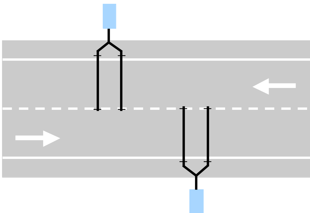
Figur 4.12 Eksempel på oppsett av slanger på 2-felts veg
