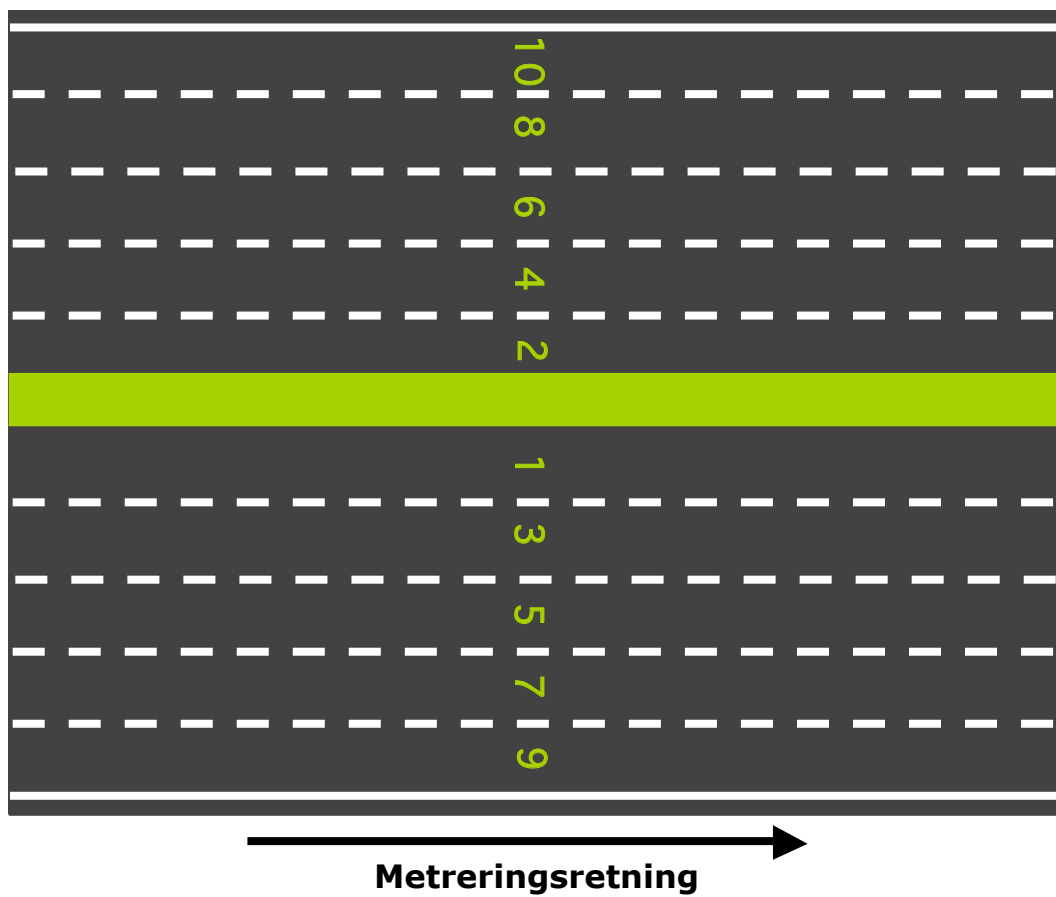
Figur 2.2 Feltnummerering på en 10-feltsveg
