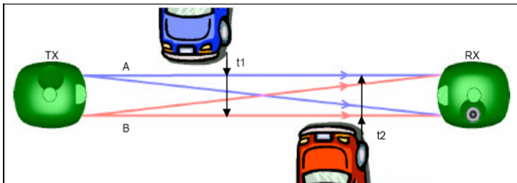
Figur 4.14 Prinsippkisse for registrering med infrarødt lys ved bruk av utstyret The Infra Red Traffic Logger (TIRTL)
