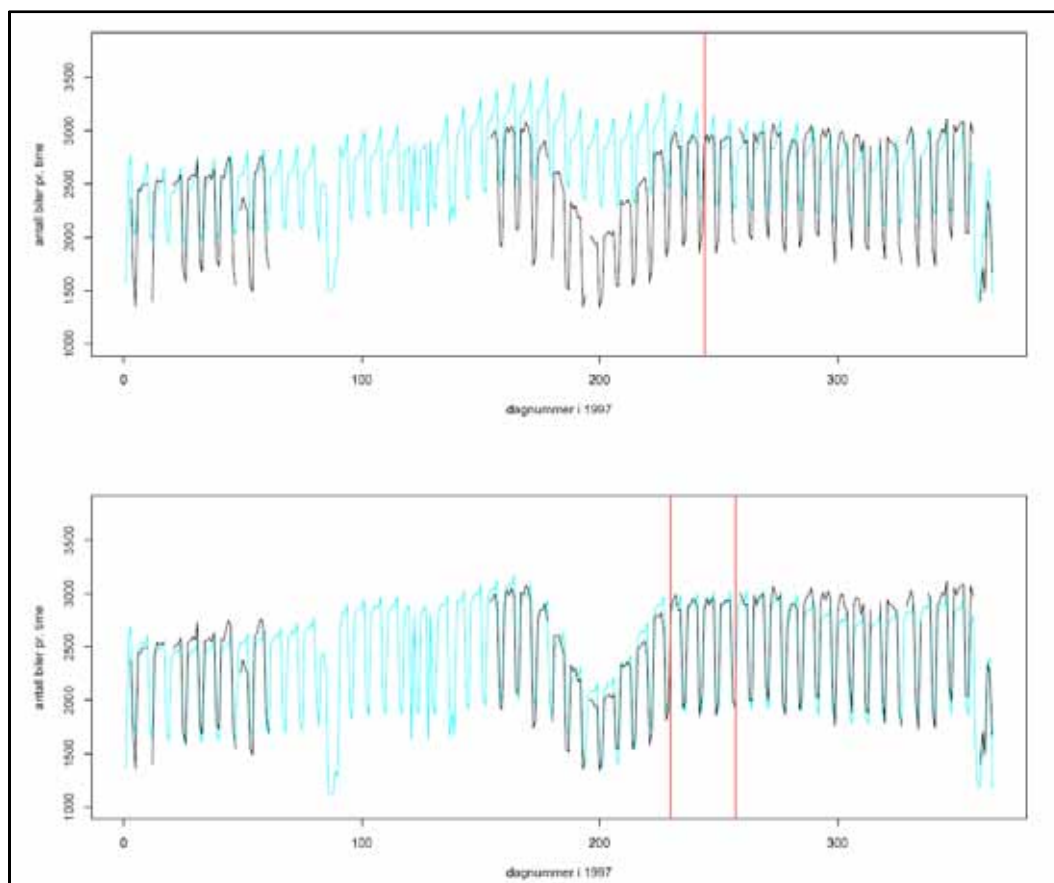
Figur 3.5 Tilpassede kurver (lyseblå) etter et døgns registrering (øverst) og fire ukers registrering (nederst). Alle tilgjengelige data er vist med sort kurve. Registreringsperioden som er benyttet ved tilpassing av kurven er vist med rødt. (Aldrin og Haug 2000)
