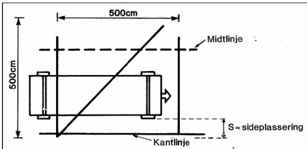
Figur 4.9 Prinsippkisse for piezoelektriske kabler ved registrering av kjøretøyenes sidevegs plassering i vegbanen.
