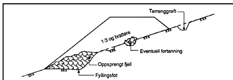
Figur 253.2 Fortanning ved berghelning 1:3 og brattere
