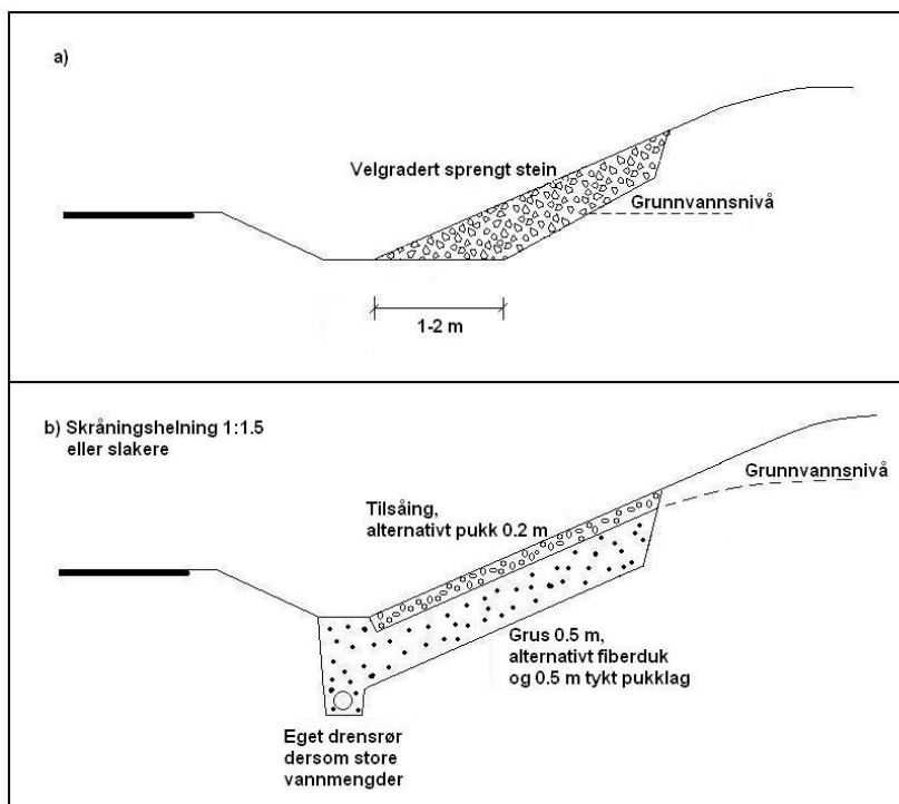
Figur 245.5 Eksempler på skråningsbeskyttelse ved masseutskifting
