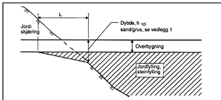
Figur 512.10 Utkiling ved overgang jordskjæring/fylling
