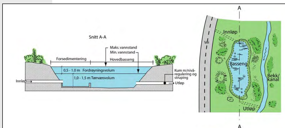
Figur 403.2 Utforming av vått overvannsbasseng
