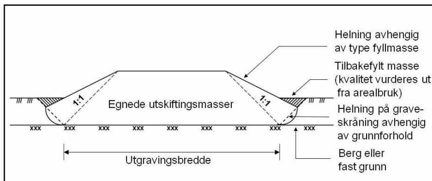
Figur 231.1 Masseutskifting ved graving
