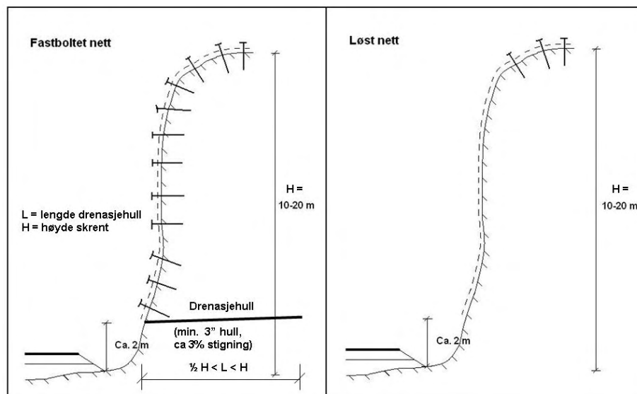
Figur 228.1 Prinsipp for sikring av bergskråning/-skjæring med nett. Nettet bør avsluttes ca. 2 meter over grøft for å hindre klatring og lek i nettet.
