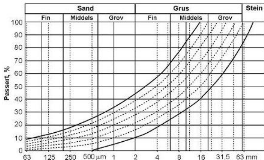
Figur 523.16B Grensekurver, Ak til bærelag og forsterkningslag
