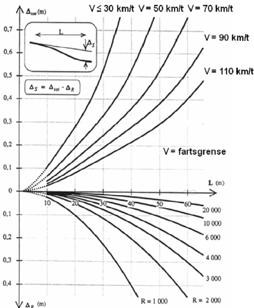
Figur 205.1 Største tillatte setningsforskjell \Delta_s på strekningen L
