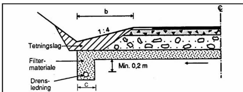
Figur 406.3 Grunn drenggrøft med drengsledning
