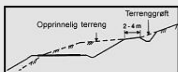
Figur 413.1 Plassering av terrenggrøft
