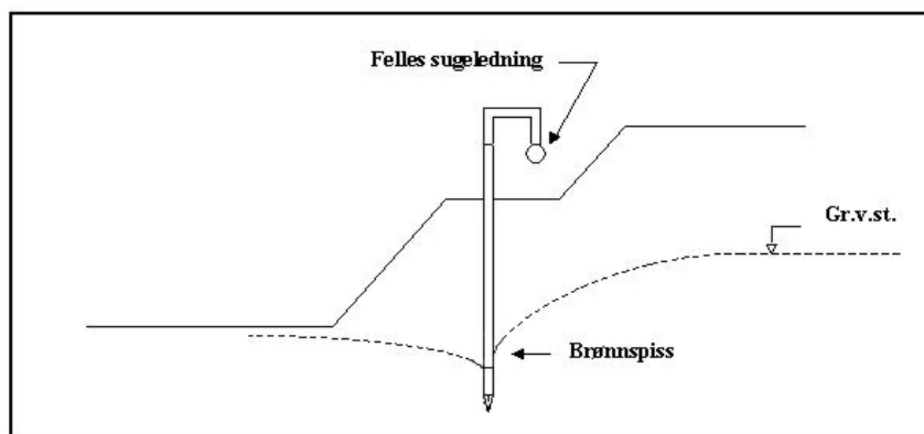
Figur 238.2 Grunnvannsenkning ved Wellpoint
