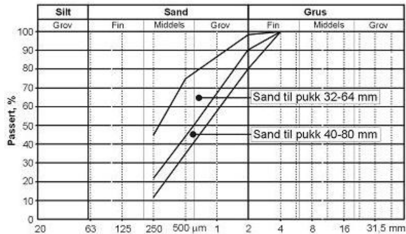
Figur 523.24 Grensekurver for sand til sementstabilisert pukk
