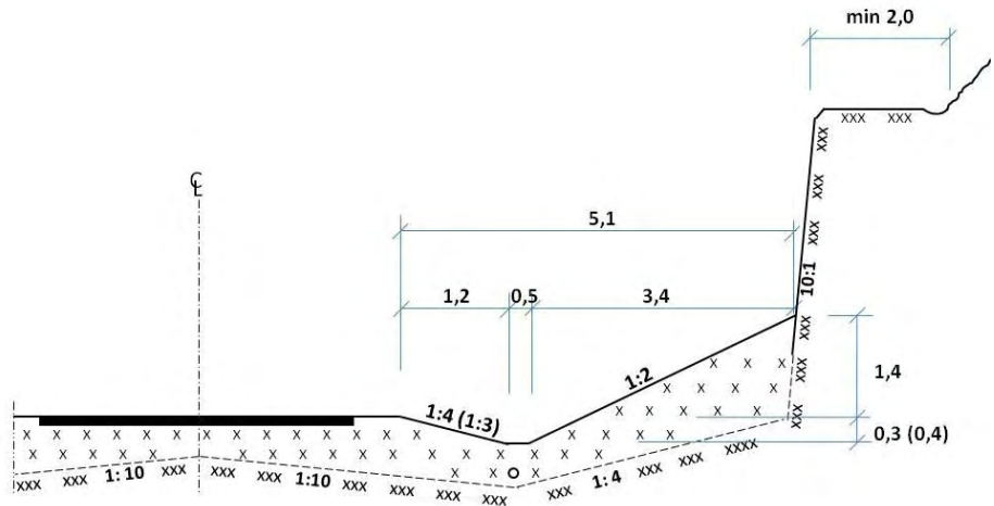
Figur 225.1 Normalprofil i bergskjæring når rekkverk ikke benyttes.
