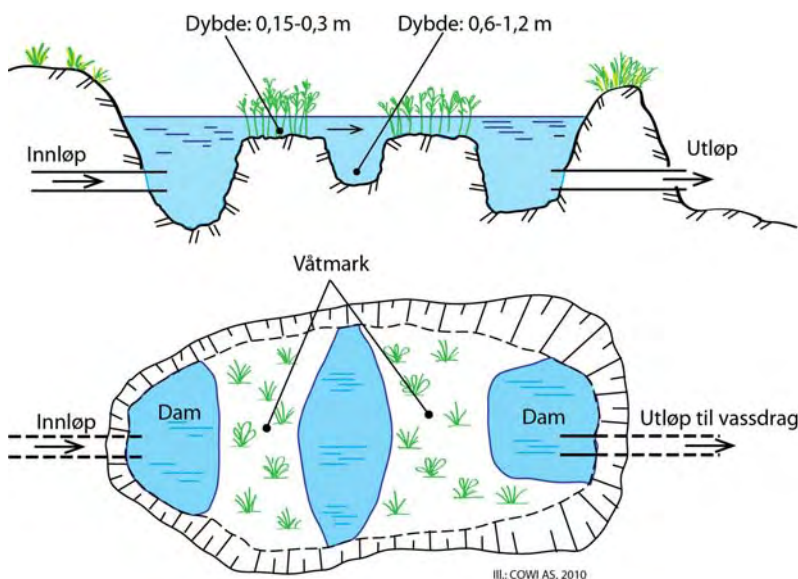
Figur 403.8. Prinsippskisse av kunstig anlagt våtmark (plan/snitt).
