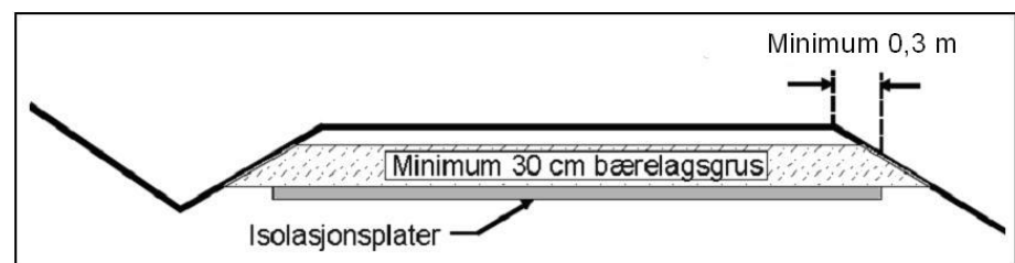
Figur 524.2 Frostsikring av veg med skumplast
