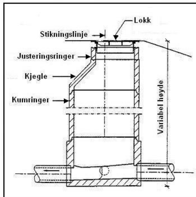
Figur 463.5 Eksempel på overvannskum
