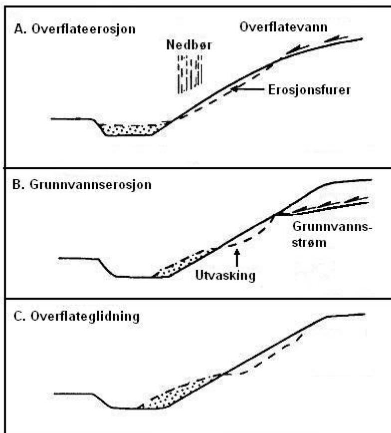
Figur 245.1 Typer av skråningsskader i jord
