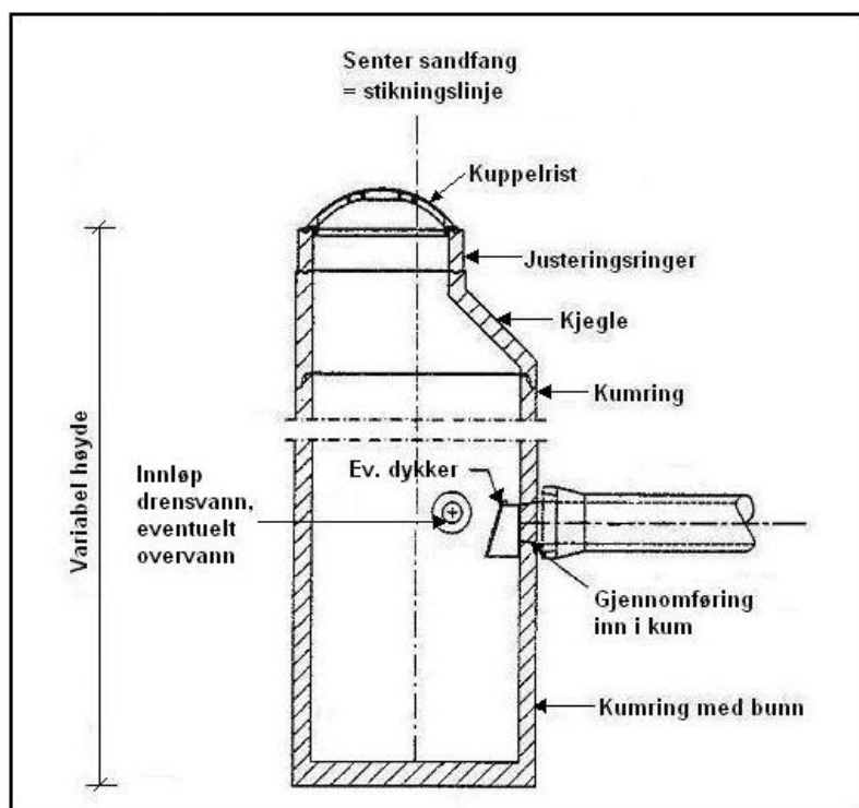
Figur 463.2 Eksempel på sandfang ("standardkum")
