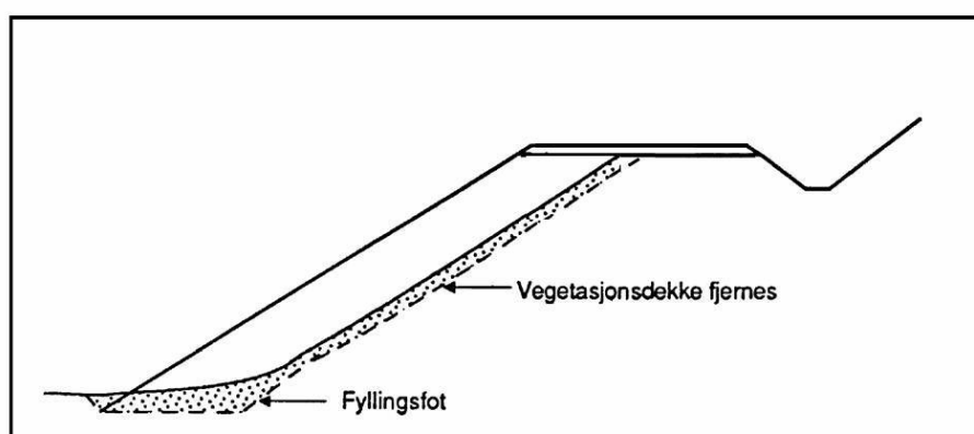
Figur 257.1 Breddeutvidelse av veg
