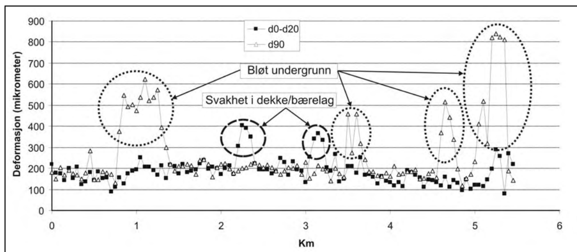
Figur V6.2 Eksempel på tolking av falloddmålinger mht. lokalisering av svake lag (d90 = nedbøyning i avstand 90 cm fra lastsenteret, d0-d20 = differanse mellom nedbøyning rett under lastsenter og nedbøyning 20 cm fra lastsenter, dvs. krumning av overflaten under lastsenteret)
