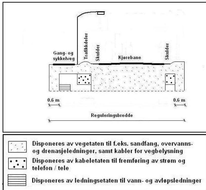
Figur 401.1 Prinsippskisse, plassering av kabler og ledninger i 2-feltsveg med separat G/S-veg
