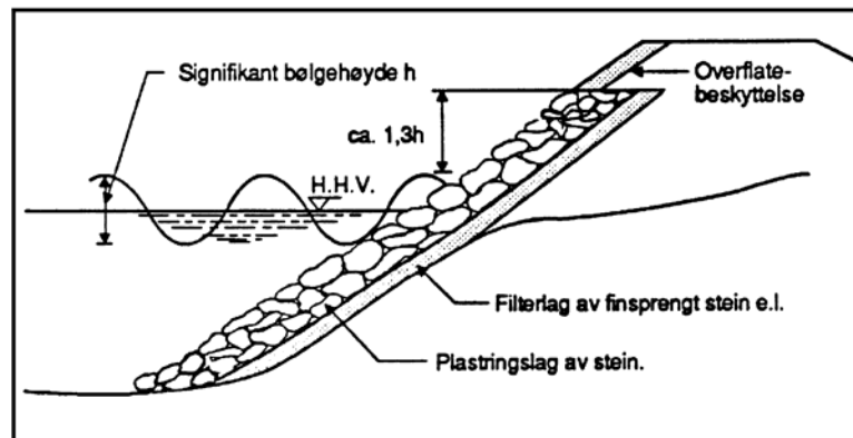
Figur 262.1 Utforming av steinplastring
