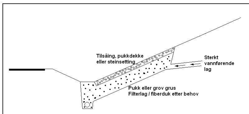
Figur 245.3 Drensgrøft for vannførende sjikt med stor vannføring
