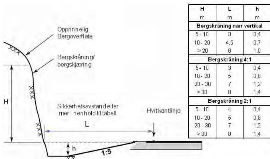
Figur 225.4 Dimensjonering av fanggrøft for steinsprang (når bergskjæringen ikke sikres på annen måte)
