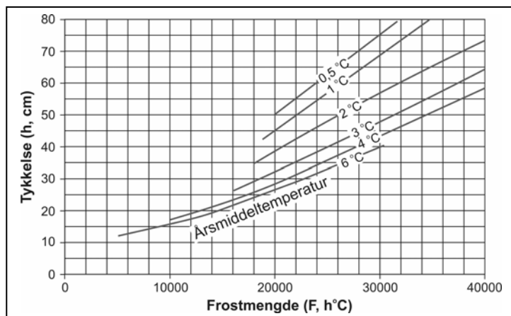
Figur V1.2 Frostteknisk dimensjonering av frostsikringslag av lettklinker eller skumglassgranulat
