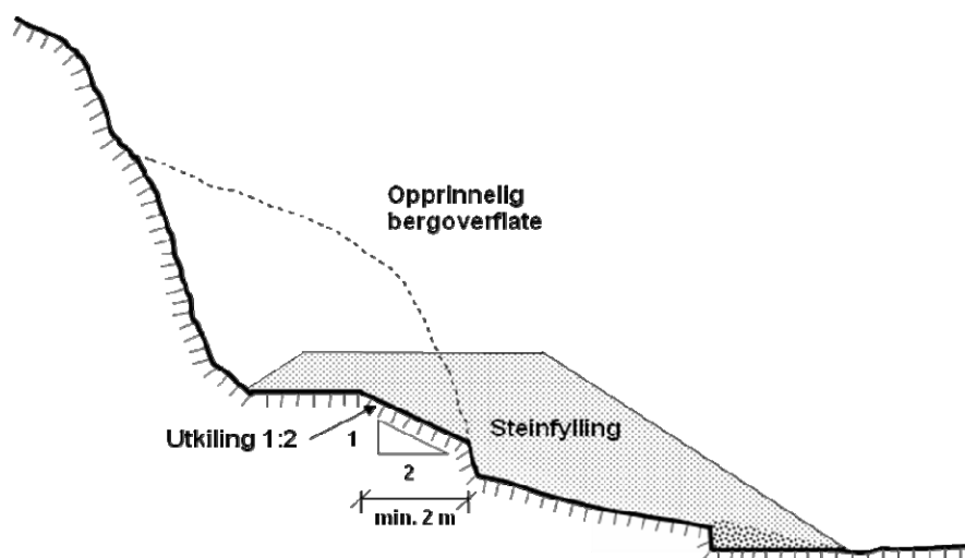
Figur 256.2 Utkiling i overgang mellom steinfylling og bergskjæring
