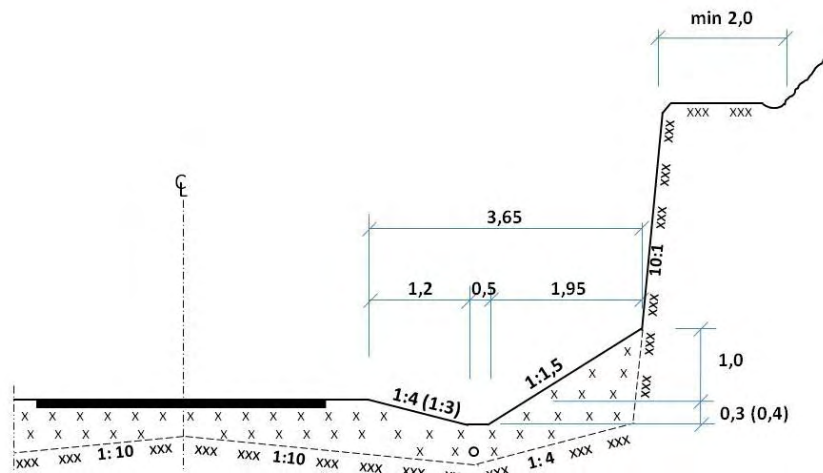
Figur 225.2 Redusert skjæringsprofil med tilbakefylling mot berg.
