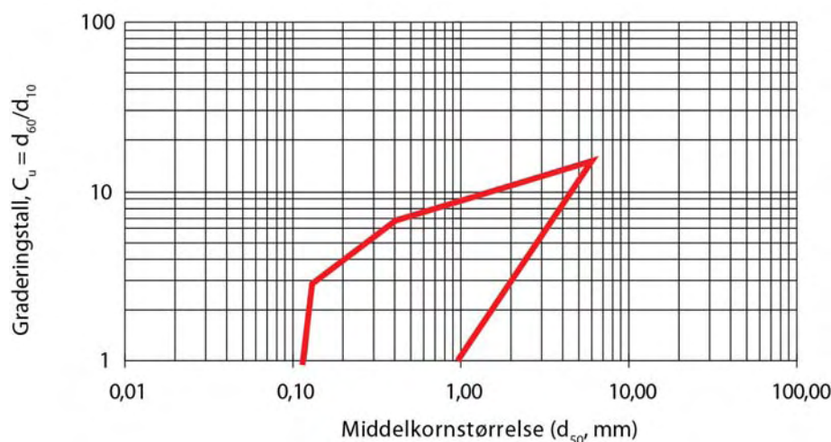
Figur 403.5 Grensekurver for anbefalte filtermasser i infiltrasjonsanlegg. Filtermasser som ligger innenfor rød grensecurve samt har d_{10} > 0,1 mm og maks 2-3 % < 0,063 mm, er tilfredsstillende.
