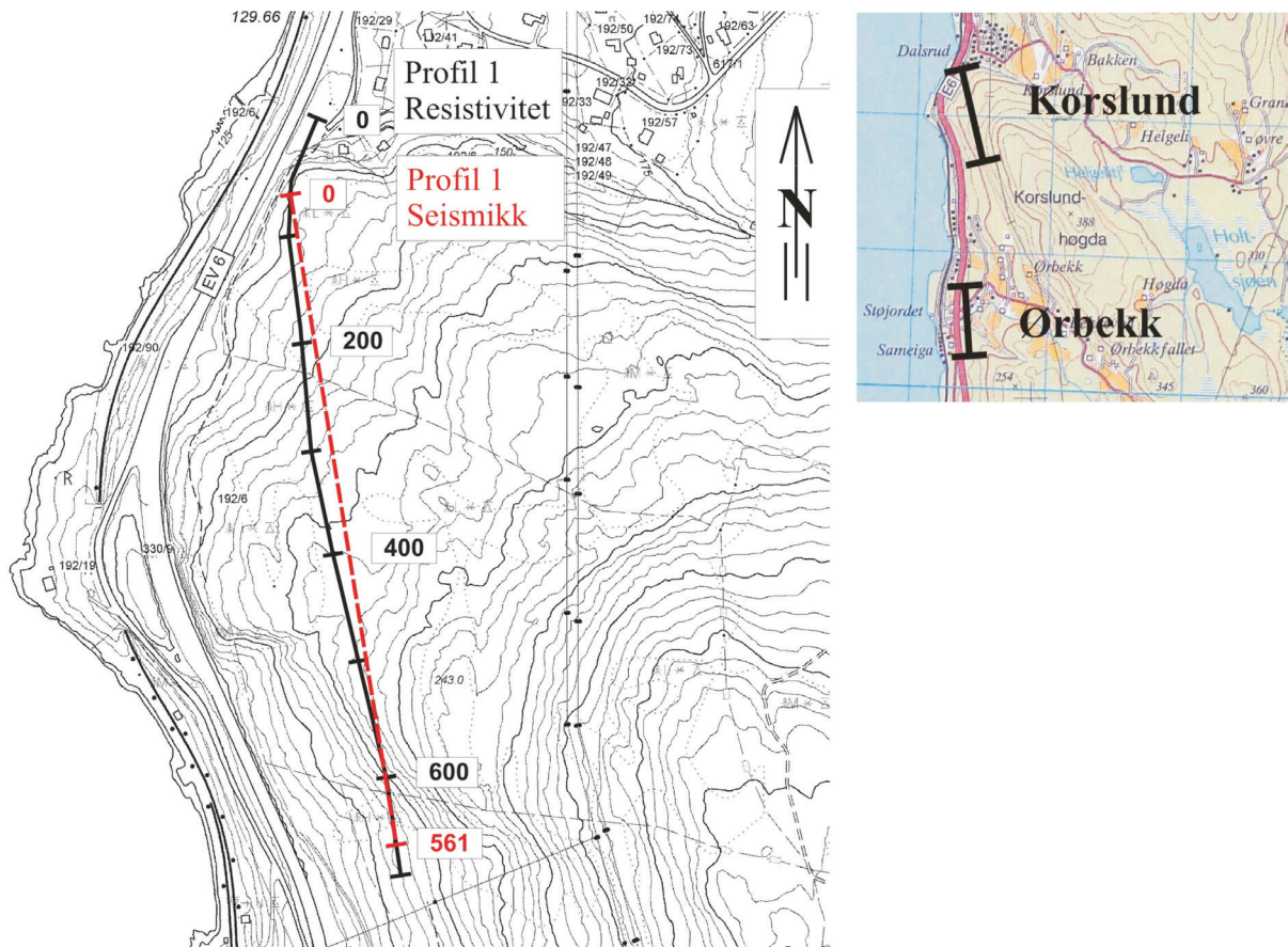
Figur 6: Lokalisering av refraksjonsseismisk profil og resistiviteitsprofil ved Korslund. Profilet med refraksjonsseismikk er markert med rød, stiplet linje (561 m), mens resistiviteitsprofilet er markert med svart linje (700 m).
