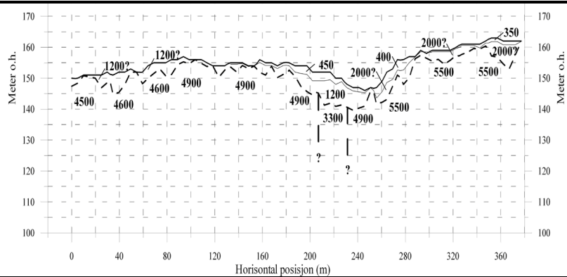
Figur 22: Sammenstilling av resistivitet og seismiske tolkninger ved Ørbekk.
