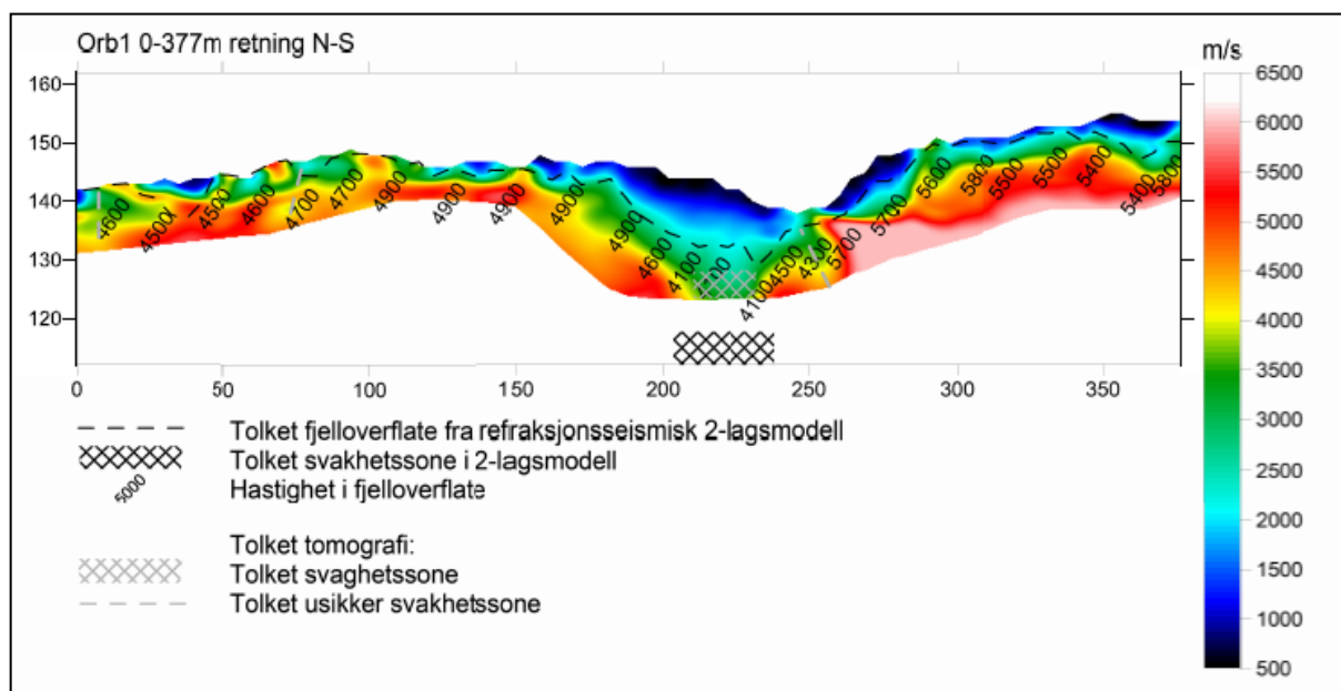
Figur 2: Opprinnelig tolking av refraksjonsseismisk profil ved Ørbekk (Wisén 2008). Overgangen fra løsmasser til fjell, hastighet i fjell og svakhetssoner fra GRM-metoden er fremstilt med stiplet linje, svartetall og svart skravur. Hastigheter fra tomografisk inversjon er angitt med fargekode og svakhetssoner er angitt med grå skravur.
