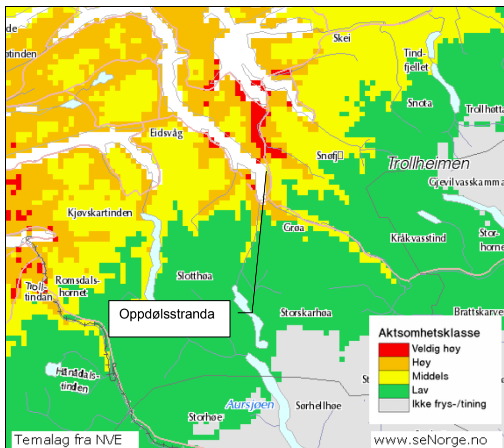
Figur 5: Historiske data fra "Sunndalsøra III", interpolert mot tilgrensede værstasjoner, er brukt for å tilbakeregne et aktsomhetskart for steinsprangfare 31.12.2004 ut fra frysing/tining kombinert med vanntilførsel.
