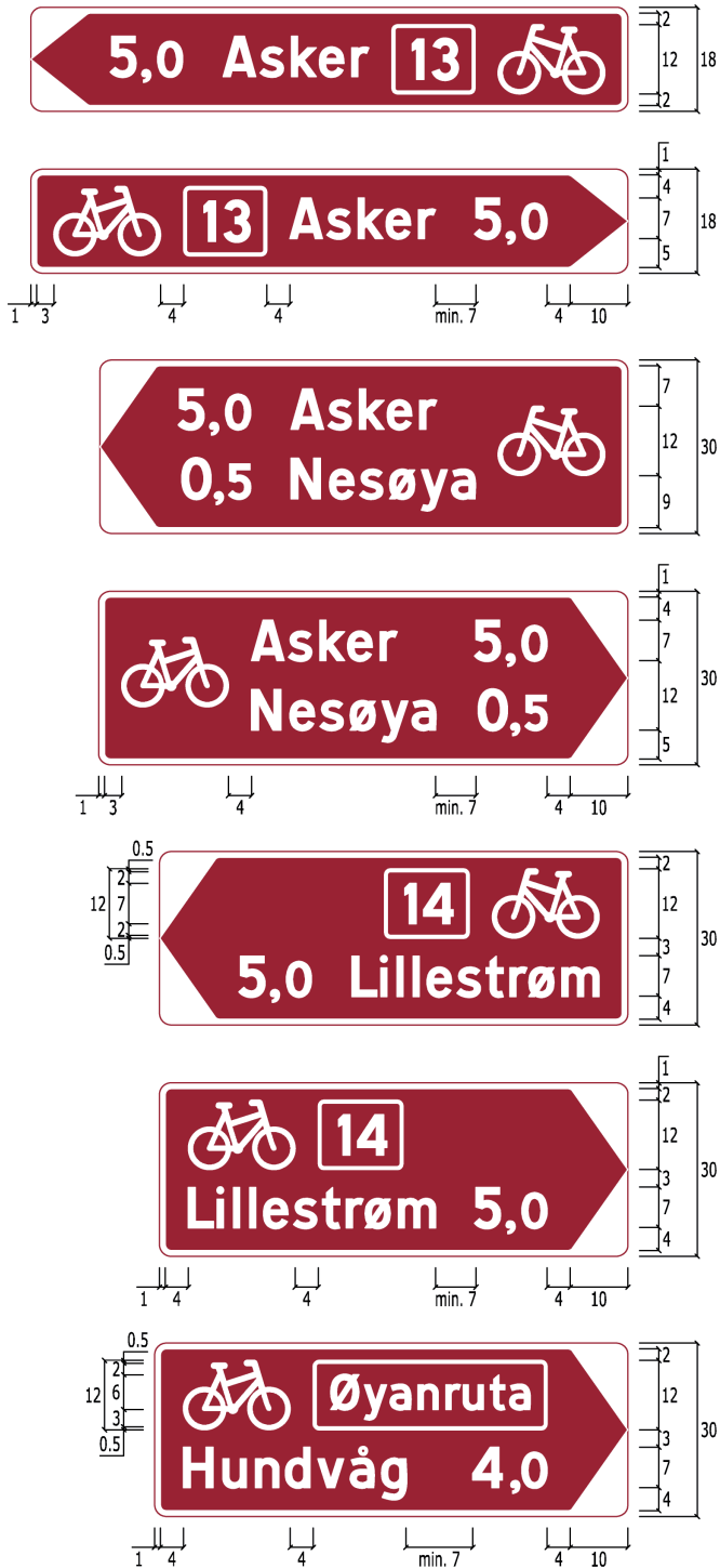
Figur 4-3.36 Utforming av skilt 751 "Vegviser for sykkelrute". Alle mål i 1/7 H.
