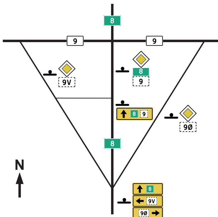
Figur 4-3.29 Eksempel på bruk av vegnummerskilt med angivelse av hovedretning og bruk av stiplede bord
