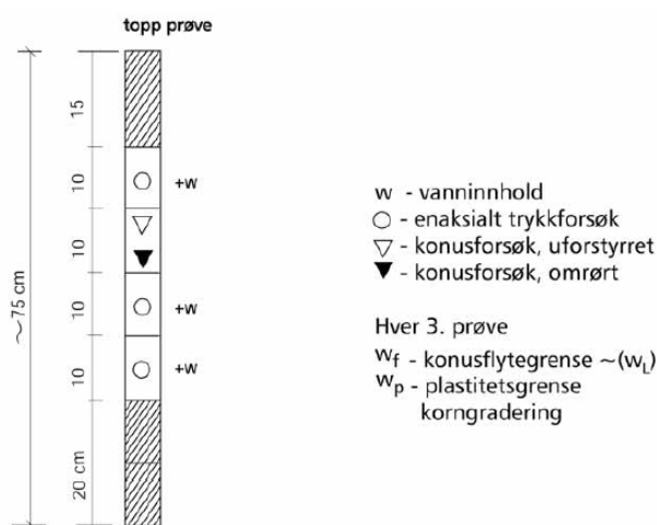
Figur 10 Inndelingen av rutineanalyserne for intakte prøver (Statens Vegvesen 2010).
