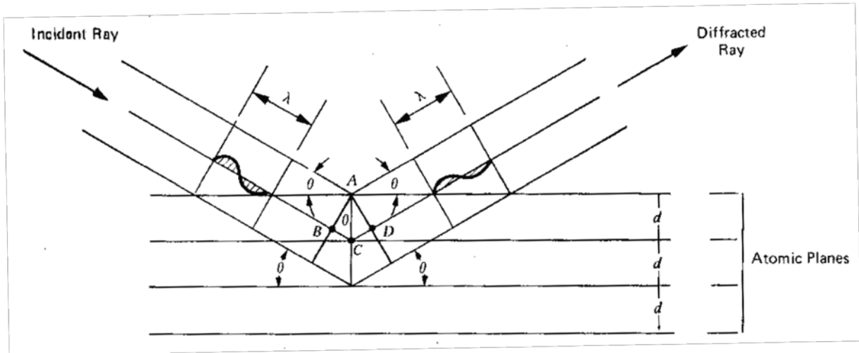
Figur 17 Skjematisk oversikt over rådende geometriske forhold, i henhold til Braggs Lov (Mitchell og Soga 2005).
