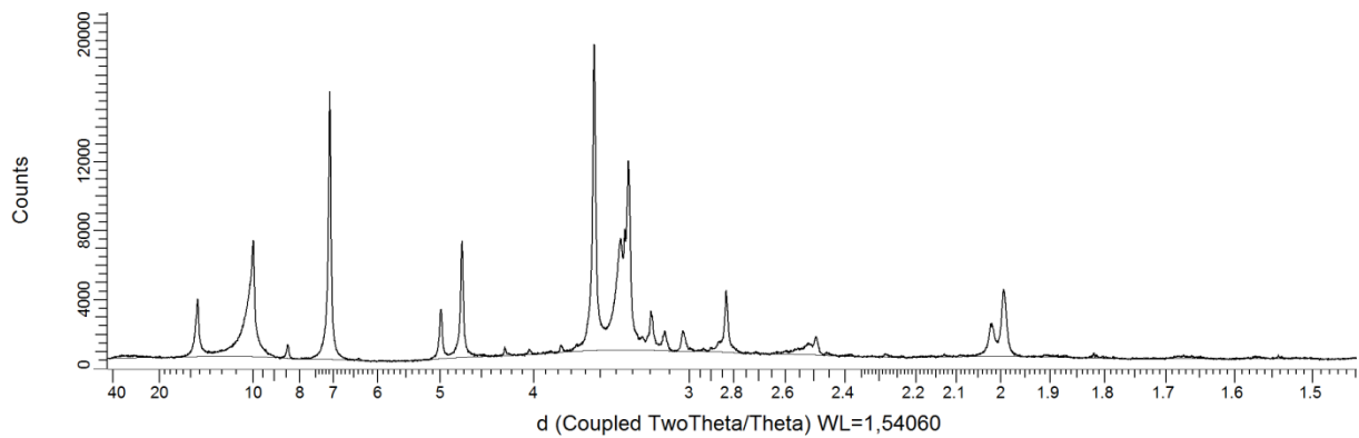
Figur 18 Diffraksjonsmønster for en leirprøve i programmet Diffrac.eva før analyse.
