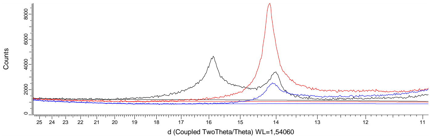
Figur 30 Viser hvordan toppen ved 14 Å (rød) ekspanderer mot 16 Å ved behandling med etylenglykol (svart), før den kollapser ved 350 °C varmebehandling. Prøven er hentet i fra Alta.
