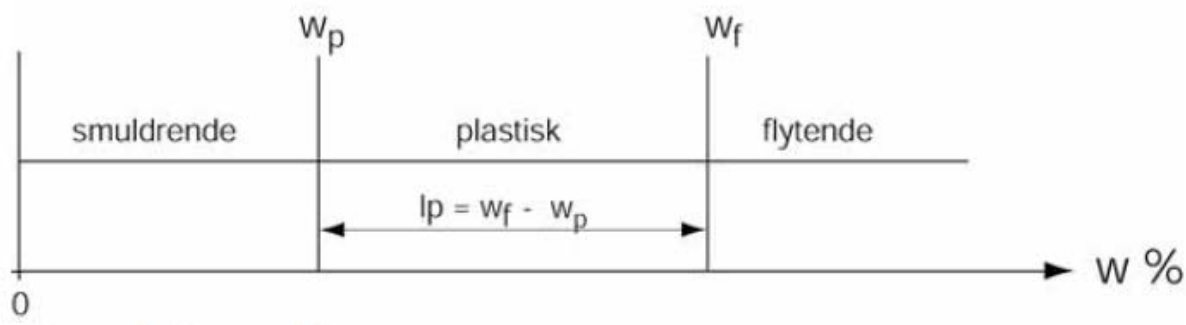
Figur 11 Konsistensitetsgrensene (Statens Vegvesen 2010).
