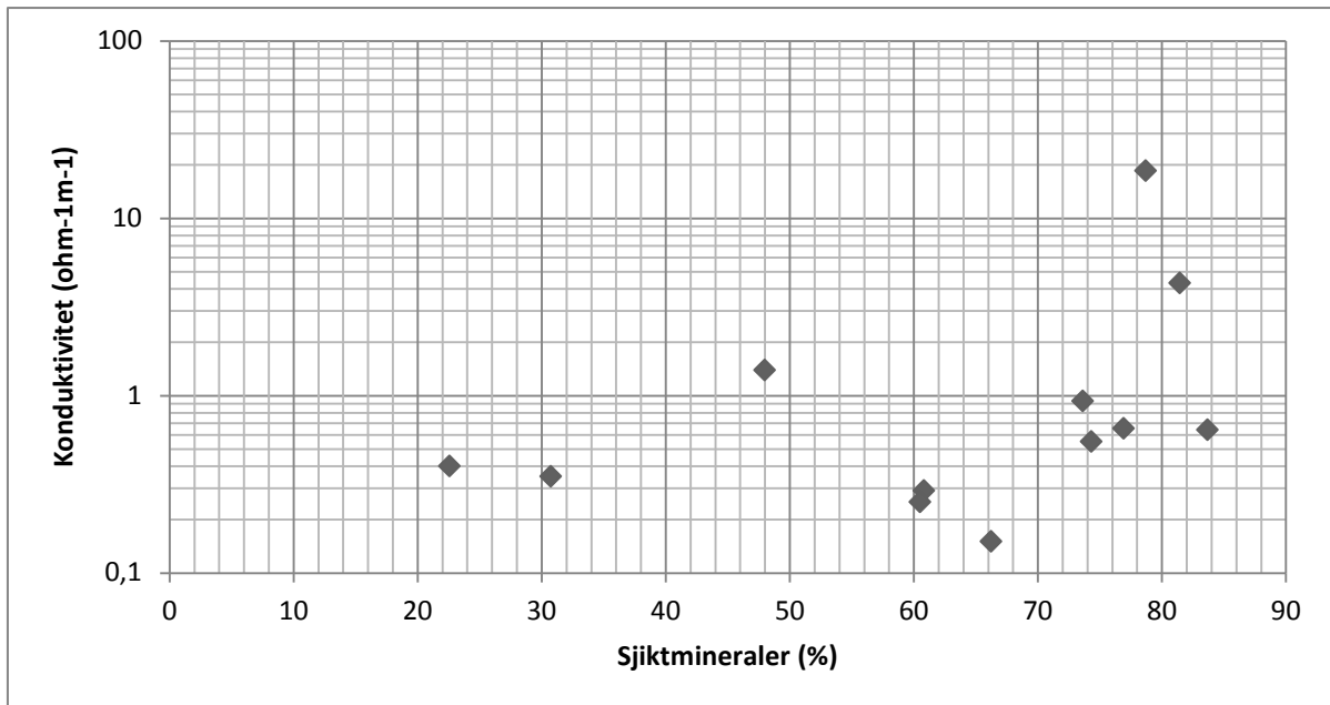
Figur 38 Konduktiviteten plottet på en logaritmisk skala mot prosentvis andel av sjiktmineraler.
