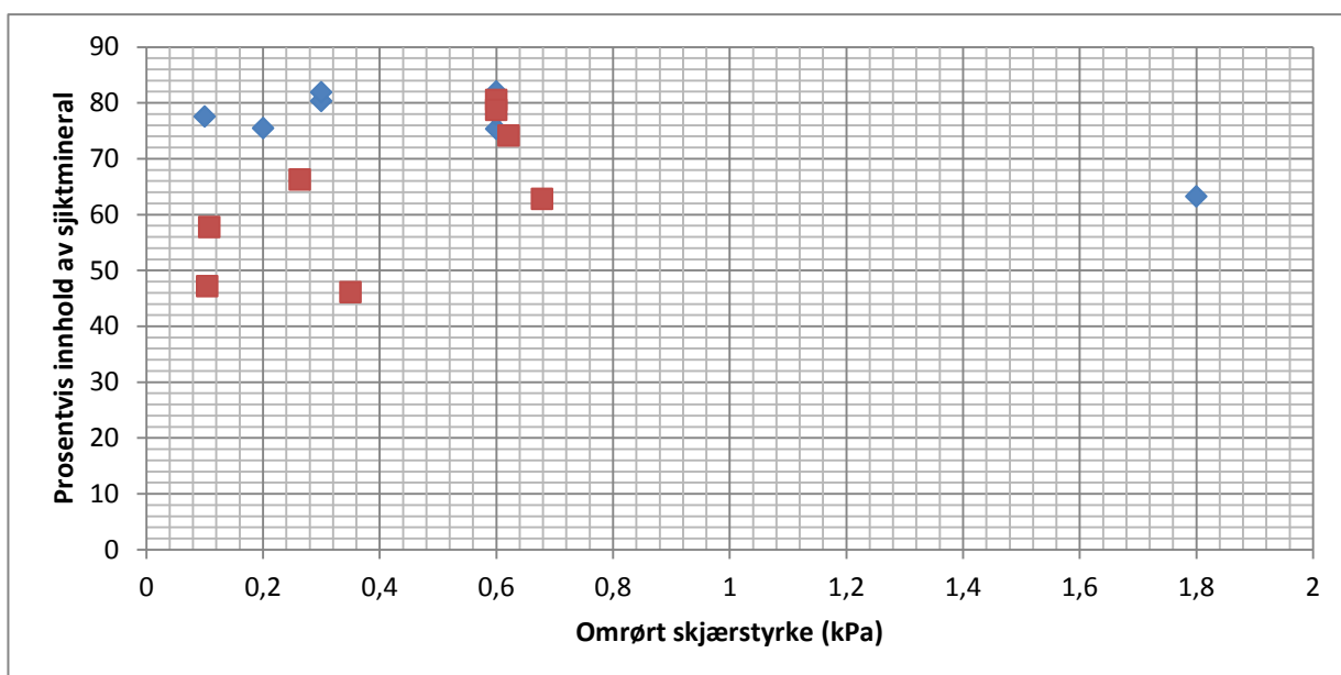
Figur 52 Prosentvis innhold av sjiktmineral mot omrørt skjærstyrke for Rundhaug Olsborg (rød) og Leira (De Blasio).
