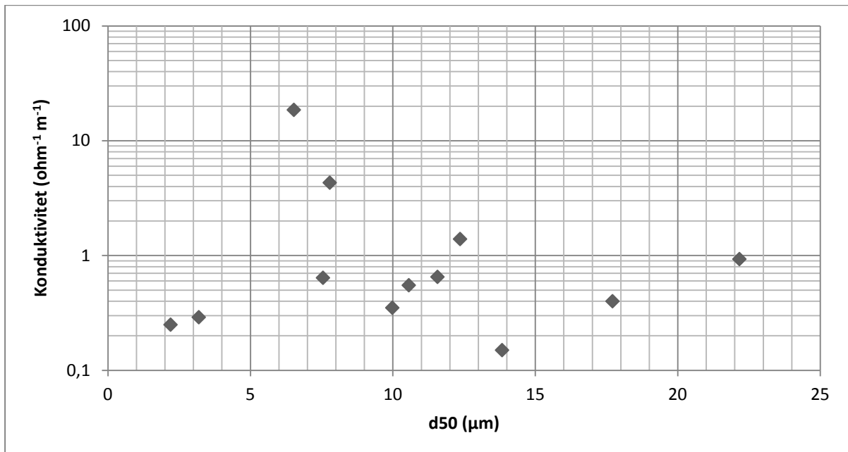
Figur 37 Konduktivitet plottet på en logaritmisk skala mot d_{50} .
