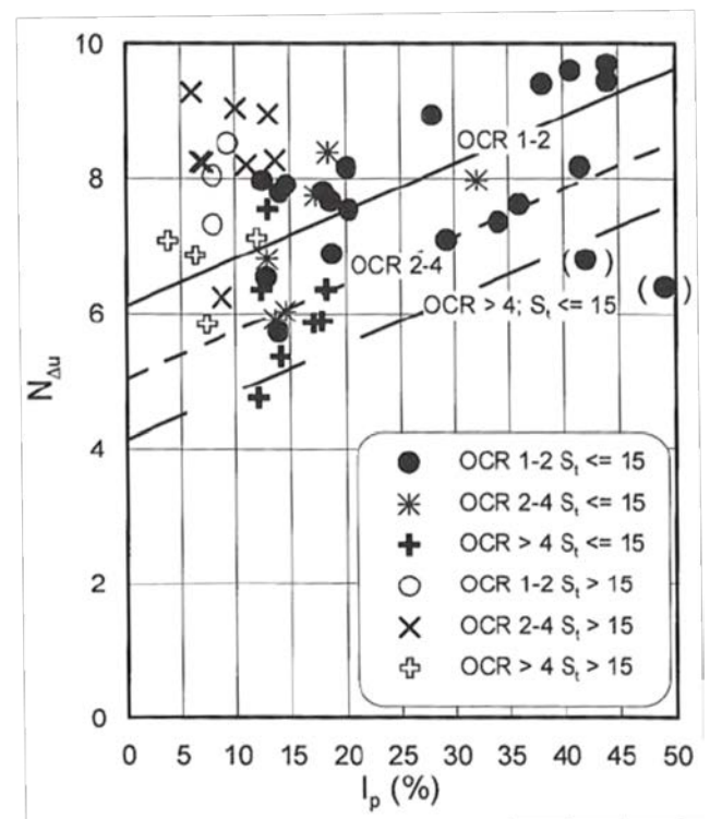
Figur 2 Plastisitetsindeksen innvirkning på poretrykksfaktoren. De to markerte punktene har ikke blitt vektlagt ved I_p -korrelasjonen, da innholdet av organisk materiale var svært høyt. Dette kan ha resultert i en økt I_p (Karlsruud et al. 2005).
