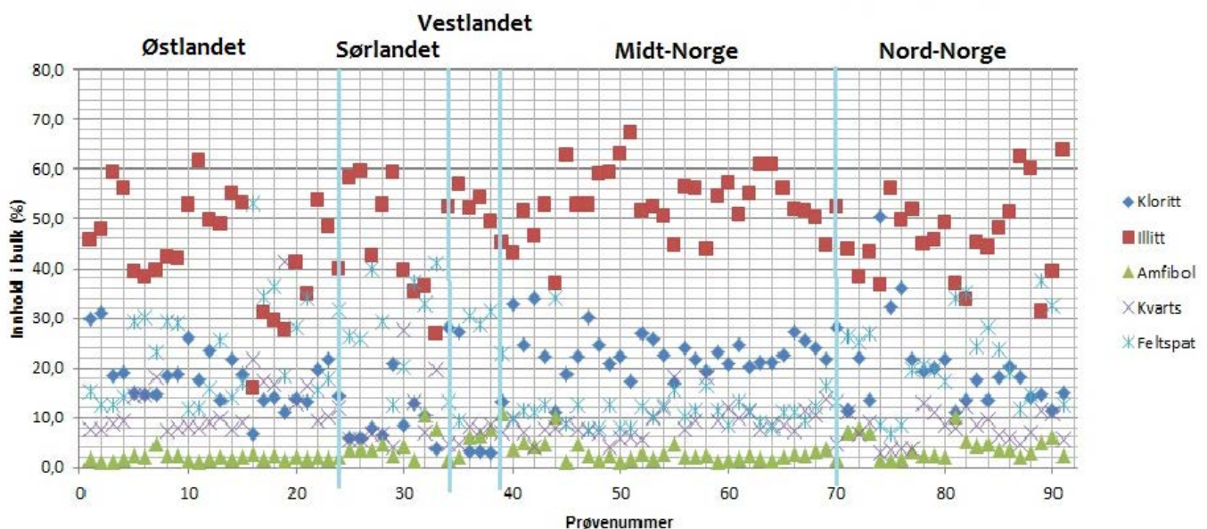
Figur 28 Variasjonene i mineralinnhold for samtlige prøver, inndelt i regioner. Innhold av pyritt og kalsitt er ekskludert.
