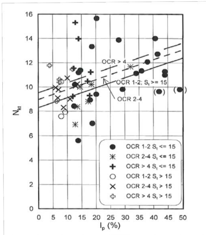
Figur 1 Plastisitetsindeksen innvirkning på CPTU faktor ( N_{kt} ) (Karlsruud et al. 2005).
