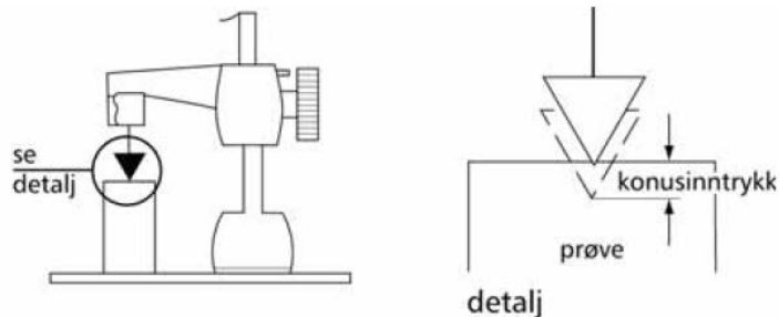
Figur 13 Konusapparat (Statens Vegvesen 2010)
