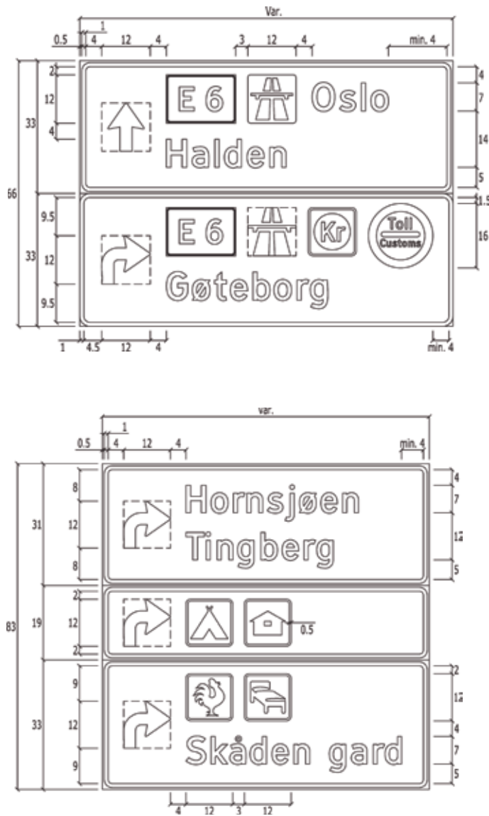
Figur 4-4.8 Eksempler på plassering av visningselementer på tabellskilt
