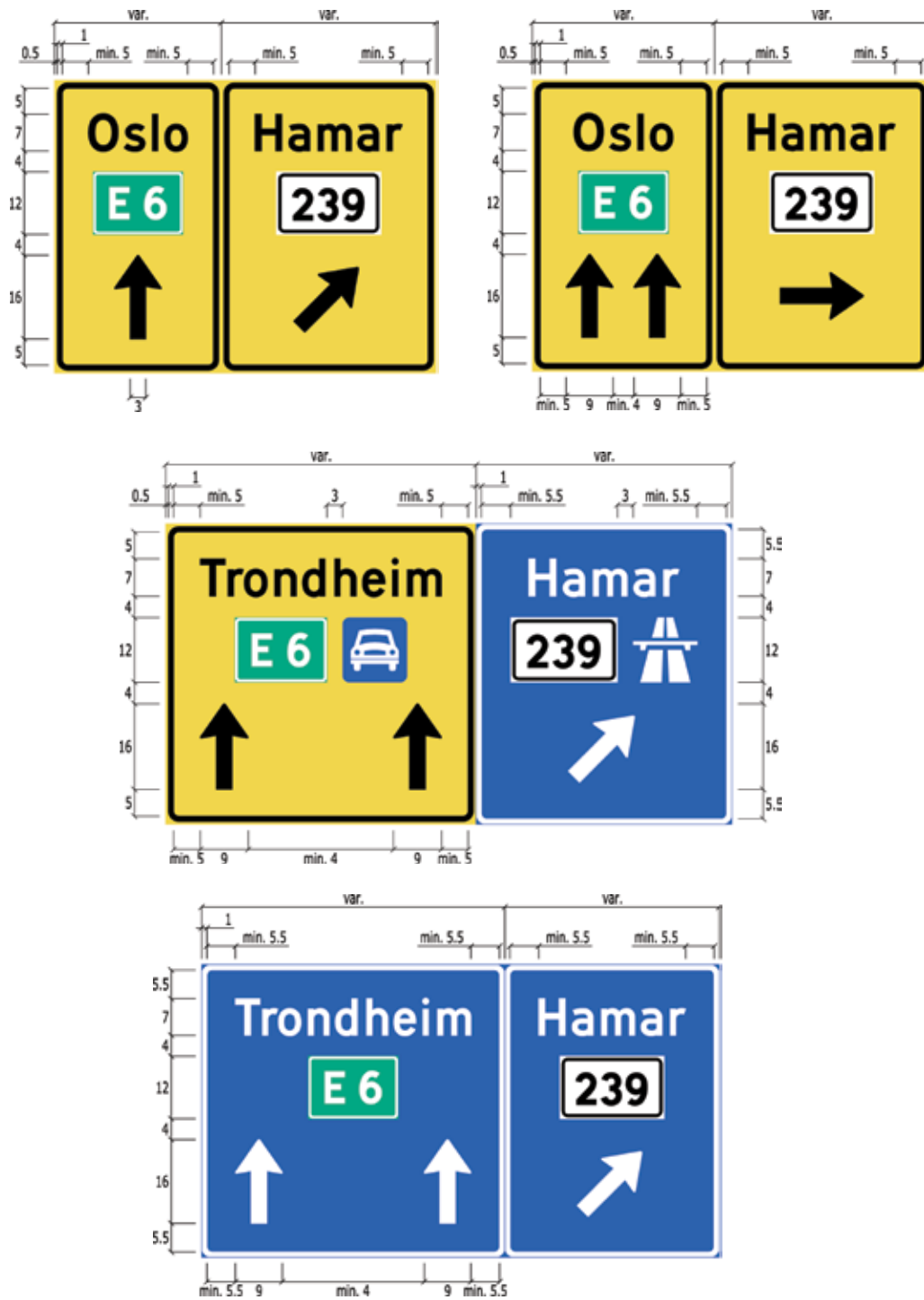
Figur 4-4.39 Eksempler på utforming av skilt 717
