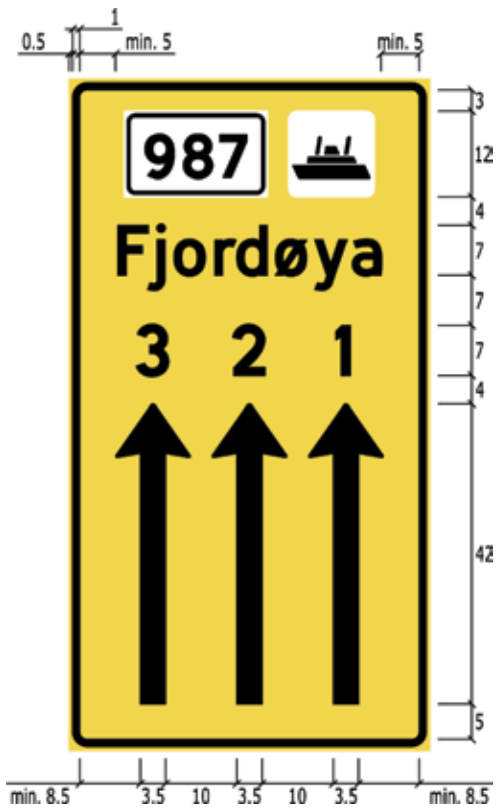
Figur 4-4.24 Eksempel på utforming av kjørefeltorienteringstavle 707.4
