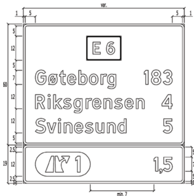
Eksempel på skilt 725.2 på motorveg.
