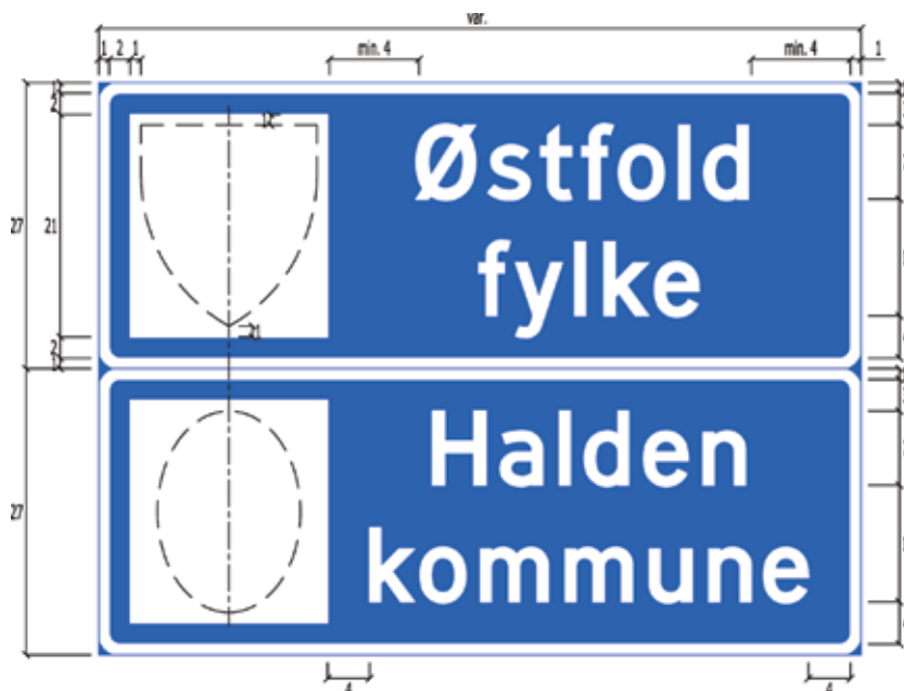
Figur 4-4.60 Utforming av skiltene 727.3F og 723.3K
