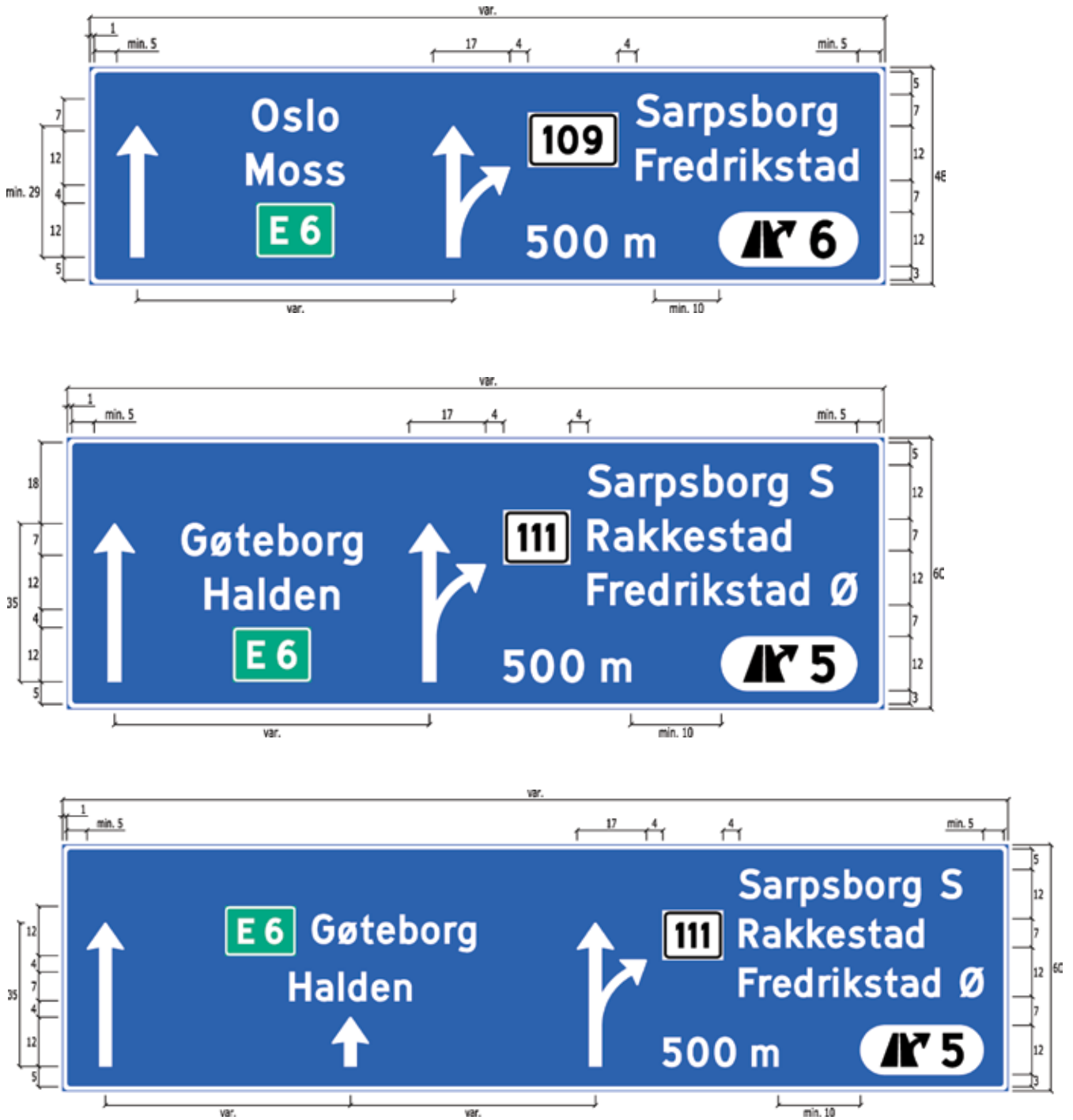
Figur 4-4.31 Eksempler på utforming av skilt 709.3
