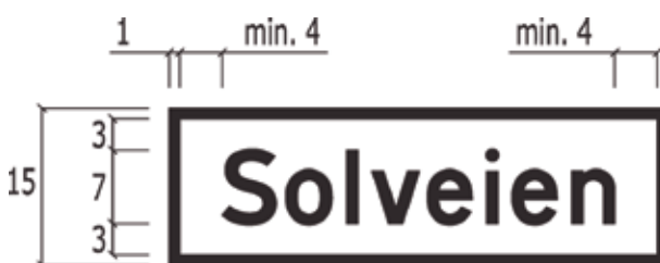
Figur 4-4.63 Utforming av skilt 729 "Gate-/vegnavnskilt"
