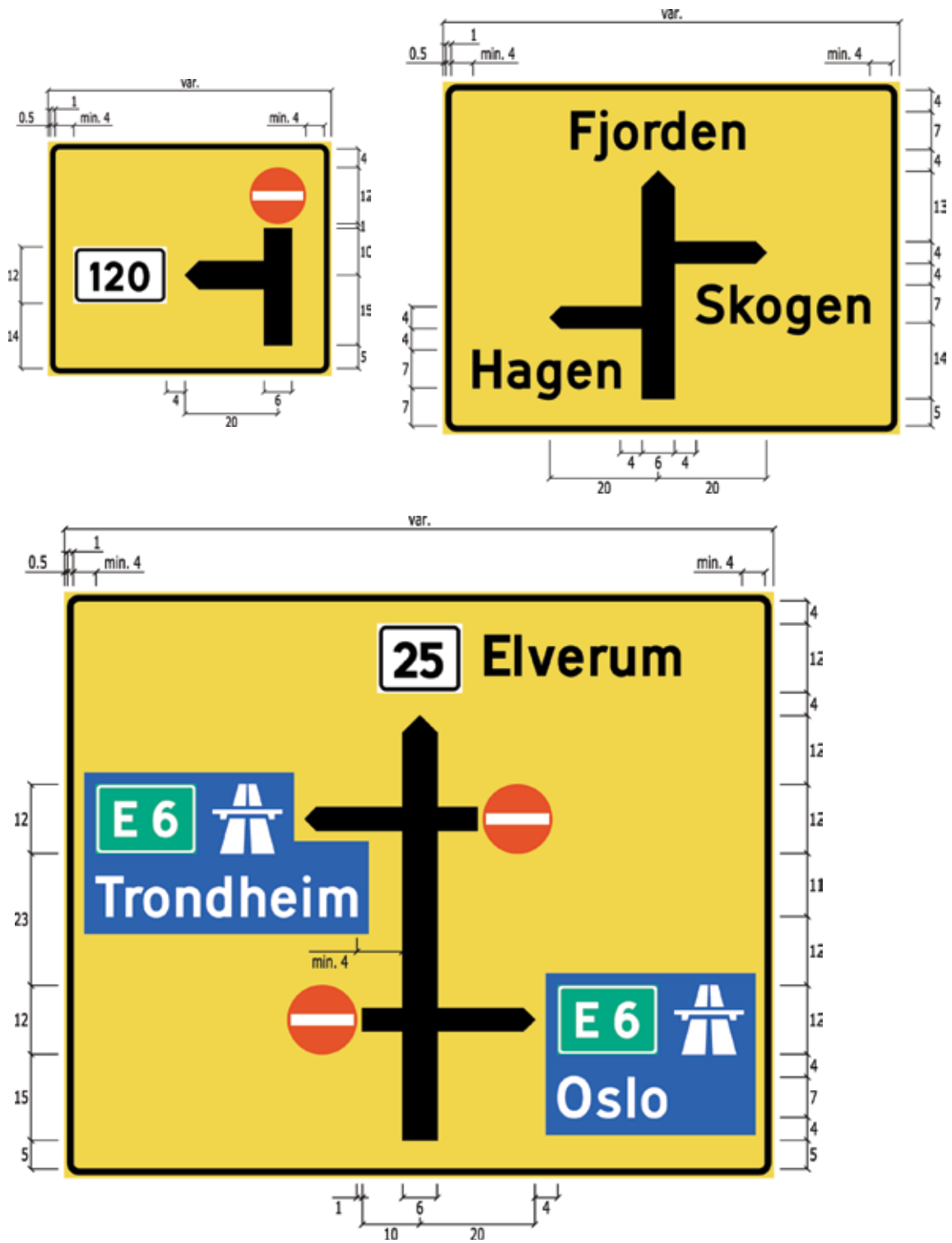
Figur 4-4.17 Eksempler på utforming av diagramorienteringstavle 703.2
