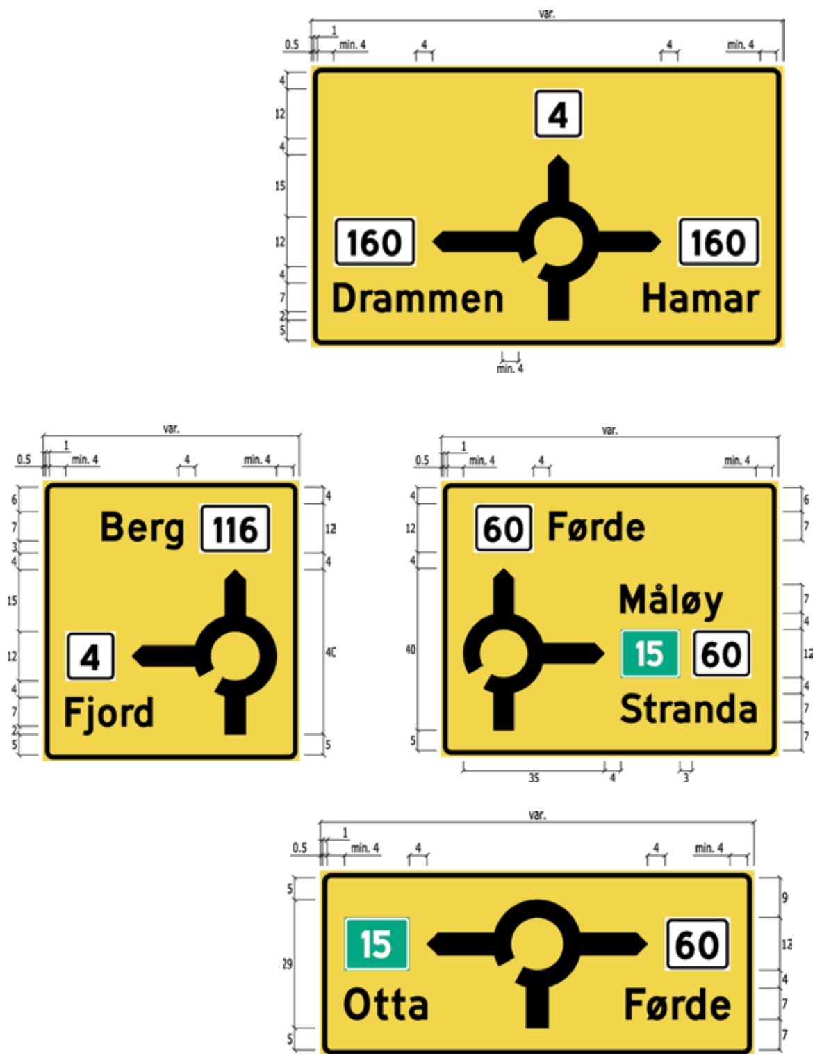
Figur 4-4.16 Eksempler på utforming av diagramorienteringstavle 703.1
