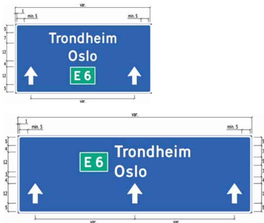
Figur 4-4.29 Eksempler på utforming av skilt 709.2
