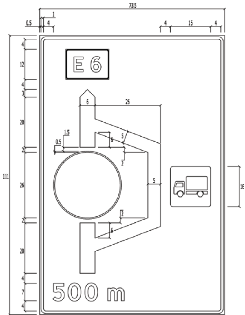
Figur 4-4.65 Eksempel på utforming av skilt 741
