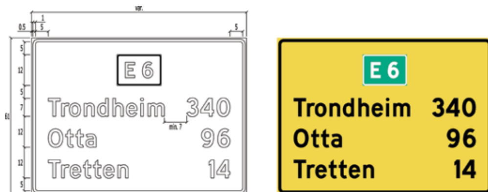
Figur 4-4.56 Eksempel på utforming av skilt 725.1
