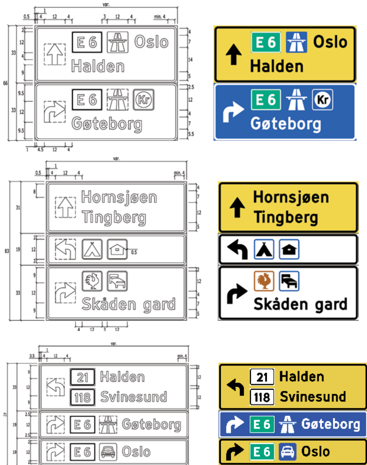
Figur 4-4.13 Eksempler på utforming av tabellorienteringstavle 701.1
