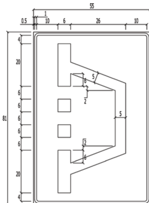
Figur 4-4.66 Utforming av skilt 743.1
