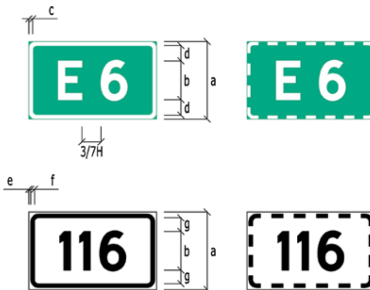
Figur 4-4.48 Eksempler på utforming av vegnummerskilt.
