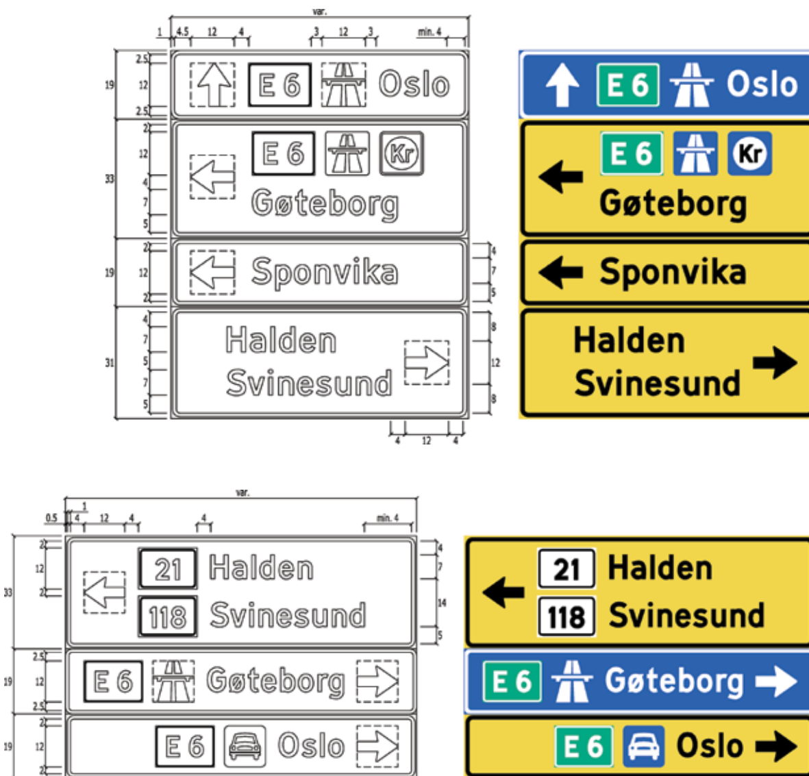
Figur 4-4.35 Eksempler på utforming av skilt 711
