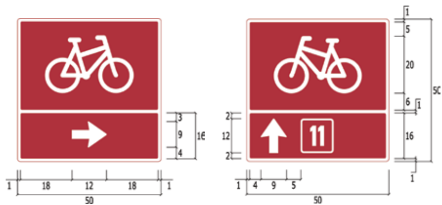
Figur 4-4.76 Eksempler på utforming av skilt 753.1 Alle mål i 1/7 H.
