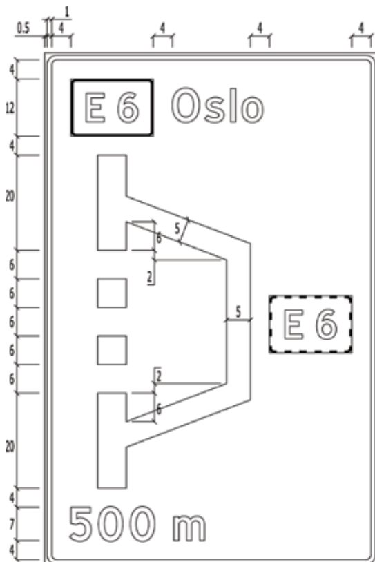
Figur 4-4.67 Eksempel på utforming av skilt 743.2
