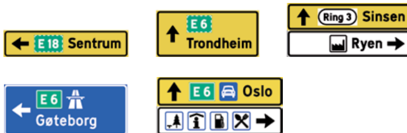
Figur 4-4.40 Eksempler på portalvegviser 719.11
