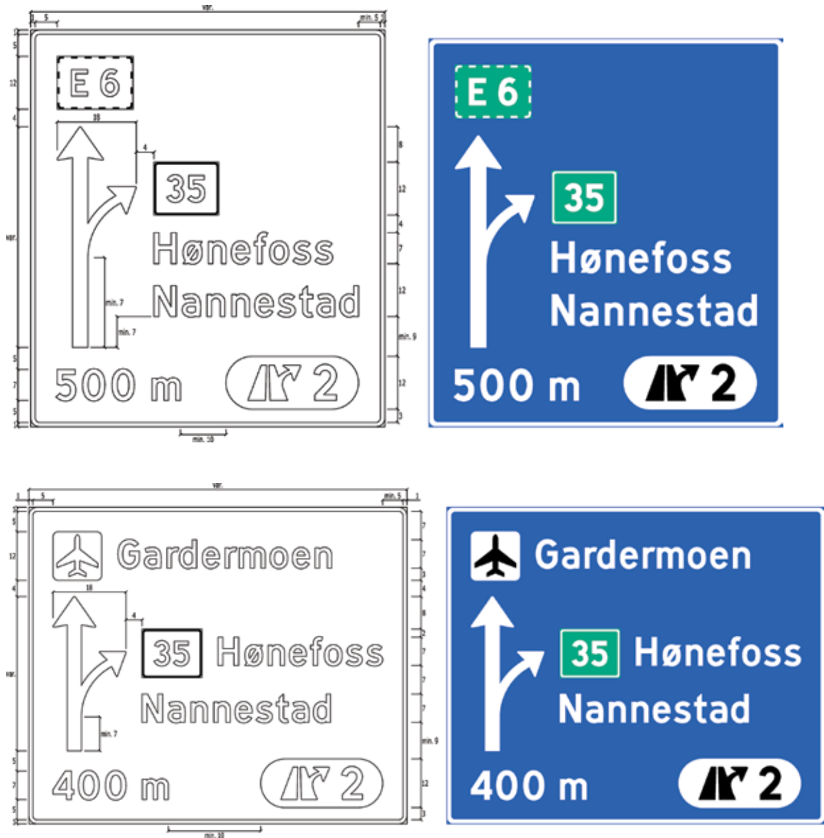
Figur 4-4.19 Eksempler på utforming av avkjøringstavle 705.2
