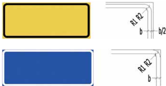
Figur 4-4.2 Standard utforming av lyse og mørke border på vegvisningsskilt. (For enkelte skilt er det fastsatt annen utforming.)
