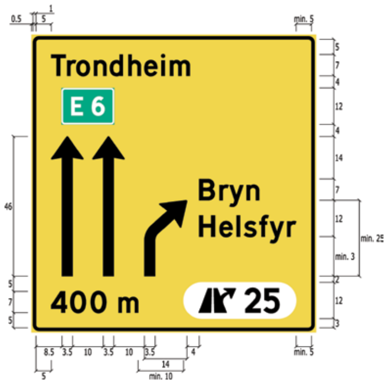
Figur 4-4.23 Eksempel på utforming av kjørefeltorienteringstavle 707.3
