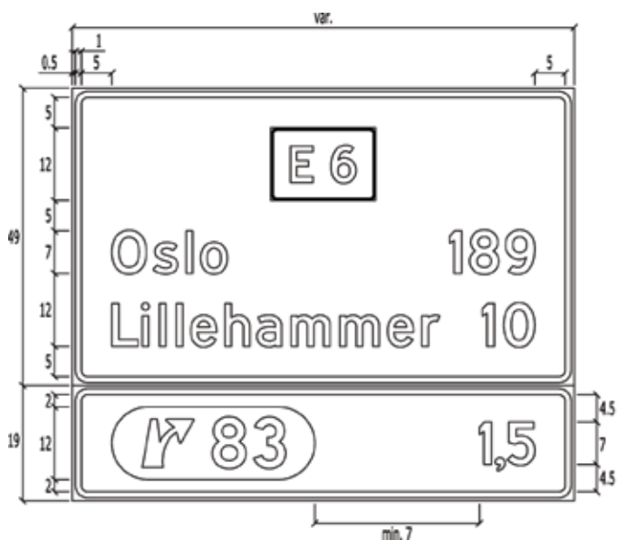
Eksempel på skilt 725.2 på tofelts (motortrafikk)veg.
