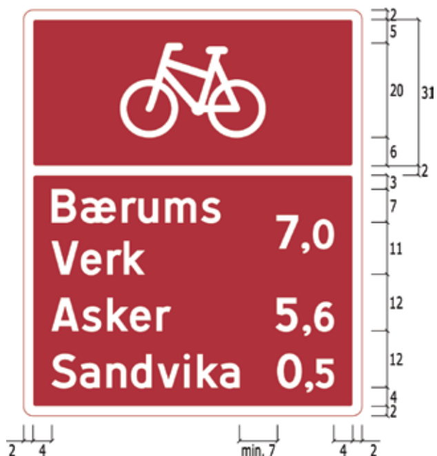
Figur 4-4.82 Eksempler på utforming av skilt 757. Alle mål i 1/7 H.
