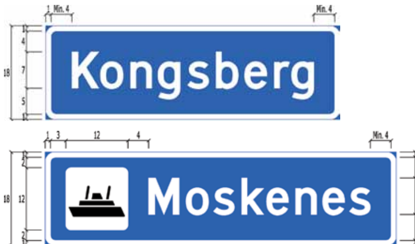
Figur 4-4.58 Utforming av skilt 727.1 og 727.2
