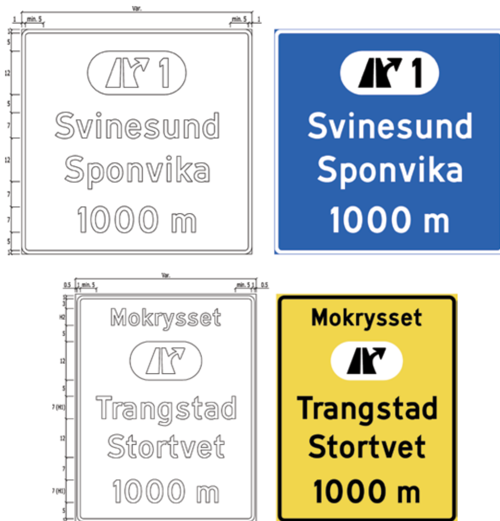
Figur 4-4.18 Eksempler på utforming av avkjøringstavle 705.1
