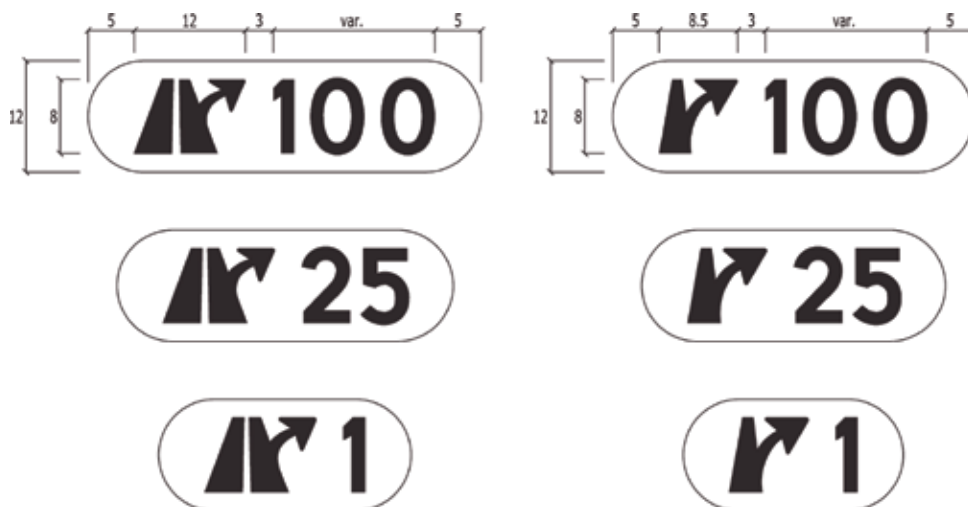
Figur 4-4.55 Utforming av kryssnummer
