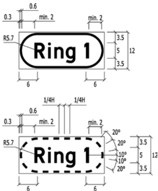
Figur 4-4.54 Utforming av skilt 723.21 og 723.22
