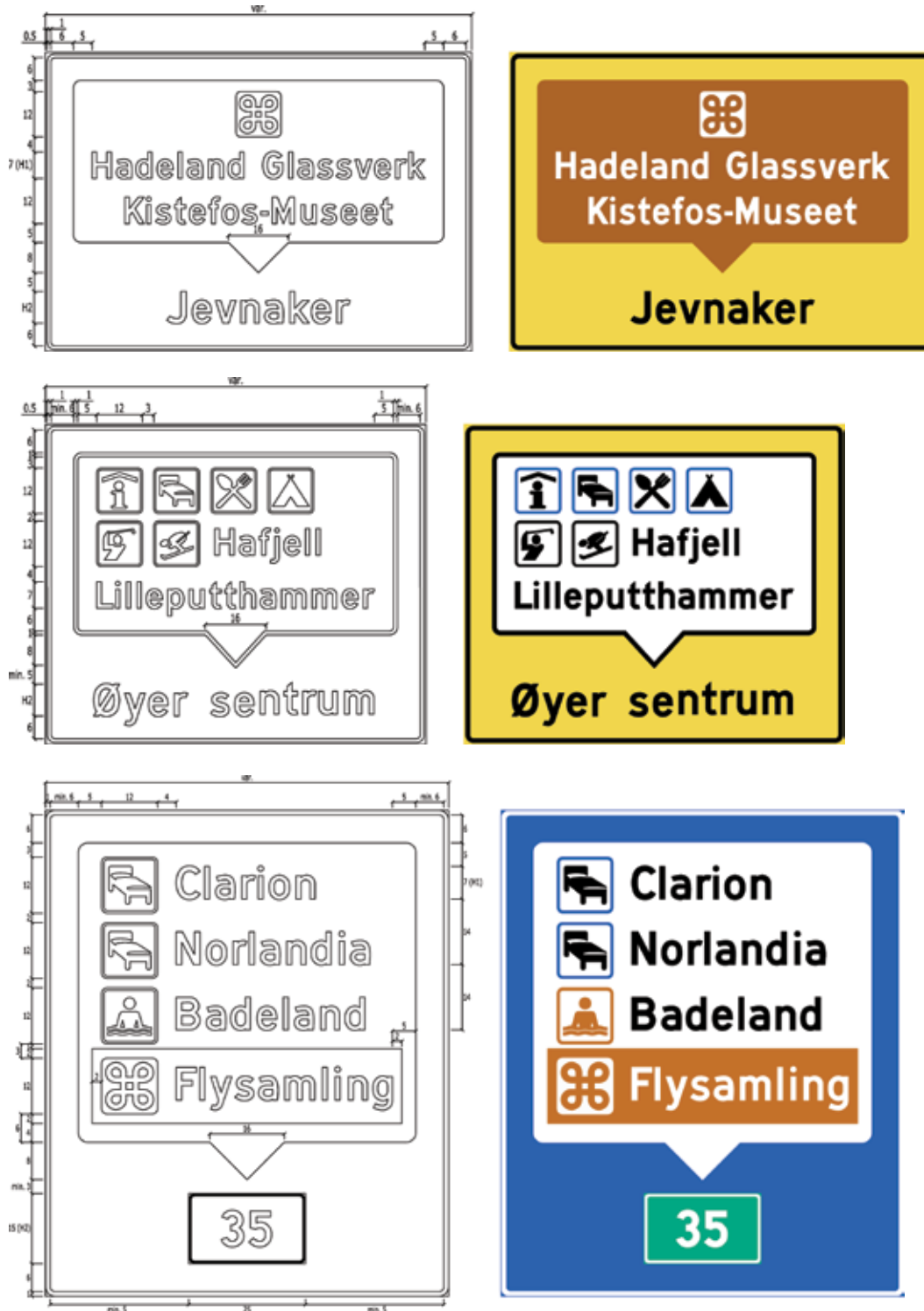
Figur 4-4.64 Eksempler på utforming av skilt 731
