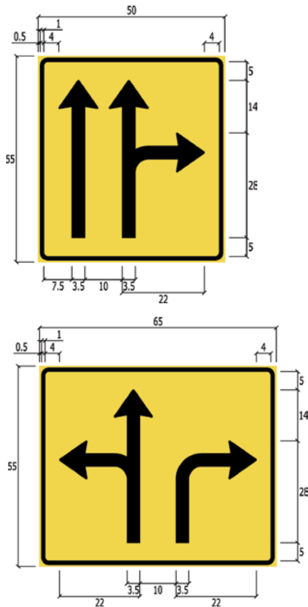
Figur 4-4.21 Eksempler på utforming av kjørefeltorienteringstavle 707.1
