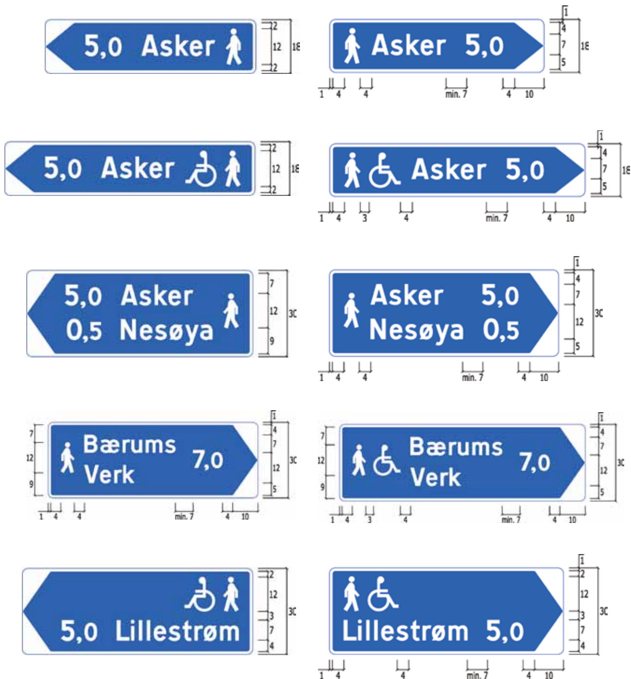
Figur 4-4.69 Eksempler på utforming av skilt 749
