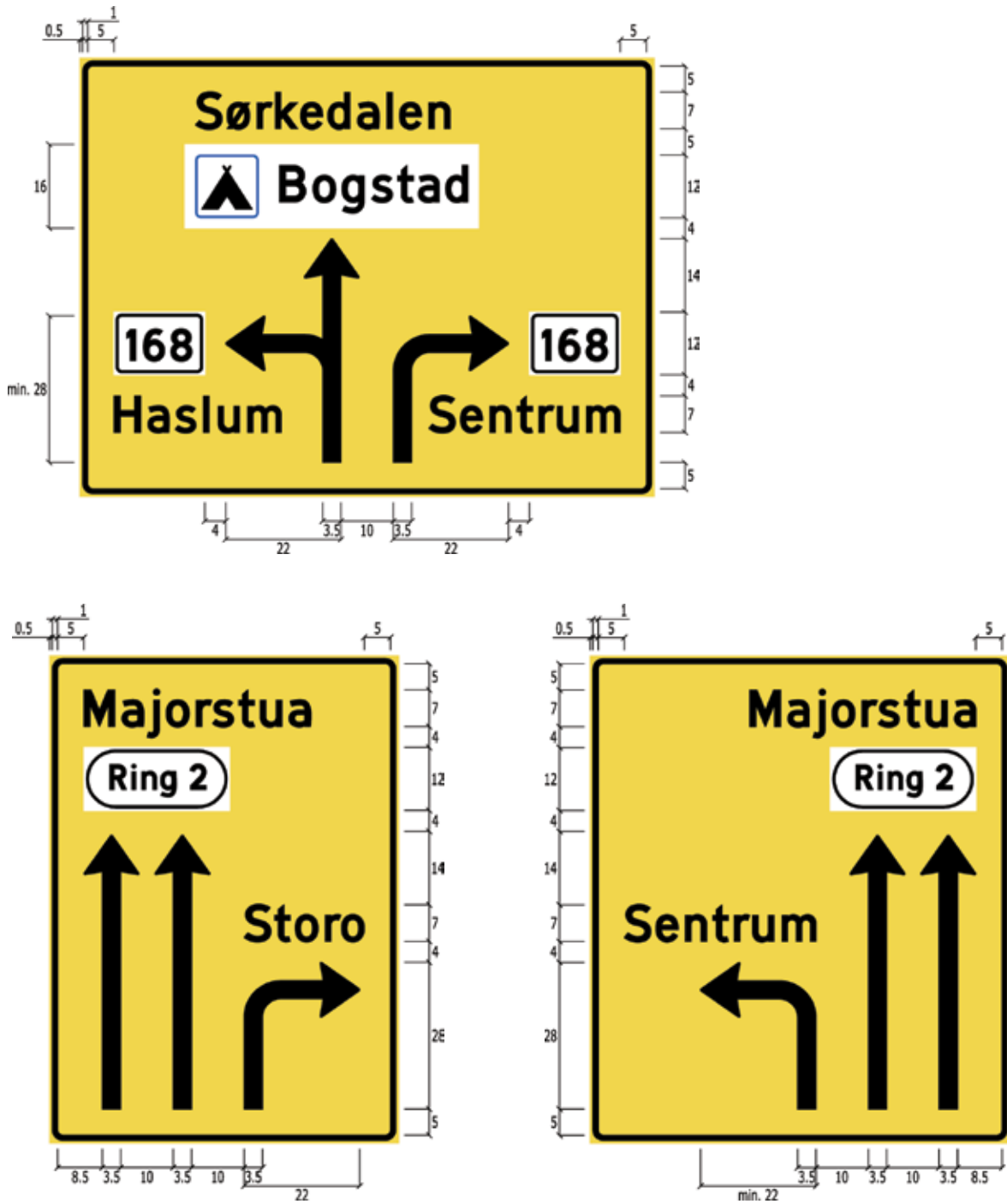
Figur 4-4.22 Eksempler på utforming av kjørefeltorienteringstavle 707.2
