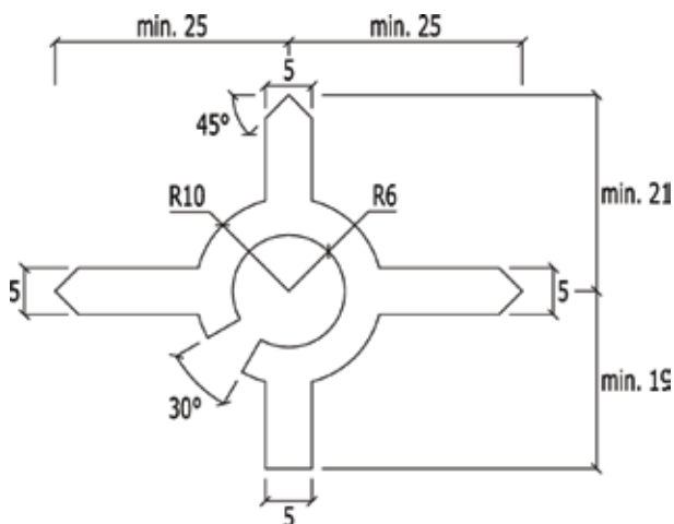
Figur 4-4.15 Standard utforming av symbol for skilt 703.1
