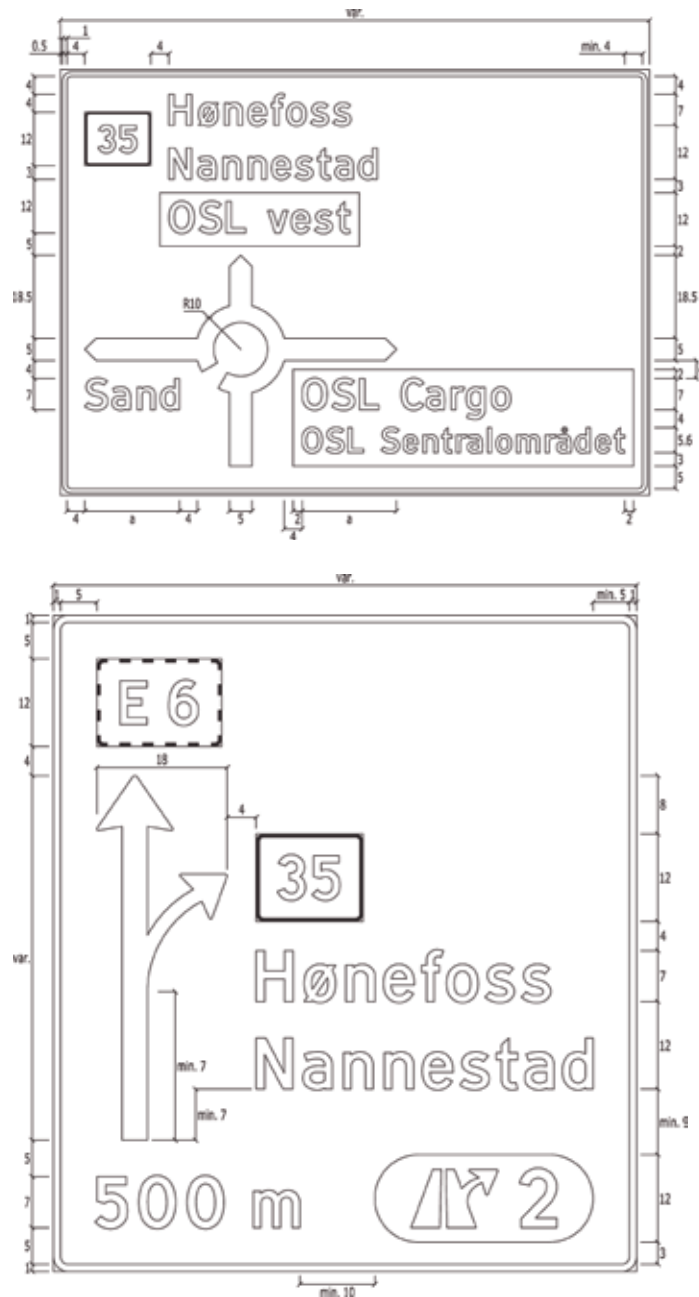
Figur 4-4.9 Eksempler på plassering av visningselementer på diagramskilt
