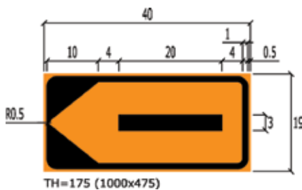
Figur 4-4.36 Eksempler på utforming av skilt 713
