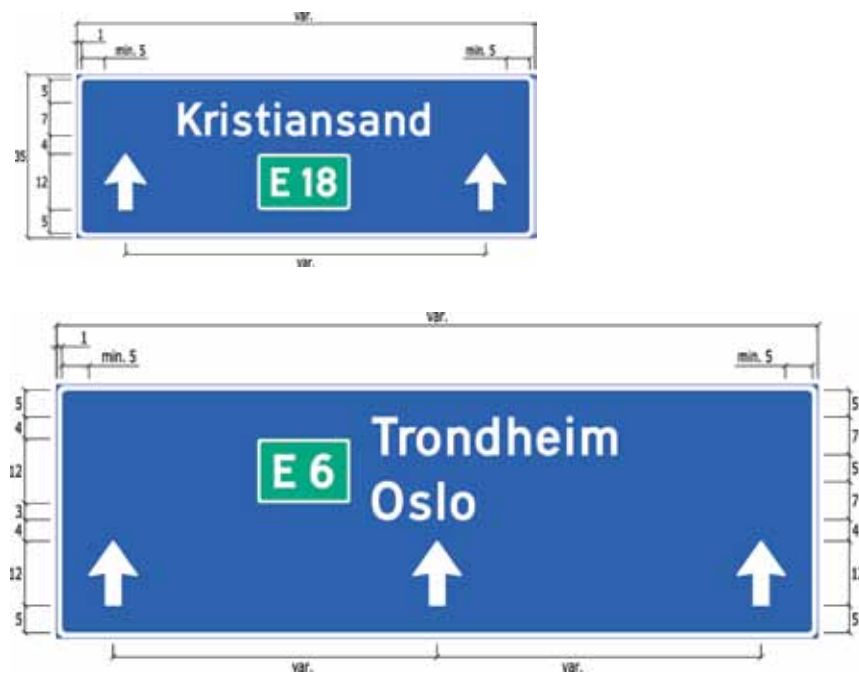
Figur 4-4.44 Eksempler på utforming av skilt 719.2
