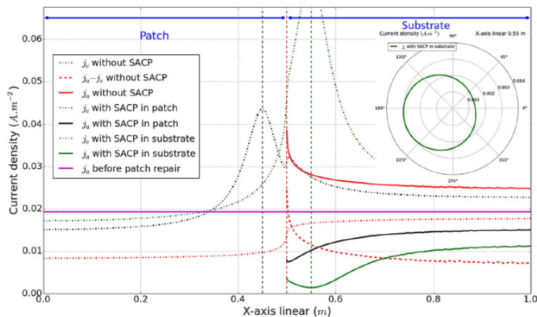
Figur 38. Strömfördelning på armering när offeranod är placerad i reparationsbetong eller originalbetong.
