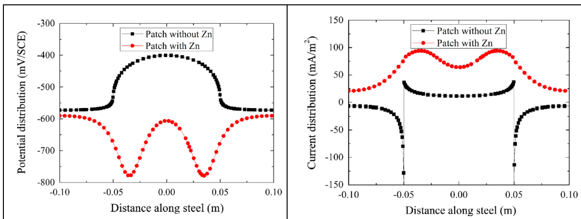
Figur 35. Simuleringsresultat. Vänsterbild: Armeringens potential med och utan offeranod. Till höger: Strömfördelning på armering med och utan offeranod.
