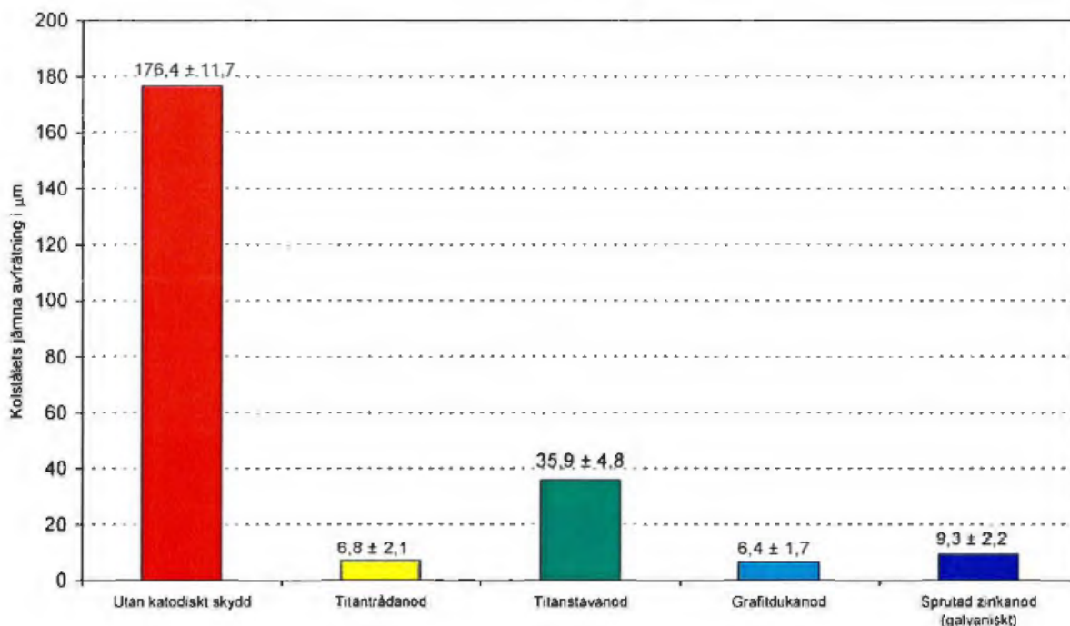
Figur 6B. Medelavrätningen efter två års exponering, uttryckt i µm, hos ingjutna provstänger av kolstål som katodiskt skyddats med olika anodsystem.
