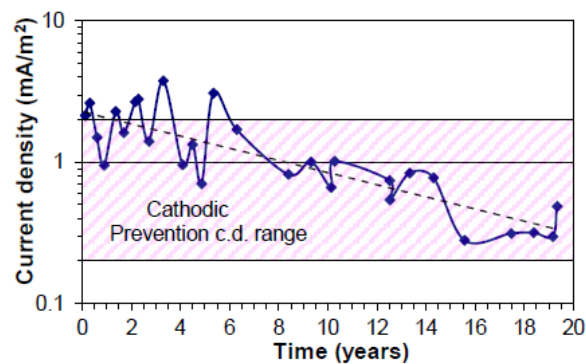
Figur 49. Uppmätta strömmar från anoder som installerats på bro nr 3.
