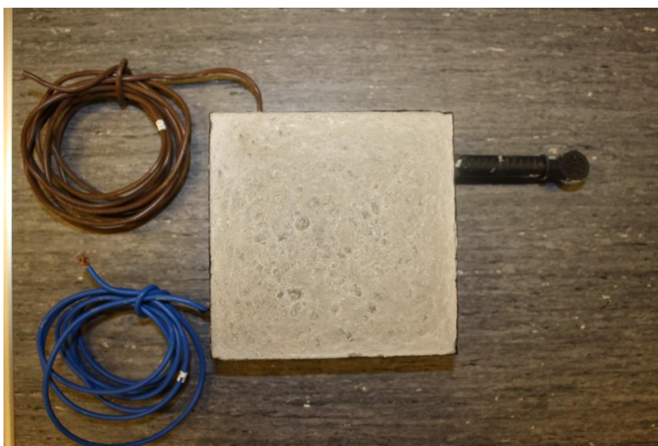
Figur 51B. Provblock efter gjutning och avformning. Den blå kabeln ansluter till stålstångena och den bruna till referenselektroden av titan med ädelmetallskikt.
