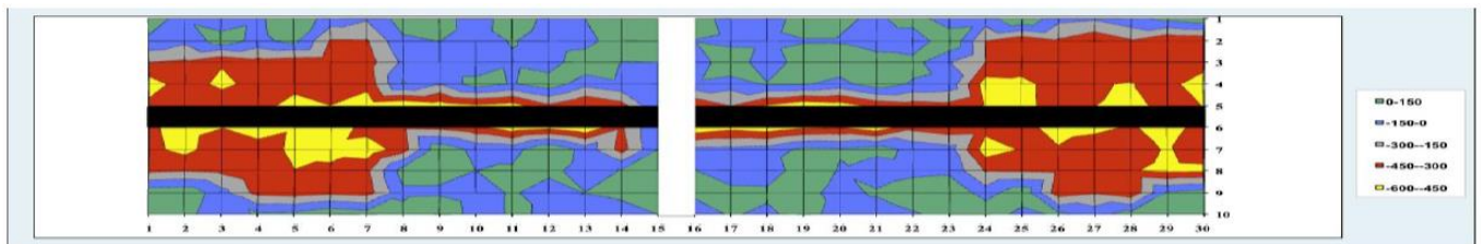
Figur 31. Potentialkartering av fogen på undersidan av bron.
