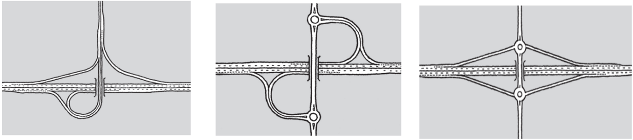
Figur 22: Trompetkryss, halvt kløverbladkryss og ruterkryss [53].
