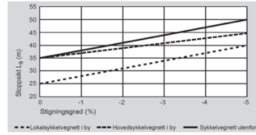
Figur 54: Stoppsikt (Ls) for syklende [8].
