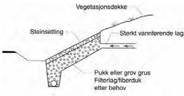
Figur 1.4 Sikring av skråning.
