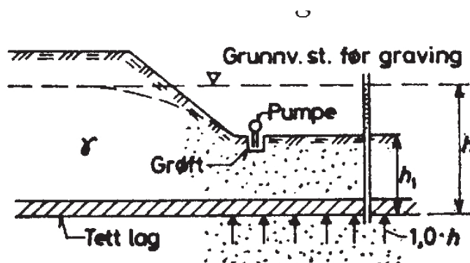
Figur 14.21 Grunnvannsenking ved pumpebunn
