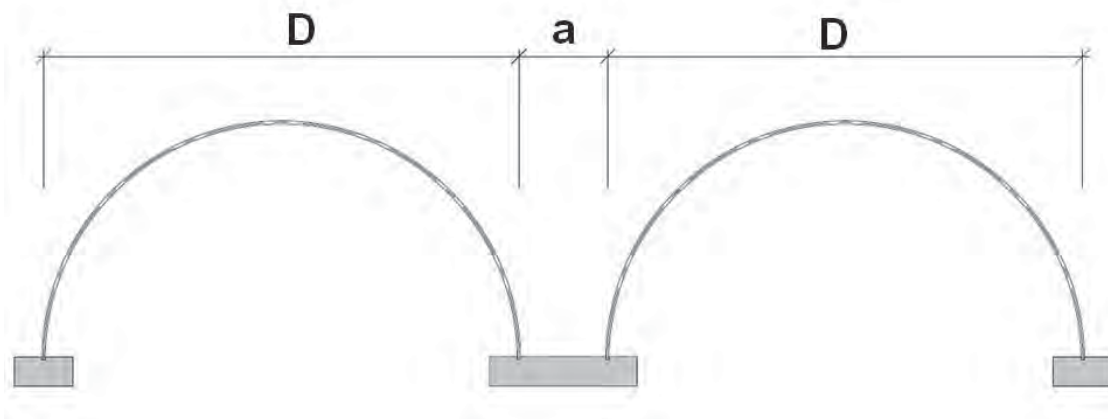
Figur 12. 17 Minimum avstand mellom samvirkekonstruksjoner med flere korrugerte rør som gjelder for samvirkekonstruksjoner bestående av rør av typen B, F og G.
