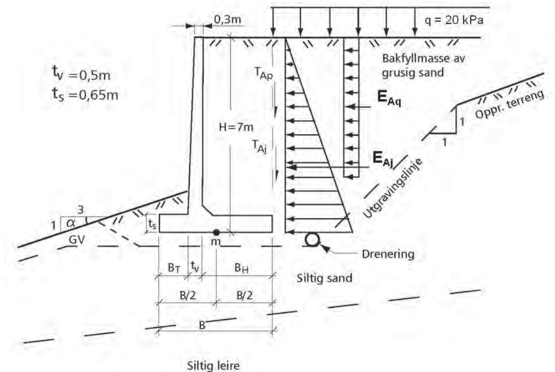
Figur 9.17 Vinkelmur på lagdelt grunn.
