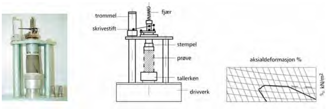
Figur 2.9 Enaksialt trykkapparat.
