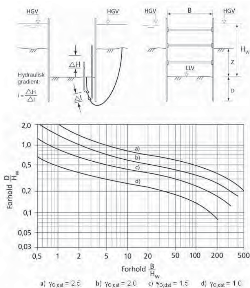
Figur 10. 16 Vurdering av sikkerhet mot hydraulisk grunnbrudd for langstrakt tørrlagt byggegrop mellom avstivede vegger. (Ref. 5)
