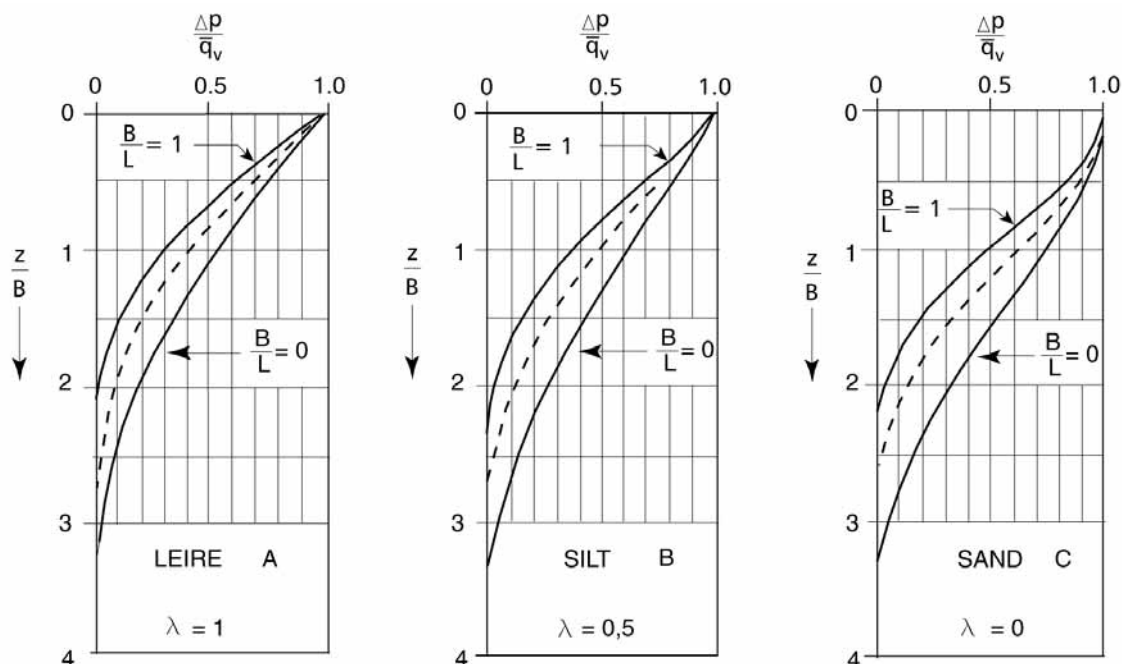
Figur 7.2 Spenningsfordeling for overflatebelastning - plastisk likevektsteori (etter: Janbu 1973; Grunnlag i Geoteknikk, Ref. 8)
