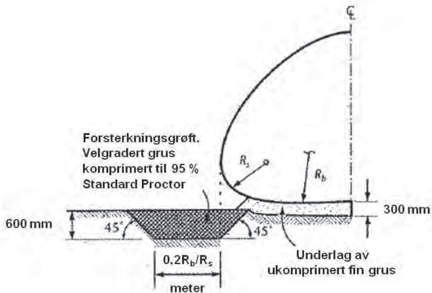
Figur 12. 30 Utskifting og forsterkning av stedlige masser ved flatbunnet rør
