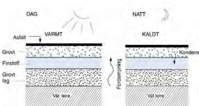
Figur 14.9 Vanntransport ved fordampning / kondens
