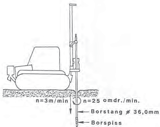
Figur 1.9 Dreietrykksondering.
