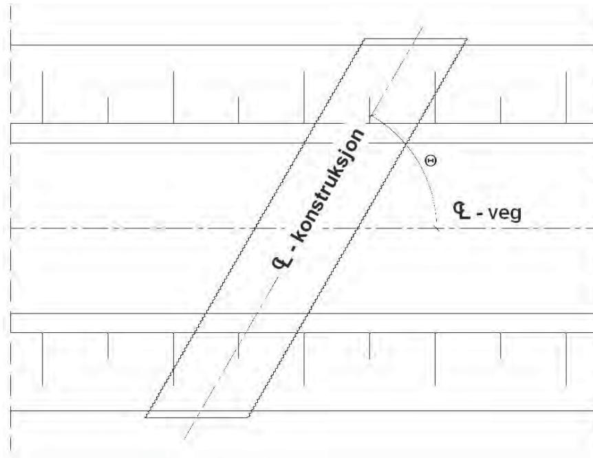
Figur 12. 14 Skjæringsvinkel \Theta mellom veg og konstruksjon
