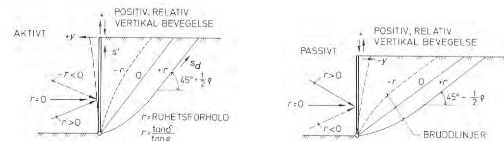
Figur 5.3 Bruddflatenes form ved positiv og negativ ruhet
