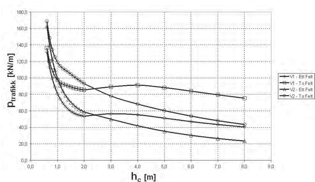
Figur 12. 23 Beregnet ekvivalent linjelast fortrafikklast for lasttype V1 og V2
