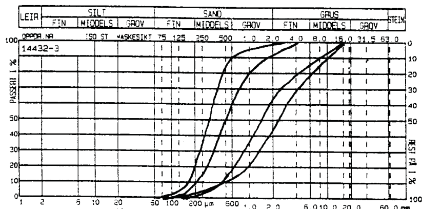
Figur 3.9 Siktekurver i breelvmateriale.
