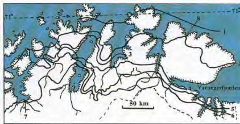
Figur 3.4d Breerandtrinn i Finnmark. Trinnet som går gjennom Alta (7) tilsvarer Raet (6). (Andersen 2000, Ref. 5).
