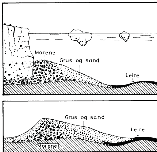
Figur 3.3: Øverst: Raet under dannelse der iskanten lå i havet. Isen skyver sammen en rygg av løsmateriale på sjøbunnen, samtidig som smeltevann avsetter grus, sand og leire. Nederst: Landhevningen løfter Raryggen opp til havnivå der den jevnes ut av bølgene. (Østerås 1974, Ref. 22)
