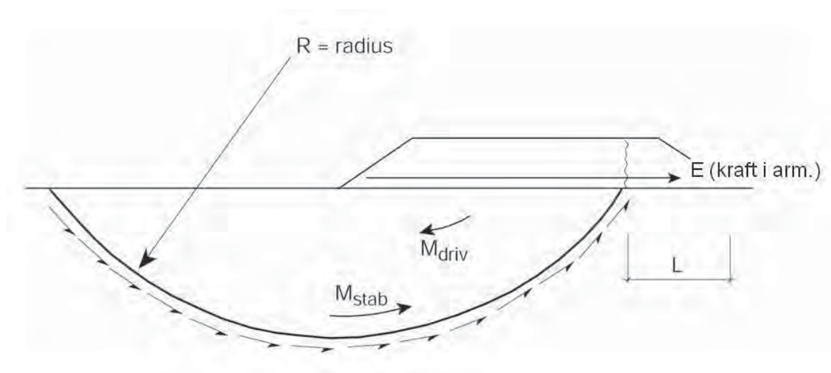
Figur 16.37 Glidesnitt - beregning av totalstabilitet.
