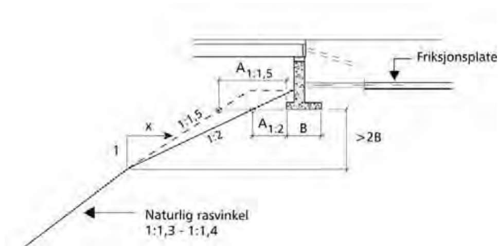
Figur 6.11 Fundament på steinfylling
