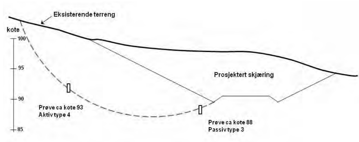
Figur 2.31 Vegskjæring - Skisse av problemstilling
