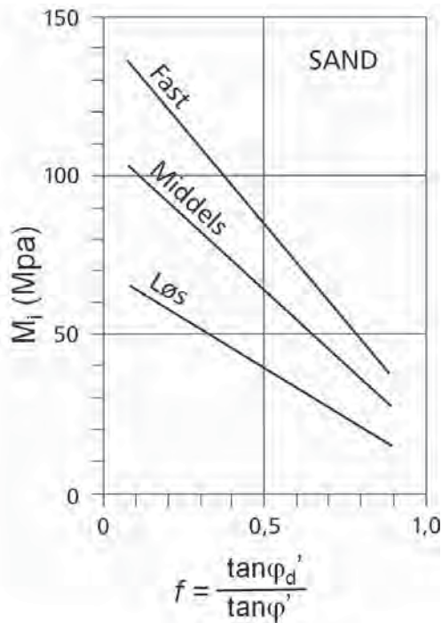
Figur 2.45 Initiel deformasjonsmodul for sand
