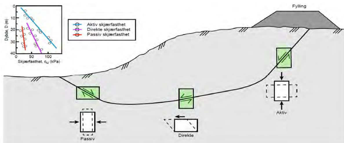
Figur 4-6 Anisotrop spenningstilstand i skråninger
