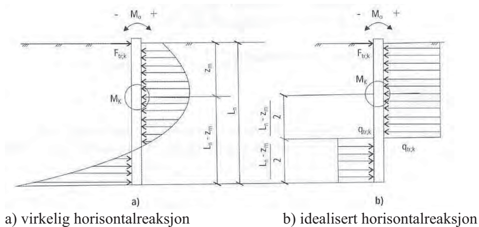
Figur 11.19 Fordeling av horisontal reaksjonskraft ved pel belastet sideveis
