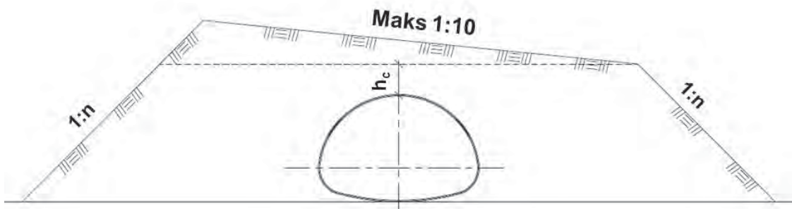
Figur 12.20 Største tillatte helning på terrenget over rørkonstruksjon
