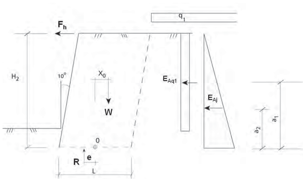
Figur 16.44 Ytre stabilitet.
