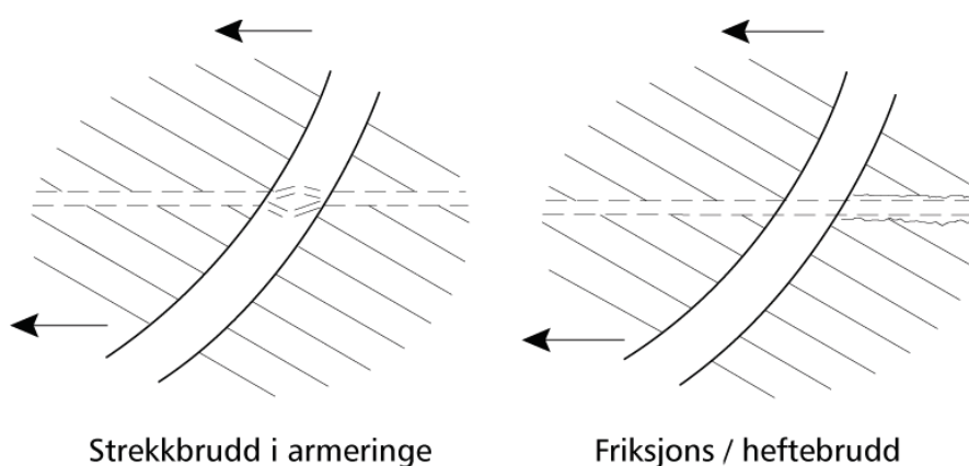
Figur 16.10 Indre Stabilitet.
