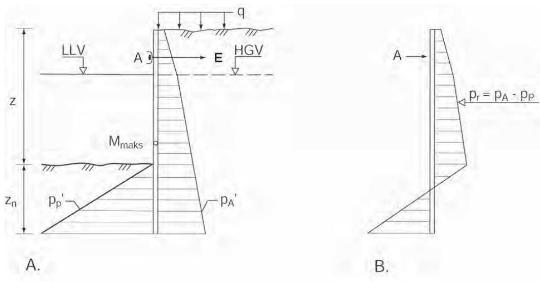
Figur 10.7 Prinsipp for håndregning (effektivspenning) av forankrede spuntvegger
