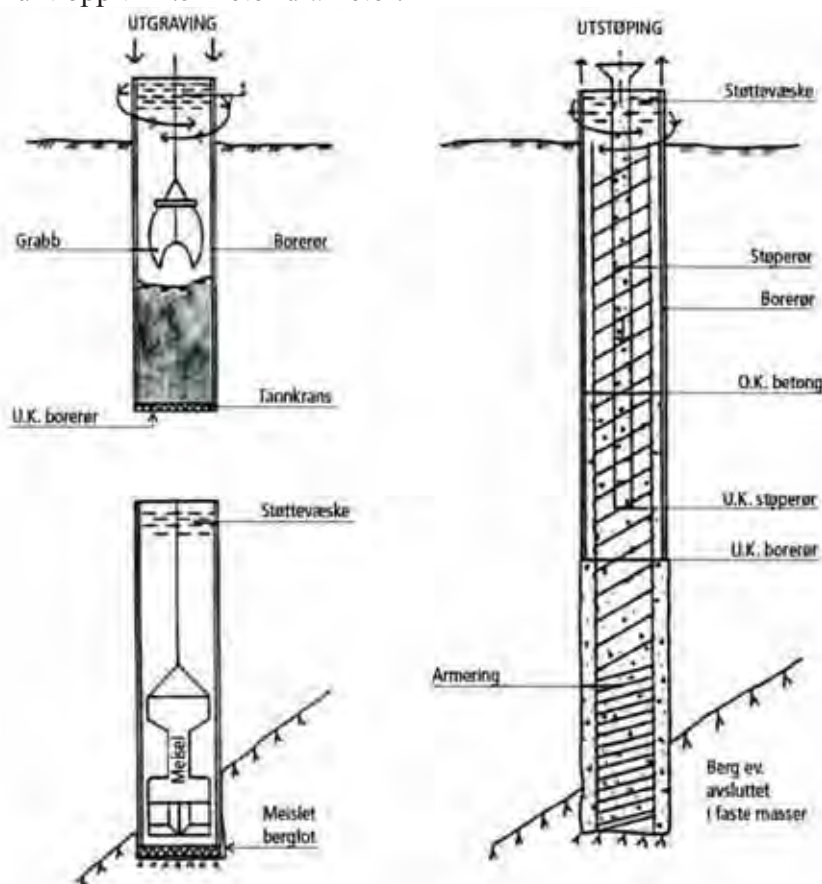
Figur 11. 36 Borede peler uten massefortrengning (kopi av figur i Ref. 3)
