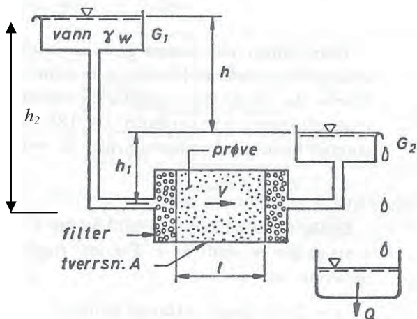
Figur 14.5 Darcy's eksperiment for måling av vannstrøm pr. tidsenhet og permeabilitet.
