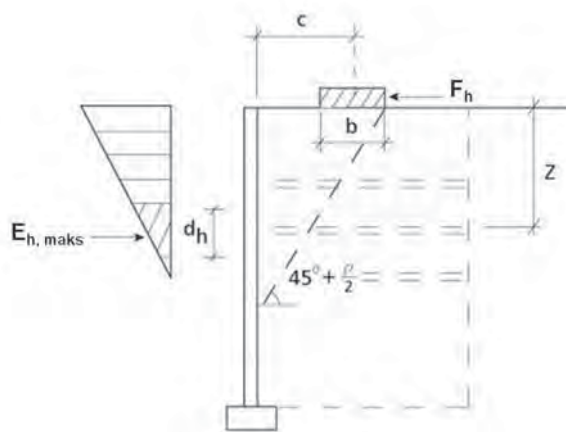
Figur 16.17 Horisontal linjelast.
