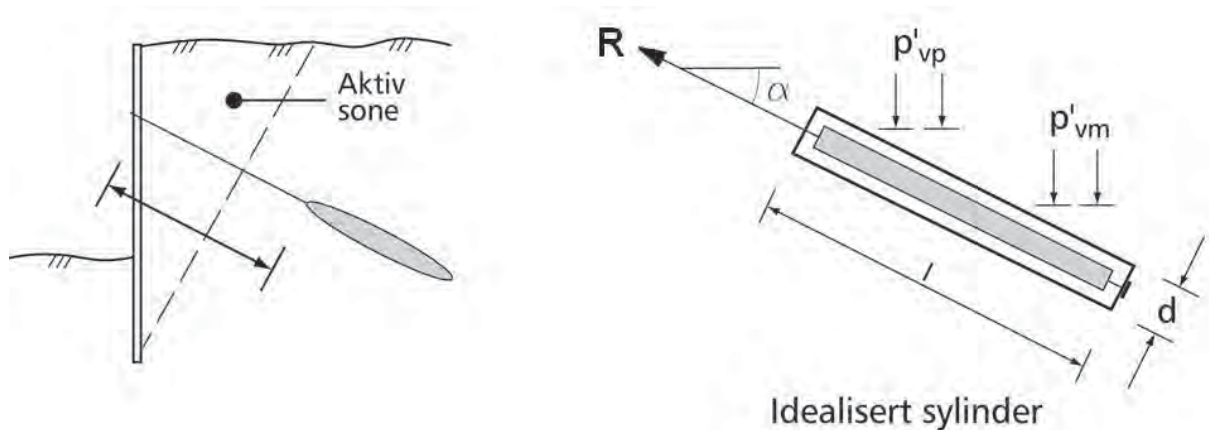
Figur 10. 26 Løsmassestag.
