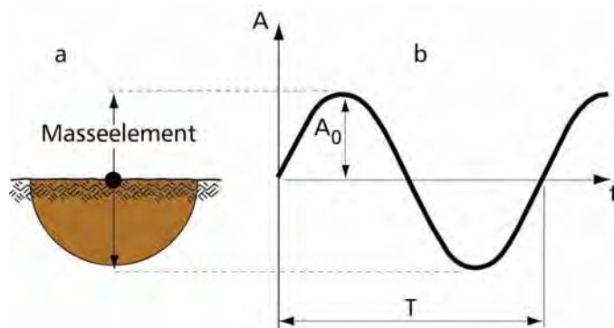
Figur 17.1 Harmonisk svinging
