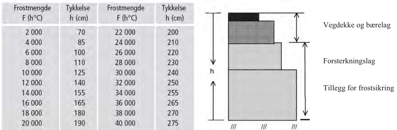
Figur 13.17 Tabell for frostsikring av veger med sand, grus og stein (fra Hb N200, 2011).
