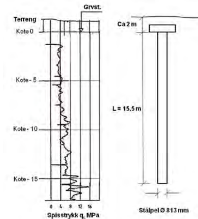
Figur 11. 13 Regneeksempel for åpen stålrørspel basert på CPTU-måling i friksjonsmasser
