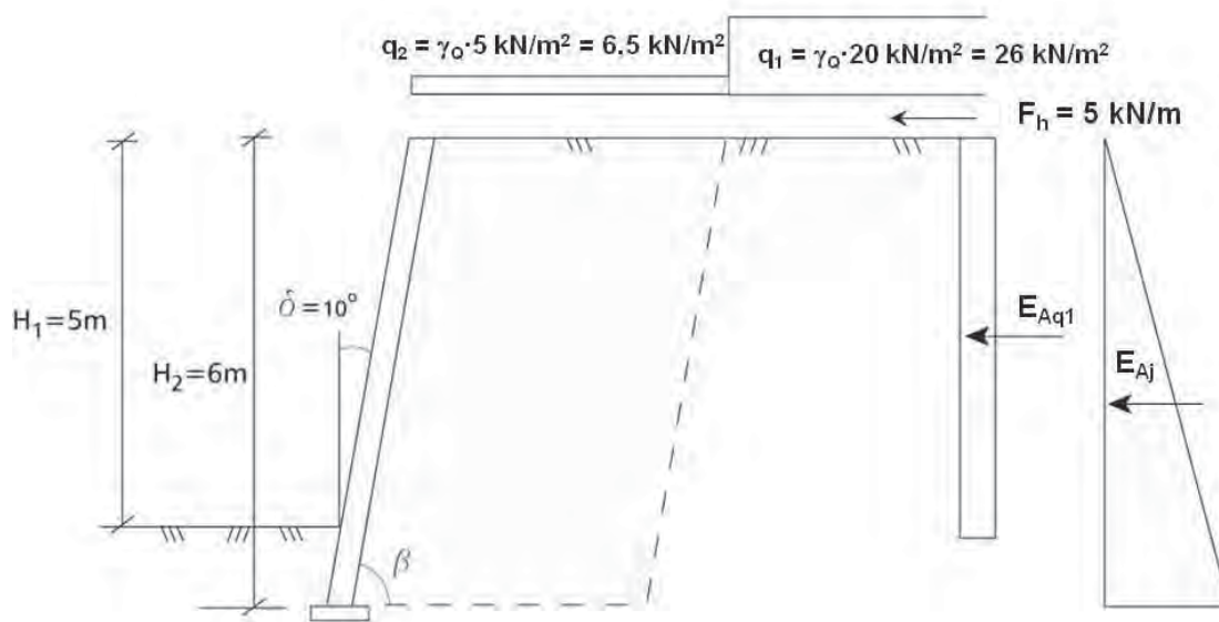
Figur 16.43 Støttekonstruksjon i armert jord.
