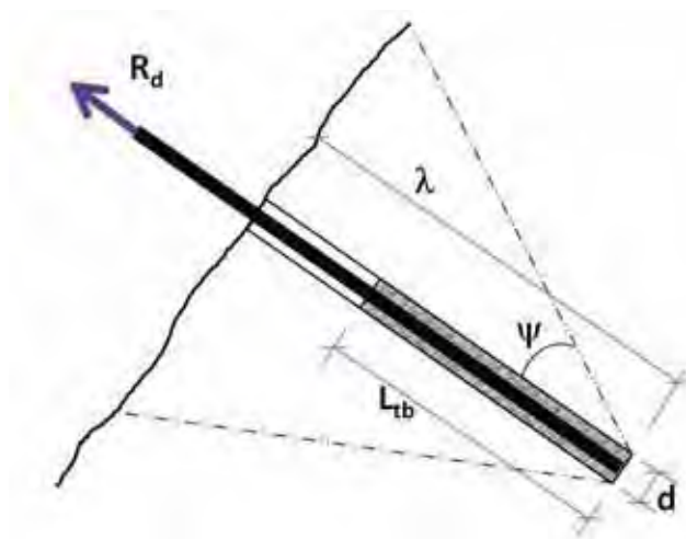
Figur 10. 35 Nødvendig forankringslengde \lambda og L_{tb} i berg.
