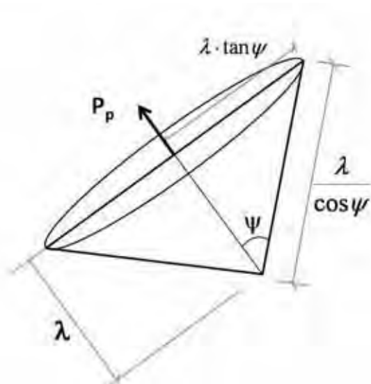
Figur 10. 20 Antatt form på uttrekslegeme.
