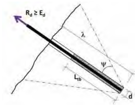
Figur 10. 18 Forankringslengde i berg
