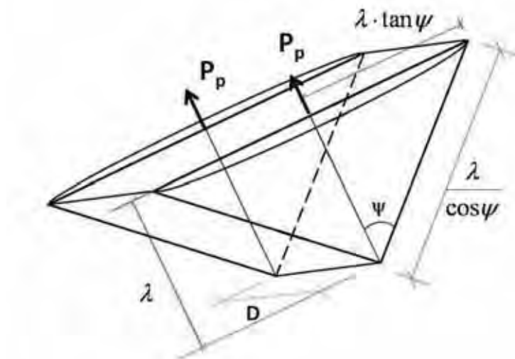
Figur 10. 25 Antatt forenklet bruddlegeme ved begrenset antall stag på rad
