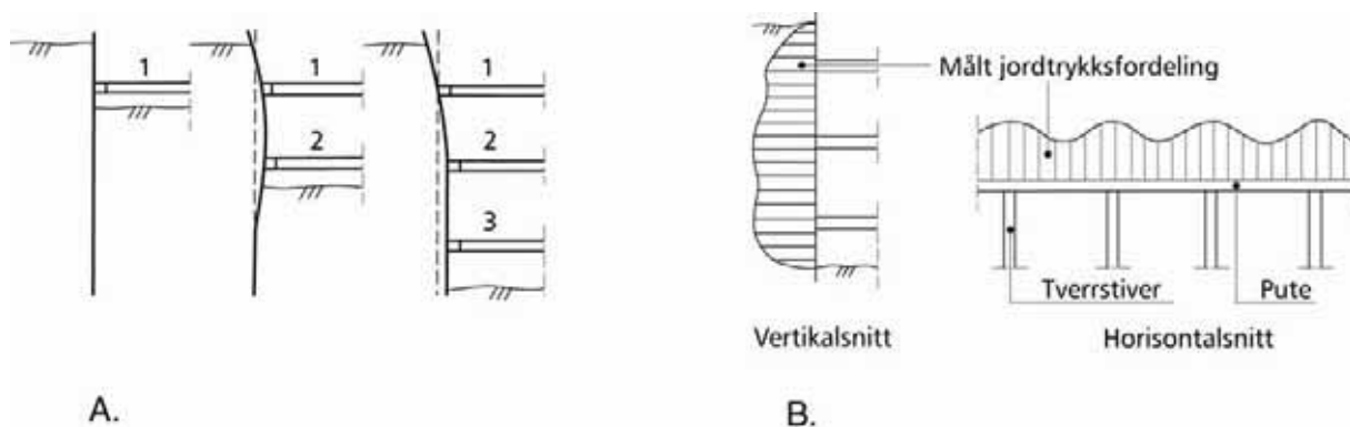
Figur 10. 9 a) Prinsippskisse av deformasjoner ved forskjellige gravestadier. b) Målt jordtrykksfordeling langs veggen.
