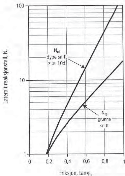
Figur 11.20 Sideveis reaksjonstall for a - \varphi analyse
