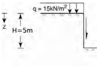
Figur 5.14 Prinsipp-skisse - horisontalt terreng.
