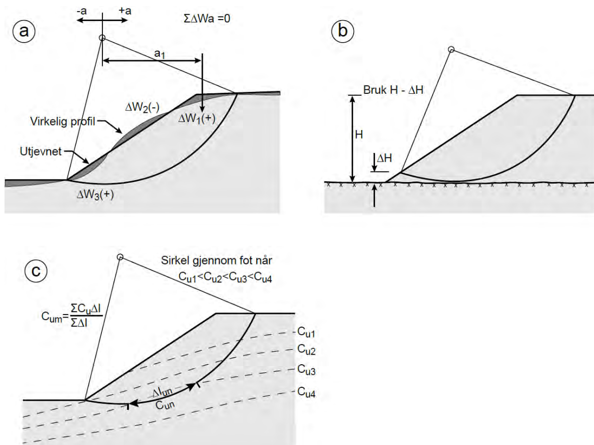
Figur 4-9 Idealisering av profiler i direkte metoden. Modifisert etter Hjeldnes (Ref. 8)
