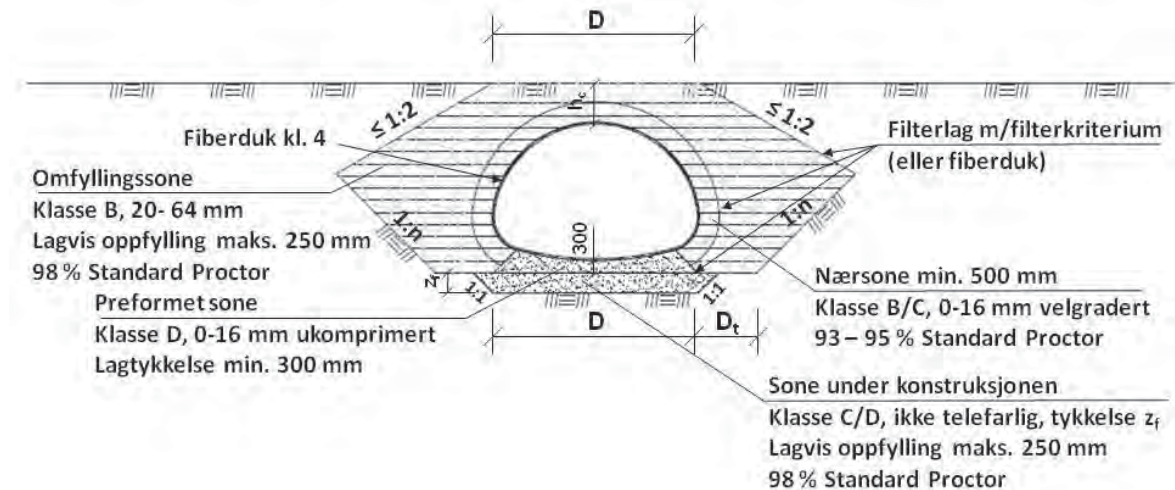
Figur 12. 29 Krav til omfyllingssoner, materialer og komprimeringsgrad
