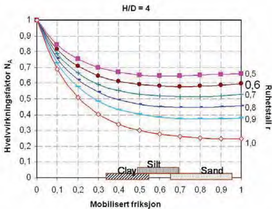
Figur 12.3 Hvelvinningsfaktoren N_A for \frac{H}{D} = 4
