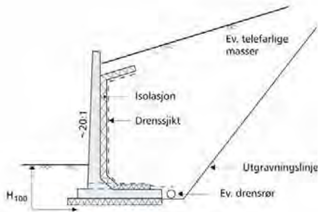
Figur 13.24 Frosssikring med isolasjonsplater.
