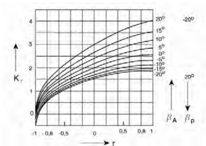
Figur 5.7 Totalspenningsanalyse, jordtrykkskoeffisienten K_r (etter NTNU).
