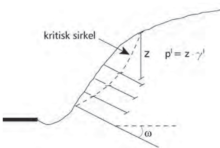
Figur 16.26 Dimensjonering av naglenes forankringskapasitet.
