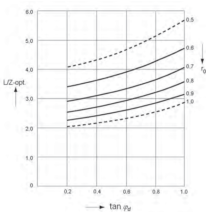
Figur 9.15 Optimal plate lengde (Døssland, 1980).
