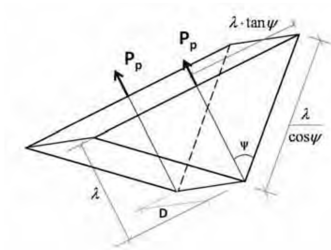
Figur 10. 24 Antatt forenklet bruddlegeme ved mange stag på rad
