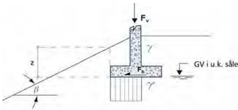
Figur 6.7 Fundament i hellende terreng, effektivspenningsanalyse.
