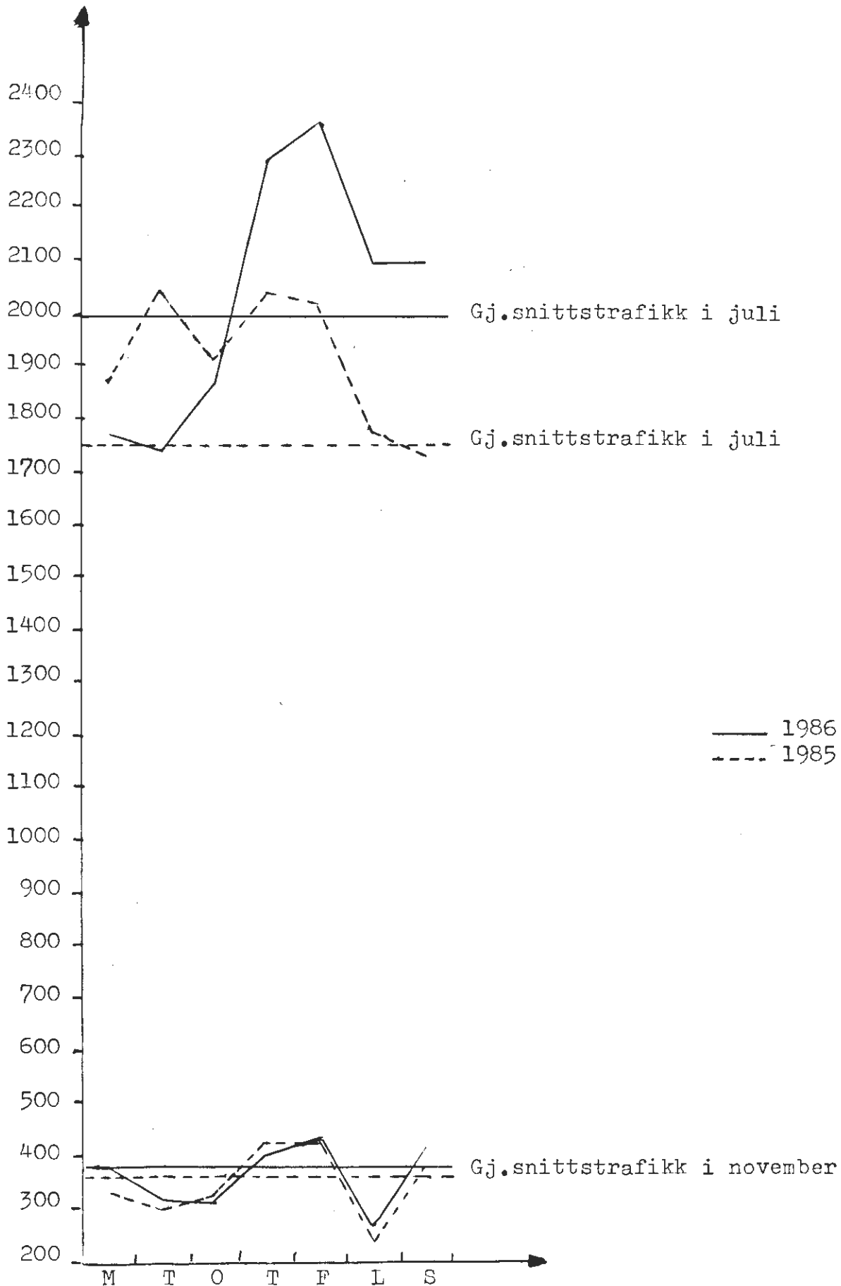
Fig. X . Døgntrafikk i personbilenheter i en uke i juli og en uke i november 1985 og 1986 Ferjestrekningen Bognes - Skarberget
