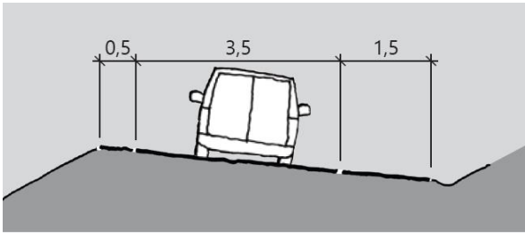
Figur D.18: Rampens tverrprofil (mål i m)
