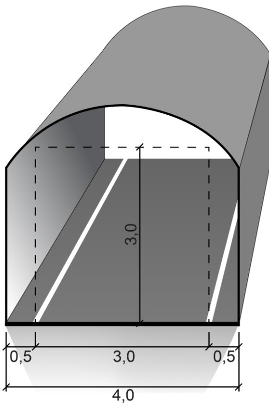
Figur V1.17 Tunnelprofil T4 (mål i m). T4 brukes for gang- og sykkelveger. T4 brukes for gangbare tverrforbindelser mellom tunneløp og for nødutganger ut av tunnel
