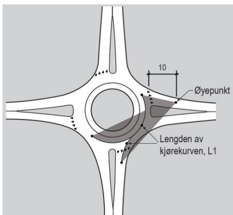
Figur D.14: Sikt til venstre for tilfarten (bakover i rundkjøringen) (mål i m)
