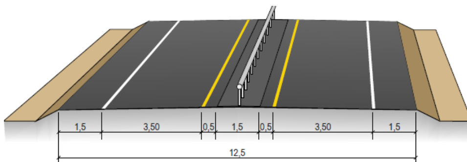
Figur C.2: Tverrprofil for H5, bredde 12,5 (mål i m)
