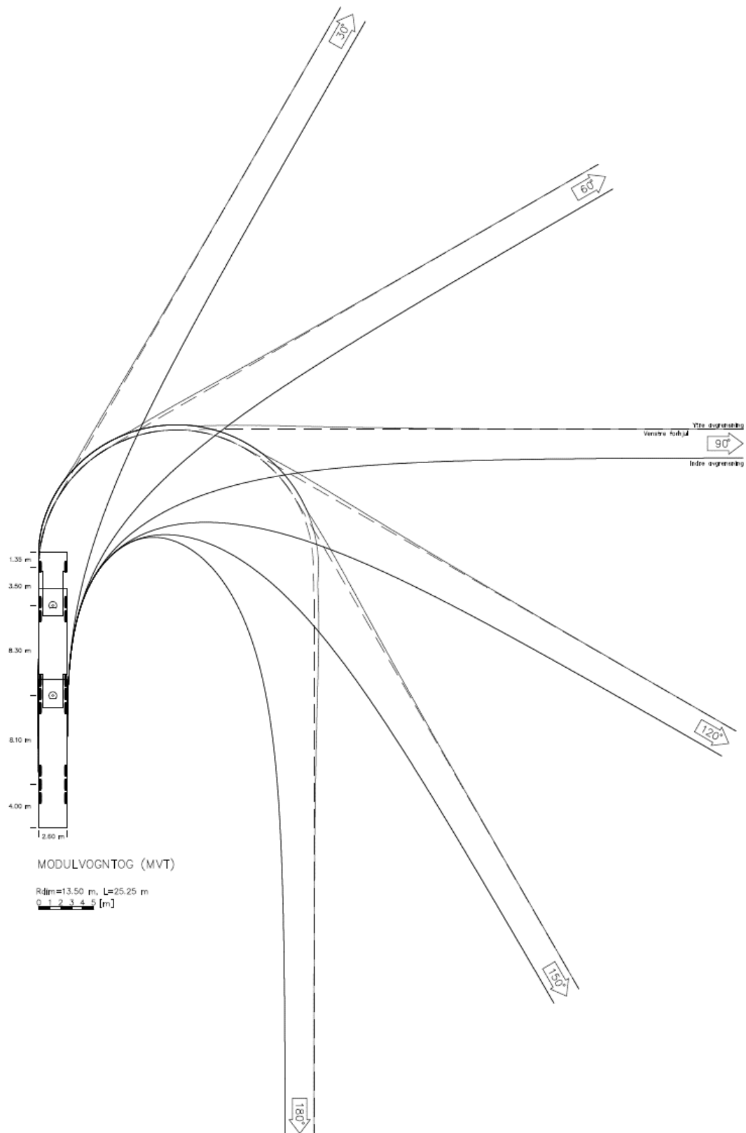
Spingskurve modulvogntog (.dwg)
