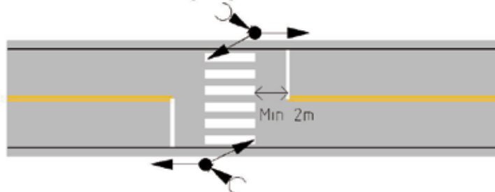
D: Enkeltstående gangfelt, Puffin
