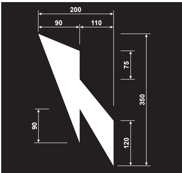
Figur 3.6 Utforming og dimensjoner for 1034.F piler for feltskifte (mål i cm)
