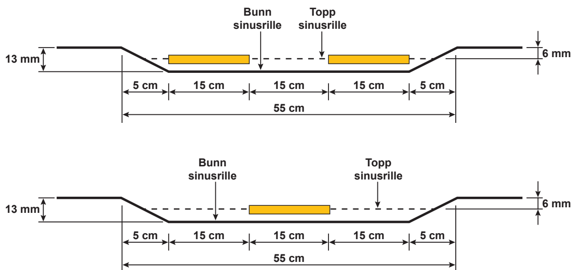
Figur 6.2 Utforming av fresespor med 0,55 m bredde
