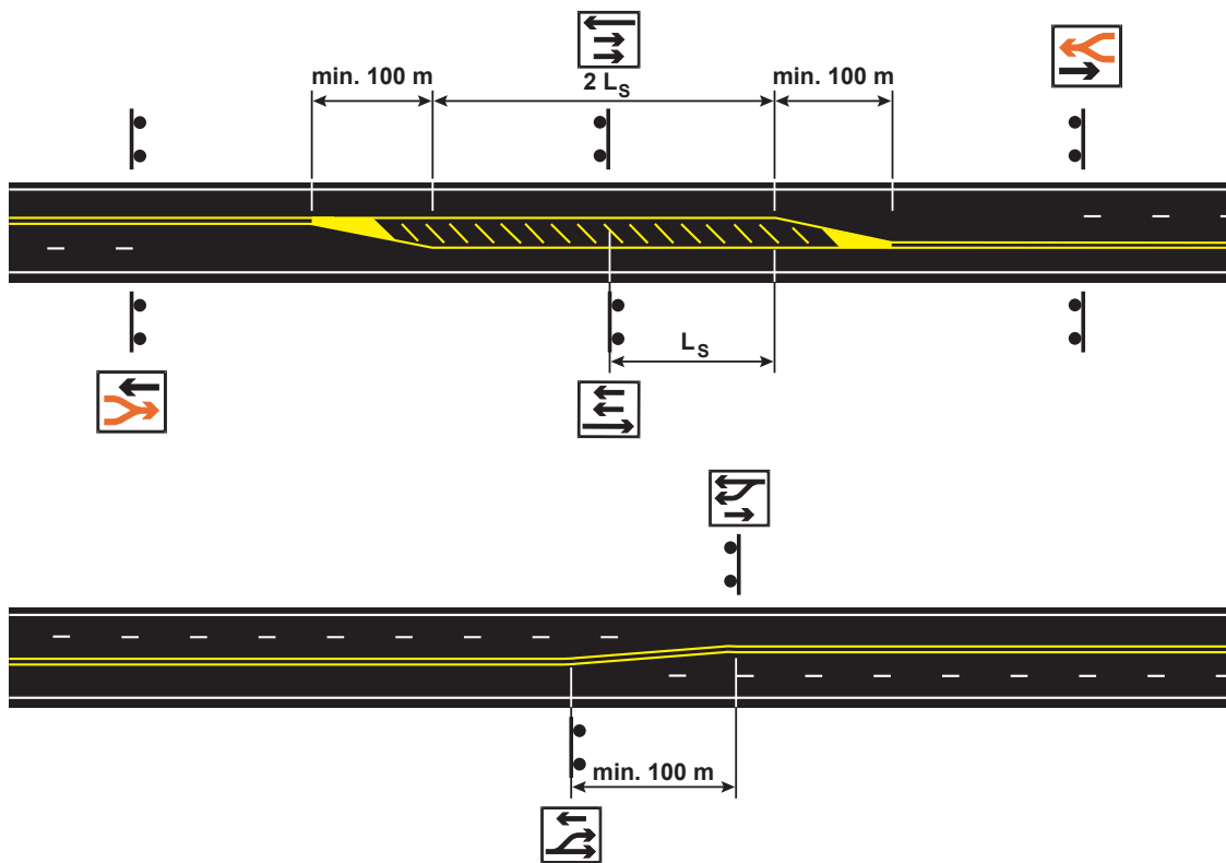
Figur 5.4 Krav til oppmerking ved veksling av kjøreretning i midtfeltet på 3-feltsveg
