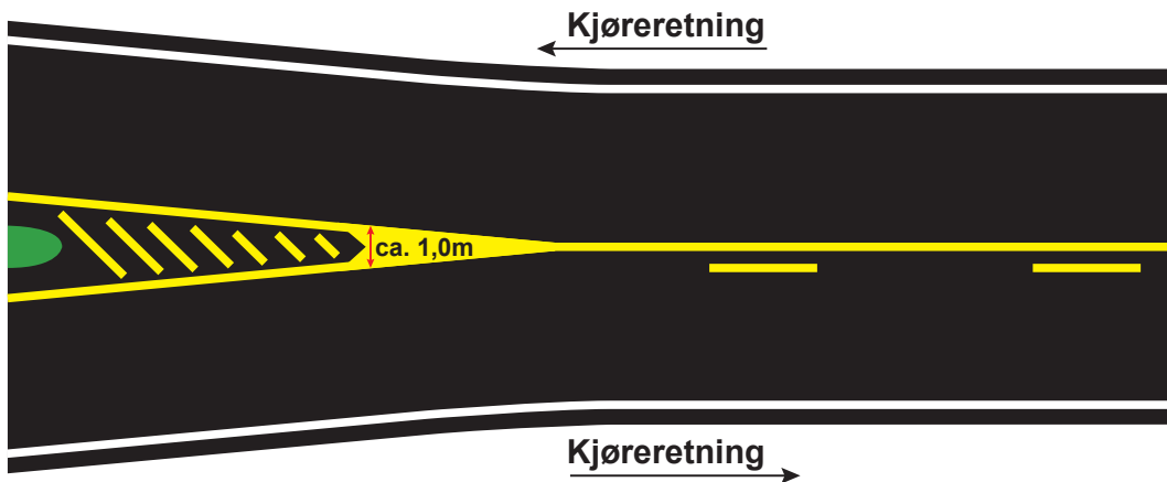
Figur 3.2 Utforming og dimensjoner for sperreområde mellom trafikk i samme kjøreretning
