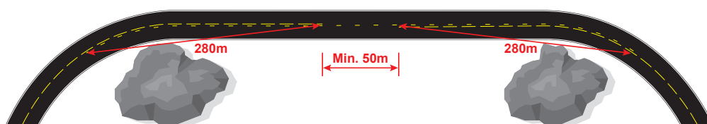
Figur 4.2 Kjørefeltlinje mellom kombinasjonslinjer
