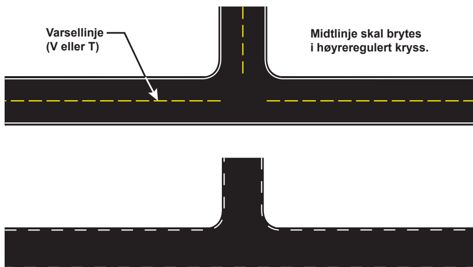
Figur 7.2 Høyreregulert kryss
