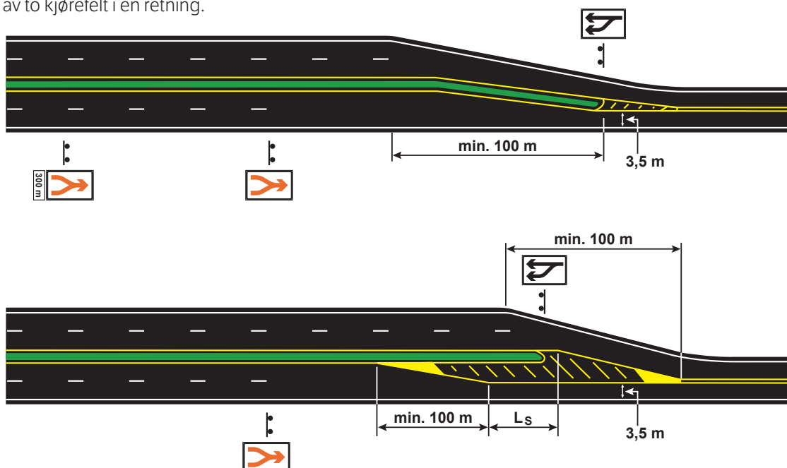
Figur 5.6 Oppmerking av overgang mellom 4-feltsveg og 2-feltsveg
