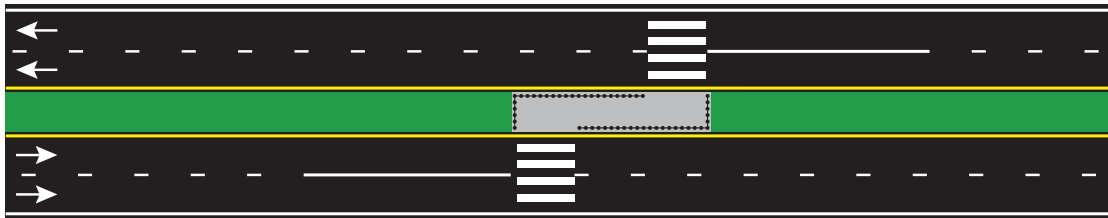
Figur 8.7 Delelinje foran gangfelt på 4-feltsveg ved fartsgrense \leq 60 km/t
