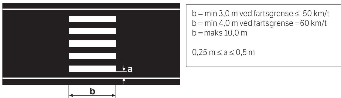
Figur 8.1 Utforming av gangfelt
