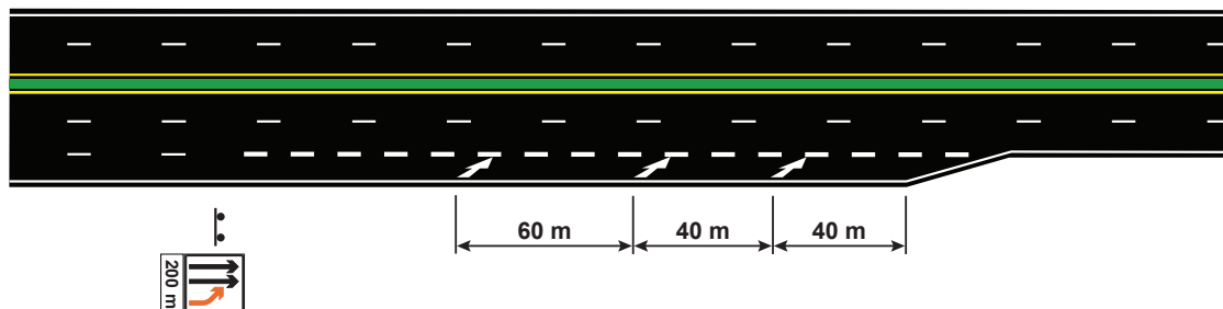
Figur 5.7 Oppmerking av kjørefeltavslutning utenfor vegkryss
