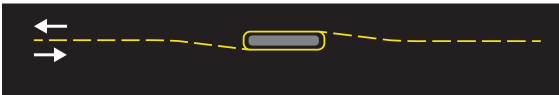
Figur 5.8 Oppmerking foran hindringer i vegbanen i gater med 2 felt og lavt fartsnivå ( \leq 50 km/t)
