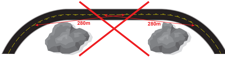
Figur 4.5 Korte kjørefeltlinjer skal ikke benyttes
