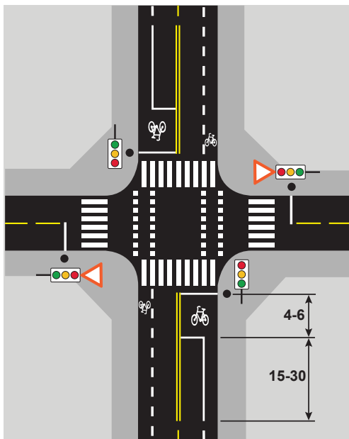
Figur 8.13 Sykkelboks i signalregulert kryss – forkjørsveg
