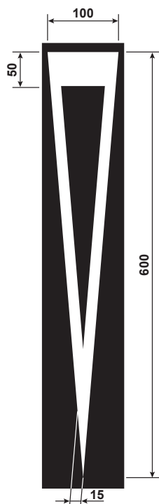
Figur 3.8 Utforming av vikesymbol
