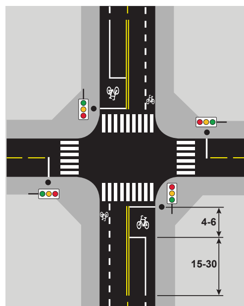
Figur 8.14 Sykkelboks i signalregulert kryss – ikke forkjørsveg
