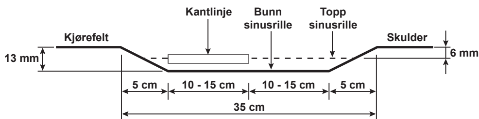
Figur 6.6 Utforming av fresespor med 0,35 m bredde
