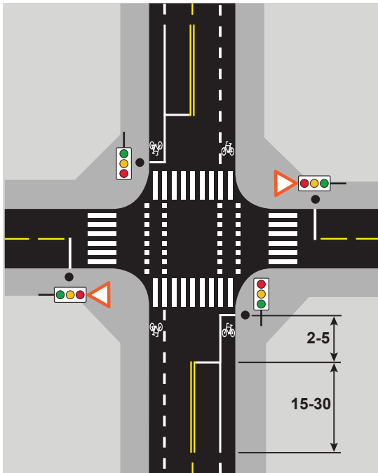
Figur 8.15 Signalregulert kryss på forkjørsvog med tilbaketrunket stopplinje uten sykkelboks
