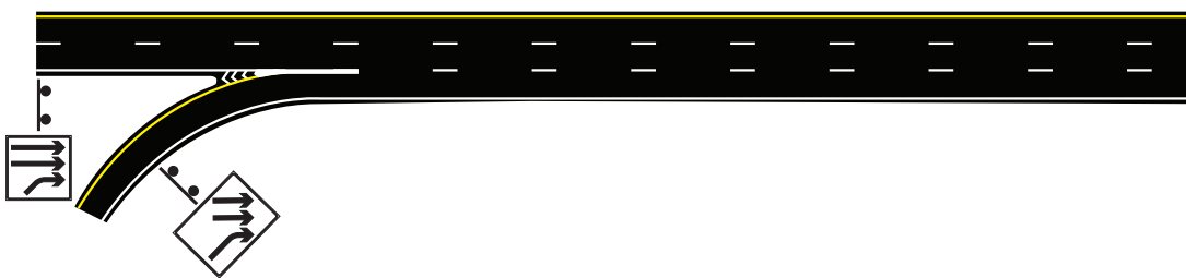
Figur 7.14 Oppmerking av feltaddisjon
