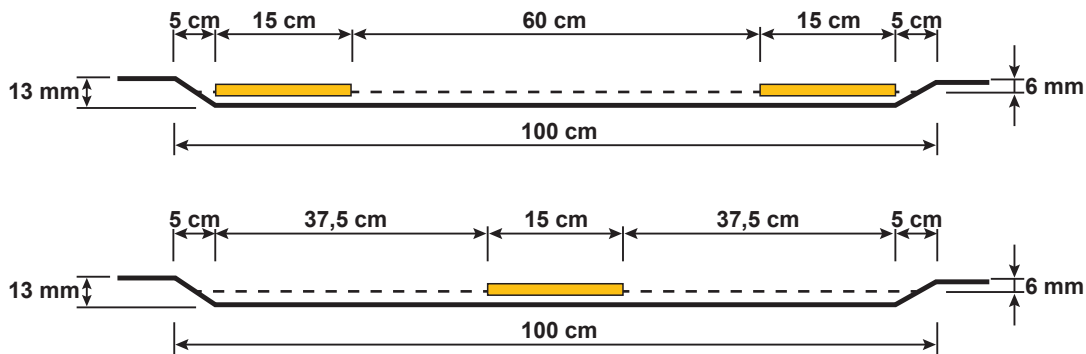
Figur 6.4 Utforming av fresespor med 1 m bredde med henholdsvis dobbel sperrelinje og varsel-linje/kjørefeltlinje
