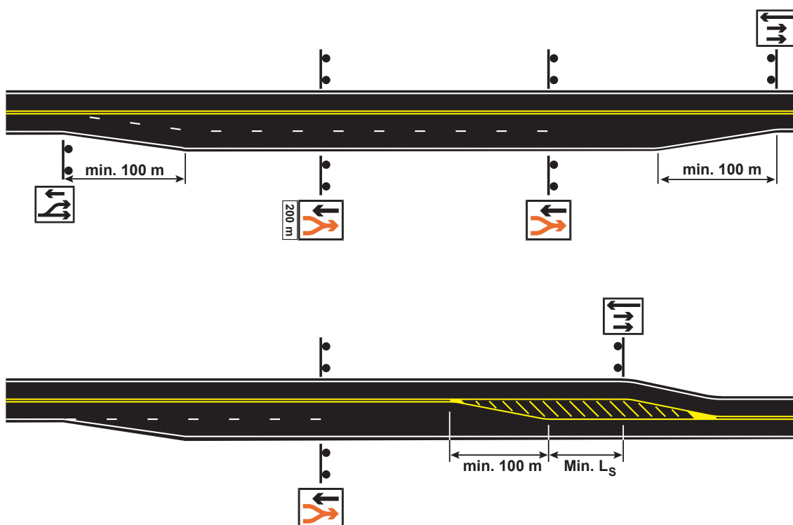
Figur 5.3 Krav til oppmerking av forbikjøringsfelt
