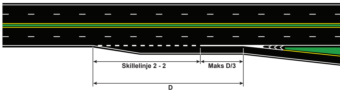
Figur 7.9 Oppmerking av retardasjonsfelt
