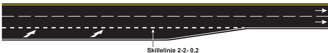
Figur 9.6 Avslutning av kollektivfelt på vegstrekning
