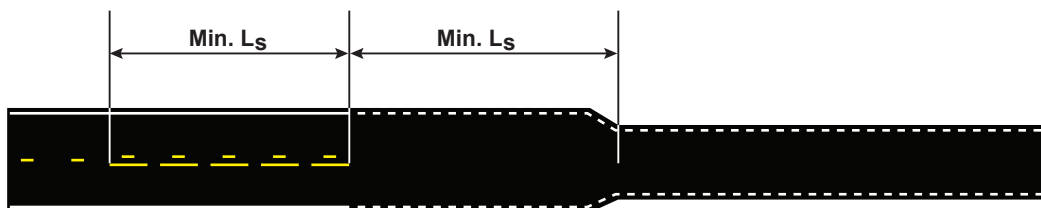
Figur 5.2 Overgang mellom 2-feltsveg og 1-feltsveg
