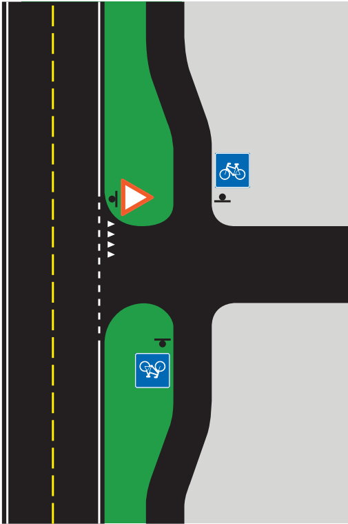
Figur 8.20 Oppmerking når kjørende på sekundærveg ikke har vikeplikt for syklende (trafikkreglene § 7 nr. 4 annet ledd)
