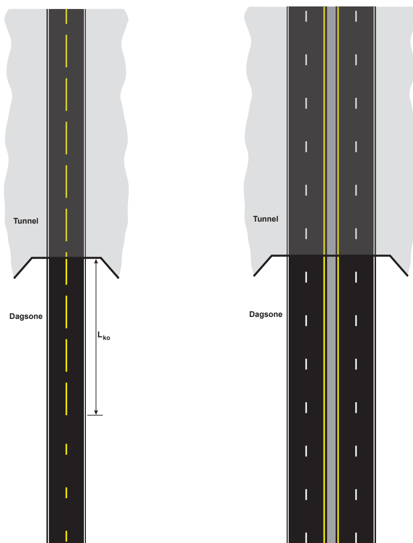
Figur 5.10 Oppmerking i 1- og 2-løps tunnel
