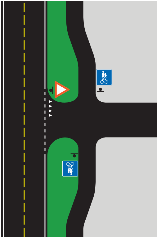
Figur 8.17 Oppmerking når kjørende på sekundærveg ikke har vikeplikt for gående og syklende (trafikkreglene § 7.2)
