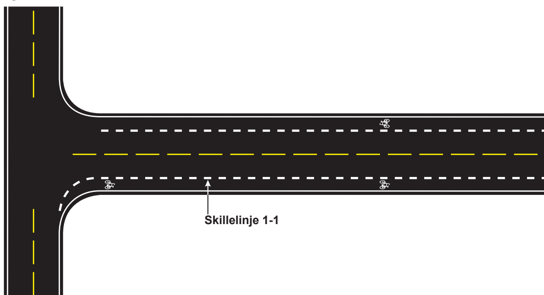
Figur 8.8 Oppmerking av sykkelfelt
