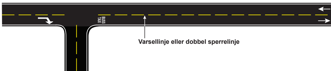
Figur 9.5 Oppmerking av veg/gate der den ene kjøreretningen er reservert for kollektivtrafikk
