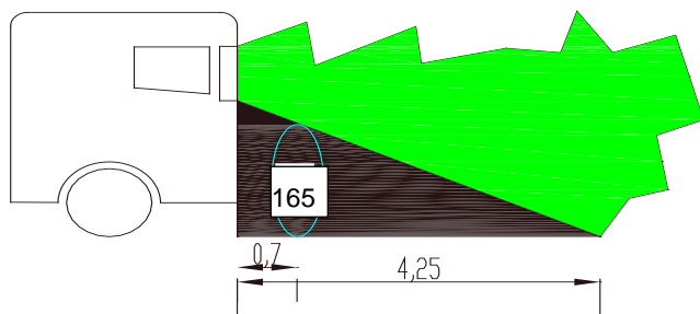
Figur 2-68 Blindsone foran lastebil. Se mørk sone på skissen over.
