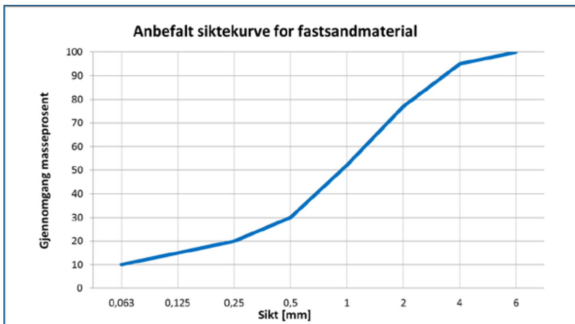
Figur 7-3 Anbefalt siktekurve for fastsandmaterialer.
