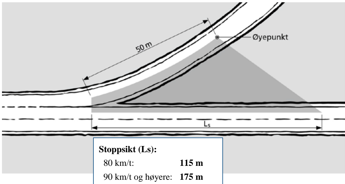
Figur 2-58 Påkjøringsramper. Areal med krav til sikt kryss (hentet fra Håndbok 111 og D2-S06 i kontrakt)
