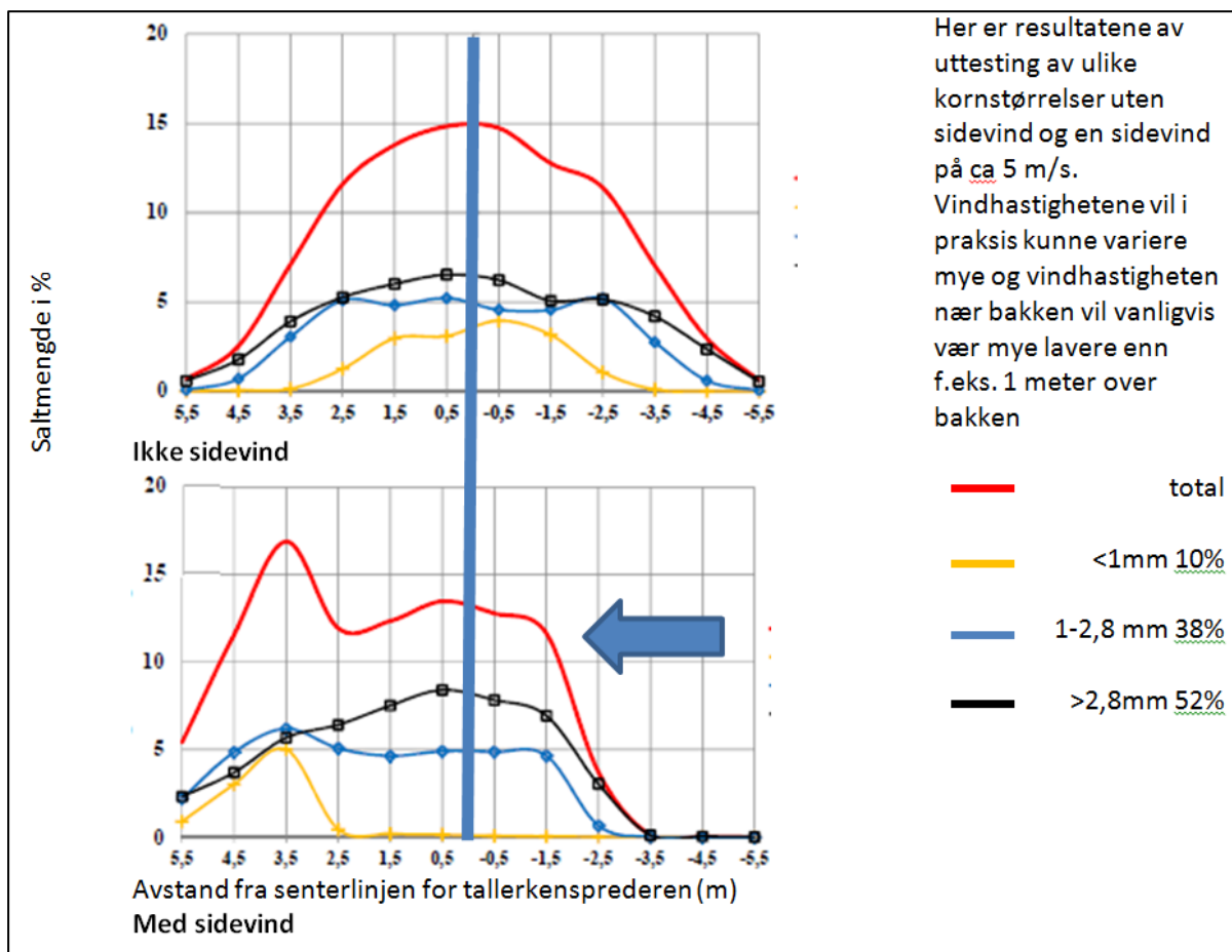
Figur 6-29 Kasteavstand/spredemønster påvirket av sidevind
