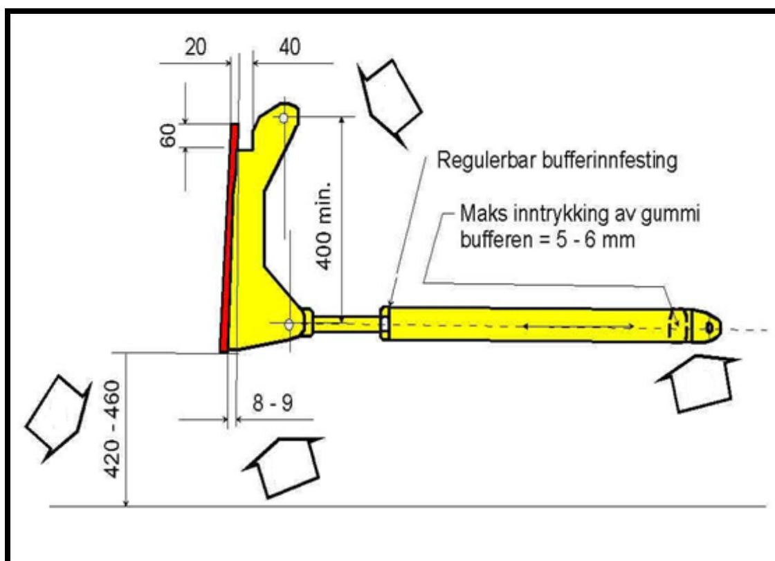
Figur 4-11 «Vegvesenstandard» brøyteplate.
