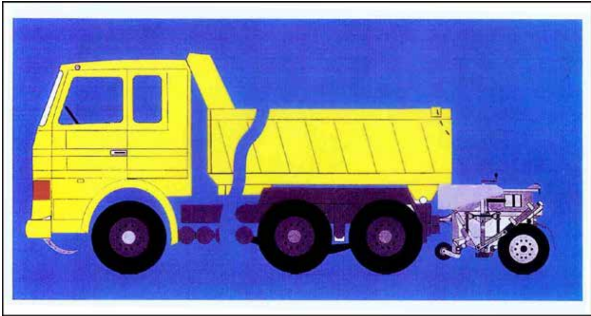
Figur 6-6: Etterhengende strøapparat.
