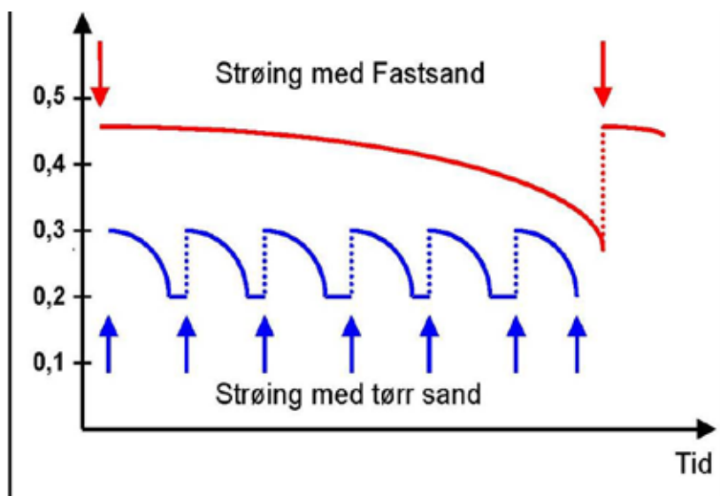
Figur 7-8 Friksjonstilskudd og varighet av sandtiltak med fastsand og tørr sand.
