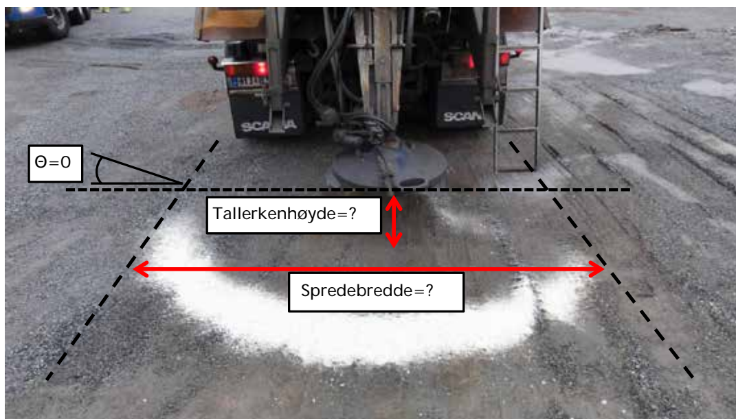
Figur 6-18 Kontroll av spredde: Tallerkenposisjon, spreddebilde (bredde og symmetri) (Foto: Dagfin Gryteselv)
