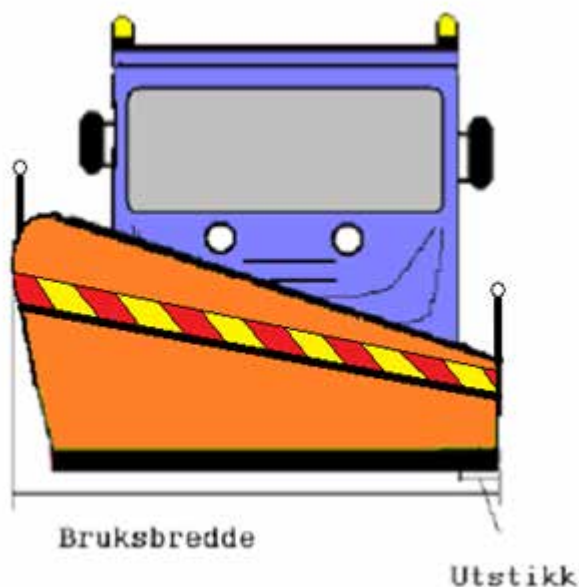
Figur 4-7 Merking av plog. Bruksbredde, utstikk og lys.
