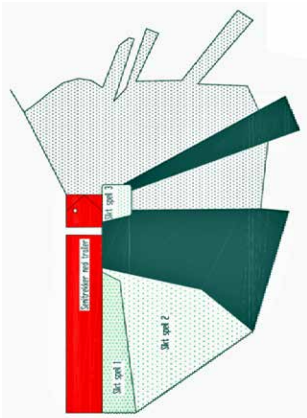
Figur 2-65 Blindsoner fra lastebilhytte. Bilen er tegnet i rødt. I mørke soner er det null sikt. Grå soner er delvis blindsoner. Se illustrasjonene nedenfor.
