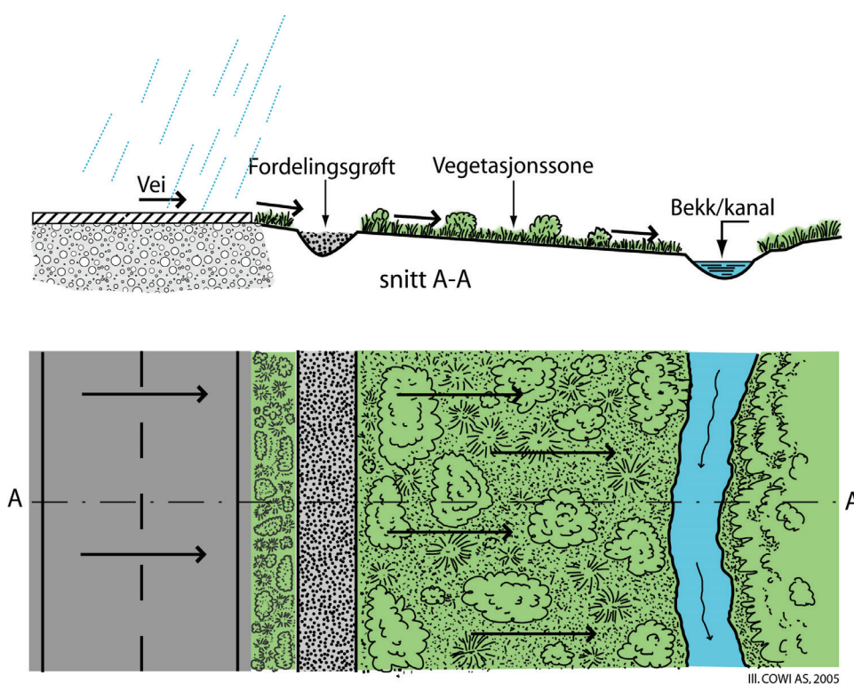
Figur 6.16. Prinsippkisse av et vegetasjonsdekket areal med lite fall for rensing av overvann (etter FHWA, 1996/ Statsbygg, 2004). (Illustrasjon: COWI AS).
