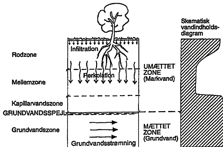
Figur 5.2. Vannbevegelse i jord (etter Mikkelsen og Jacobsen, 1993).
