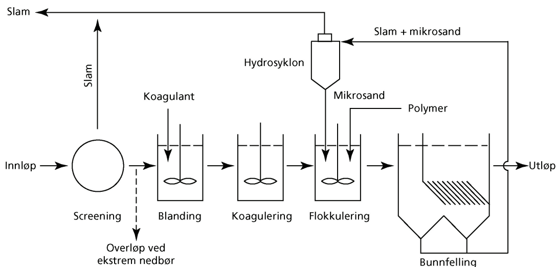
Figur 6.21 Prinsipp for funksjonen ved ballastet flokkulering.
