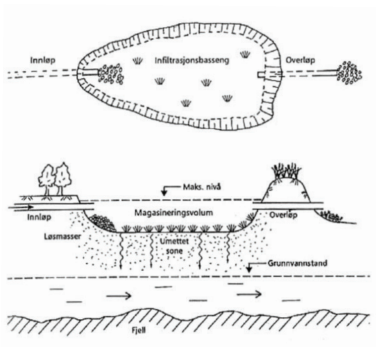
Figur 6.9. Prinsippskisse av et infiltrasjonsbasseng (plan/snitt).
