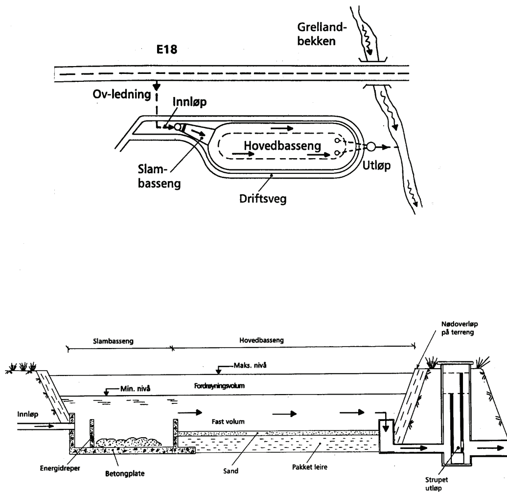
Figur 6.5. Prinsippkisse av vått overvannsbasseng (plan/snitt) bygd i forbindelse med E18 i Vestfold og E6 i Oslo/Akershus.
