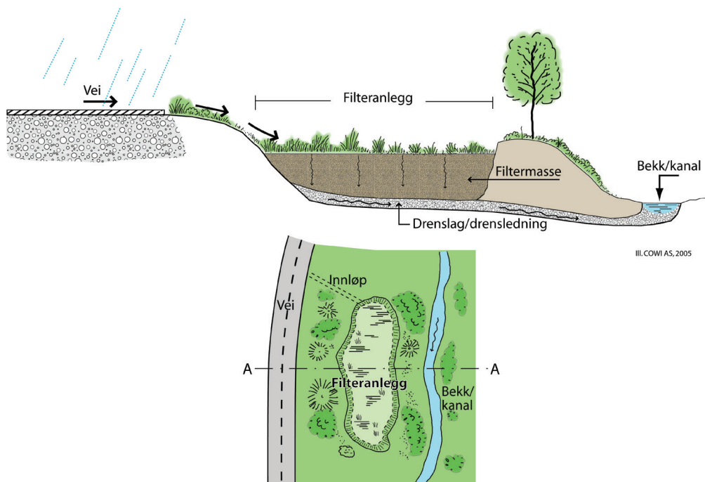
Figur 6.17. Utsnitt av et åpent sandfilter.
