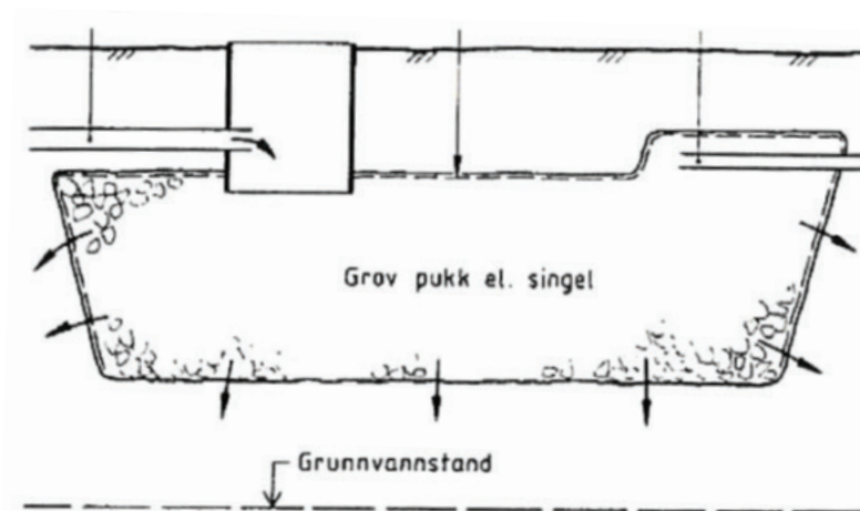
Figur 6.13 Prinsippskisse av perkolasjonsmagasin med infiltrasjonskum og overløp (Byggforsk, 1989).
