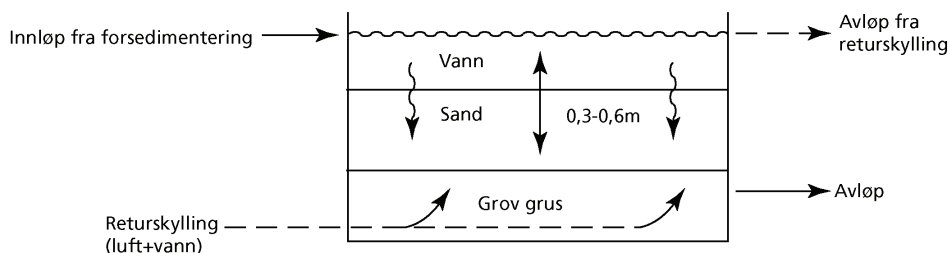
Figur 6.20 Prinsipp for nedstrøms sandfilter med returskylling.
