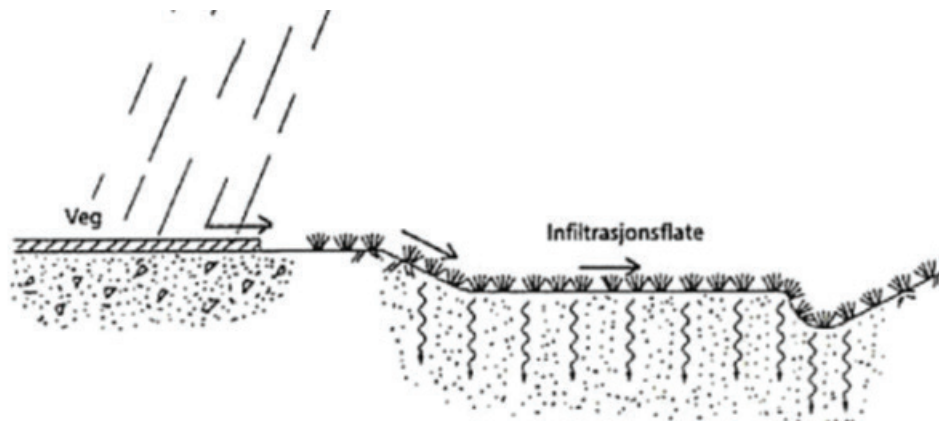
Figur 6.12. Prinsippskisse av enkel infiltrasjon på grasdekt areal.
