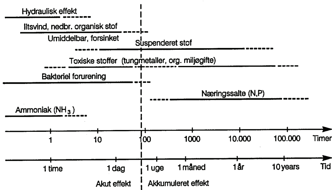
Figur 4.2. Tidsskala for resipienteffekter i forbindelse med utslipp av overvann (Hvitved- Jacobsen et al., 1994)
