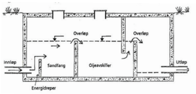
Figur 6.22. Prinsippkisse av et lukket slambasseng med oljeavskilling.
