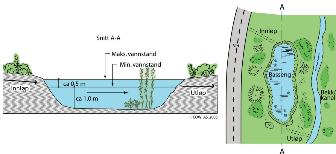
Figur 6.2. Prinsippsskisse av et vått overvannsbasseng med horisontal gjennomstrømming (snitt/plan) (Illustrasjon: COWI AS).
