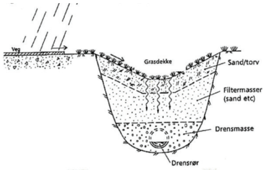
Figur 6.18. Skisse av en sandfiltergrøft.
