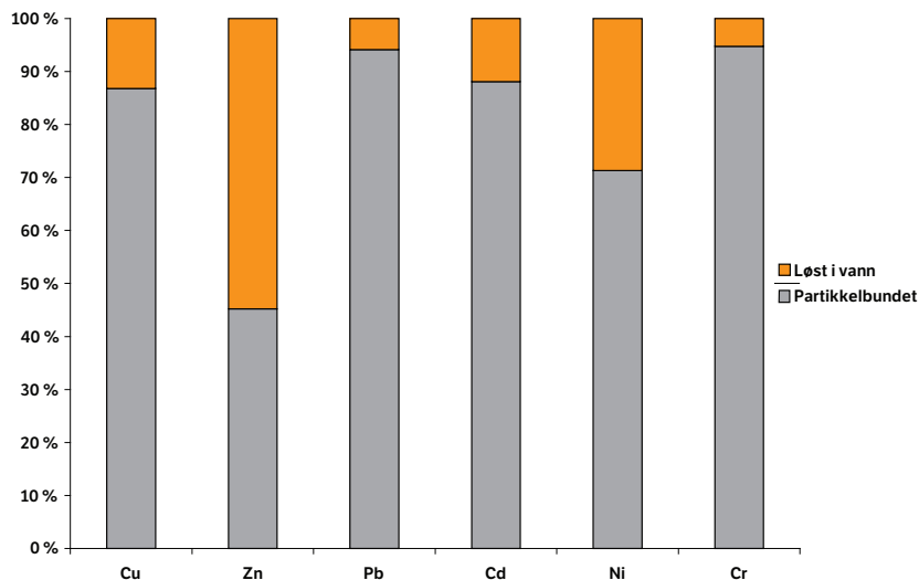
Figur 4.3. Forholdet mellom løste og partikkelbundne metaller i avrenning fra tunnelvask i Nordbytunnelen mai 2000.
