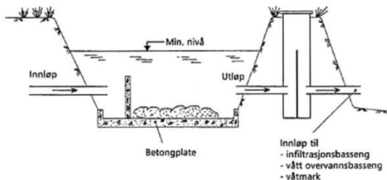
Figur 6.23. Prinsippskisse av et åpent slambasseng med oljeavskilling (dykket utløp).
