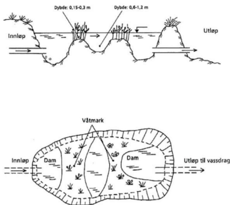
Figur 6.14. Prinsippskisse av kunstig anlagt våtmark (plan/snitt).
