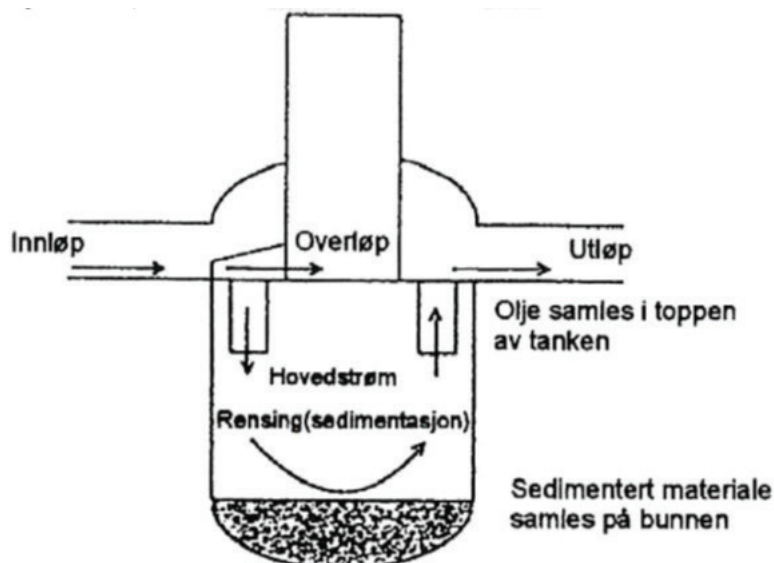
Figur 6.24. Prinsippskisse av en sedimentasjonstank, type "Stormceptor" (Stormwater Corporation, Inc., 1995).
