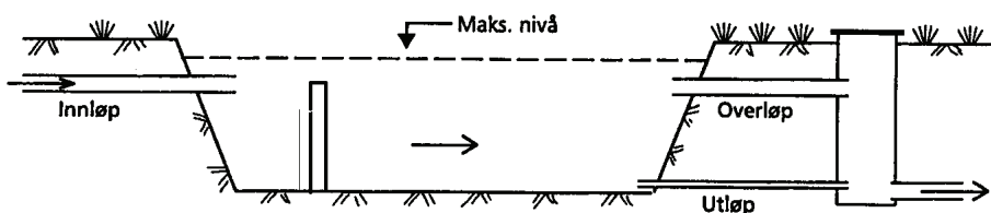
Figur 6.1. Prinsippkisse av et overvannsbasseng.
