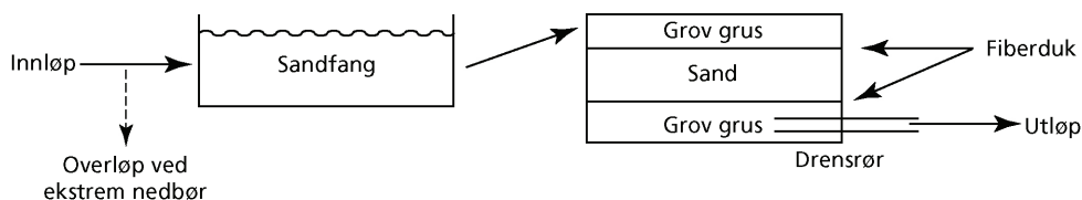
Figur 6.19. Skisse av et lukket sandfilter (plan/snitt).
