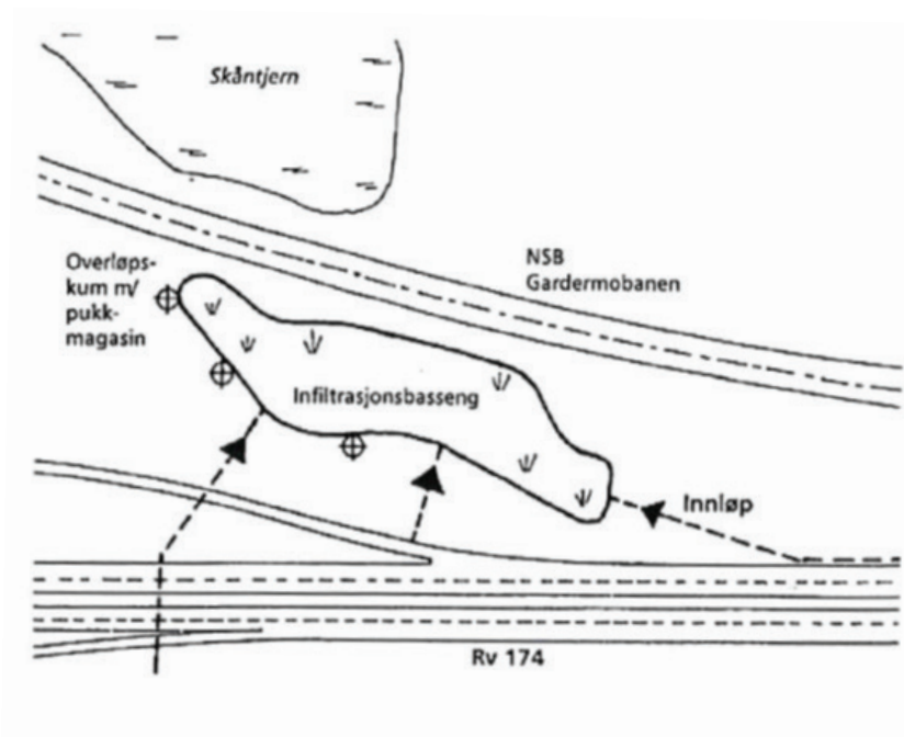
Figur 6.10. Skisse (plan/snitt) av infiltrasjonsbasseng bygd langs rv. 174 i Akershus (Illustrasjon: COWI AS).
