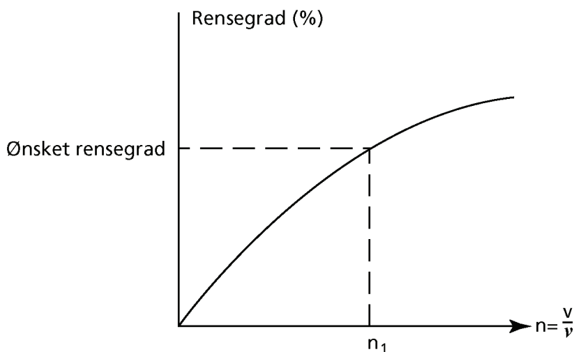
Figur 6.4. Rensegrader for suspendert stoff (TSS) og totalt fosfor (TP) i våte overvannsbasseng i Danmark og USA som funksjon av forholdet mellom bassengvolum og avrenningsvolum ved et middelregn ( n = V/v ), (USEPA, 1986; Hvitved-Jacobsen et al., 1987; Hvitved-Jacobsen et al., 1994).
