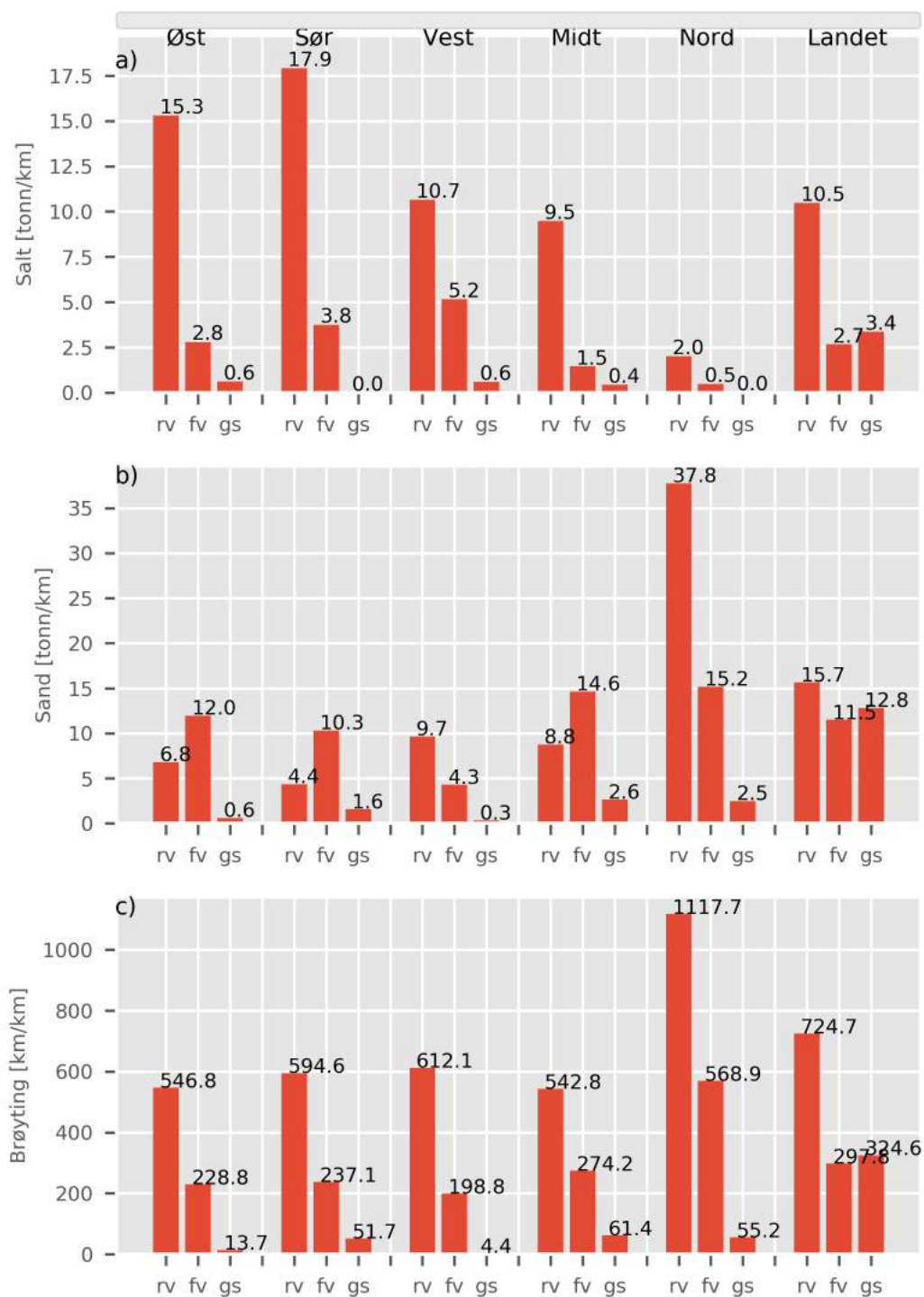
Figur 4. Vintermengder sesongen 2018/2019 fordelt på vegkategori.
