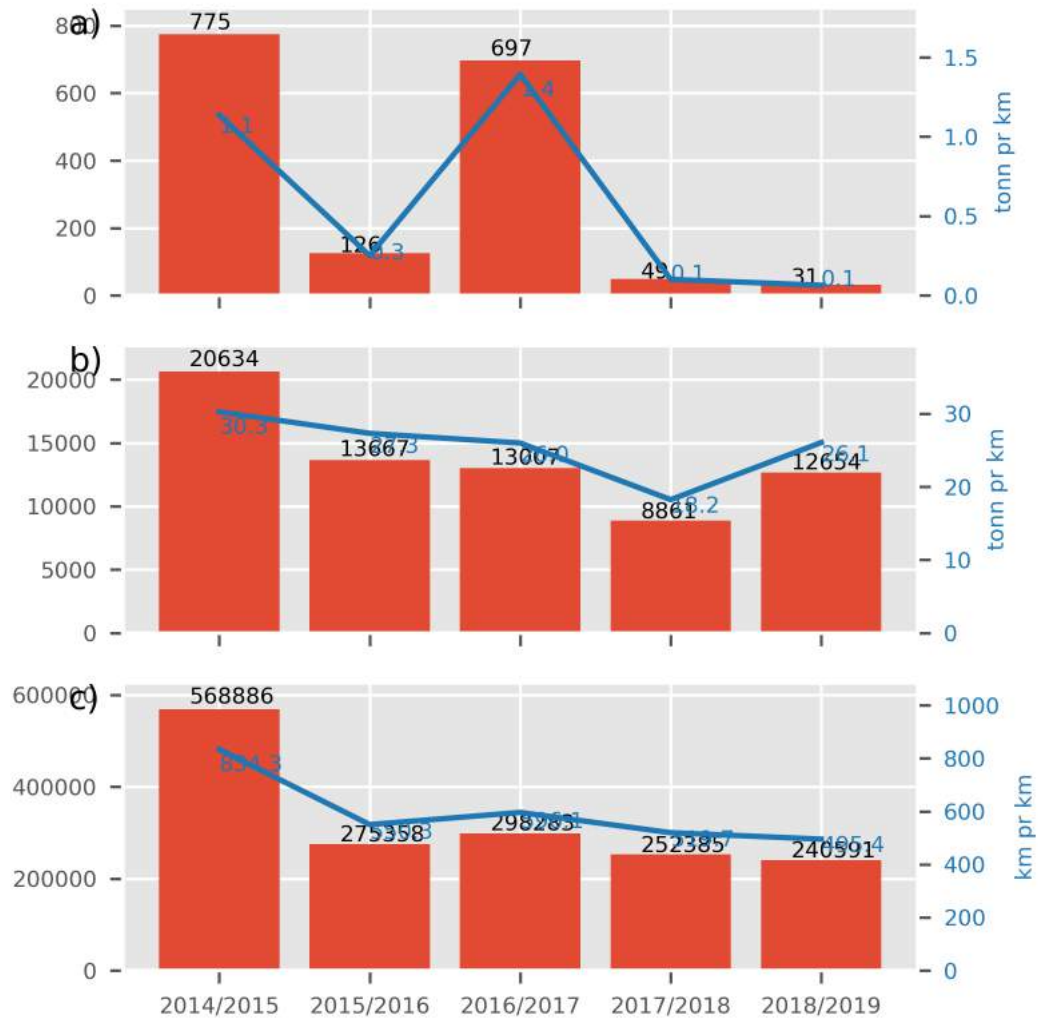
Figur 95. Mengder totalt og per km fra sesongen 2014/2015 til 2018/2019. a) Saltmengder b) Sandmengder c) Kilometer brøyting
