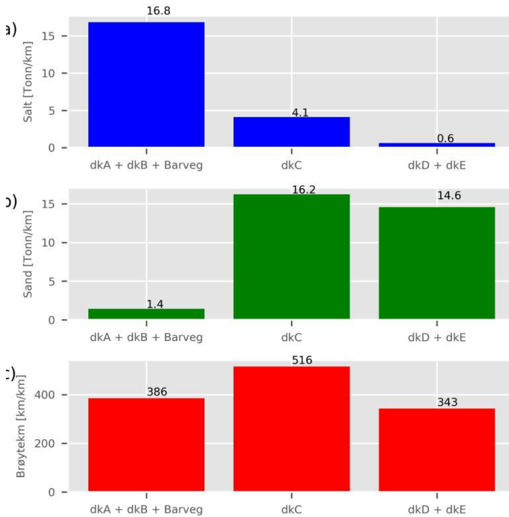
Figur 6. Fordeling av mengder på ulike driftsklasser for sesongen 2018/2019. a) Saltmengder per km veg, b) Sandmengder per km veg, c) Brøytekm per km veg
