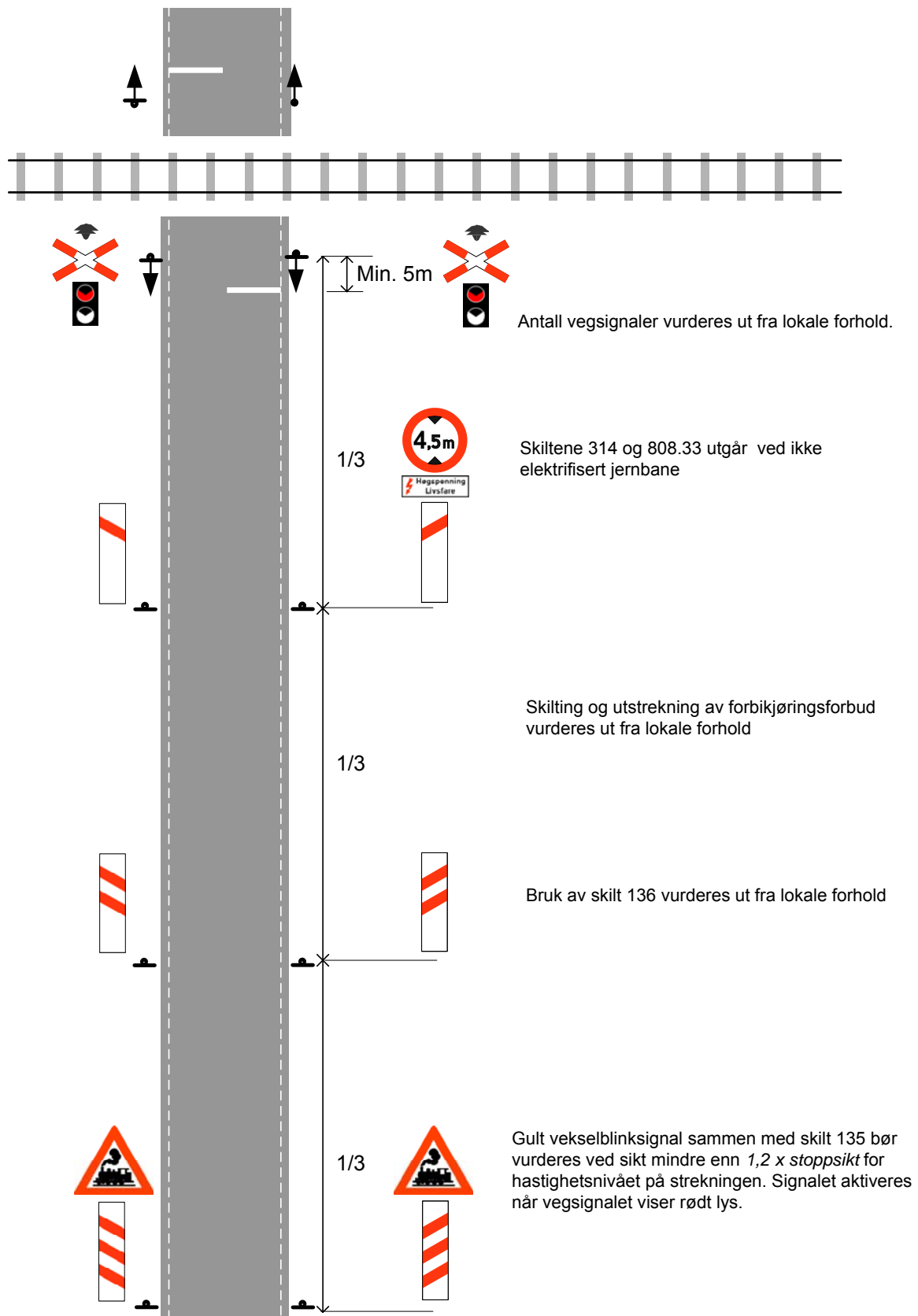
Figur 1.7 Sikringsnivå 1b: Planovergang med vegsikringsanlegg
