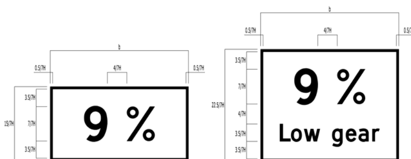
Figur 4.15 Utforming av underskilt 813
