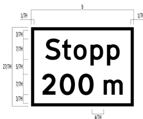
Figur 4.20 Utforming av underskilt 824
