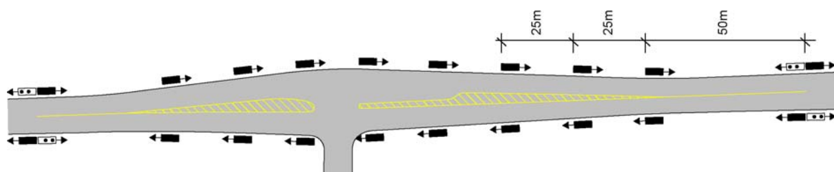
Figur 2.22. Plassering av kantstolper i kanalisert vegkryss
