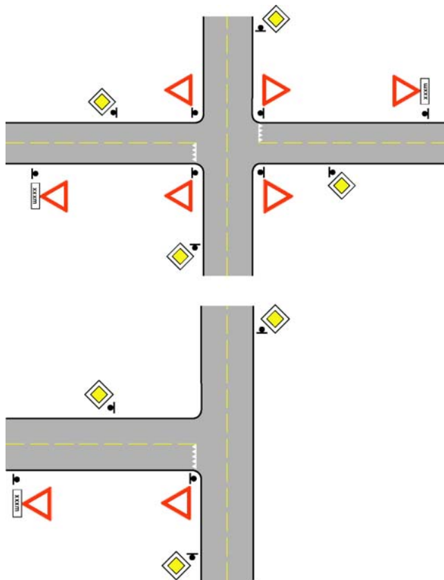
Figur 3.5 Brudd på forkjøringsveg i kryss - eksempel på anvendelse av skilt 202/802 og 206 i X-kryss og T-kryss
