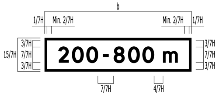
Figur 4.6 Plassering av tekst på underskilt 804
