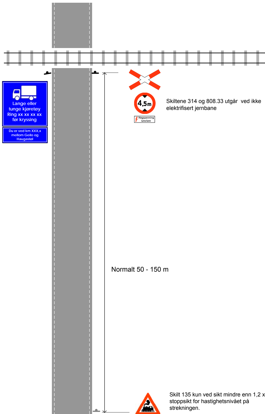
Figur 1.9 Sikringsnivå 2: Planovergang uten vegsikringsanlegg på privat veg med offentlige trafikkskilt
