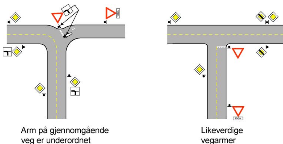
Figur 3.2 Skilting av forkjørsvog i vegkryss med 90 graders vinkelendring
