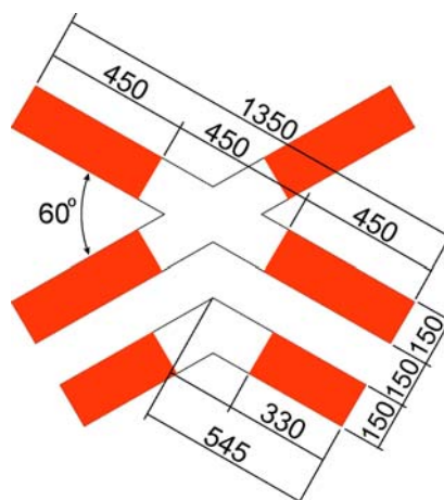
Figur 1.12 Størrelse og utforming av skilt 138. Mål i mm
