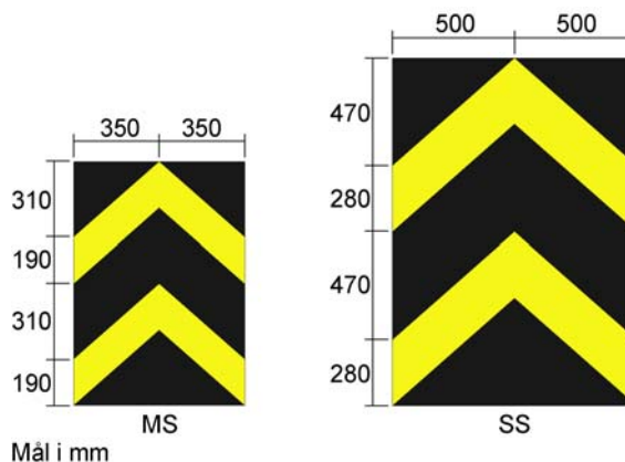
Figur 2.15 Størrelse og utforming av skilt 912
