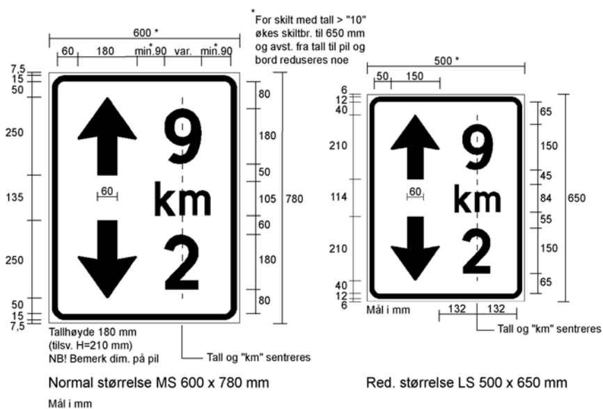
Figur 2.19 Størrelse og utforming av skilt 916
