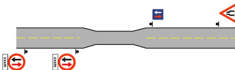
Figur 3.7 Eksempel på anvendelse av skilt 106, 212 og 214 ved veginnsnevring
