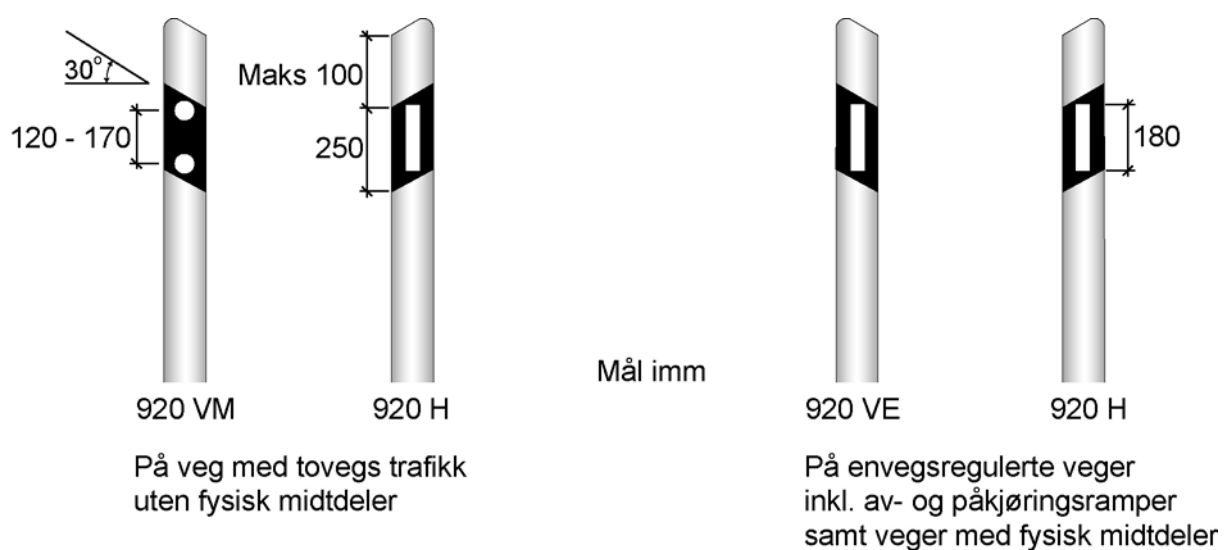
Figur 2.25. Detalj av kantstolper med refleks
