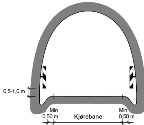
Figur 2.16 Plassering av skilt 914 i forhold til kjørebane.
