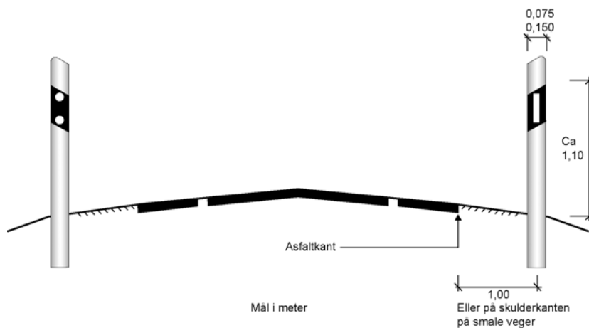
Figur 2.20. Normal plassering av kantstolper på tofelts veg med trafikk i begge retninger
