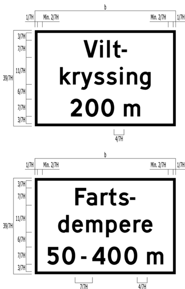
Figur 4.10 Eksempler på utforming av kombinerte underskilt 808/802 og 808/804
