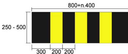
Figur 2.13 Størrelse og utforming av skilt 908
