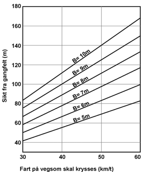
Figur 1.13 Siktkrav i gangfelt uten forvarsling
