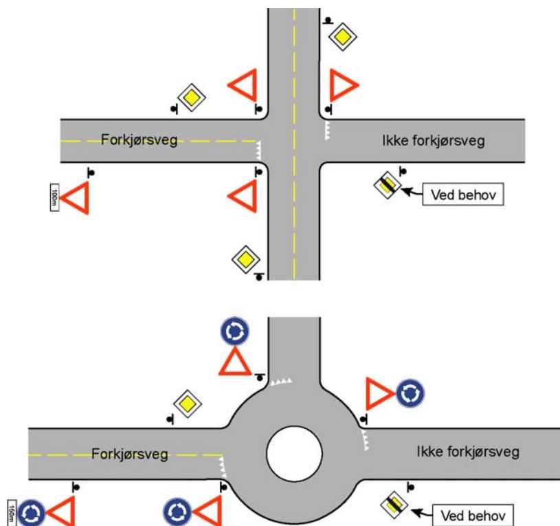
Figur 3.6 Slutt på forkjørsvveg i kryss - eksempel på anvendelse av skilt 202/802 og 208
