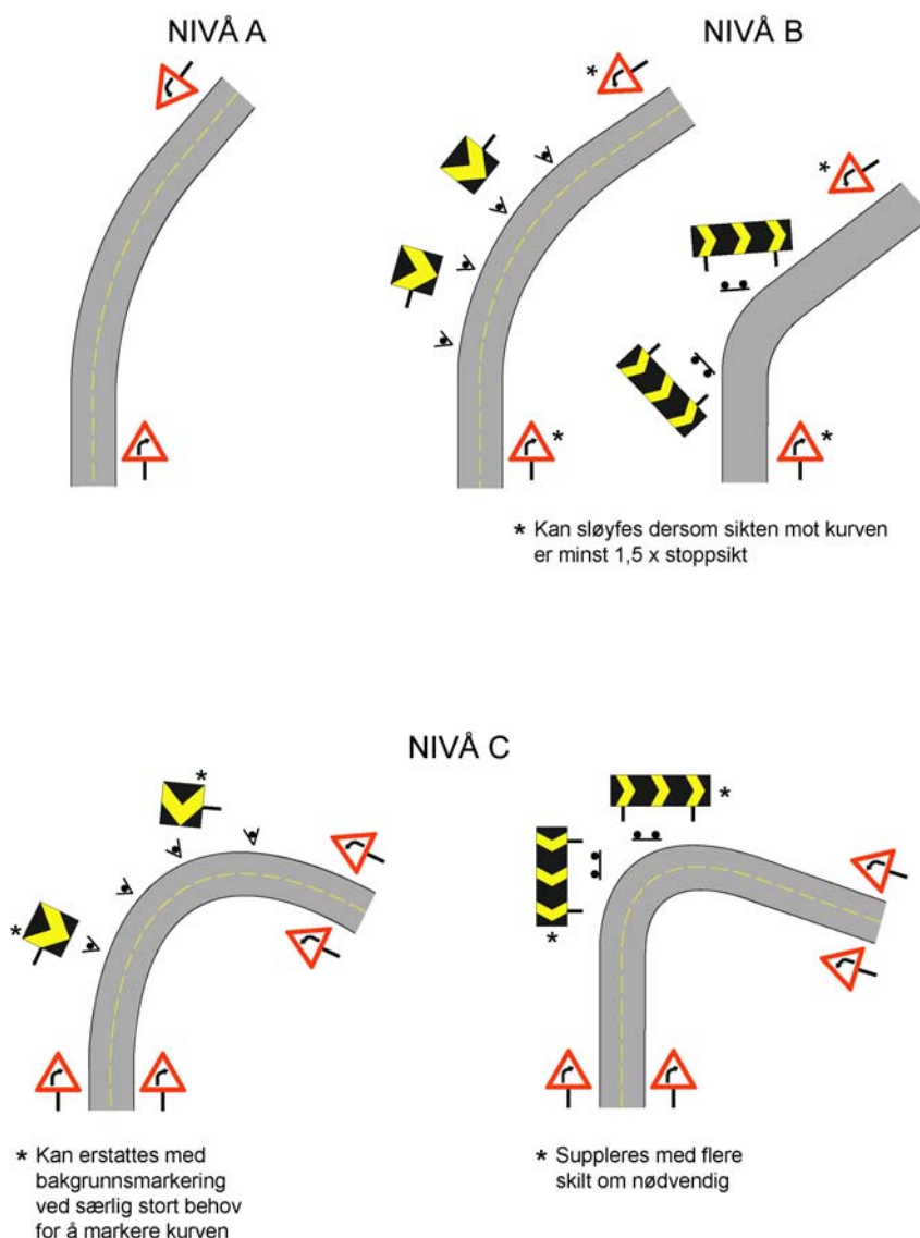
Figur 2.2 Eksempler på ulike nivåer for skilting av farlige kurver ut fra kurvenes skarphet og overraskelsesgrad
