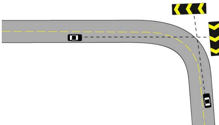
Figur 2.3 Eksempel på skilting med bakgrunnsmarkering i kurve med liten radius og stor vinkelendring
