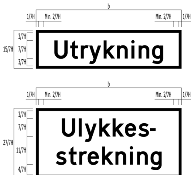
Figur 4.9 Plassering av tekst på underskilt 808
