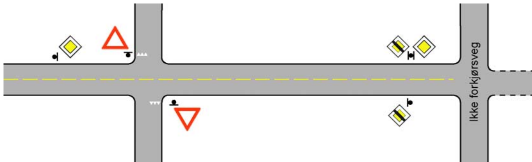
Figur 3.3. Avslutning av forkjørsvog foran kryss med veg som ikke er forkjørsvog - eksempel på anvendelse av skilt 208
