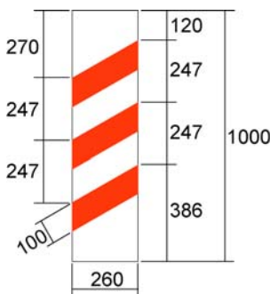
Figur 1.11 Størrelse og utforming av skilt 136. Mål i mm
