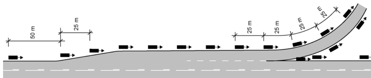
Figur 2.23. Plassering av kantstolper på rampe
