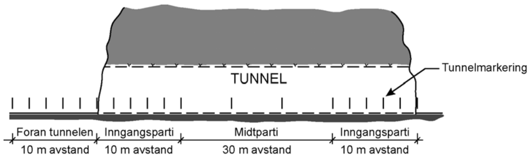
Figur 2.17 Avstand mellom tunnelmarkeringer.
