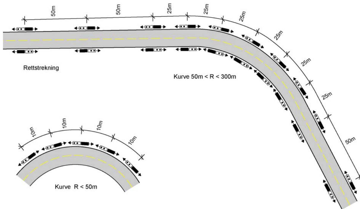
Figur 2.21. Plassering av kantstolper på tofelts veg, rettstrekning og i kurver
