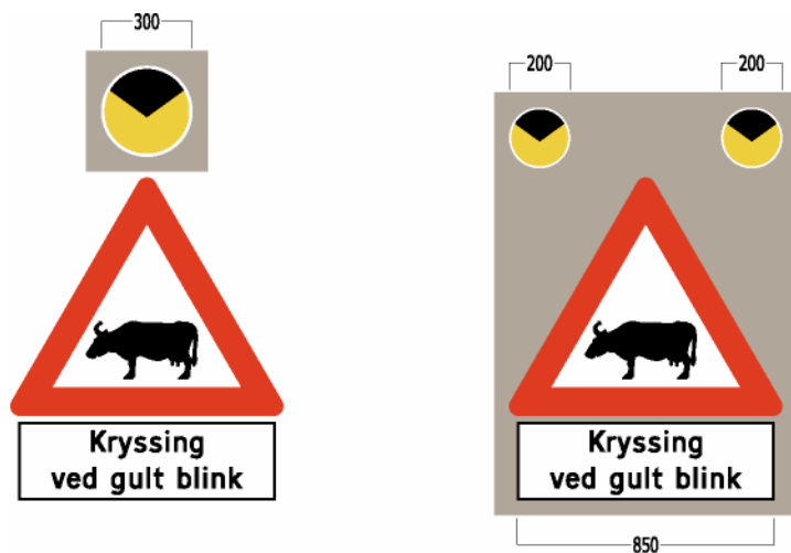
Figur 1.14 Skilt 146.4 "Ku" med gult blinksignal
