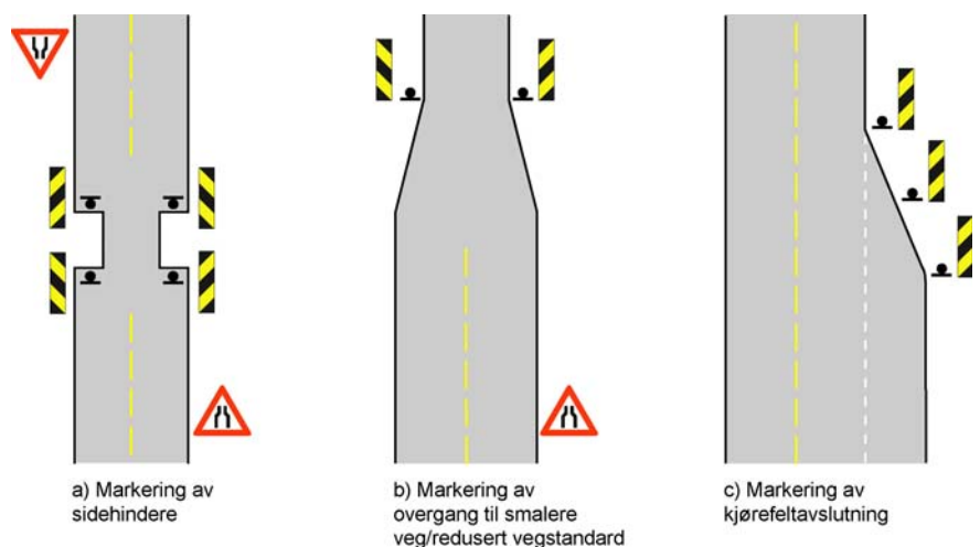
Figur 2.11. Eksempler på markering av sidehindre, veginnsnevring og kjørefeltavslutninger
