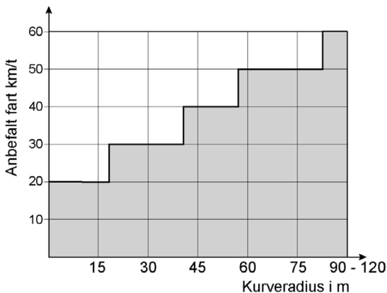
Figur 4.12 Anbefalt fart for ulike kurveradier
