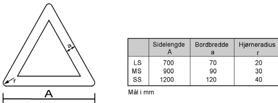
Figur 1.1 Fareskilt – størrelse og utforming
