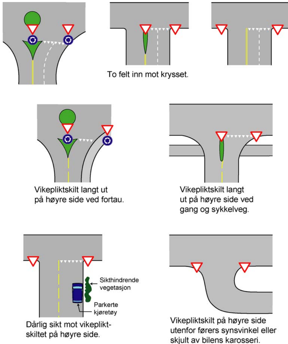
Figur 3.1. Eksempler på tosidig plassering av vikepliktskilt
