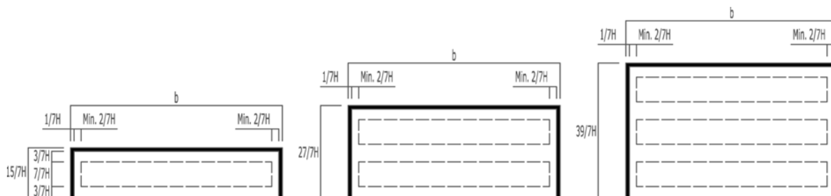
Figur 4.1 Underskilt med tekst - grunnform
