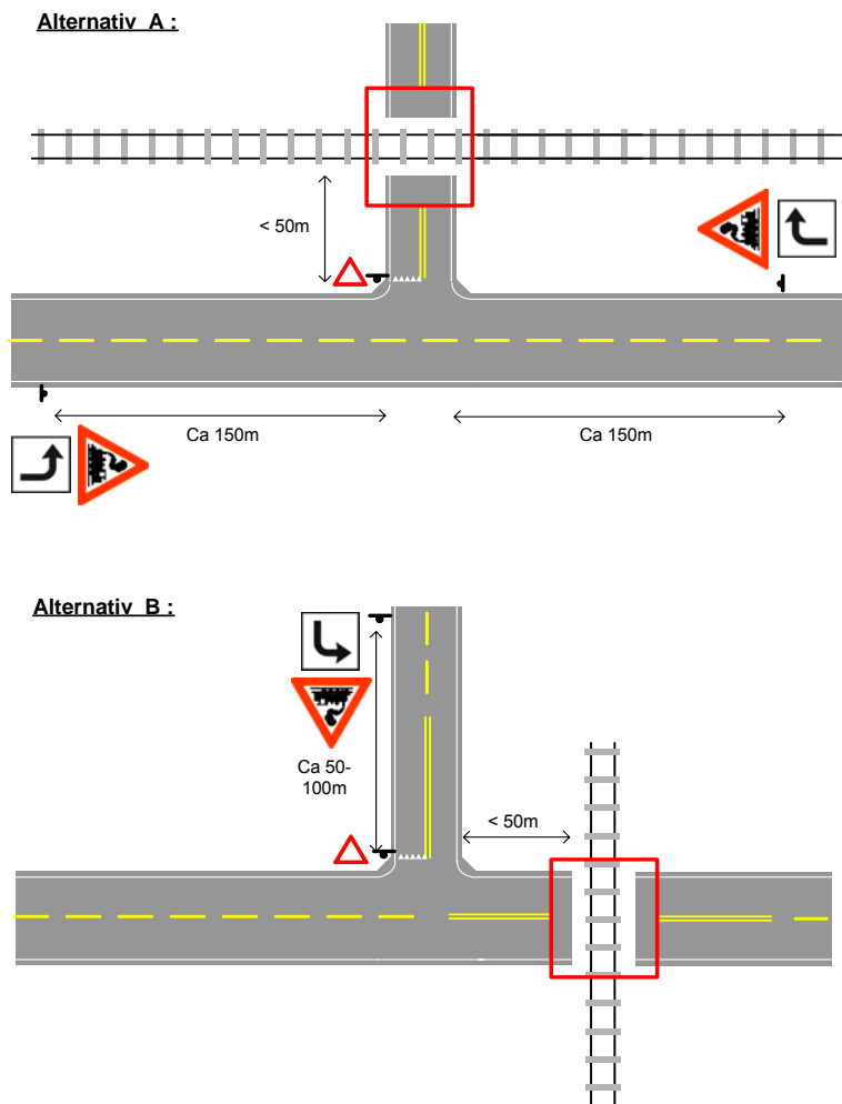
Figur 1.10 Planoverganger ved vegkryss
