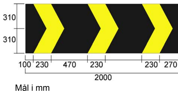
Figur 2.7 Størrelse og utforming av skilt 902
