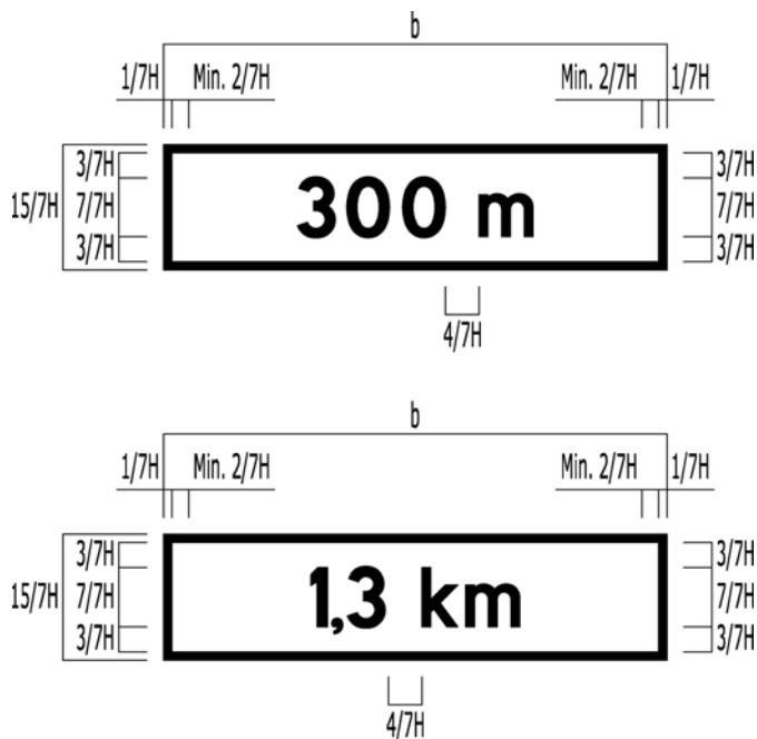
Figur 4.4 Plassering av tekst på underskilt 802
