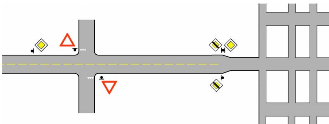
Figur 3.4. Avslutning av forkjørsvog på vegstrekning - eksempel på anvendelse av skilt 208
