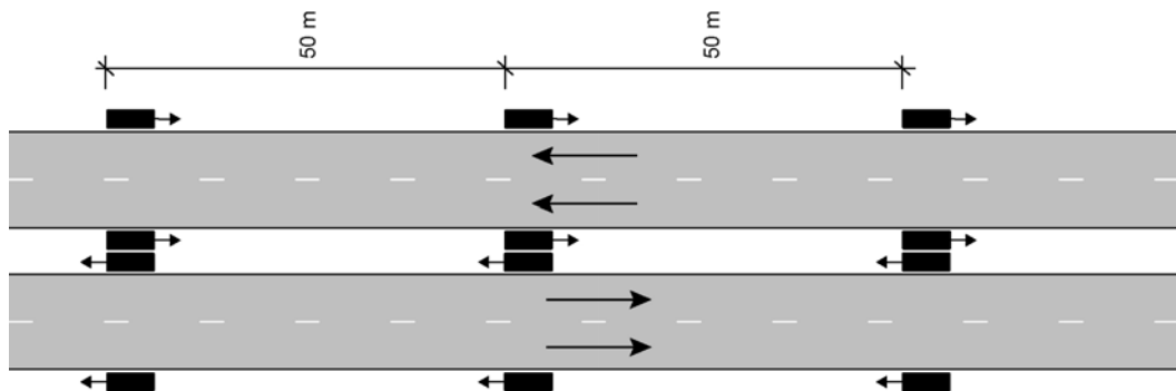
Figur 2.24. Plassering av kantstolper på veg med fysisk midtdeler
