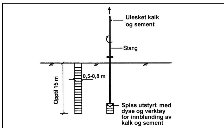
Figur 237.1 Kalk/semmentpel – prinsipptegning
