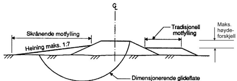
Figur 233.1 Nyttverdi av motfyllingsområde bør vurderes ved utforming
