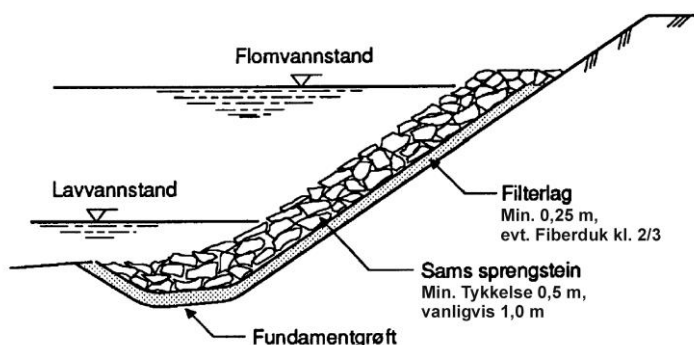
Figur 261.1 Elveforbygning av stein
