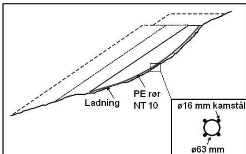
Figur 231.4 Massefortregning ved sprengning i plastslanger plassert på sjøbunn
