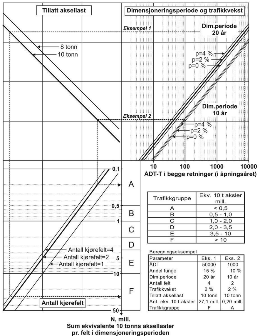
Figur 510.2 Beregning av trafikbelastning, N
