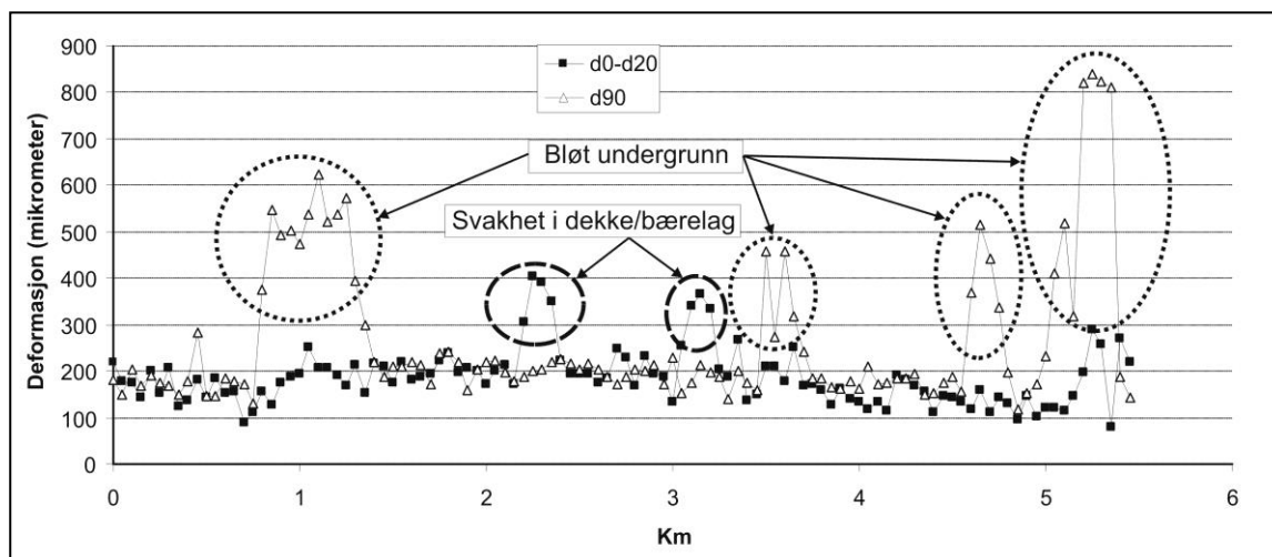
Figur V6.2 Eksempel på tolking av falloddmålinger mht. lokalisering av svake lag ( d_{90} = nedbøyning i avstand 90 cm fra lastsenetret, d_0-d_{20} = differanse mellom nedbøyning rett under lastsenetret og nedbøyning 20 cm fra lastsenetret, dvs. krumning av overflaten under lastsenetret)
