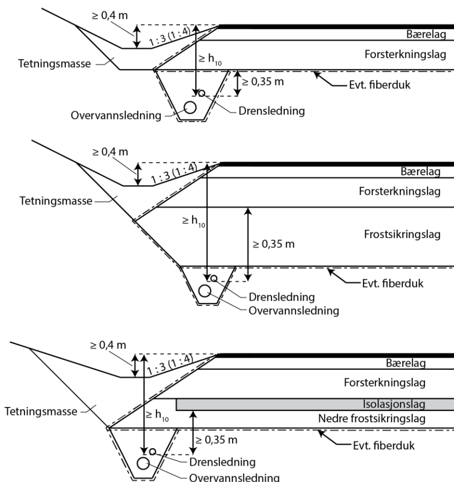
Figur 406.4 Grunne overvannsgrøfter og lukket drenering
