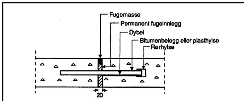
Figur 663.6 Ekspansjonsfuge, eksempel
