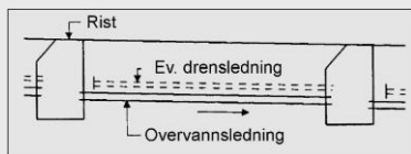
Figur 433.1 Overvannsledning og eventuell dremsledning
