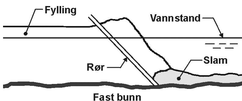
Figur 231.3 Massefortrengning med ladning i rør lagt på fyllingsfront for overfylling og sprengning
