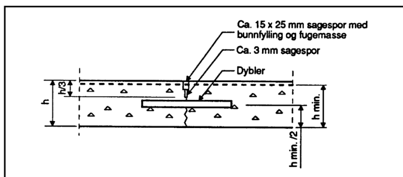
Figur 663.5 Forseglet tverrfuge, eksempel
