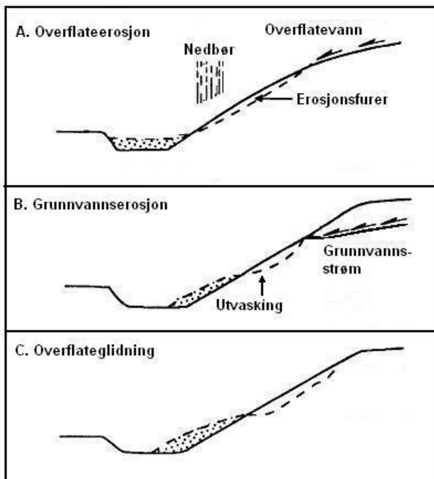
Figur 245.1 Typer av skråningsskader i jord
