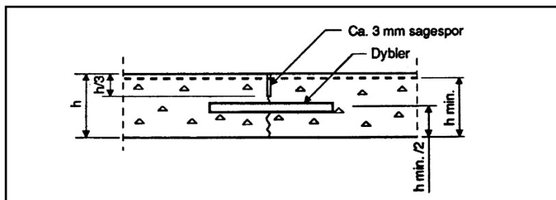
Figur 663.4 Uforseglet tverrfuge, eksempel
