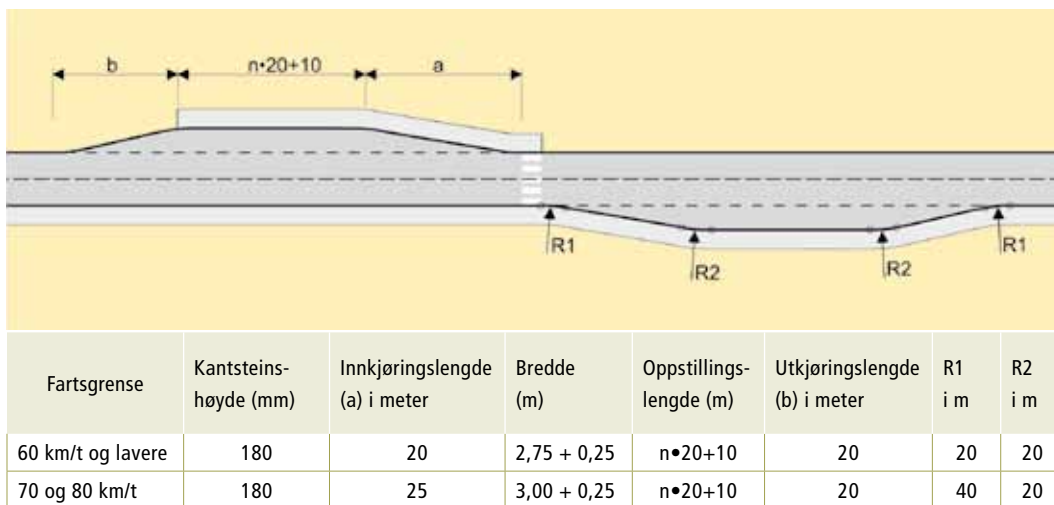
Figur 41 Plassering av busslommer i motsatte retninger på tofelts veg med karakteristiske mål. NB Gangfelt bør vurderes i de enkelte tilfelle, men kun der farten er 60 km/t eller lavere (se egne kriterier). Ved 4-felts veger og/eller fart over 80 km/t bør det etableres delende trafikkøy mellom kjørebane og busslommen, se figur 42.
