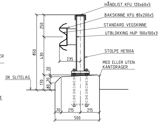
ALTERNATIV SNITT LAVT INNERREKKVERK UTEN PANELER
