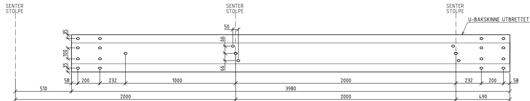
STANDARD U-BAKSKINNE UTBRETET 1:10
