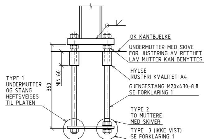
ALTERNATIV 2: FOTPLATE OG BOLTEGRUPPE - M20 INNSTØPTE HYLSE UTEN UNDERSTØP 1:5
