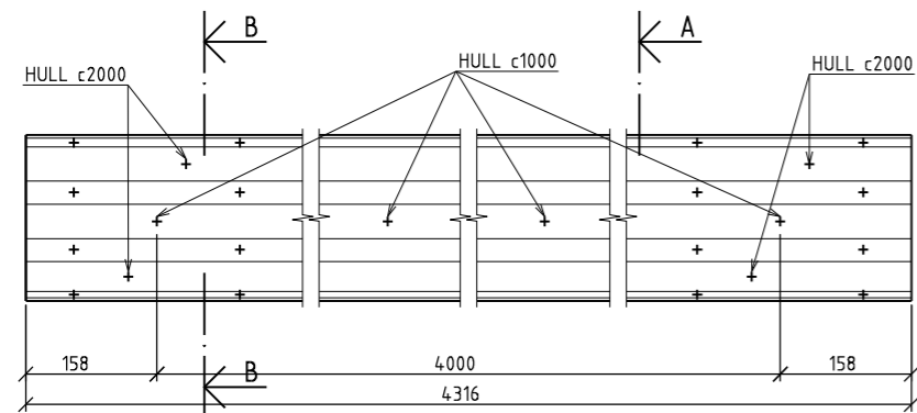
OPPRISS STANDARD BAKSKINNE 1:5
