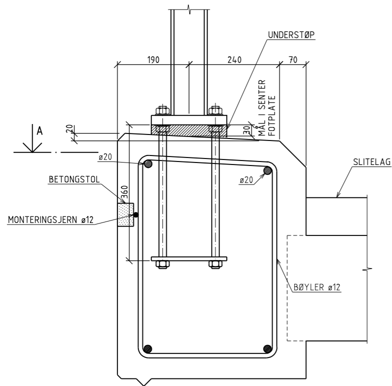
SNITT I KANTDRAGER VED FOTPLATE FOR REKKVERKSTOLPER 1:5
