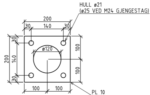
FORANKRINGSPLATE FOR BOLTEGRUPPE 1:5
