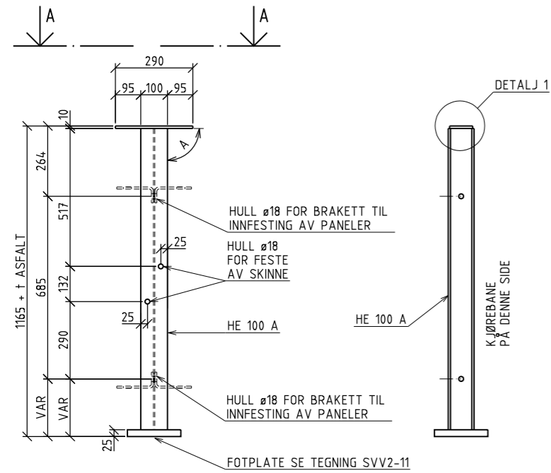
OPPRISS STOLPE FRONT 1:10
