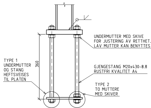
ALTERNATIV 1: FOTPLATE OG BOLTEGRUPPE - M20 MED UNDERSTØP 1:5
