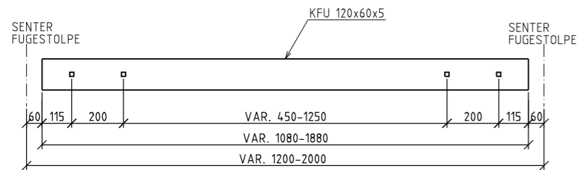
PLAN FUGEHÅNDLIST I FUGE, Plasseres mellom fugestolper 1:10
