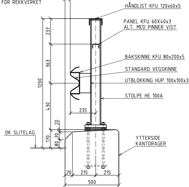
SNITT I REKKVERK STOLPE MED FOTPLATE 1:10
