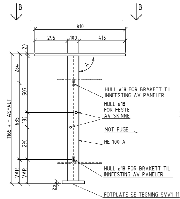
OPPRISS FUGESTOLPE FRONT, SE FORKLARINGER 1 1:10
