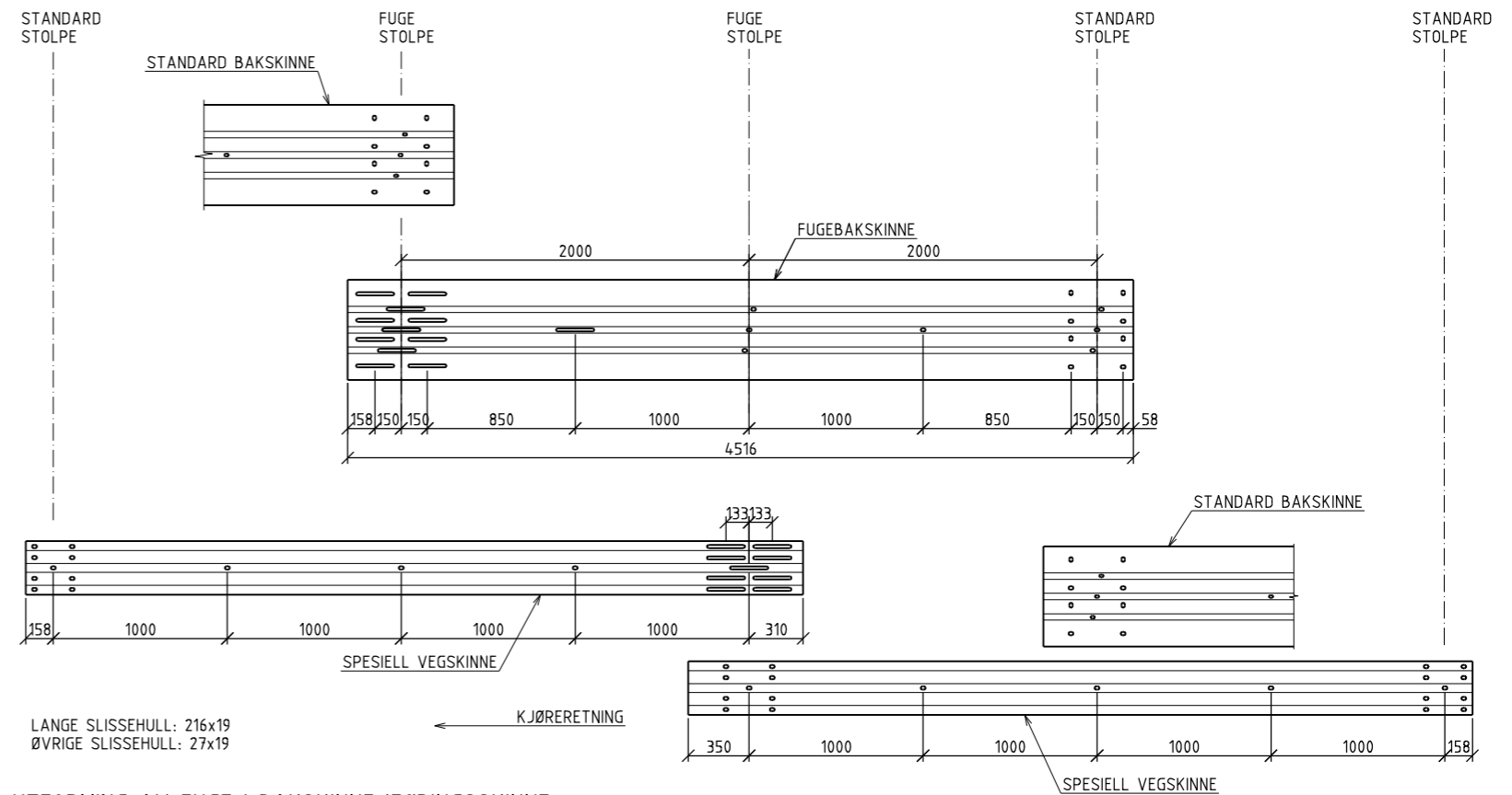
UTFORMING AV FUGE I BAKSKINNE/FØRINGSSKINNE 1:20
