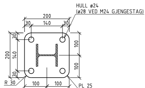
FOTPLATE OG BOLTEGRUPPE 1:5
