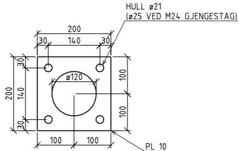
FORANKRINGSPLATE FOR BOLTEGRUPPE 1:5
