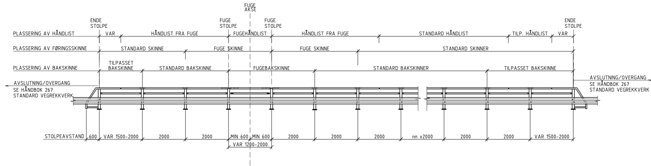
OPPRISS REKKVERK 1:50
