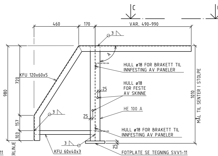
OPPRISS ENDESTOLPE 1:10
