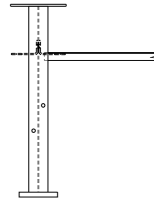
MONTASJESKISSE STOLPE MED KANTBJELKE 1:10
