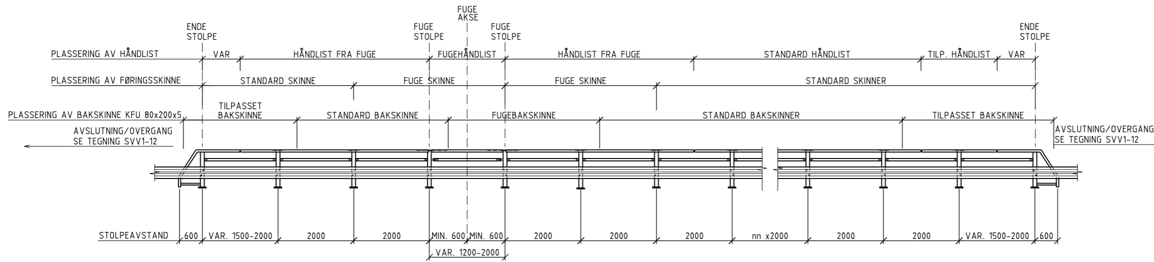
OPPRISS REKKVERK 1:50
