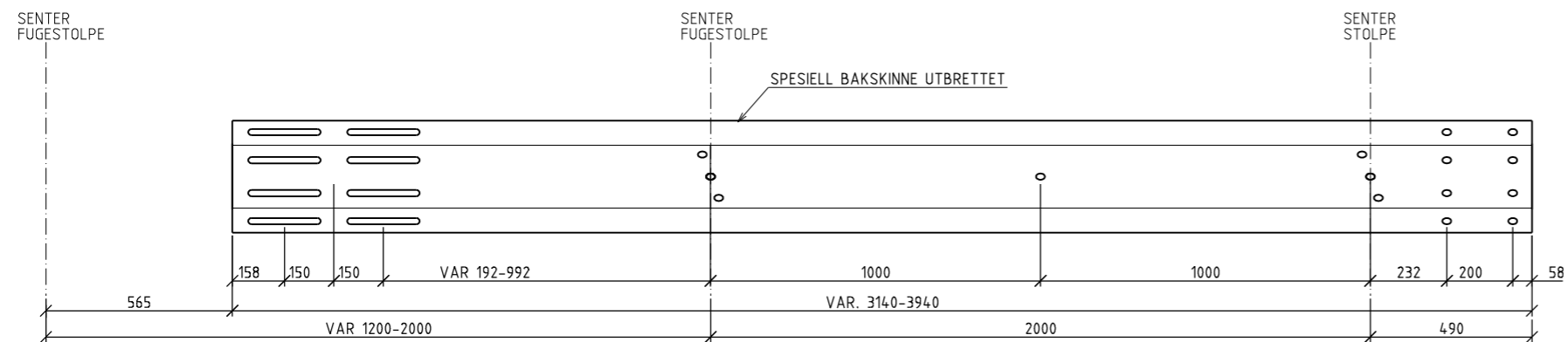
FUGEBAKSKINNE UTBRETET 1:10
