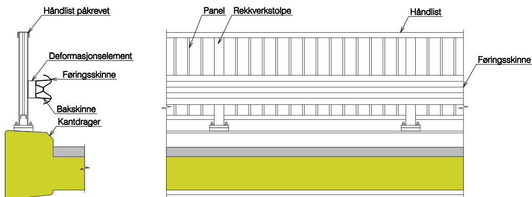
Figur 1.2 Ettergivende ståltrekkverk
