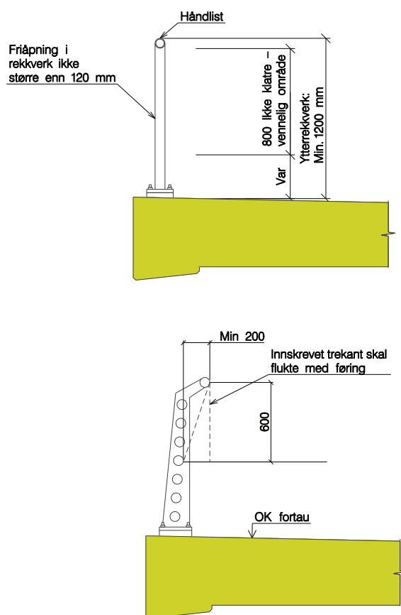
Figur 3.6 Sikring mot klatring
