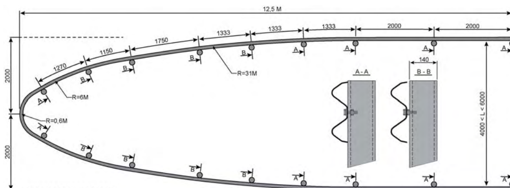
Figur 23. SVS-endeend
