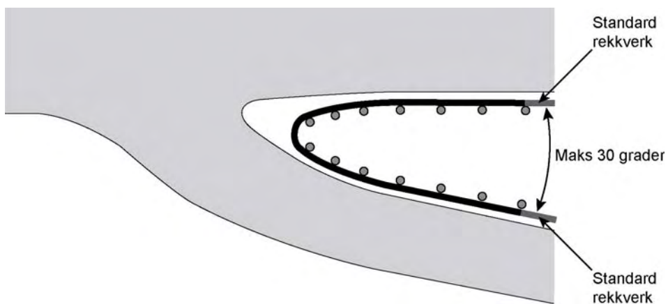
Figur 26. Avkjøring til sideveg under 30 grader.
