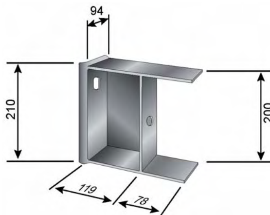
Figur 7. Standard utblokkingsbøyle
