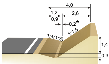
b) skråningshelning 1:1,5
