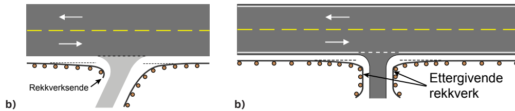
Figur 4.6 a)-b) Eksempler på avslutninger av rekkverk ved vegkryss og avkjørsle
