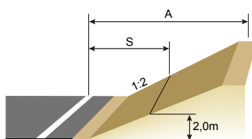
b) Stigning 1:2
