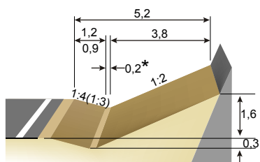
a) skråningshelning 1:2
