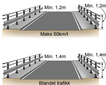
Figur 3.9 Minstekrav til brekkverk på bruer med gangtrafikk
