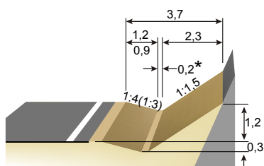
b) skråningshellning 1:1,5
