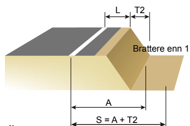
Figur 2.4 Sikkerhetssonens bredde ved fallende terreng
