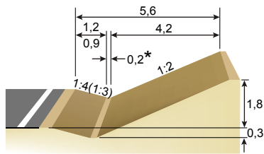
a) skråningshelning 1:2
