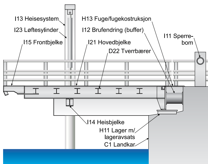
Lengdesnitt
