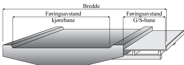
Fig. 7.9.1-7 : Skisse som viser føringsbredder for beregning av kjørebane- og G/S-areal
