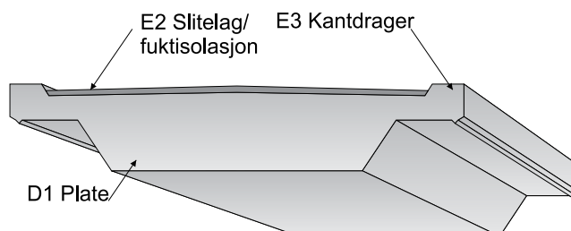
Fig. 5.5.4-1: Element D1 Plate og elementer for slitelag/ fuktisolasjon og kantdrager
