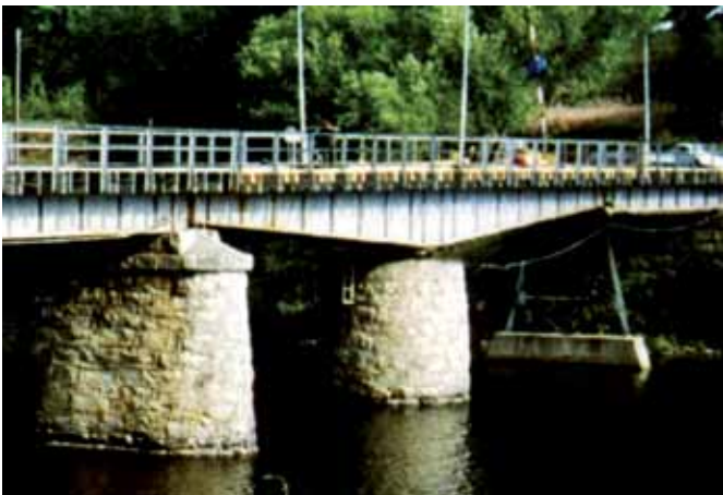
Fig. 4.3.8-6: Svingbru, likearmet, bjelker. Byggverkstype 861
