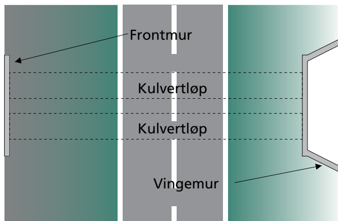
Fig. 5.5.6-2: Element F Konstruksjoner i fylling, Rørkulvert med to løp og vingemur
