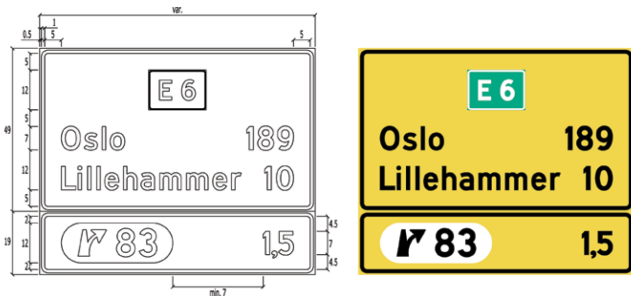
Eksempel på skilt 725.2 på tofelts (motortrafikk)veg.
