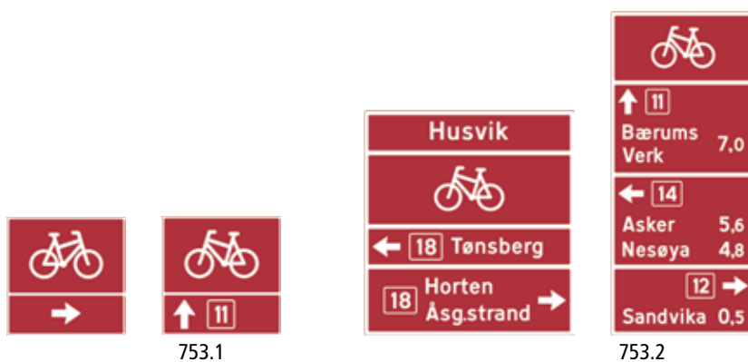
Figur 4-4.74 Utføringsvarianter for skilt 753 (eksempler)
