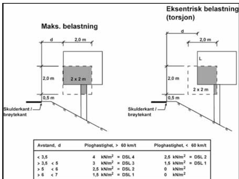
Fig. 77 Bestemmelse av dynamisk snøbrøytebelastning (DSL-klasse) på trafikkskilt montert på stolper og master
