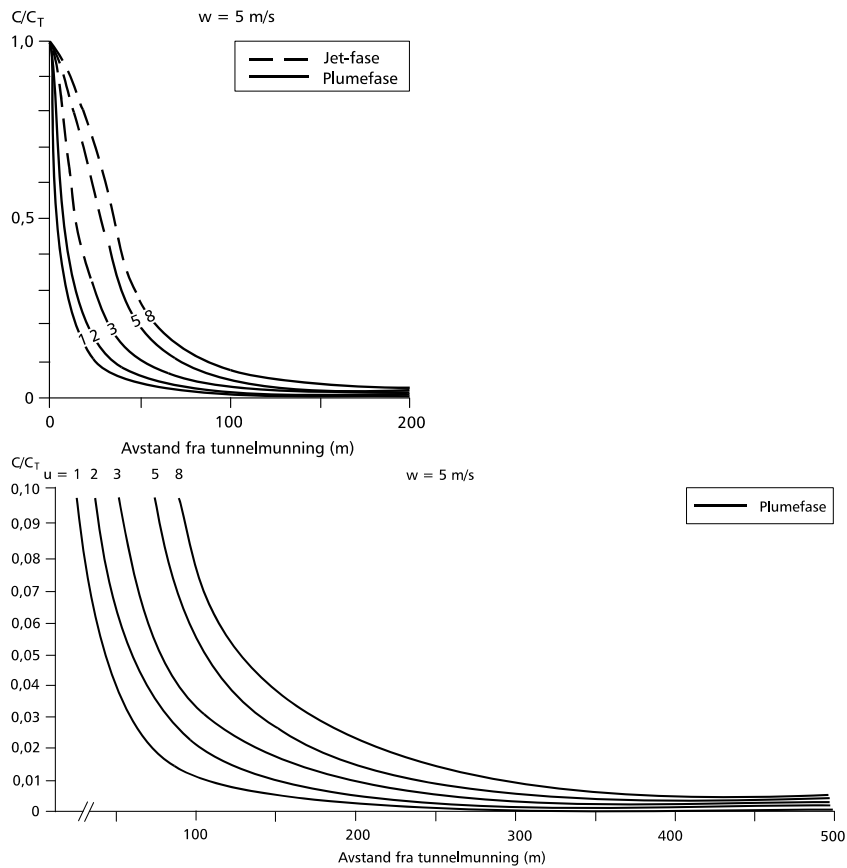
Figur A.4 Nomogrammer for spredningsberegninger vindhastighet w = 5 \text{ m/s}
