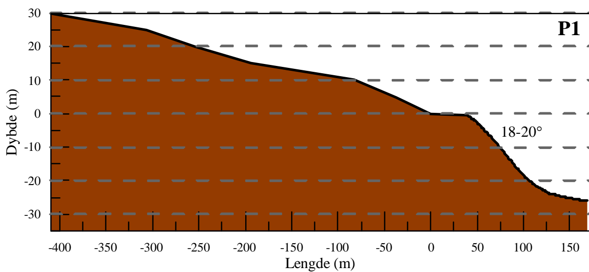
Figur D3: Topografiske profil P1 ved Halvspannet, se Figur D1 og Figur D2 for lokalitet.
