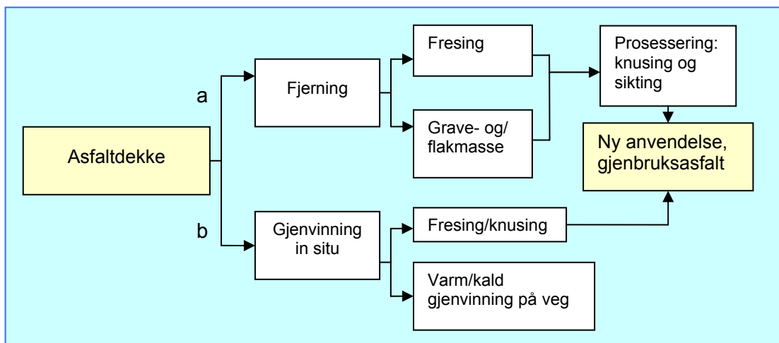
Figur 4: Prosesser ved asfaltgjenvinning: (a) fjerning av gammelt asfaltdekke ved fresing eller graving, etterfulgt med knusing og sikting; eller (b) gjenvinning på stedet
