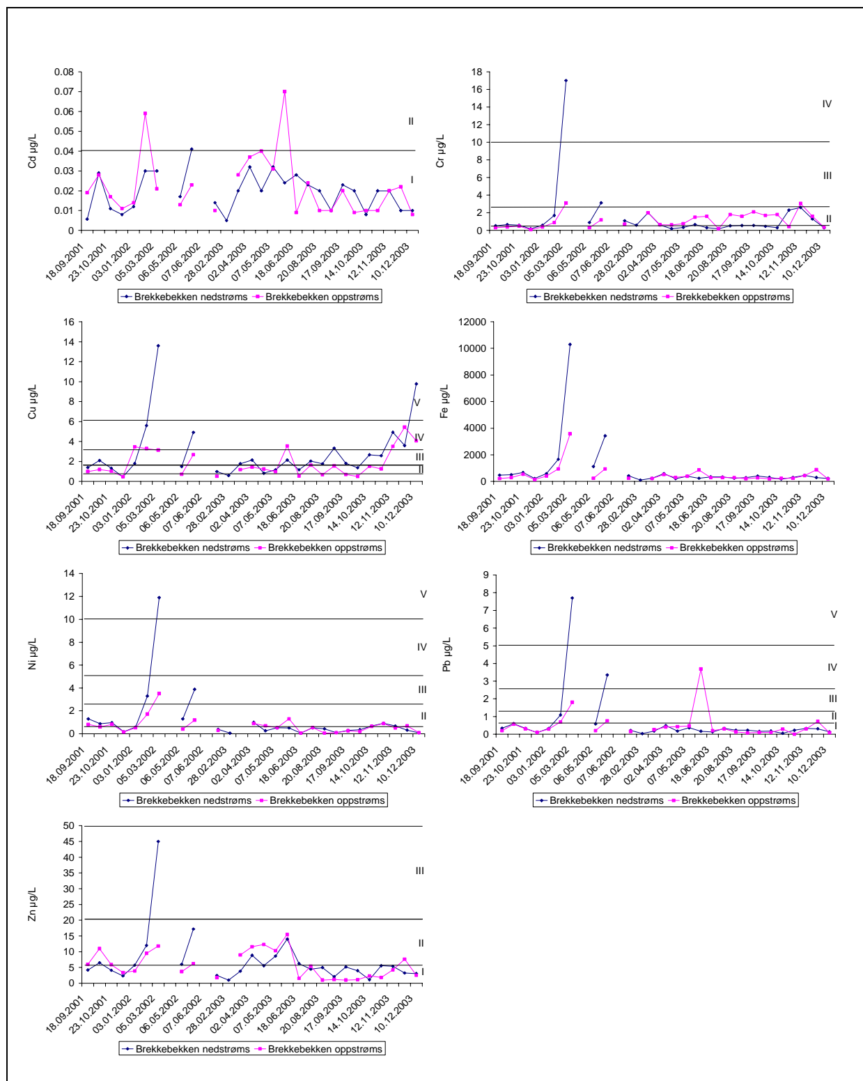
Figur 11. Konsentrasjoner av utvalgte tungmetaller 2001-2003 i Brekkebekken oppstrøms og nedstrøms E18. Vegen åpnet 31.10.2001.
