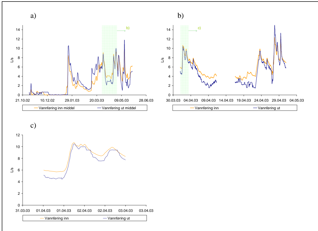
Figur 21. Data fra februar – mars 2002 med ulik grad av oppløsning: a) døgnmiddel, b) 5 - minutters intervall over ca 1 mnd., c) 5 - minuttintervall over ca 2 døgn. Farget felt angir utsnitt for neste figur.
