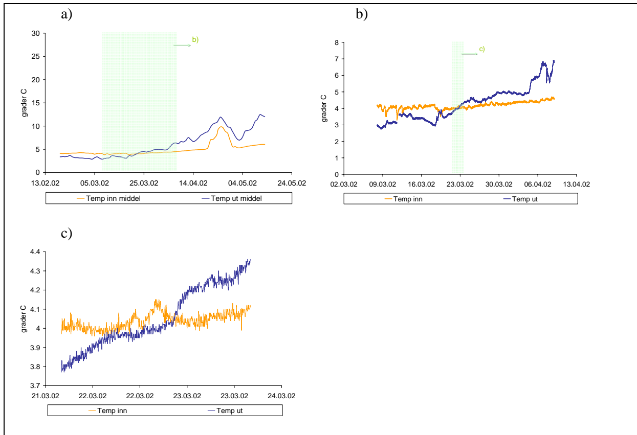
Figur 27. Data fra februar – mars 2002 med ulik grad av oppløsning: a) døgnmiddel, b) 5 - minutters intervall over ca 1 mnd., c) 5 - minuttersintervall over ca 2 døgn. Farget felt angir utsnitt for neste figur.
