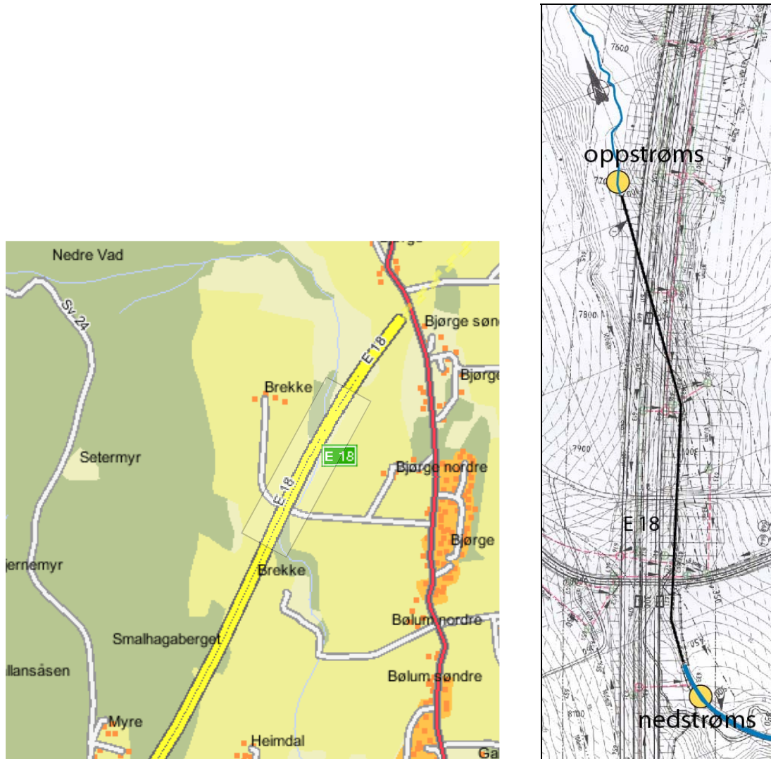
Figur 6. Beliggenhet av Brekkebekken og stasjonsplassering oppstrøms og nedstrøms E 18. Blå farge viser hvor bekken går åpent, mens svart viser hvor bekken går i kulvert.
