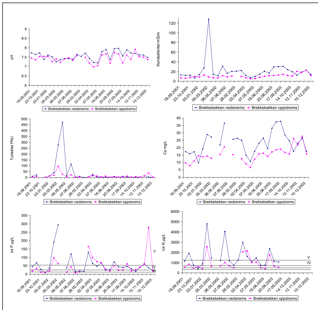
Figur 8. Konsentrasjoner av utvalgte kjemiske parametere 2001-2003 i Brekkebekken oppstrøms og nedstrøms E18. Vegen åpnet 31.10.2001.
