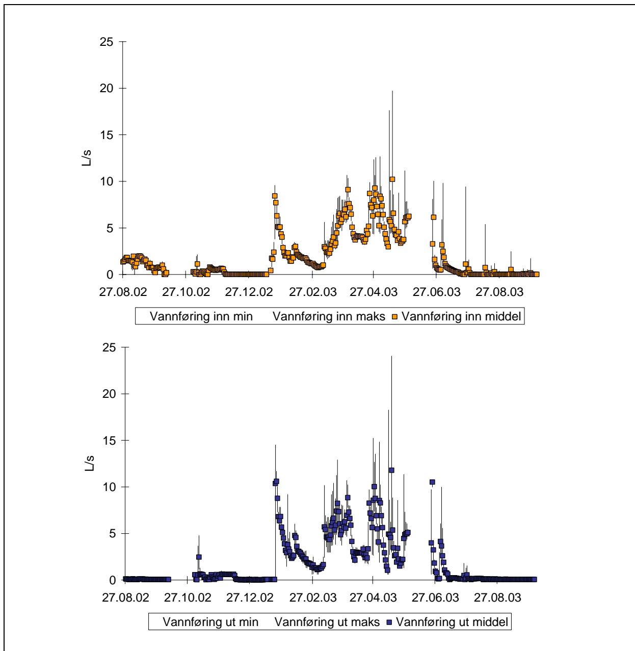
Figur 18. Vannføring målt ved innløp og ved utløp fra august 2002 til oktober 2003. Angitt som døgnmiddel og som maksimums- og minimumsverdier per døgn.
