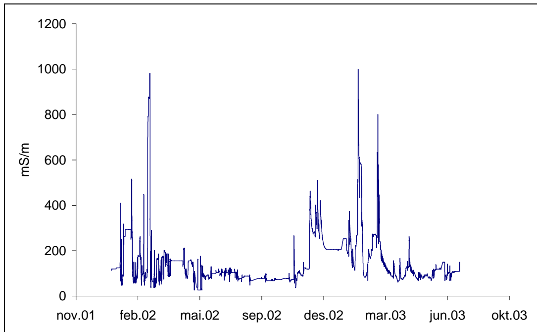
Figur 10. Konduktivitet målt ved Gutu/Skoer målestasjon i 2002 og halve 2003.
