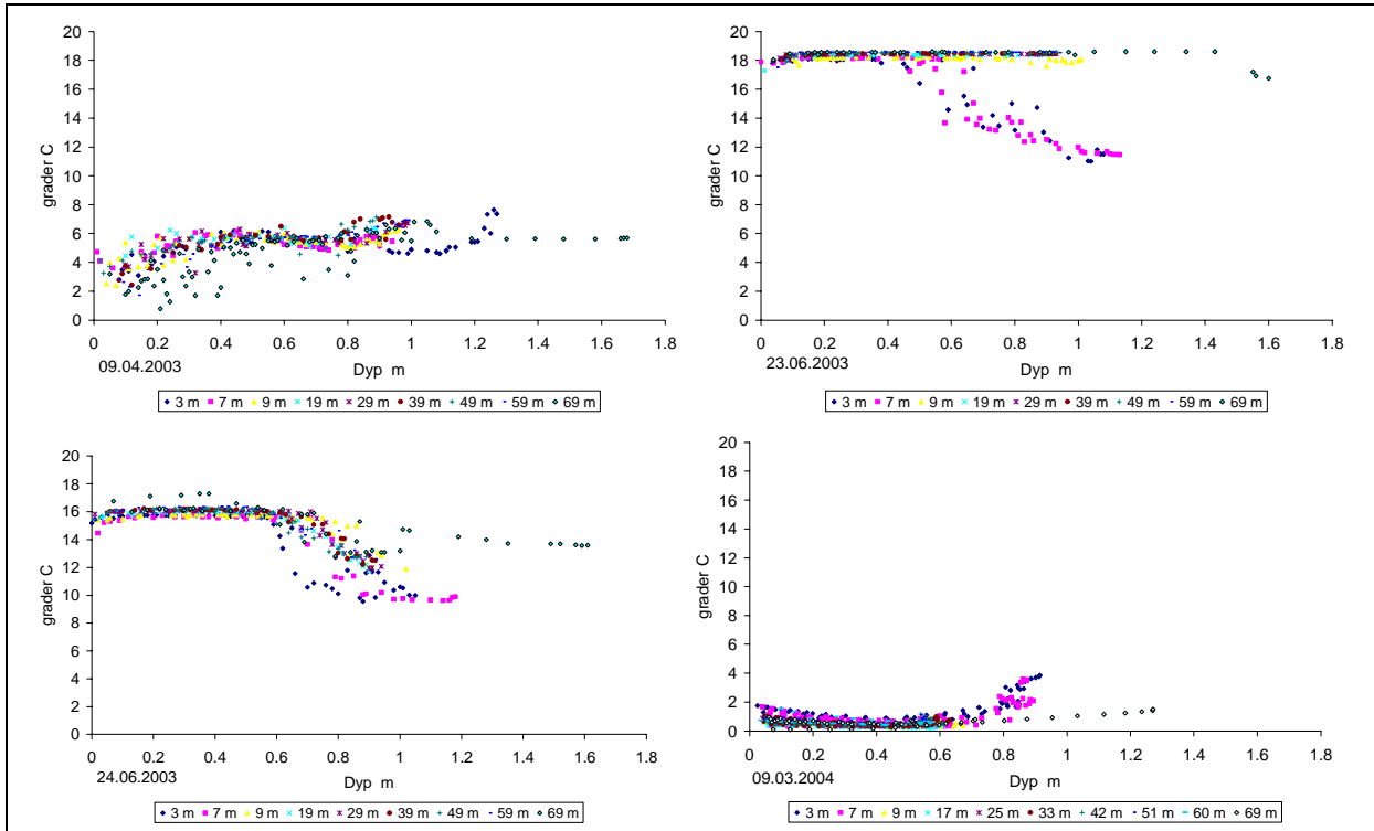
Figur 36. Fordeling av alle temperaturmålinger i dyptet for hver dato. Angitt for hvert prøvetakingstverrsnitt av bassenget.
