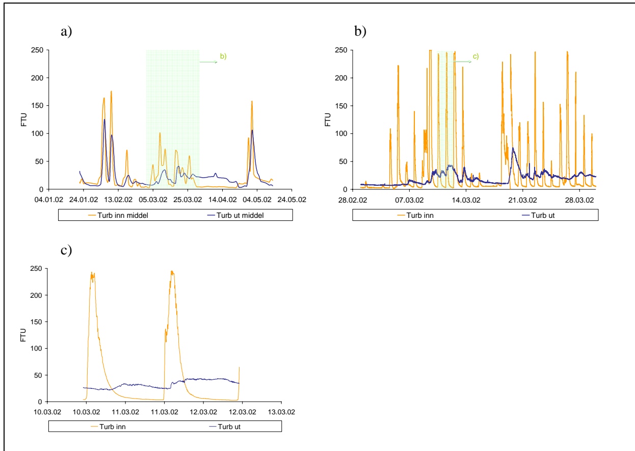
Figur 31. Data fra februar – mars 2002 med ulik grad av oppløsning: a) døgnmiddel, b) 5 - minutters intervall over ca 1 mnd., c) 5 - minuttersintervall over ca 2 døgn. Farget felt angir utsnitt for neste figur.
