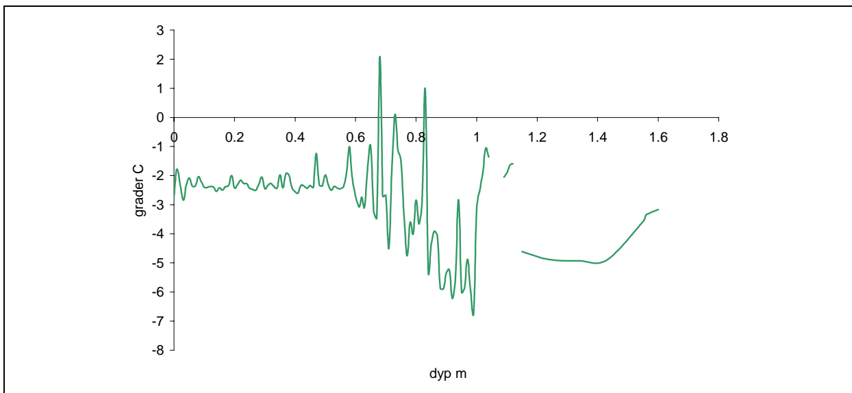
Figur 36. Fordeling av alle temperaturmålinger i dyptet for hver dato. Angitt for hvert prøvetakingstverrsnitt av bassenget.
