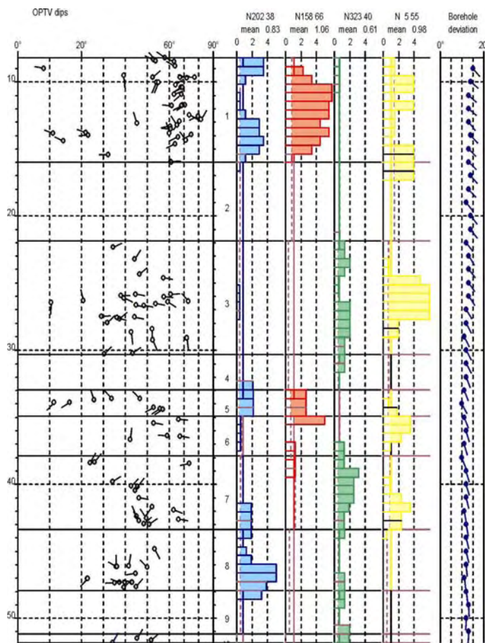
Figur 5. Sprekkelogg for tolket borehull. Til venstre vises de individuelle sprekke-plott. Pilhodene angir individuelle sprekkers fall, mens halen viser fallretning (nord opp). Histogrammene viser hvor i borehullet de forskjellige sprekke-mønstre opptrer (sprekkefrekvens). Høyre kolonne viser borehullsforløp med fall og retning. Heltrukne horisontale linjer angir grenser mellom definerte soner.
