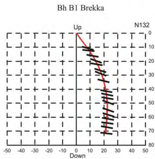
Bh B1 Brekka. Vertikalprosjeksjon i hullretning N132. Gjennomsnittlig strøk og fall N026 11.
