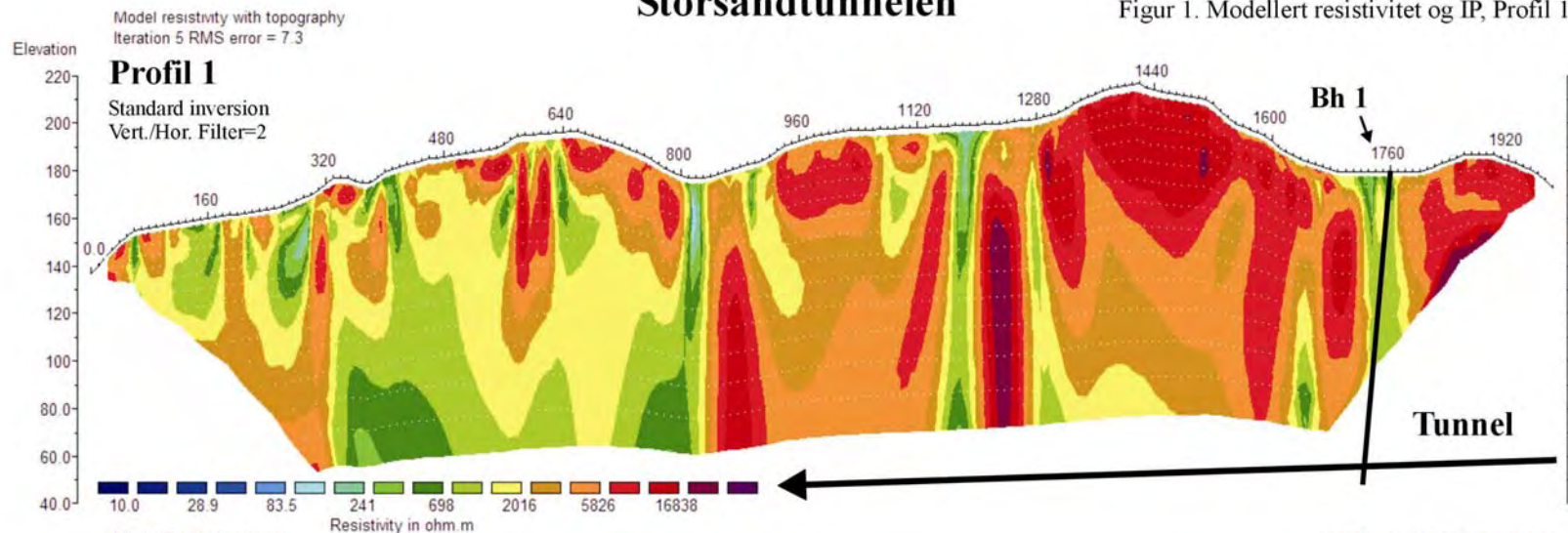
Figur 1. Modellert resistivitet og IP, Profil 1
