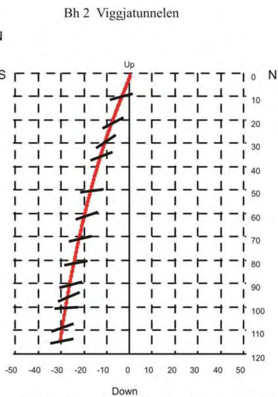
Bh 2. Vertikalprosjeksjon N - S med lagdelingens fallvinkel. Gjennomsnittlig strøkkretning og fallvinkel er N 72 13.
