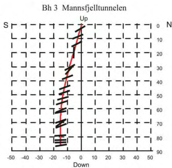
Bh 3. Vertikalprosjeksjon N-S med lagdelingens fallvinkel. Gjennomsnittlig strøkkretning og fallvinkel er N 80 19.
