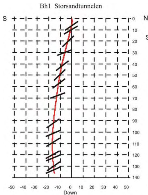
Bh 1. Vertikalprosjeksjon N - S med lagdelingens fallvinkel. Gjennomsnittlig strøkkretning og fallvinkel er N 89 32.
