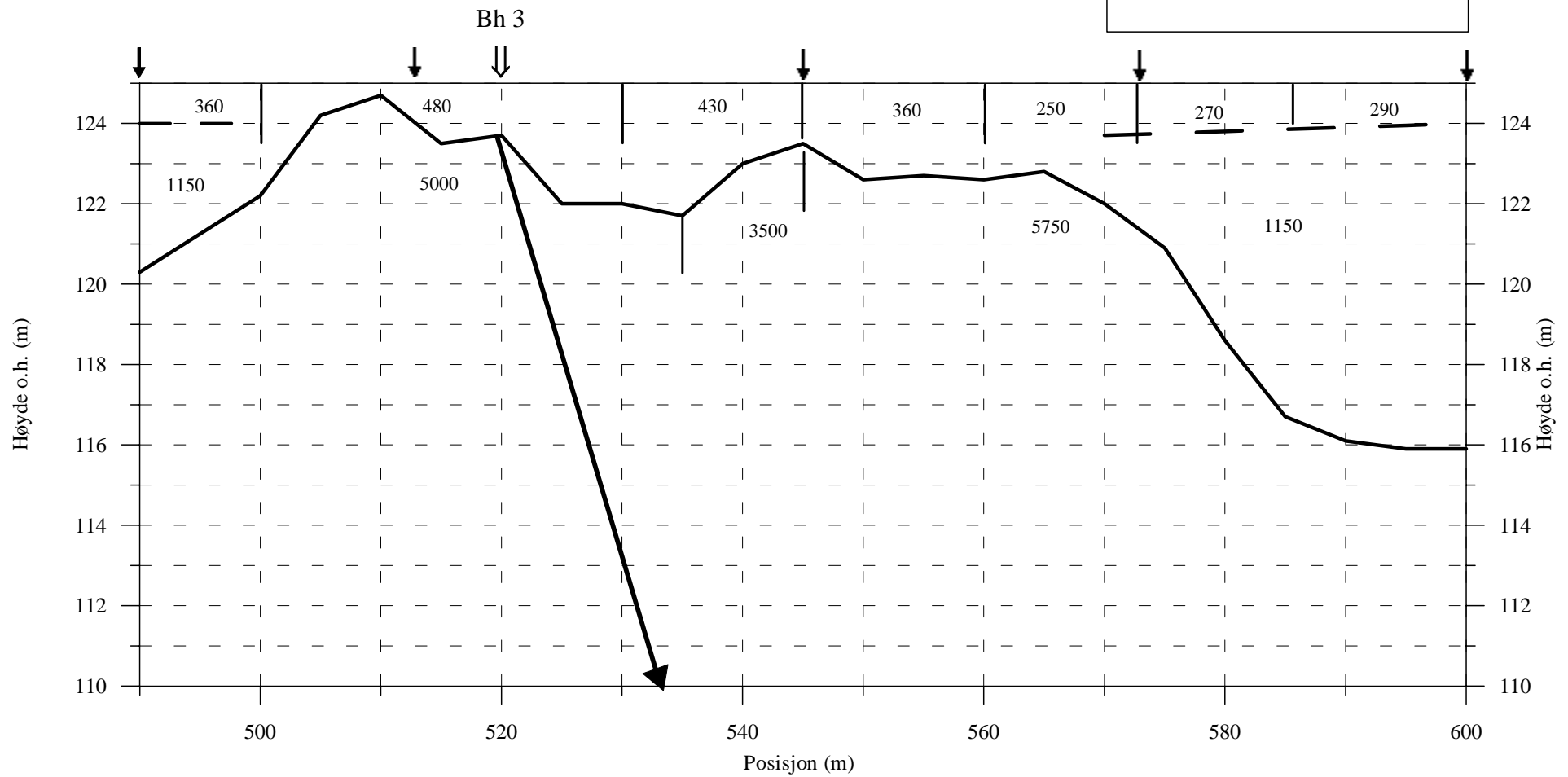
Figur 9. Mannsfjelltunnelen, tolkning av seismisk profil S3.
