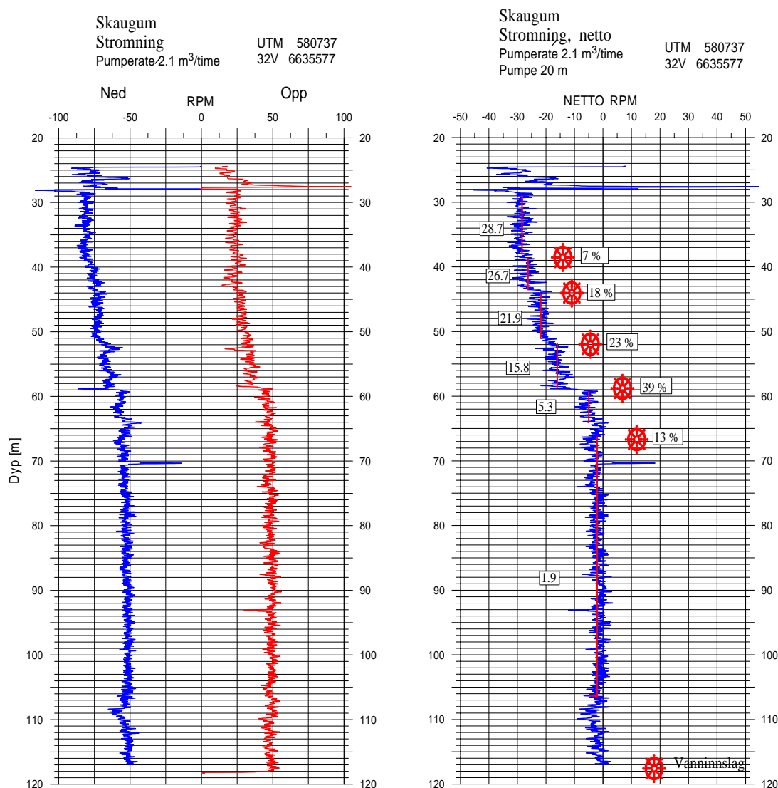
Figur 23. Bh 1, Skaugum. Strømningsmåling. Kontinuerlig logg med hastighet 5 m/min (til venstre). Netto strømming (omdreiningstall) med indikert vanninnstrømning (til høyre).
