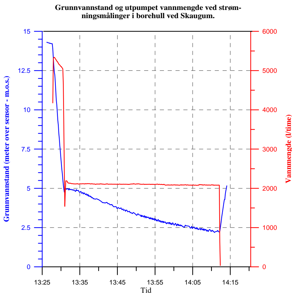
Figur 22. Grunnvannsstand og utpumpet mengde ved strømningsmålinger i borehull ved Skaugum.
