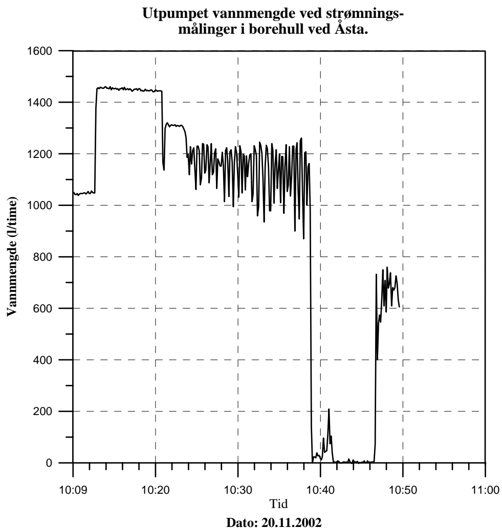
Figur 26. Åstad. Utpumpet vannmengde i borehull
