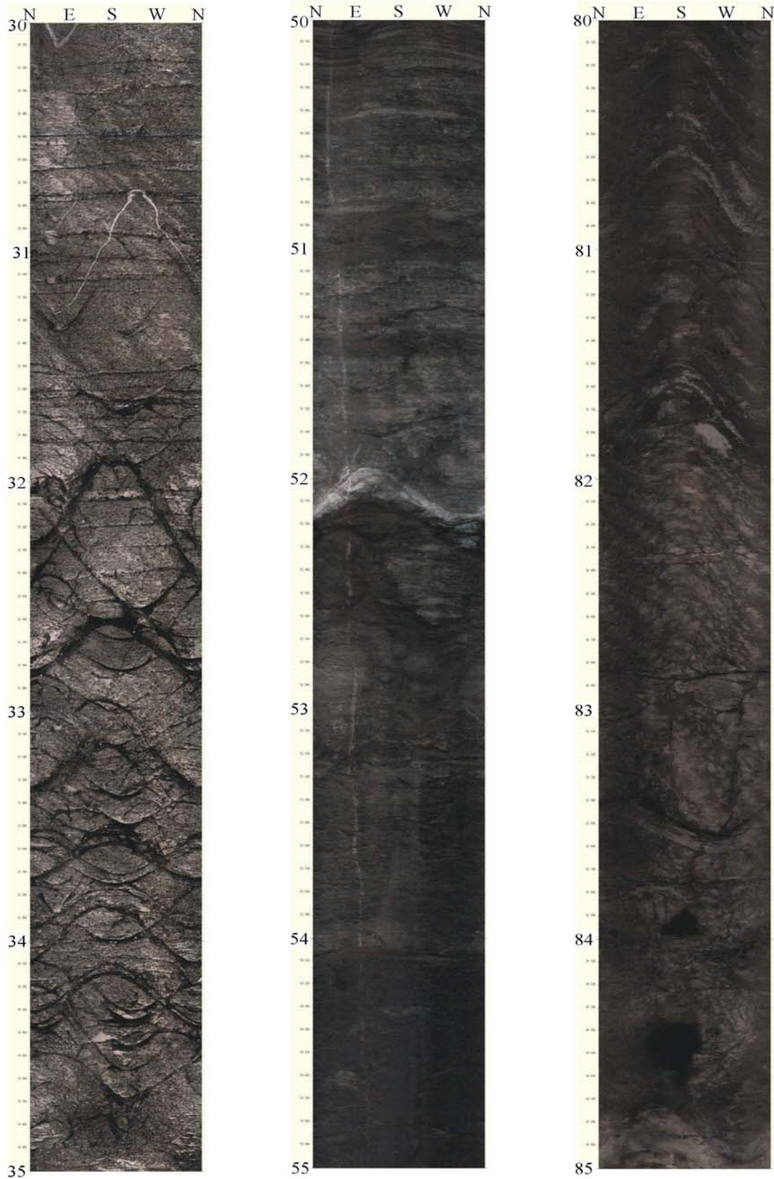
Figur 17. Bh 3, Staverhagan. Bildelogg av seksjoner fra borehullet. 30-35 m (oppsprukket lavabergart), 50-55 m(Askergruppen) og 80-85 m (Kambro silur).
