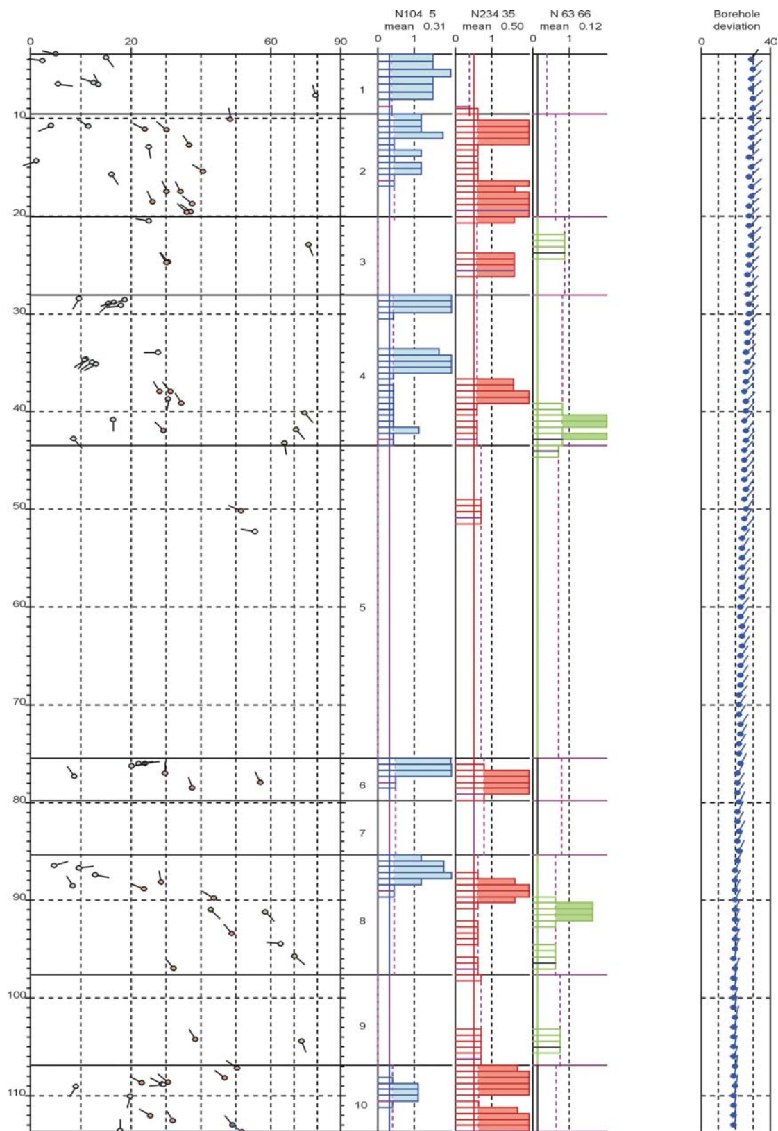
Figur 13. Bh 2, Åstad. Frekvenshistogram over indikerte sprekker i borehullet.
