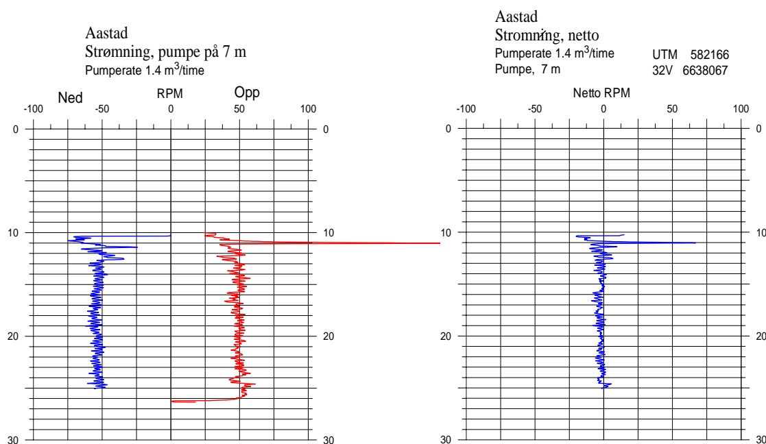
Figur 25. Bh 2, Åstad. Strømningsmåling. Kontinuerlig logg med hastighet 5 m/min, 10-15 m (venstre). Netto strømming med indikert vanninnstrømning ved ca 11 m (til høyre).
