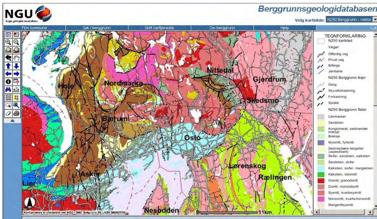
Figur 1. Oversiktskart som viser hovedtrekkene i berggrunnen i Oslo og tilstøtende områder (se NGUs nettside: www.ngu.no ). Kommunegrensene er vist med røde linjer. Se tekst for kort beskrivelse av berggrunnsgeologi. For mer detaljert informasjon om berggrunnen henvises det til NGUs trykte kart over området (Berthelsen et al. 1996, Nordgulen 1999).
