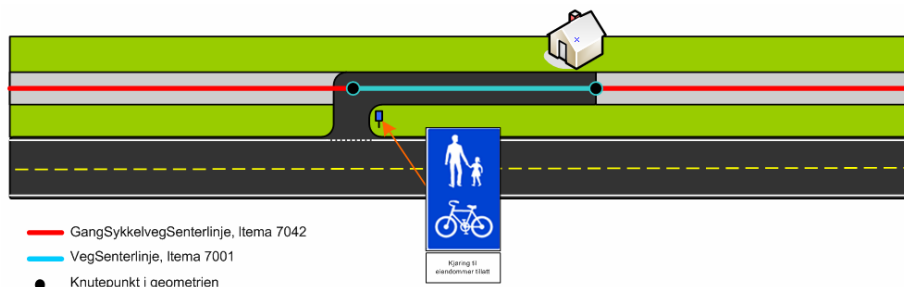
Figur 75 Gs-veg går over veg til eiendom, men denne vege er skiltet som gs-veg. I slike tilfeller skal vege kodes som kjøreveg, men vegkategori vil være gang- og sykkelveg.
