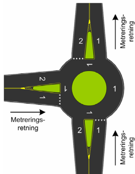
Figur 53: Rundkjøring med ett felt
