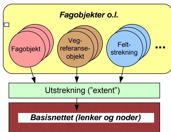
Figur 21: Fagobjekter, vegreferanseobjekter og feltstrekningobjekter (som inneholder feltkoden) spennes ut i basisnettet
