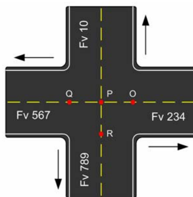
Figur 39: Fv10 er den viktigste vegen og ”eier” dermed arealet i krysset. Strekningene P–Q, P–R og P–O skal ha egenskapen ”sekundærveg type 2”.
