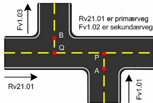
Figur 38: Fellesstrekning i forkjøvet X-kryss. Strekningen P-Q er fellesveg mellom rv. 21 og fv. 1, der riksvegen er primærveg.
