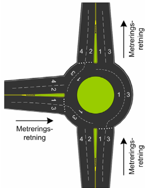
Figur 54: Rundkjøring med flere felt
