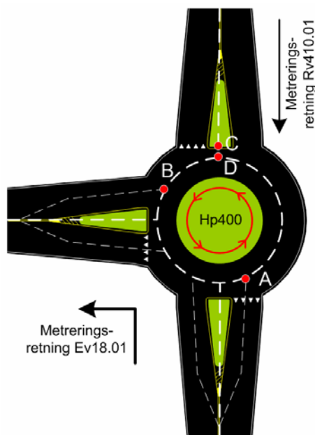
Figur 41: Metring av primærveg og parsellskjøt (sekundær veg type 2) i forbindelse med rundkjøring
