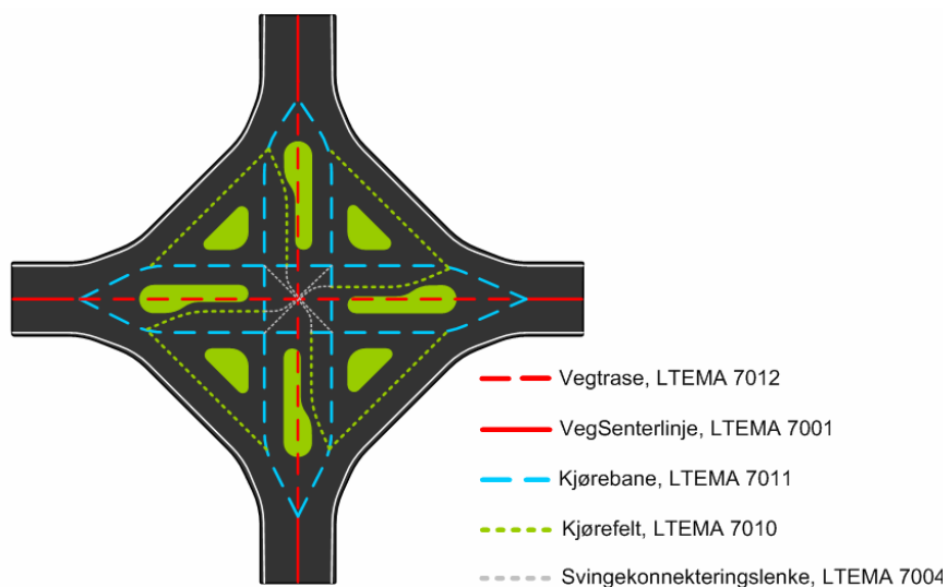
Figur 28: Geometri i kryss, alle nivåer
