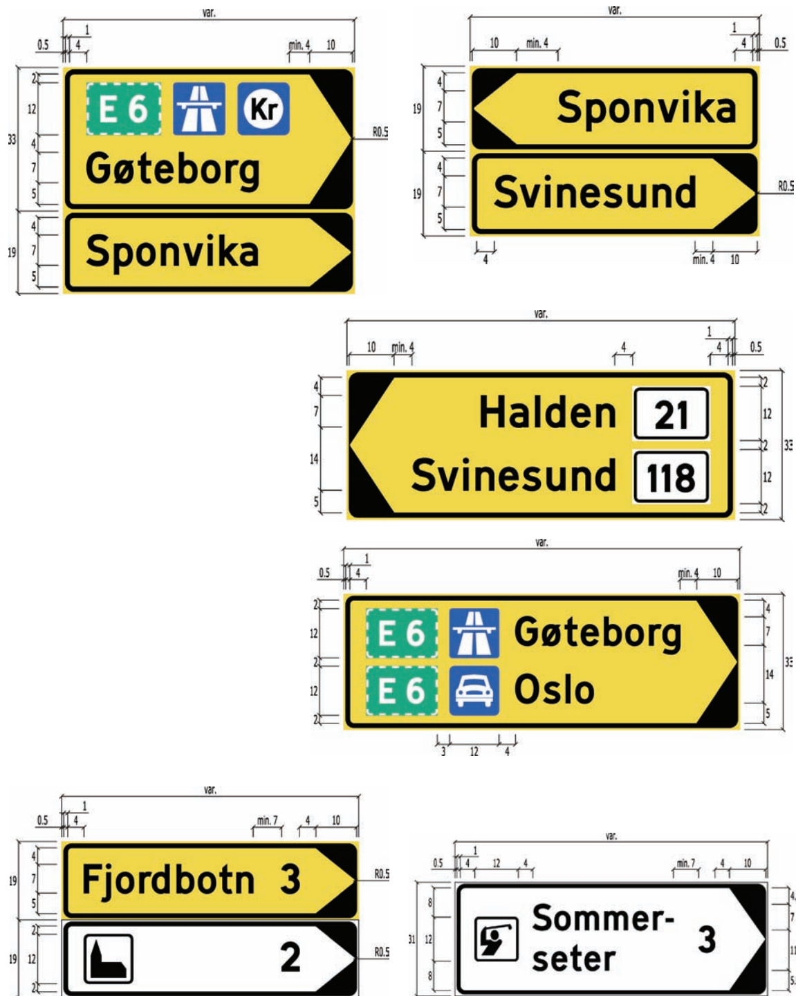
Figur 4-4.37 Eksempler på utforming av skilt 713
