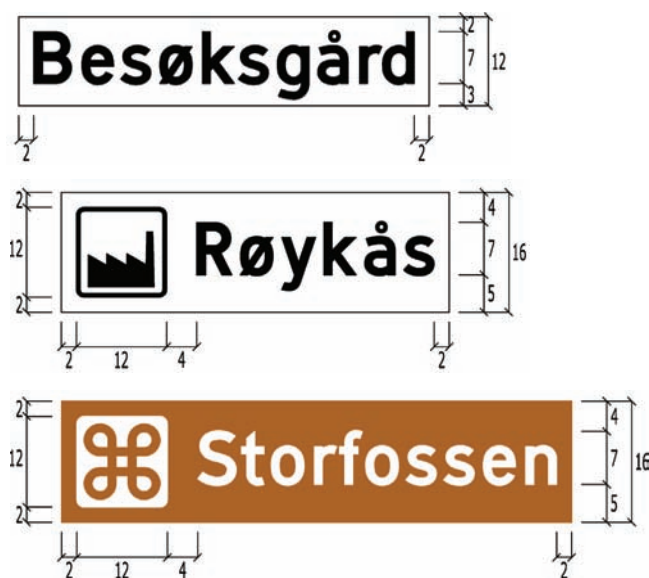
Figur 4-4.11 Plassering av symboler og tekst på felt med avvikende farge. Mål i syvdeler av H
