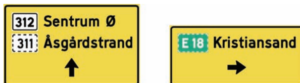
Figur 4-4.41 Eksempler på portalvegviser 719.12
