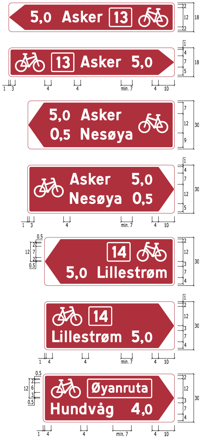
Figur 4-4.73 Eksempler på utforming av skilt 751. Alle mål i 1/7 H.
