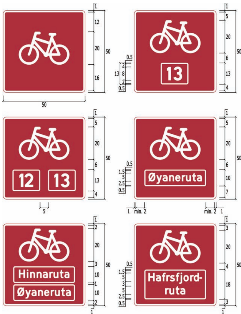
Figur 4-4.80 Eksempler på utforming av skilt 755. Alle mål i 1/7 H
