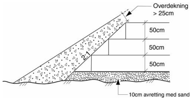
Figur 15.4 EPS fylling – skråningshelning.
