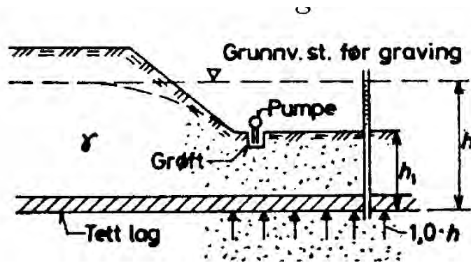
Figur 14.31 Grunnvannsenking ved pumpeump
