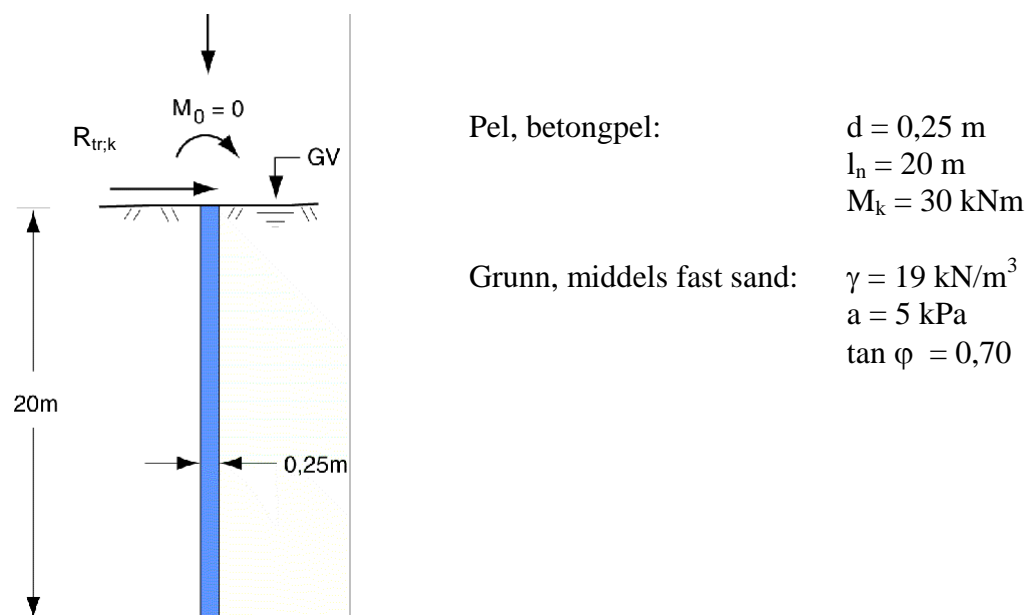
Figur 11. 22 Eksempel - friksjonspeler i sand, horisontal bæreevne
