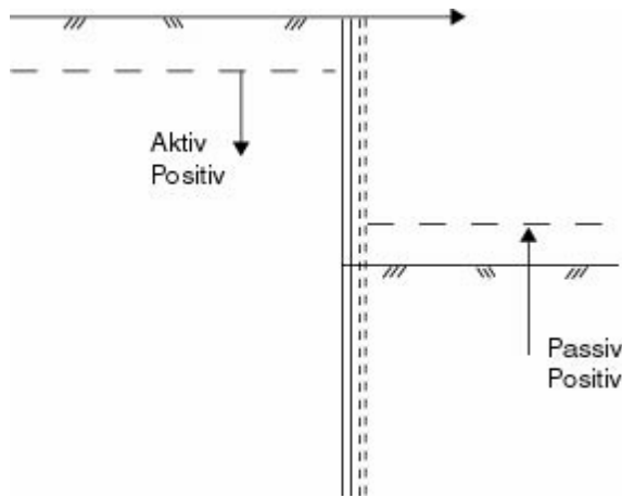
Figur 10.3 Definisjon av positiv ruhet for aktiv og passiv tilstand.
