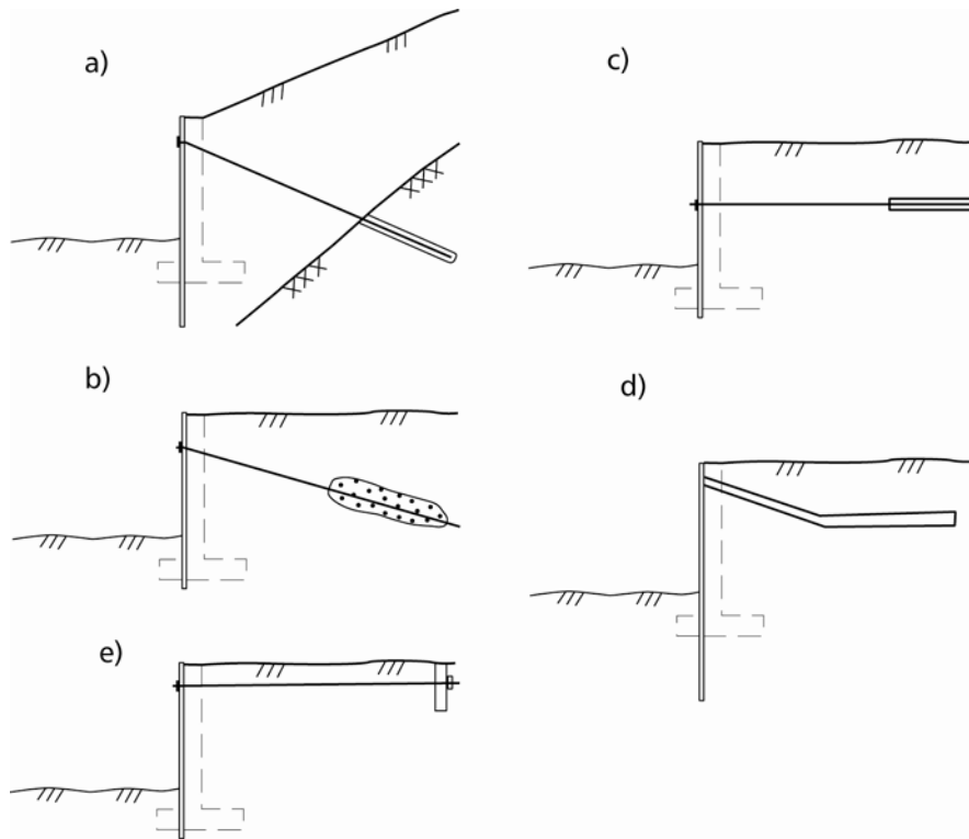
Figur 10.17 Ulike typer forankringer; a) bergstag, b) løsmassestagg, c) horisontal forankringsplate, d) friksjonsplate, e) vertikal forankringsvegg.
