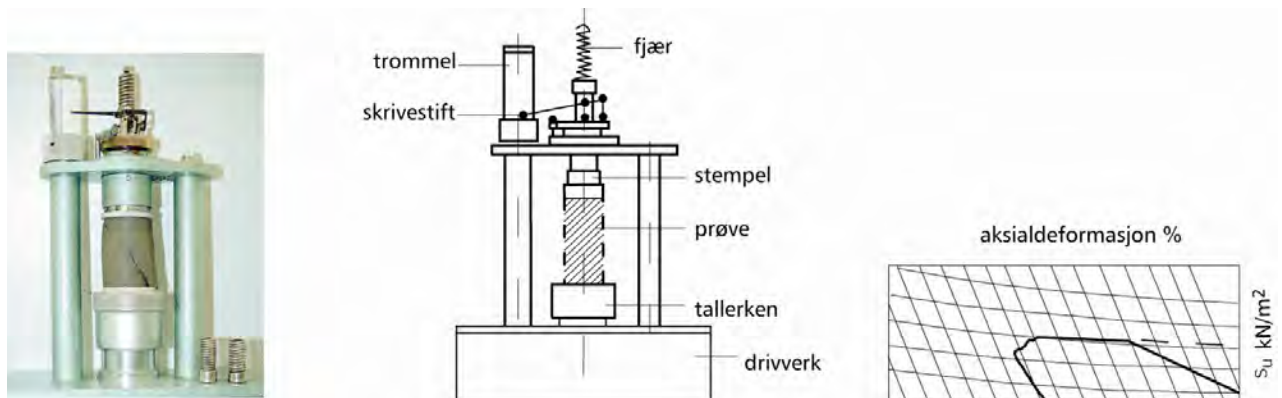
Figur 2.9 Enaksialt trykkapparat.
