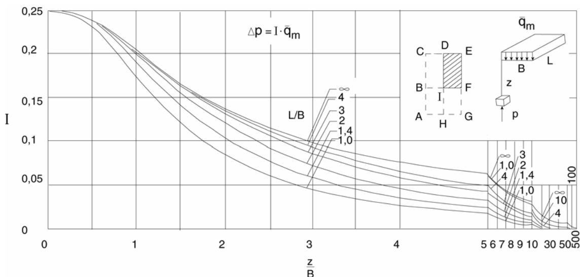
Figur 7.3 Spenningsfordeling for overflatebelastning - elastisk teori. (Boussinesq)
