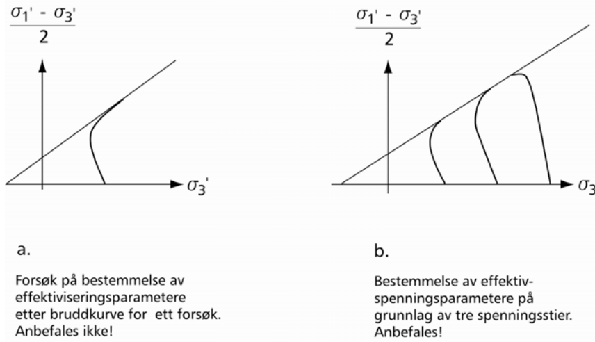
Figur 2.25 Bestemmelse av effektivspenningsparametere
