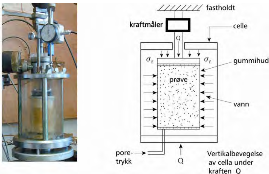
Figur 2.19 Prinsippskisse av treakscelle
