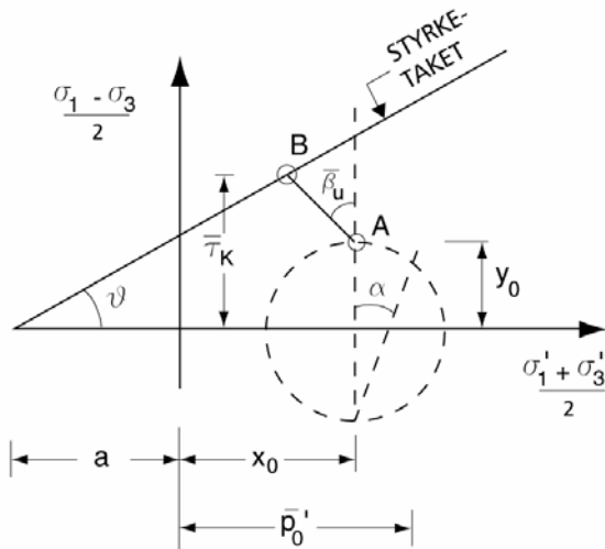
Figur 4.12: Spenningstilstander ved aD\varphi - analyse (MIT – plott)
