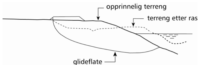
Figur 1.3 Stabilitet av fylling.
