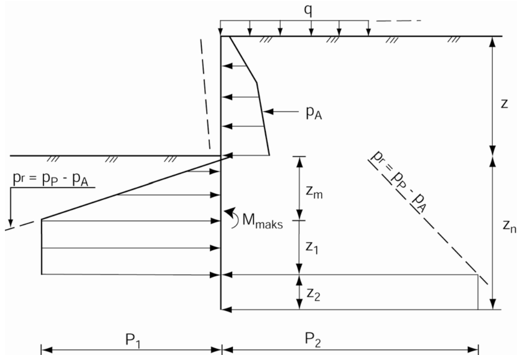
Figur 10. 5 Prinsipp for håndregning av utkraget spunt med spuntfot i løsmasser. Effektivspenningsanalyse.
