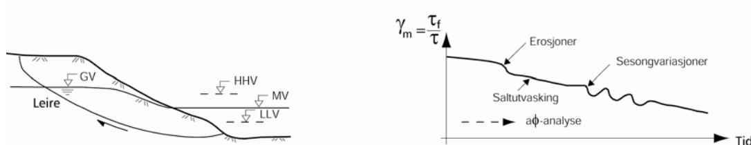
Figur 4.5: Brudd i naturlige leirskråninger (Aarhaug, 1984)
