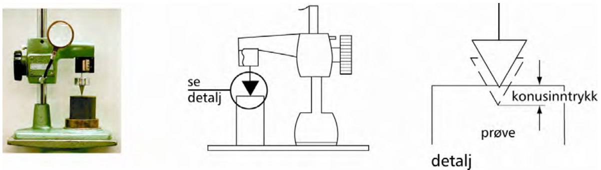
Figur 2.11 Konusapparat
