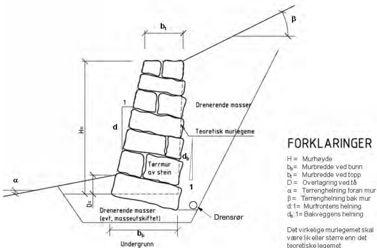
Figur 9.4 Snitt av maskinmurt tørrmur.
