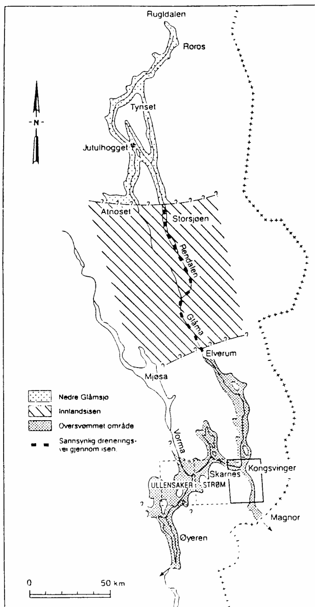
Figur 19.13 Tapningen av den brede sjøen i Nord-Østerdalen – Rendalen. (Longva 1987.)
