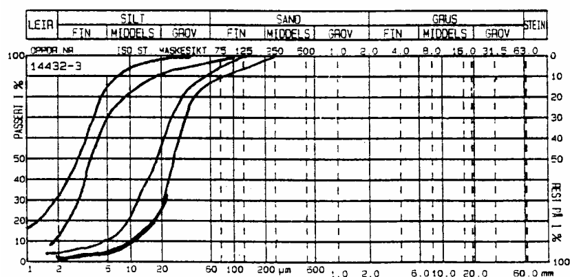
Figur 19.14b Sikteturver fra mørke lag av finsilt og leire og lyse lag av silt og finsand. (Andersen m. fl. 1969.) (se også fig. 19.14a)
