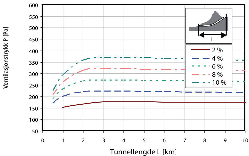
Figur D.10 Ventilasjonstrykk 20 MW brann, jevn stigning og \Delta p = 64 Pa.
