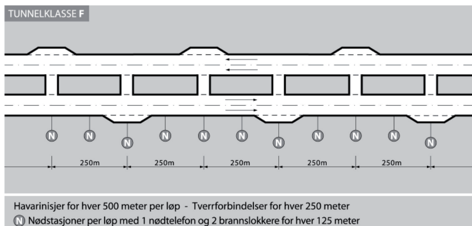
Figur 6.6 Nisjer og utstyr, tunnelklasse F
