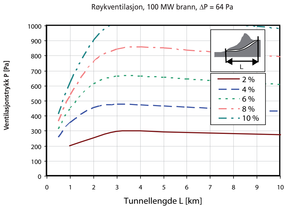
Figur D.32 Ventilasjons trykk 100 MW brann, jevn stigning og \Delta p = 64 Pa.
