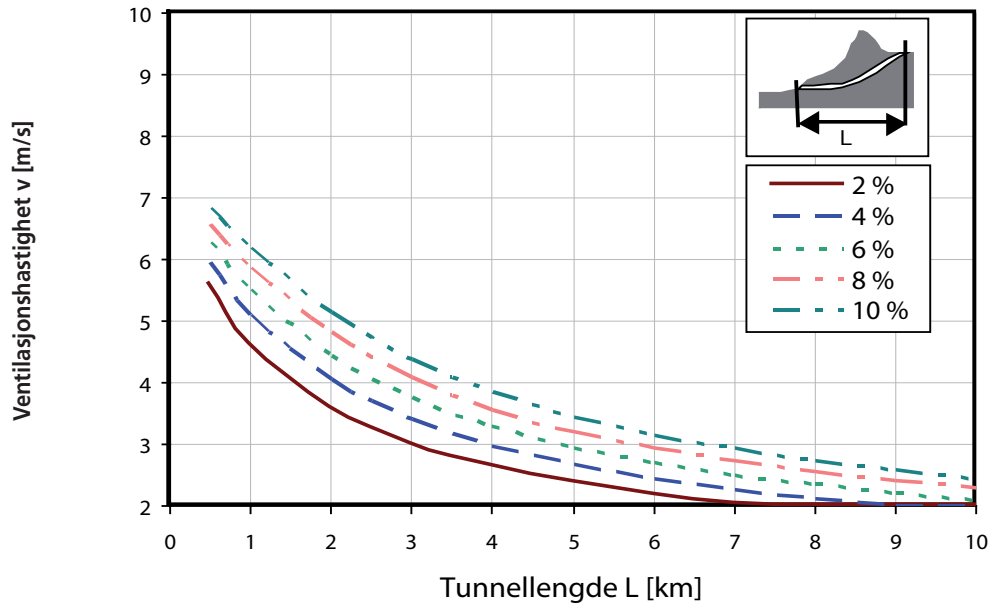
Figur D.9 Ventilasjonshastighet 20 MW brann, jevn stigning og \Delta p = 64 Pa.
