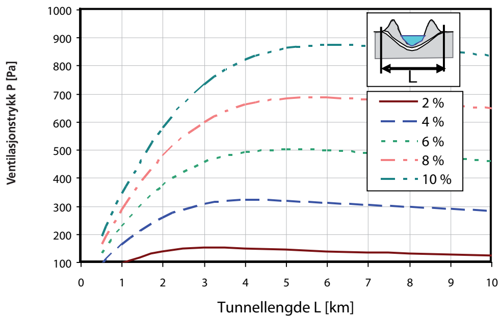
Figur D.20 Ventilasjonstrykk 100 MW brann, stigning over halv lengde og \Delta p = 0 Pa.
