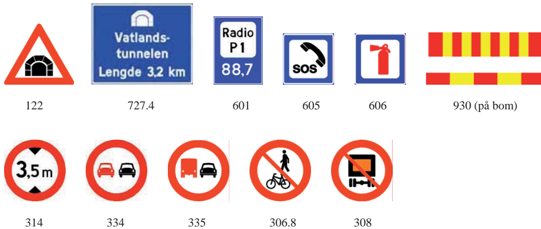
Figur 4.22 Aktuelle skilt utenfor tunnel
