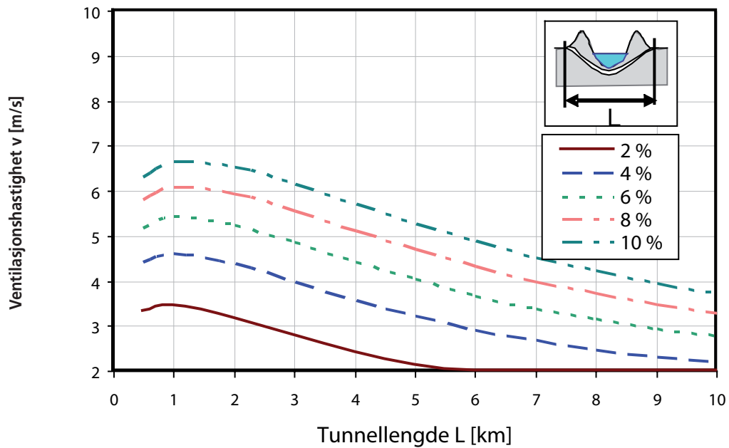
Figur D.19 Ventilasjonshastighet 100 MW brann, stigning over halv lengde og \Delta p = 0 Pa.
