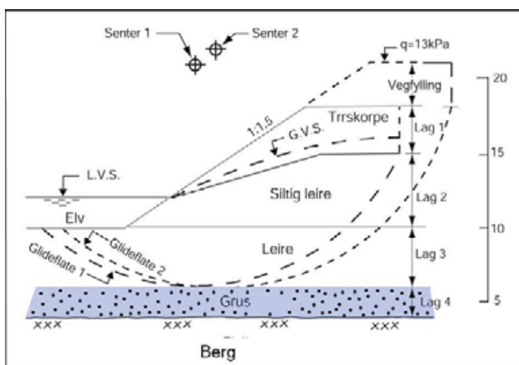
Figur 4. 17 Beregningseksempel
