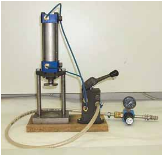
Figur 2.35 Komprimeringsapparat
