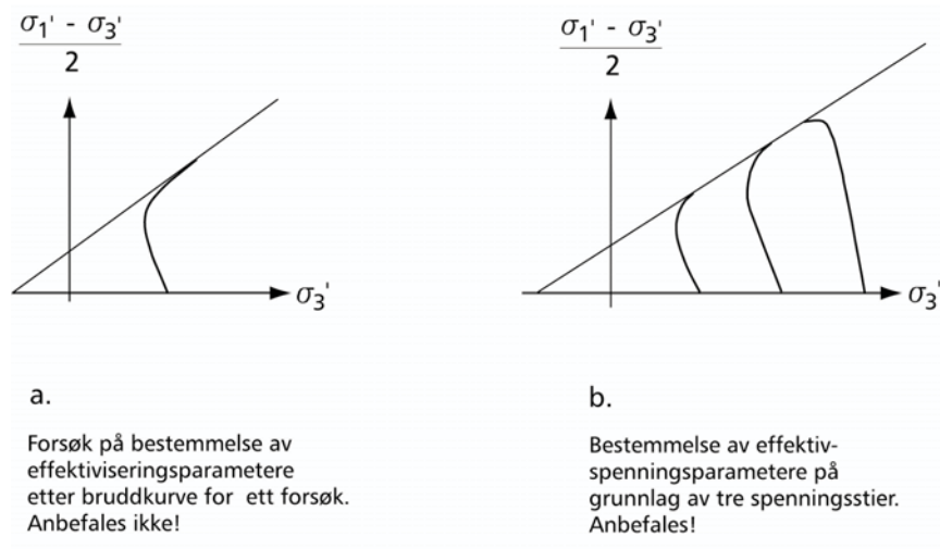
Figur 2.25 Bestemmelse av effektivspenningsparametere
