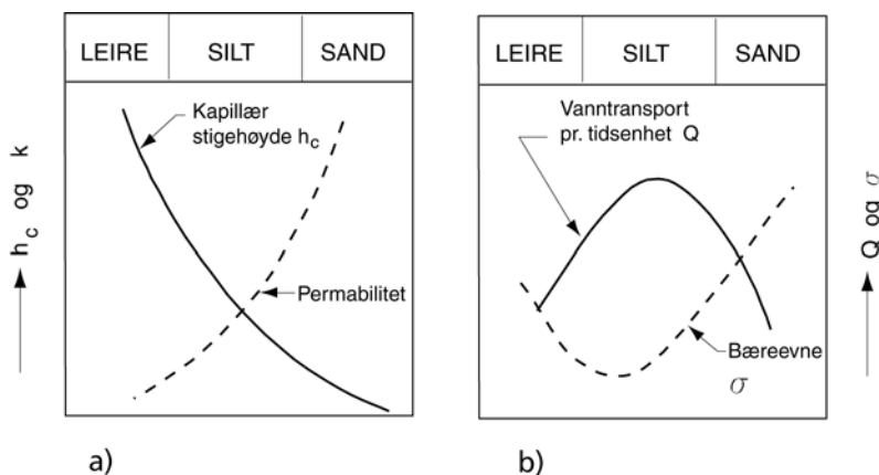
Figur 14.8 Effekter av kapillær oppsuging.
