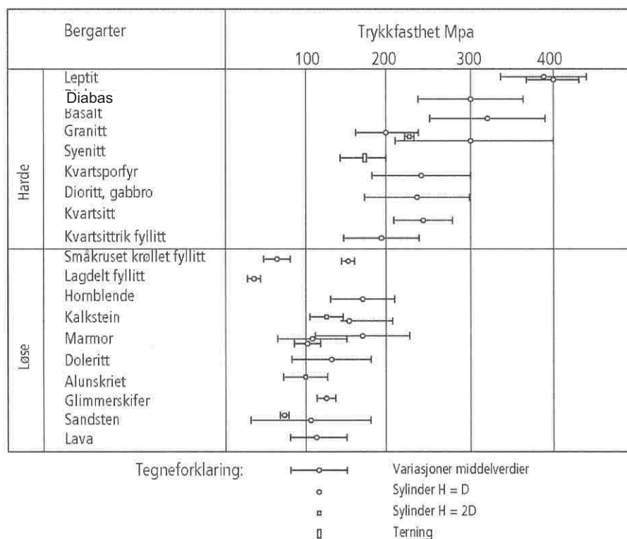
Figur 11. 18 Bergarters trykkfasthet
