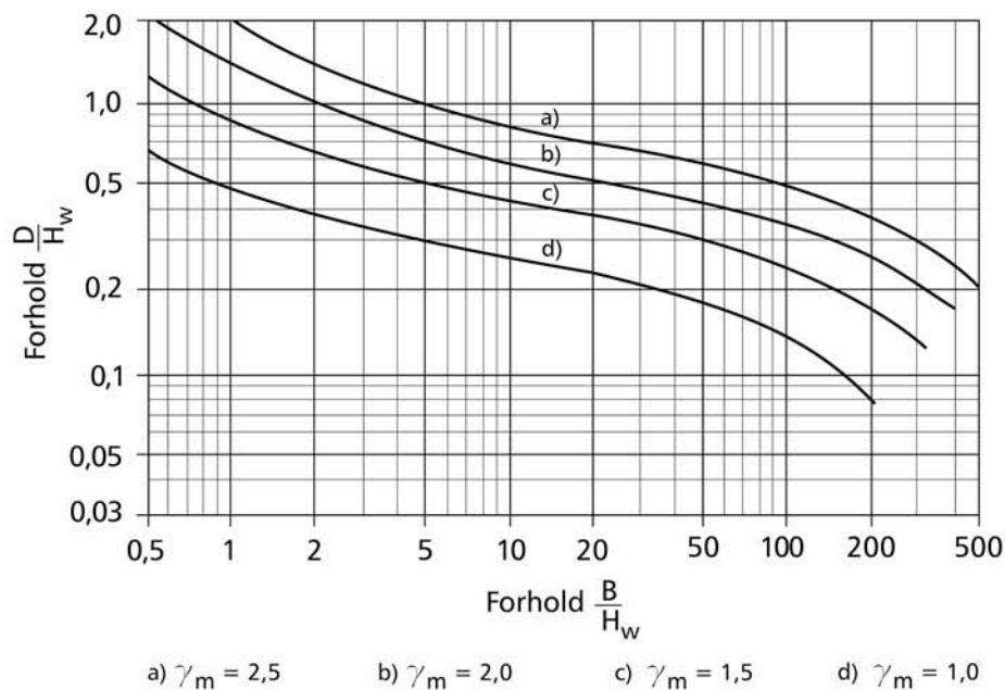
Figur 10. 16 Vurdering av sikkerhet mot hydraulisk grunnbrudd for langstrakt tørrlagt byggegrop mellom avstivede vegger. (Etter Janbu, Bjerrum og Kjærnsli 1956)
