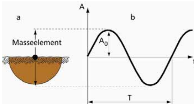
Figur 17.1 Harmonisk svinging
