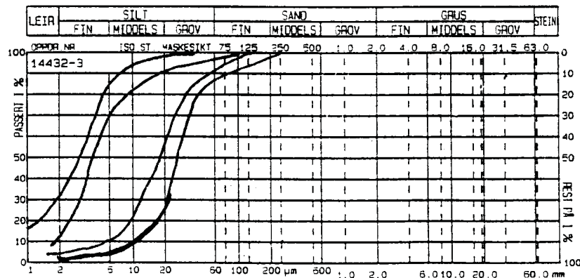
Figur 3.14b Siktetekurver fra mørke lag av finsilt og leire og lyse lag av silt og finsand. (Andersen m. fl. 1969, Ref. 3) (se også figur 3.14a)
