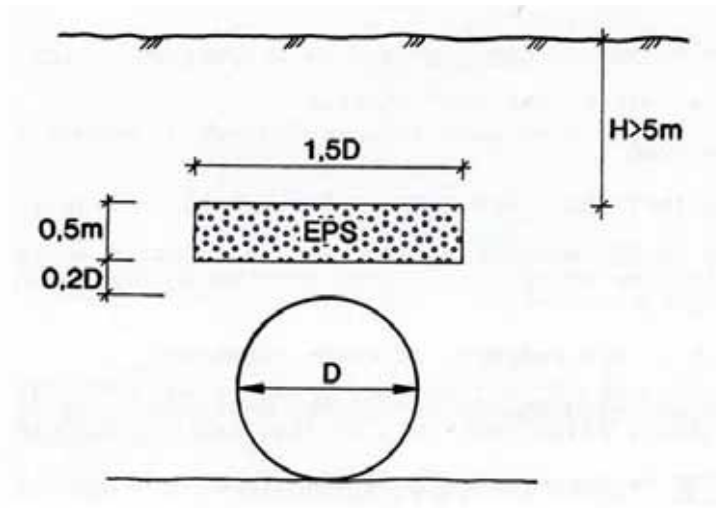
Figur 12. 4 Belastningsreduksjon ved bruk av EPS
