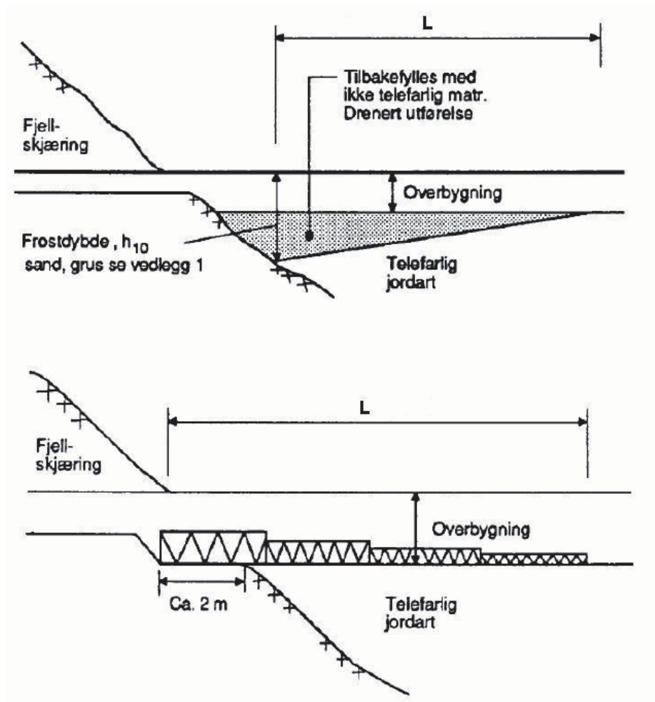
Figur 13.21 Overgang fjellskjæring - telefarlig grunn/underbygning (fra Hb 018, 2005).
