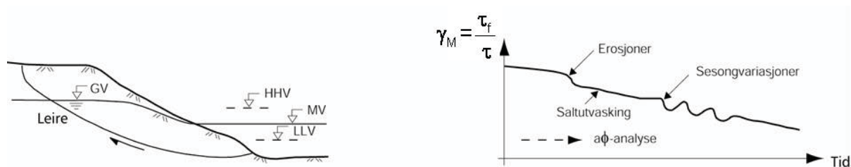
Figur 4.5 Brudd i naturlige leirskråninger (Aarhaug, 1984, Ref. 20)
