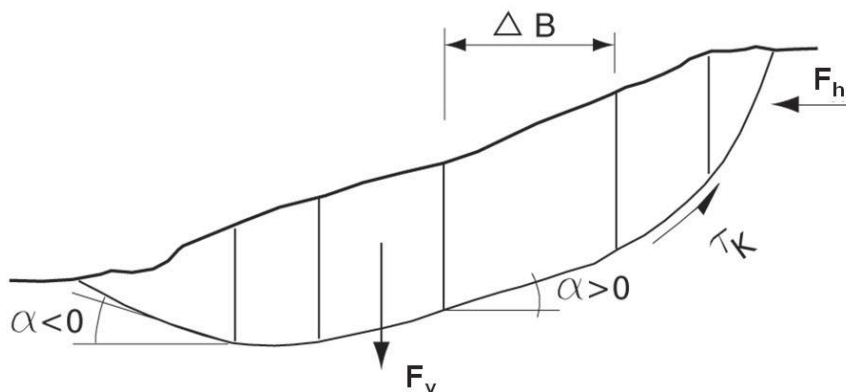
Figur 4.3 Sammensatt skjærflate.
