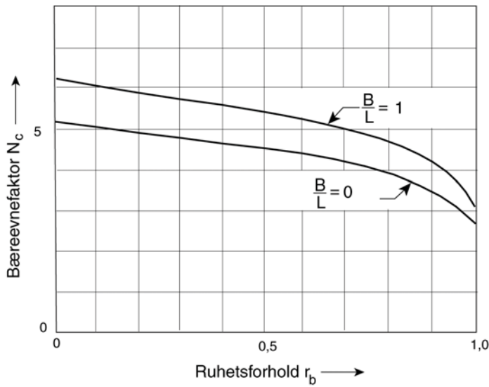
Figur 6.9 Bæreevnepålitelighetsfaktor N_c for totalspenningsanalyse – horisontalt terreng (Etter Janbu, 1973, Ref. 2)
