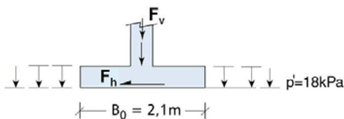
Figur 6.18 Fundament i horisontalt terreng med udrenert kortidslast.
