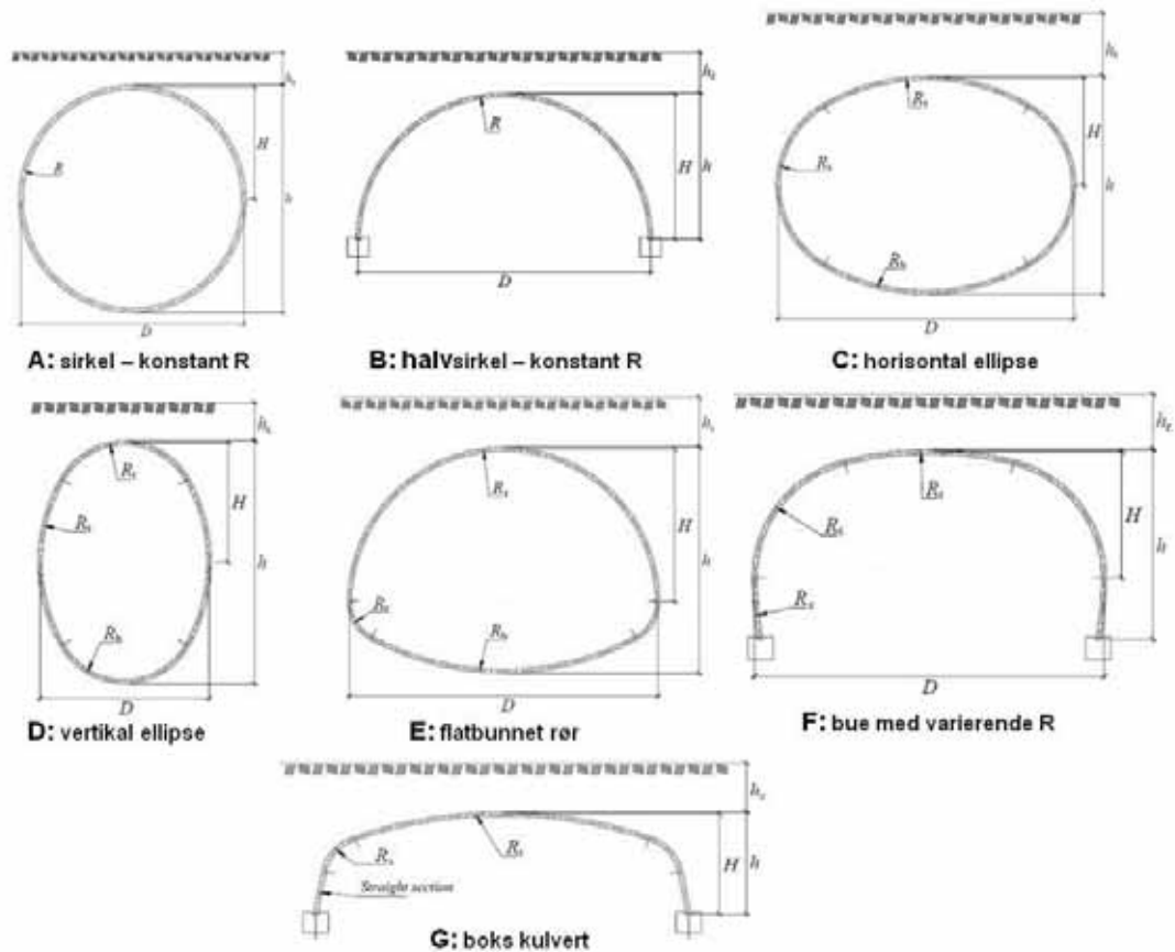
Figur 12. 8 Skisser av ulike tverrsnittformer
