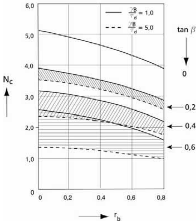
Figur 6.10 Bæreevnepålitelighetsfaktor – forenklet diagram for overslagsberegning, gjelder for B/L = 0 .
