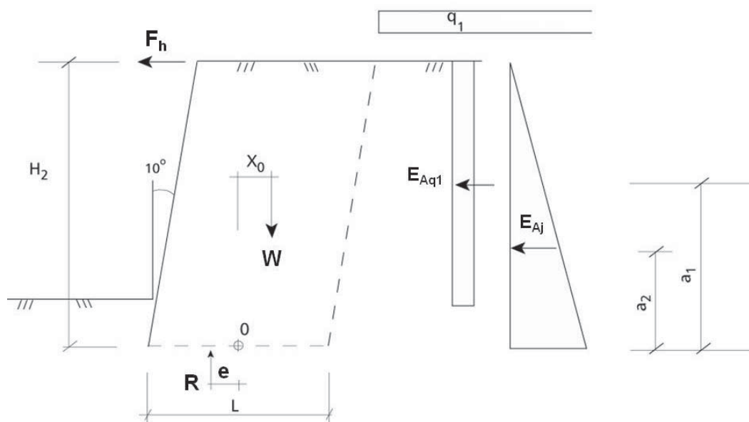
Figur 16.44 Ytre stabilitet.
