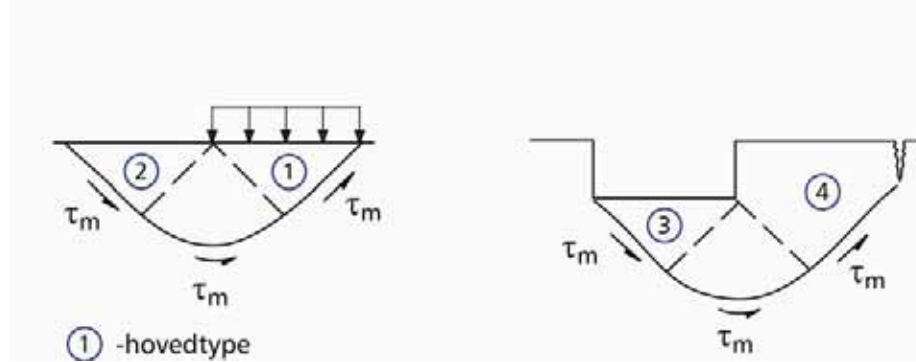
Figur 2.23 Prinsipp for valg av hovedtype treksialforsøk
