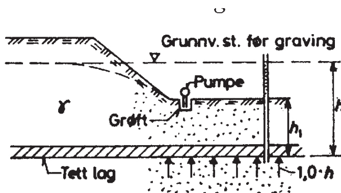
Figur 14.21 Grunnvannsenking ved pumpebasseng
