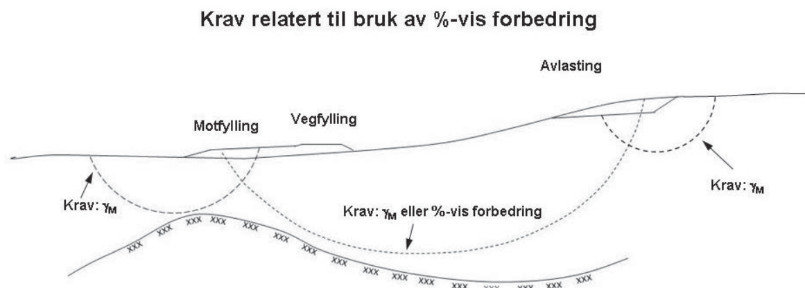
Figur 0.5 Illustrasjon av %-vis forbedring og krav til \gamma_M .
