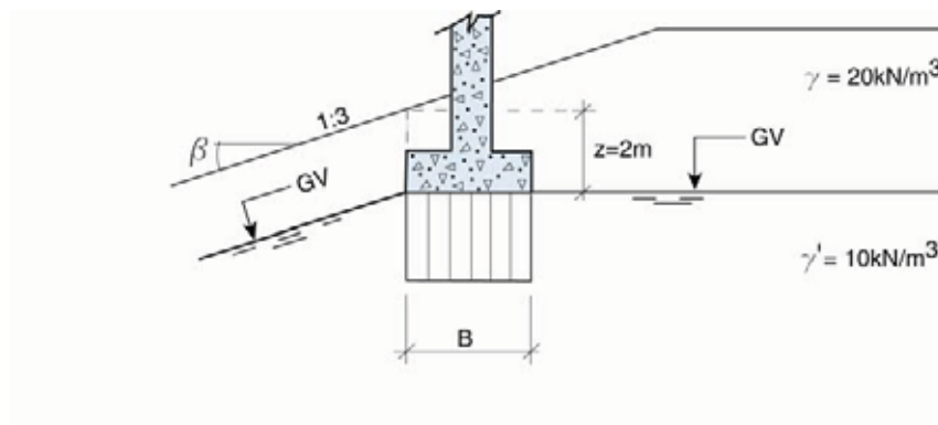
Figur 6.15 Langstrakt fundament i skrått terreng - effektivspenningsanalyse.
