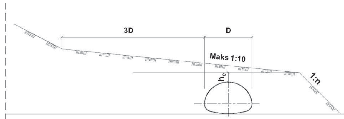
Figur 12.21 Krav til avstand fra rørkonstruksjonen til brattere terrenghelning
