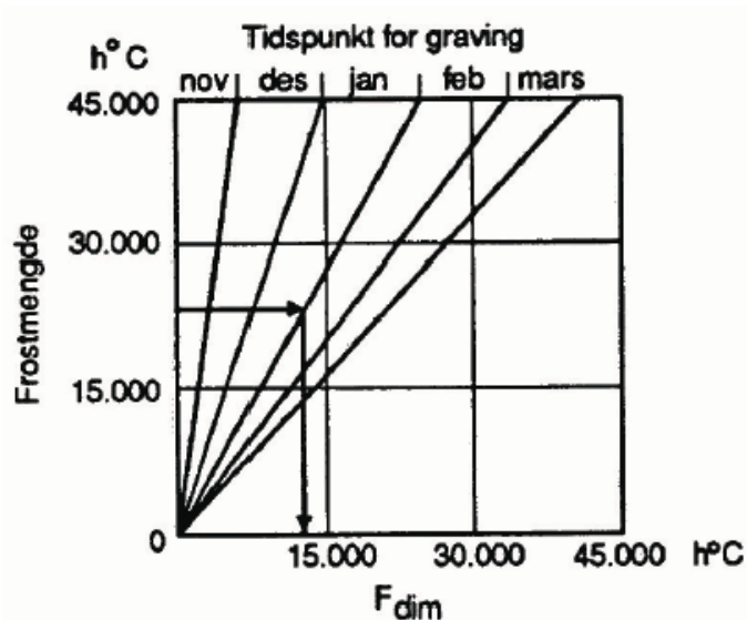
Figur 13.31 Bestemmelse av F_{dim} ut fra frostmengde og valgt tidsperiode (fra Hb 018, 2005)
