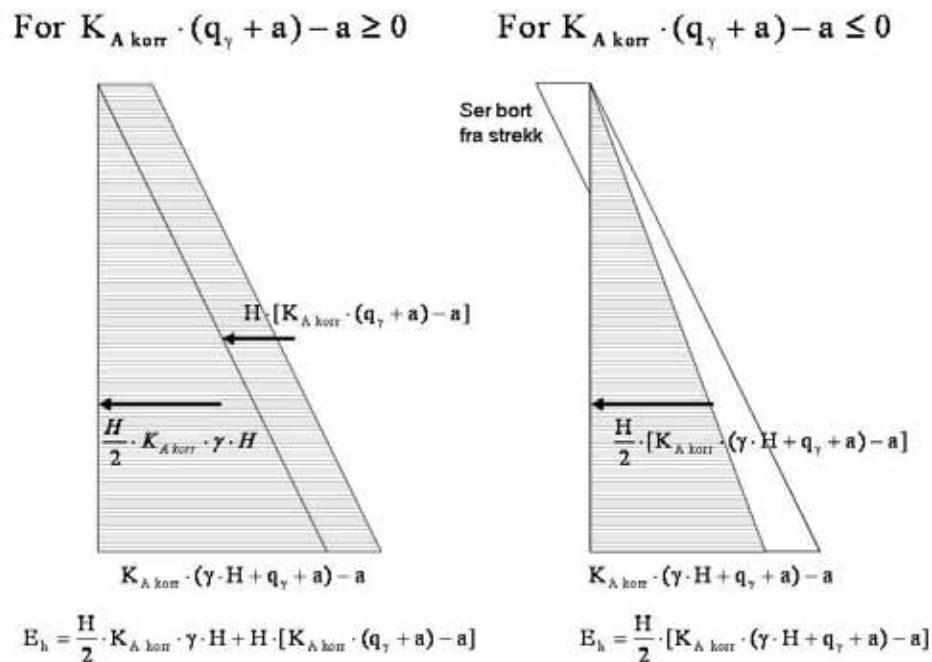
Figur 9.8 Jordtrykk mot tørrmur avhengig av q_\gamma og attraksjonens størrelse
