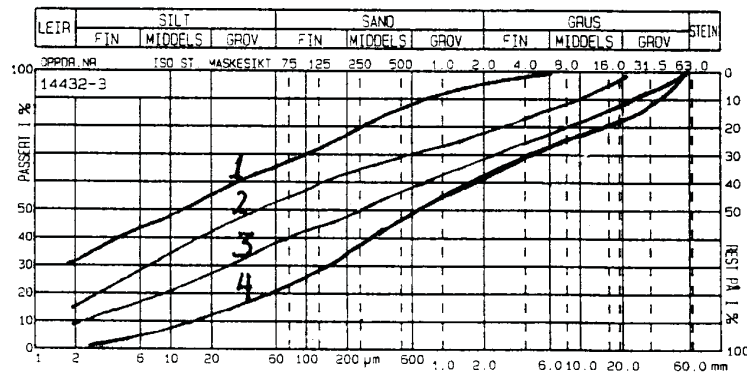
Figur 3.8 Sikteturver i bunnmorene. 1: Moreneleire, breen har beveget seg over marine, finstoffrike avsetninger. 2: Morene av svake, glimmerrike bergarter (fyllitt og glimmerskifer). 3: Morene av harde gneisbergarter. 4: Morene av hovedsakelig granitt.
