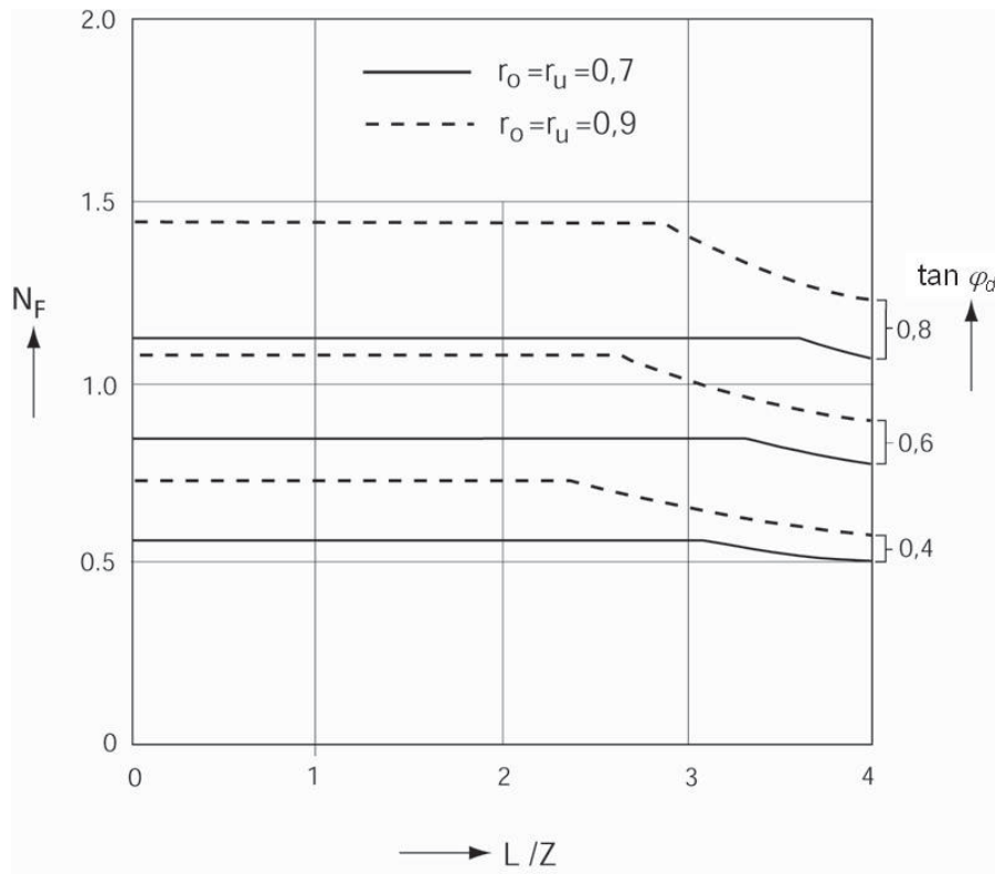
Figur 9.13 Friksjonsfaktor N_F for friksjonsplate (Døsland 1980 videreutviklet for Hb 016).
