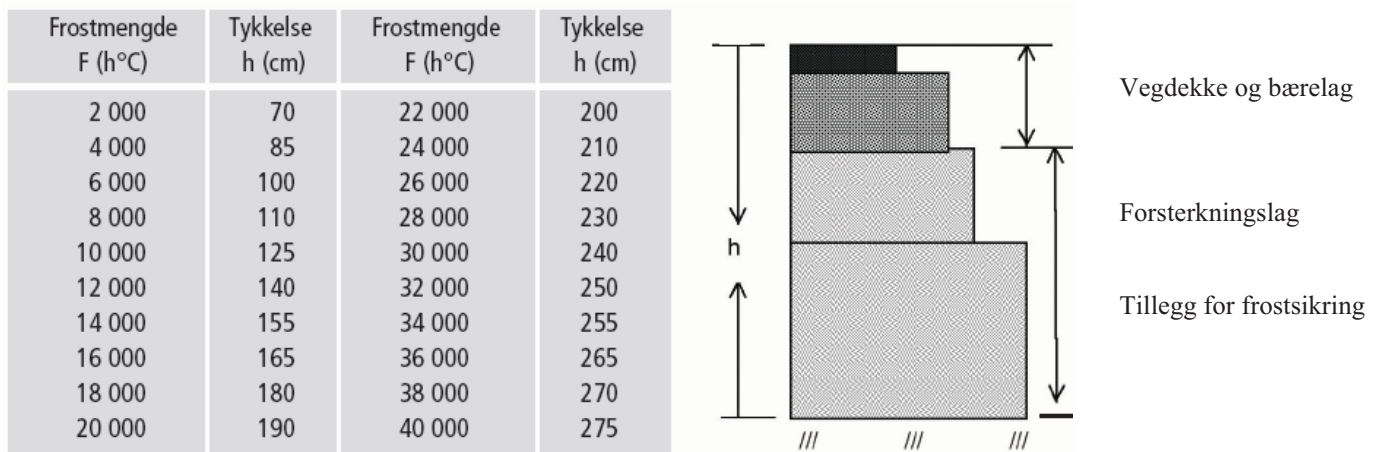
Figur 13.17 Tabell for frostsikring av veger med sand, grus og stein (fra Hb 018, 2005).
