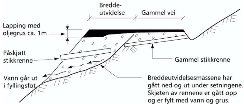
Figur 14.22 Bredeutvidelse med påfølgende brudd på stikkrenne.
