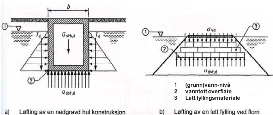
Figur 15.2 Krefter som påvirker konstruksjoners stabilitet mot oppløfting
