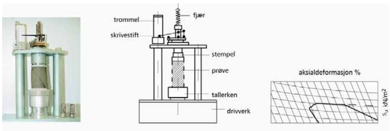
Figur 2.9 Enaksialt trykkapparat.
