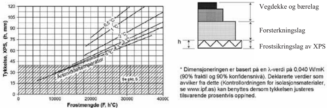
Figur 13.19 Frostteknisk dimensjonering med isolasjonsplater av ekstrudert polystyren XPS (fra Hb 018, 2005)
