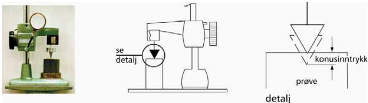
Figur 2.11 Konusapparat
