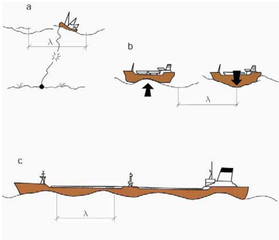
Figur 17.3 Bølgelengdens betydning
