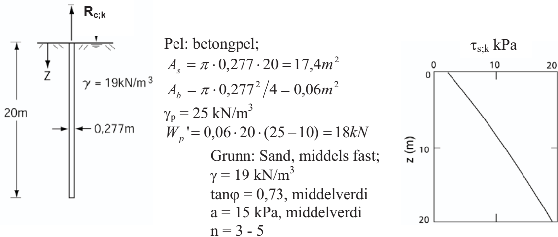
Figur 11. 14 Eksempel - strekkpel
