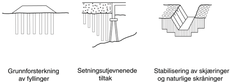
Figur 15.8 Kalk- / sementpelers anvendelsesområder.
