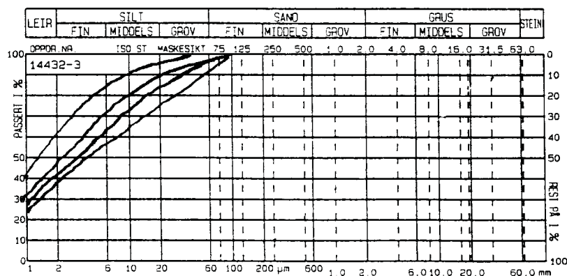
Figur 3.16 Siktekurver i hav- og fjordavsetninger.
