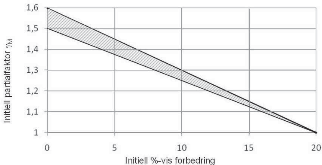
Figur 0.4 Krav til %-vis forbedring av stabilitetsforhold ved totalspenningsanalyse
