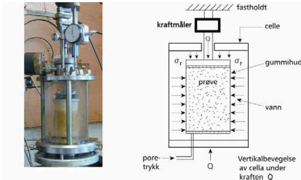
Figur 2.19 Prinsippskisse av trekselle
