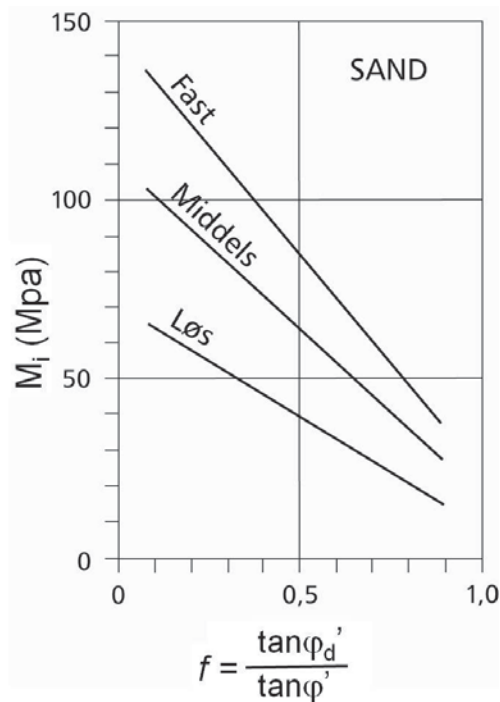
Figur 2.45 Inital deformasjonsmodul for sand
