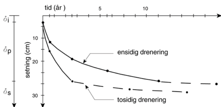
Figur 7.21 Tidsforløp - overslag.
