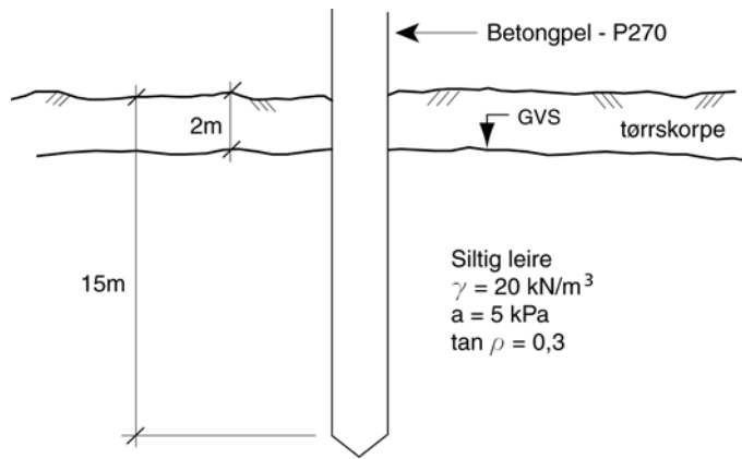
Figur 13.35 Betongpel i frossen jord.
