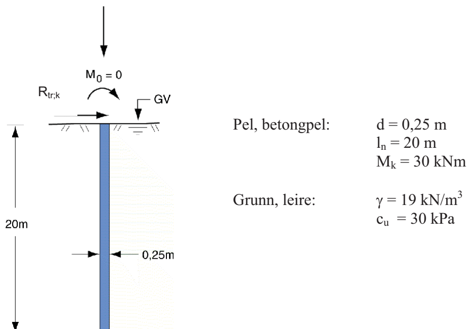
Figur 11. 25 Eksempel - friksjonspil i leire, horisontal bæreevne korttidsbelastning
