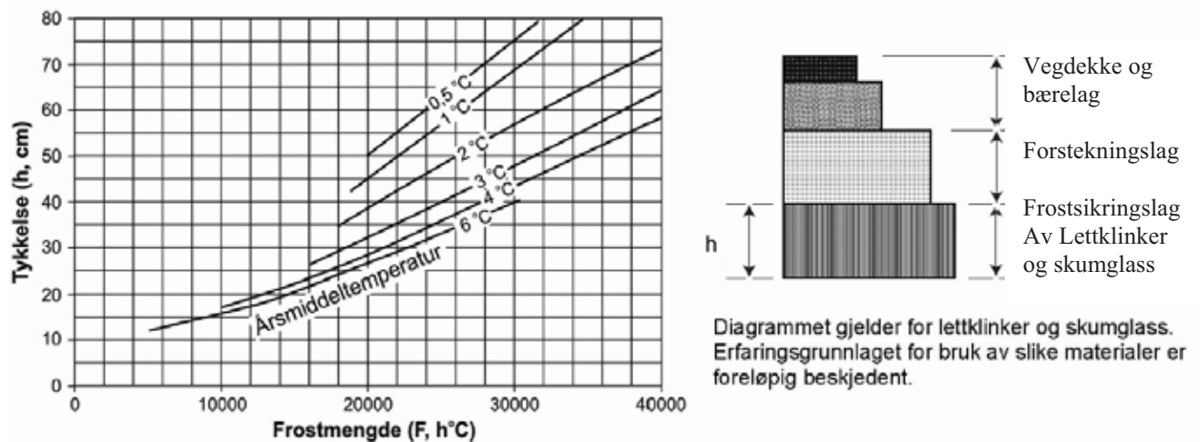
Figur 13.18 Frostteknisk dimensjonering av frostsikringslag med lettklinker og skumglass (fra Hb 018, 2005)
