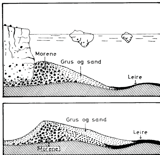
Figur 3.3: Øverst: Raet under dannelse der iskanten lå i havet. Isen skyver sammen en rygg av løsmateriale på sjøbunnen, samtidig som smeltevatn avsetter grus, sand og leire. Nederst: Landhevingen løfter Raryggen opp til havnivå der den jevnes ut av bølgene. (Østerås 1974, Ref. 22)
