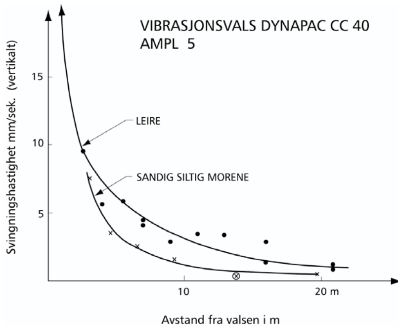
Figur 17.18 Målt svingningshastighet ved vibrering med 10 t vibrerende tandemvals (fra Appelftoft et al. ).
