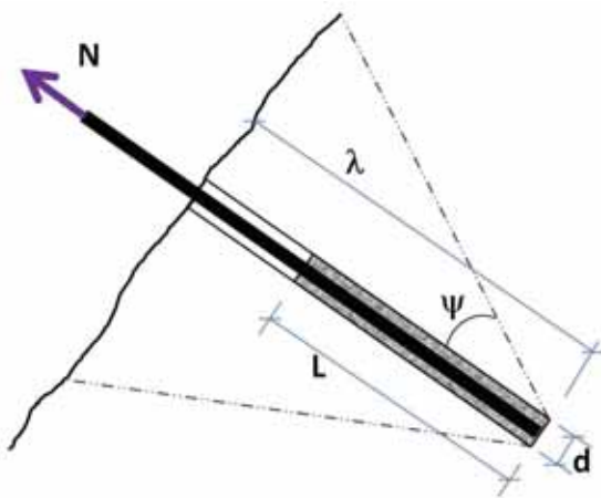
Figur 10. 35 Nødvendig forankringslengde \lambda og L i berg.
