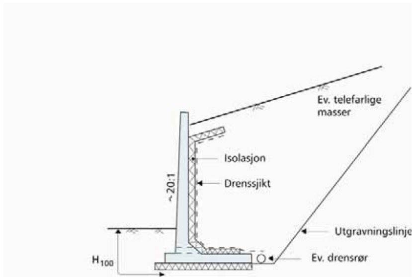
Figur 13.24 Frostsikring med isolasjonsplater.
