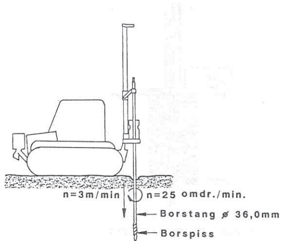
Figur 1.9 Dreietrykksondering.
