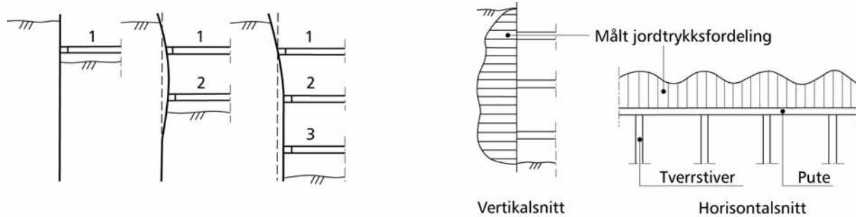
A. Figur 10. 9 a) Prinsippskisse av deformasjoner ved forskjellige gravestadier. B. b) Målt jordtrykksfordeling langs veggen.
