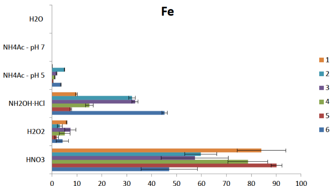
Figur 11: Mobilitet av Fe etter sekvensiell ekstraksjon på ulike bergartar frå Gran.
